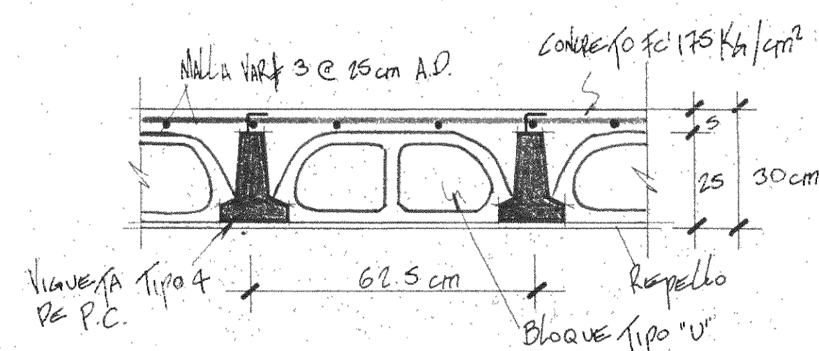
DET. DE ENTREPISO sin escala
