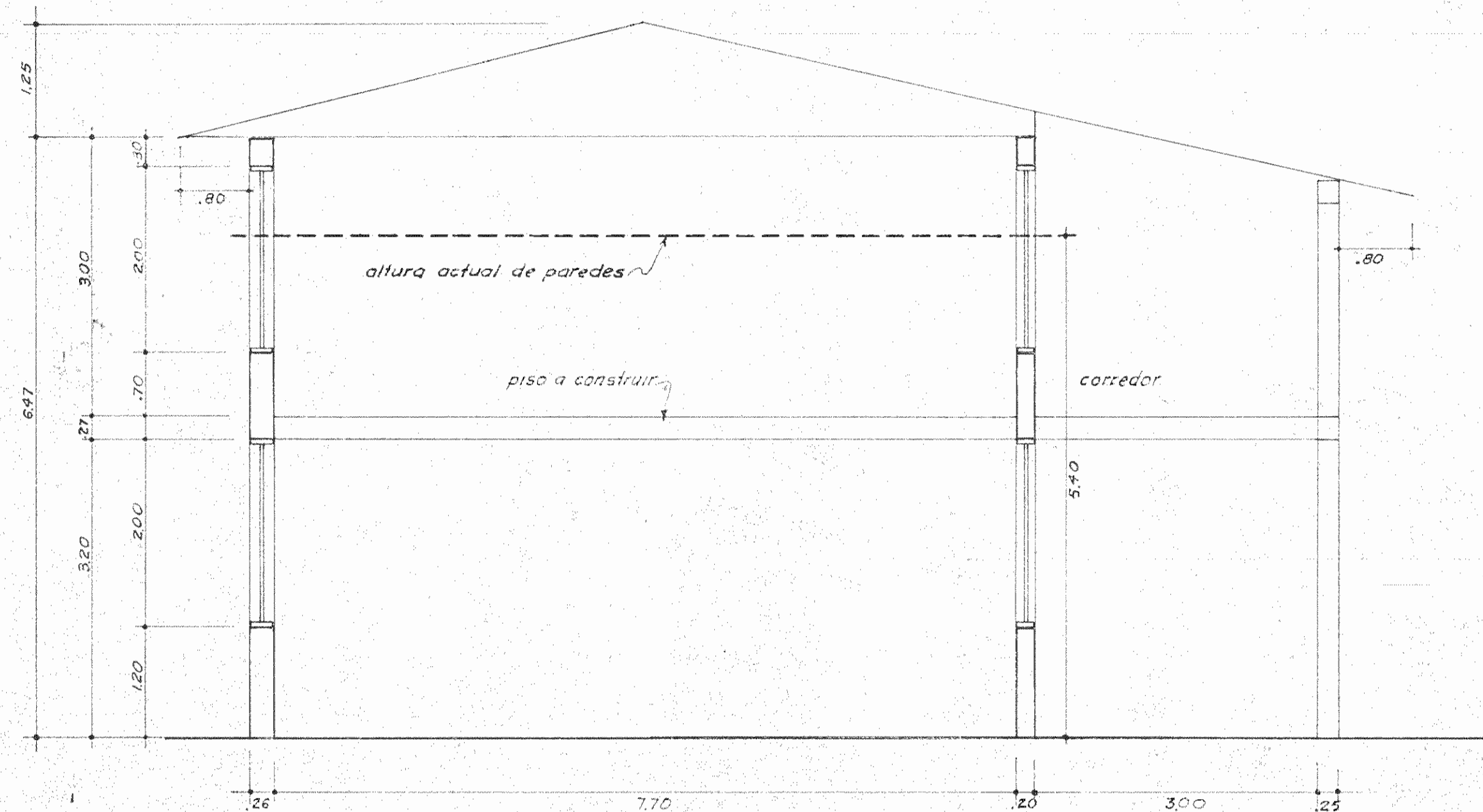
corte 1=50
