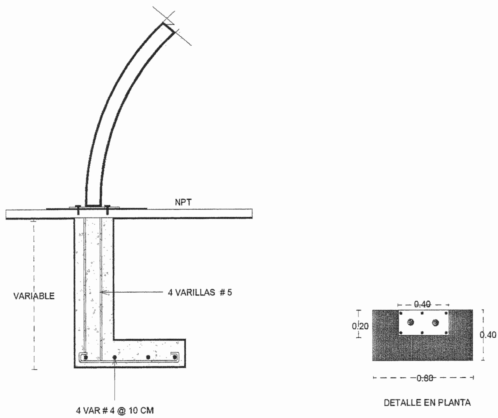
DETALLE DE PEDESTAL
