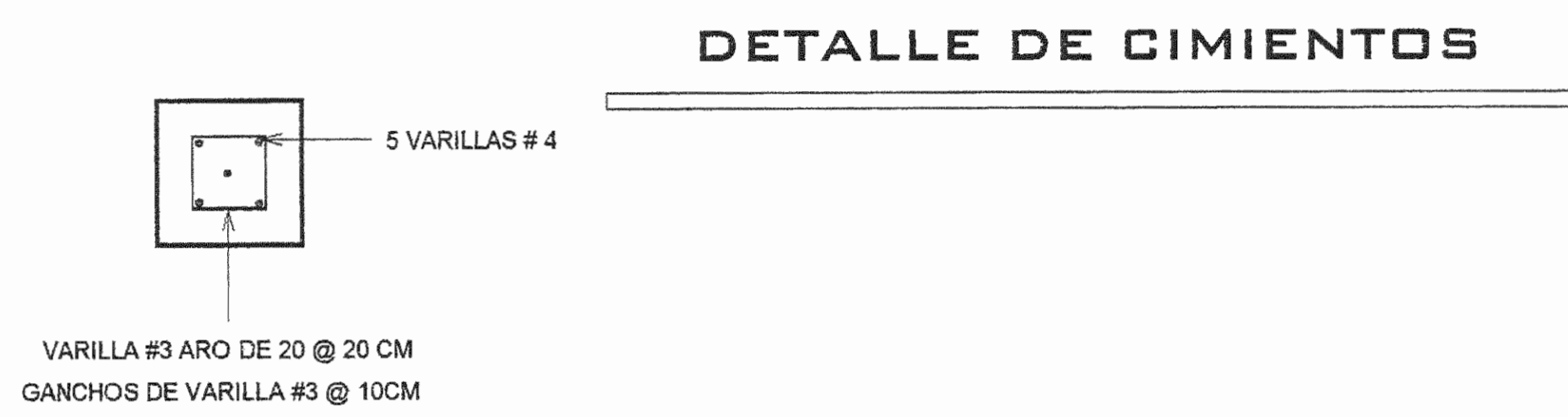
DETALLE DE CIMIENTOS
