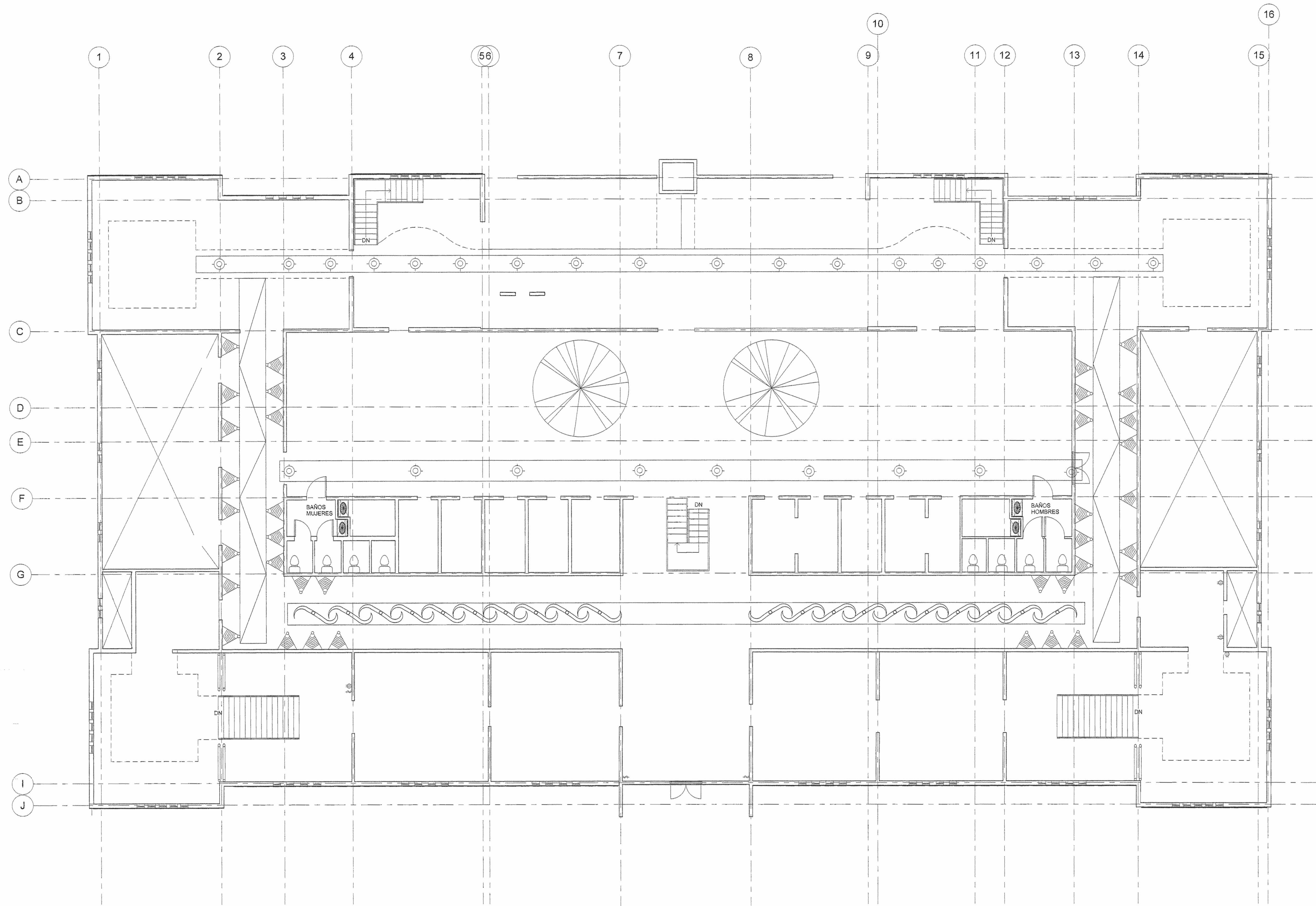
PLANTA ILUMINACION Y REDES SEGUNDO NIVEL
