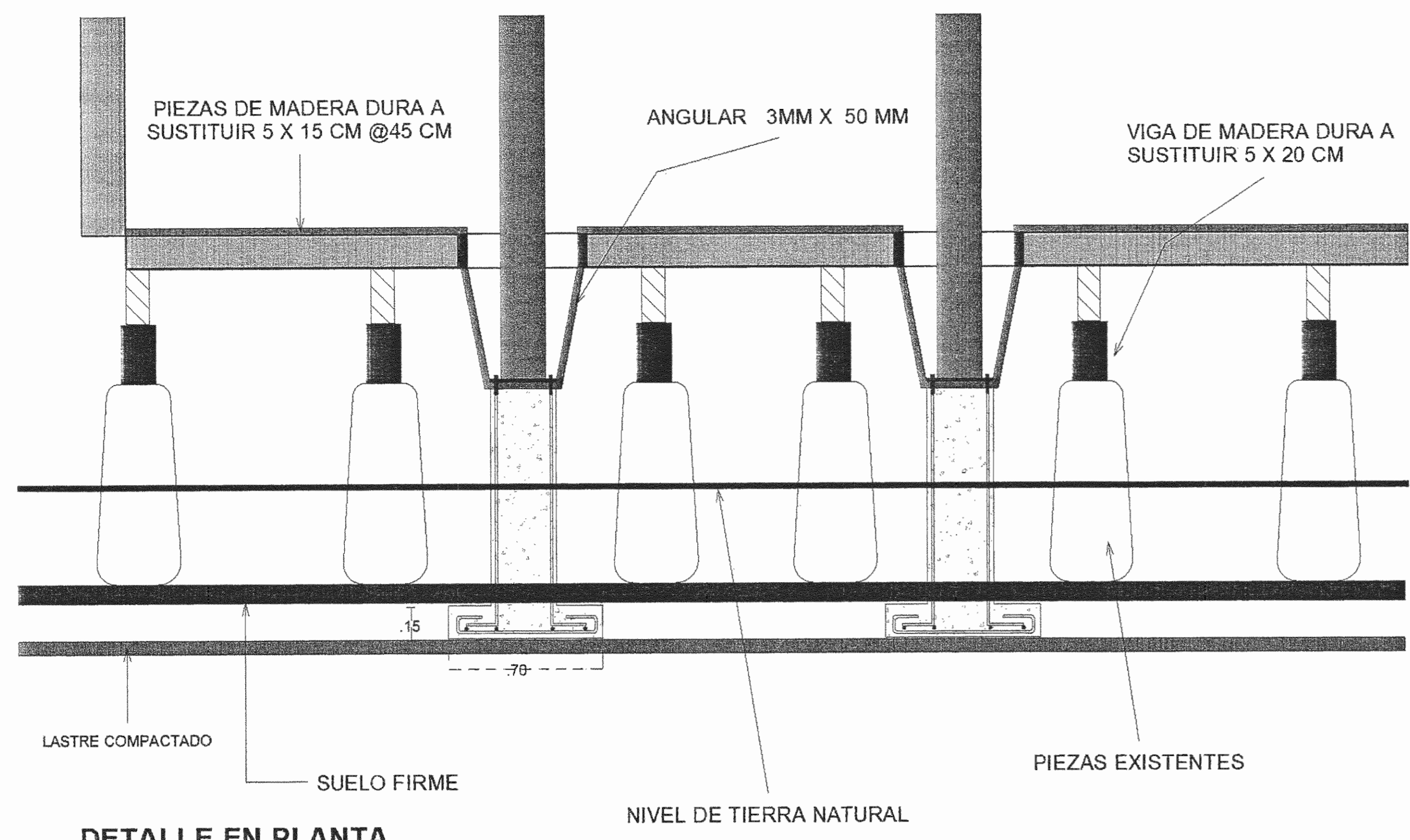
DETALLE EN PLANTA
