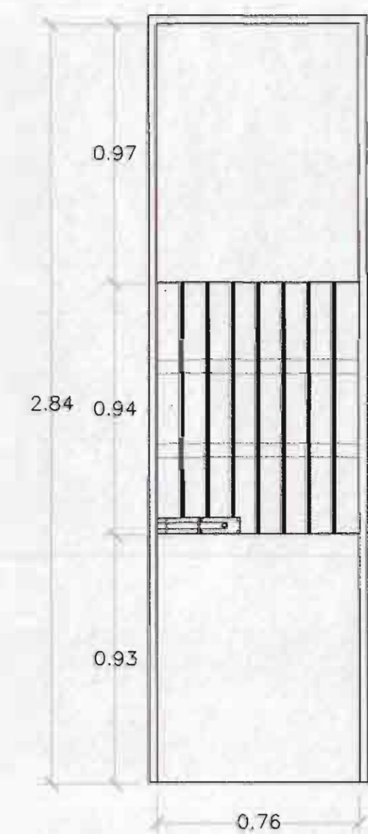
DETALLE DE PUERTAS TIPO B ESCALA 1:20
