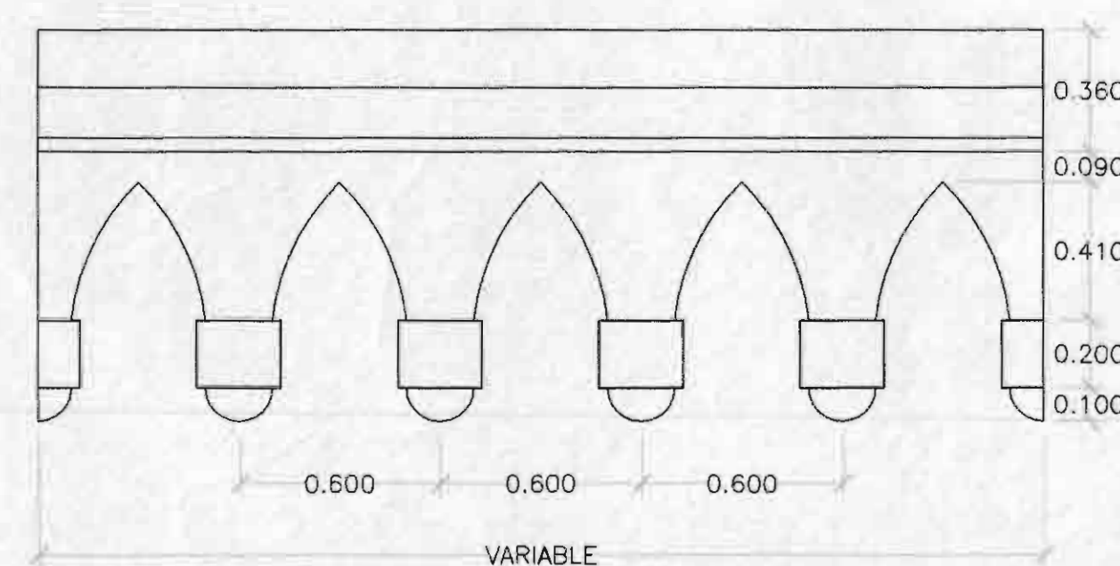
DETALLE DECORADO TIPO 2 ESCALA 1:20
