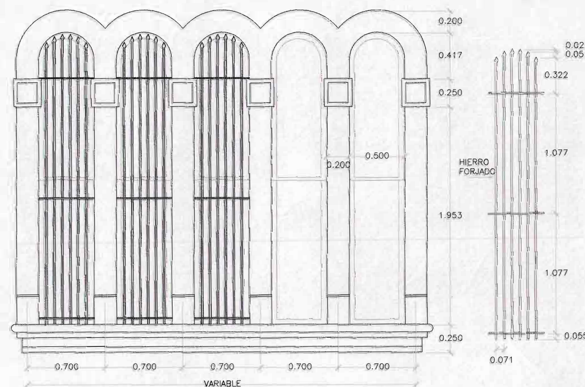
DETALLE DE REJAS VENTANAS TIPO 2 ESCALA 1:20
