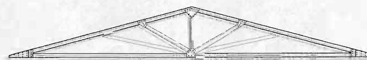
VISTA FRONTAL DE CONJUNTO ESTRUCTURAL DE CERCHAS DEL TORRION TIPO 2 ESCALA 1:50
