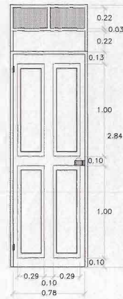
DETALLE DE PUERTAS TIPO C ESCALA 1:20
