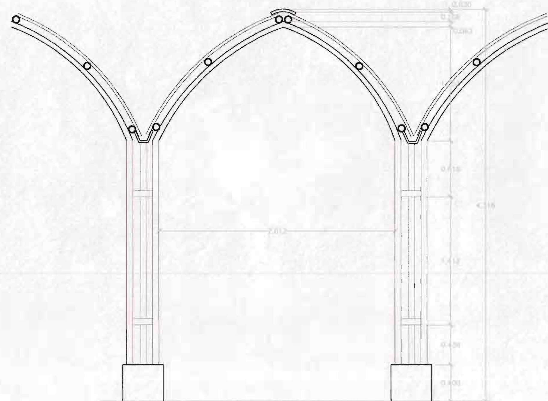
DETALLE DE ARCO METALICO ESCALA 1:25
