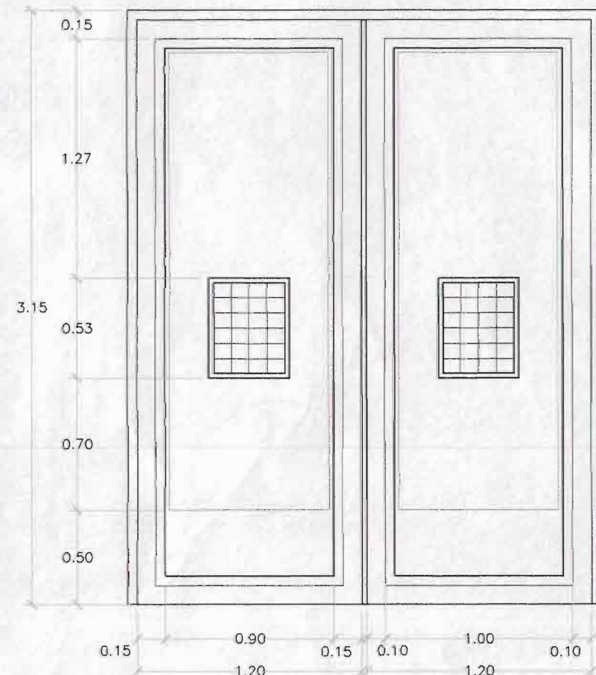
DETALLE DE PUERTAS TIPO A ESCALA 1:20
