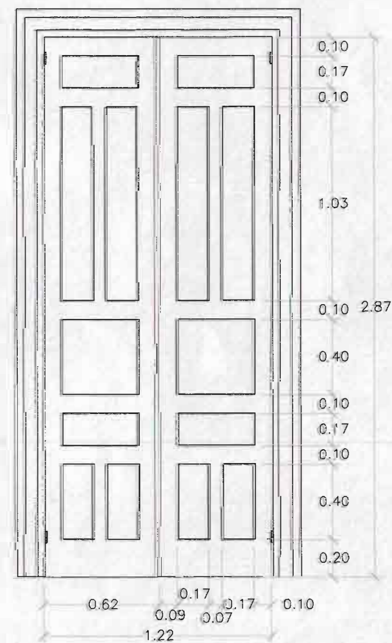
DETALLE DE PUERTAS TIPO E ESCALA 1:20
