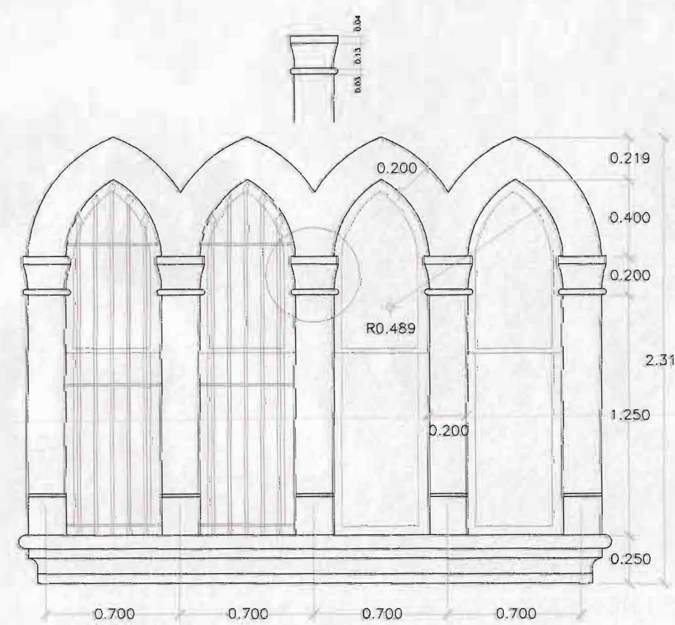
DETALLE DE VENTANAS TIPO 1 ESCALA 1:20
