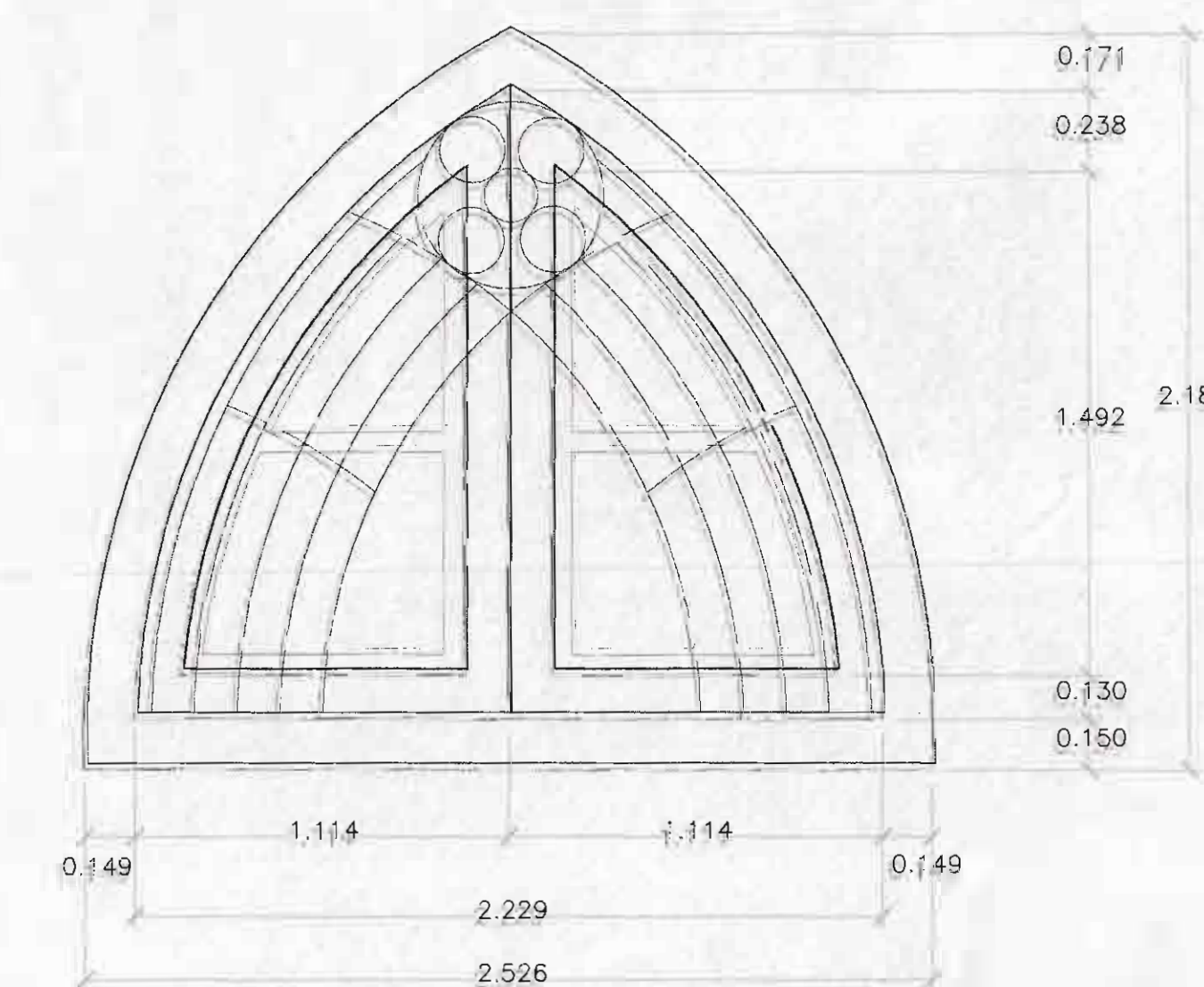
DETALLE DE VENTANA TIPO 3 ESCALA 1:20
