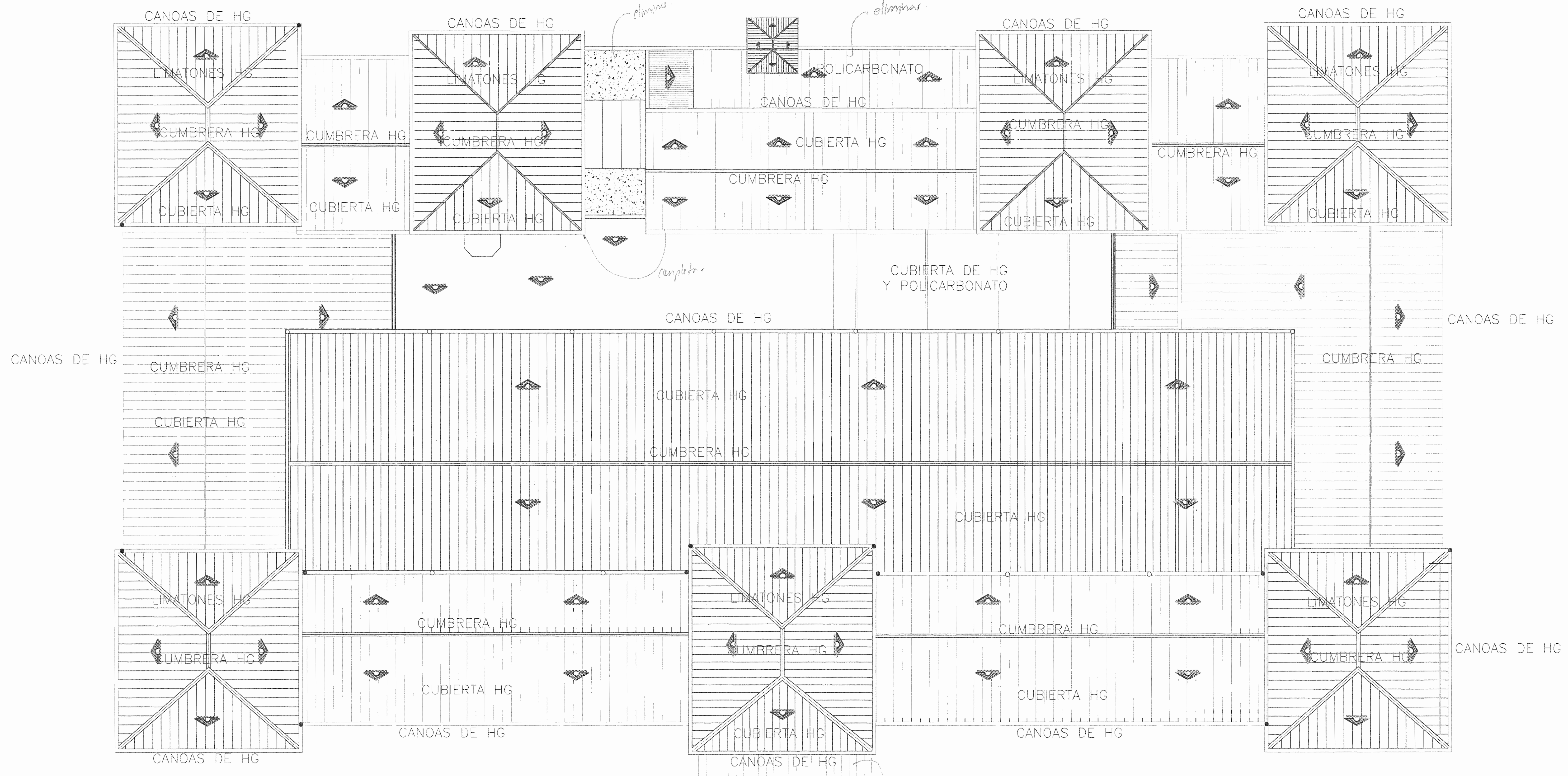
PLANTA DE DISTRIBUCION DE CUBIERTAS . ESC 1:75
