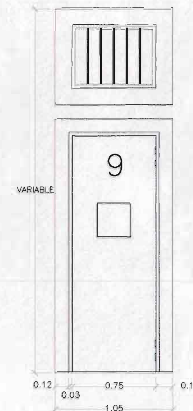
DETALLE DE PUERTAS TIPO D ESCALA 1:20
