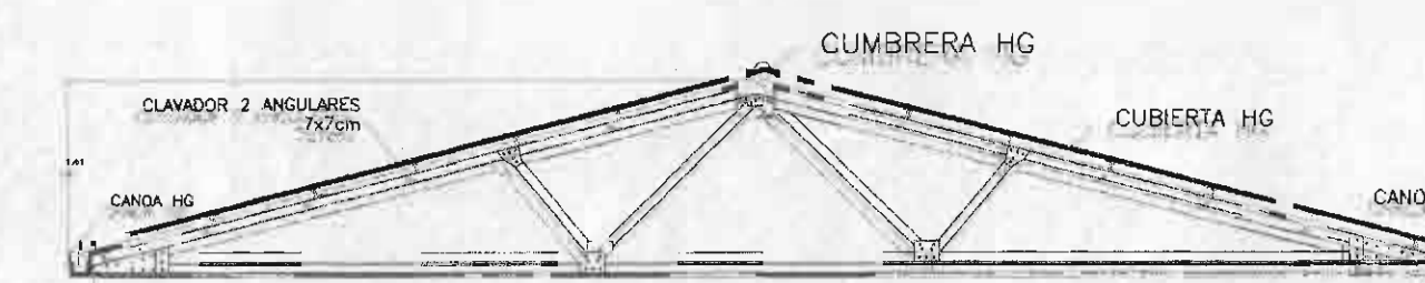
DETALLE DE CERCHAS TIPO 1 ESCALA 1:75
