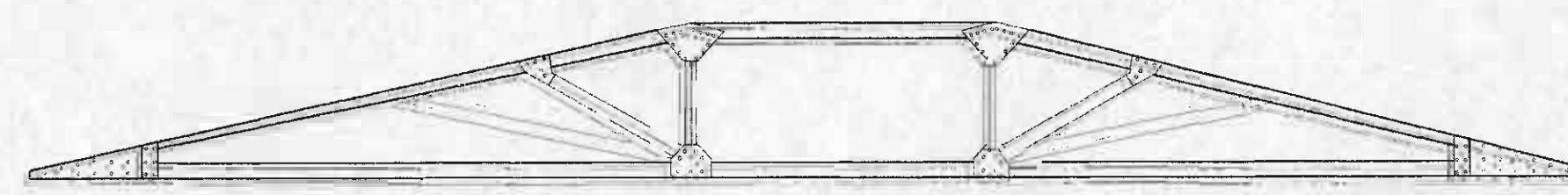
VISTA LATERAL DE CONJUNTO ESTRUCTURAL DE CERCHAS DE TORRIONES TIPO 1 ESCALA 1:50
