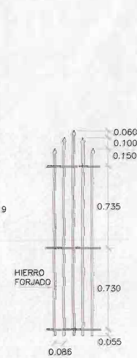
DETALLE DE REJAS VENTANAS TIPO 1 ESCALA 1:20
