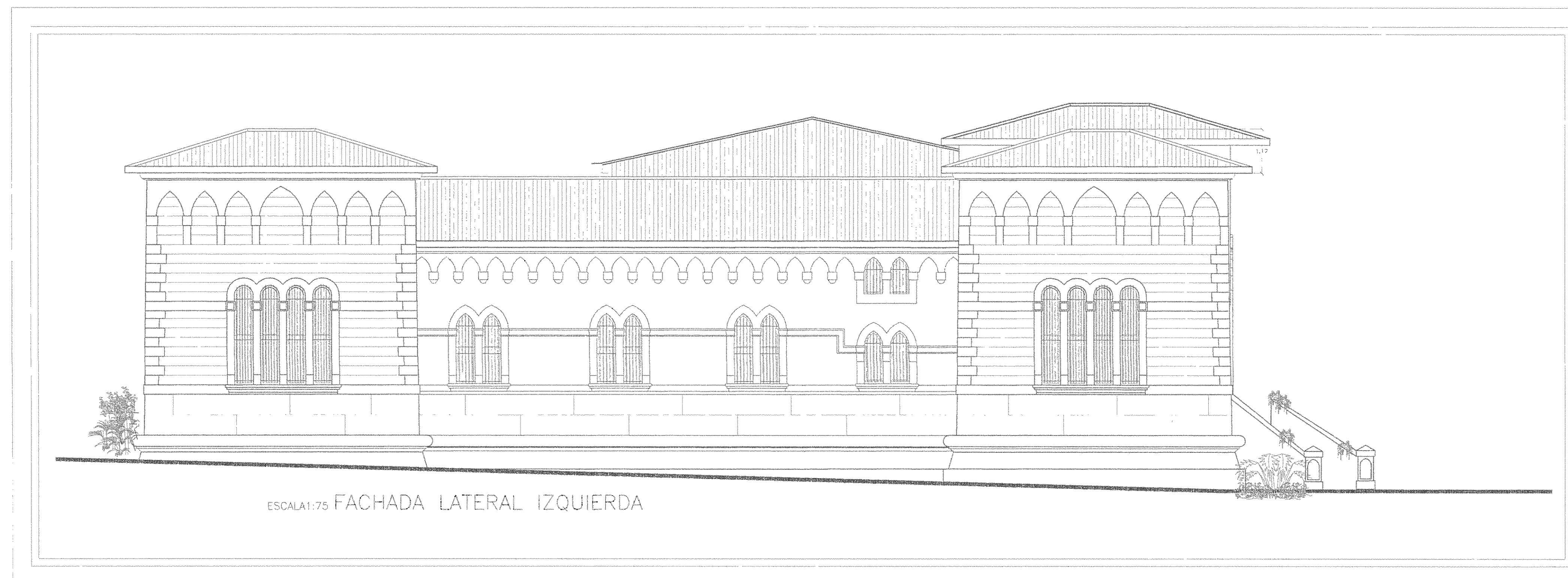
FACHADA LATERAL DERECHA EDIFICACION ANTIGUA. ESC 1:75
