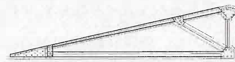
COMPONENTE BASICO DE CONJUNTO ESTRUCTURAL DE CERCHAS DE TORRION TIPO 3 ESCALA 1:50
