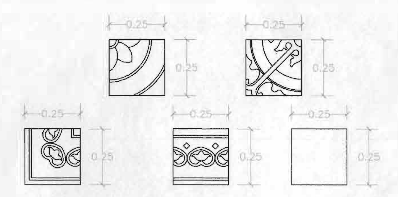
DETALES DE CADA CUADRANTE DE MOSAICO ORIGINAL ESCALA 1:10
