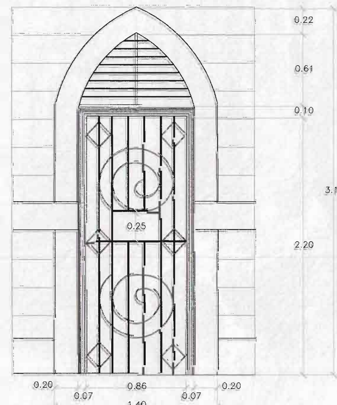
DETALLE DE PORTON TIPO A' ESCALA 1:20
