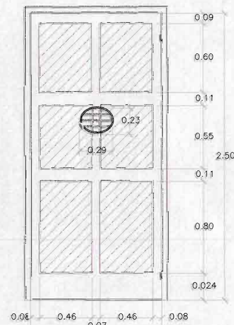
DETALLE DE PUERTAS TIPO F ESCALA 1:20
