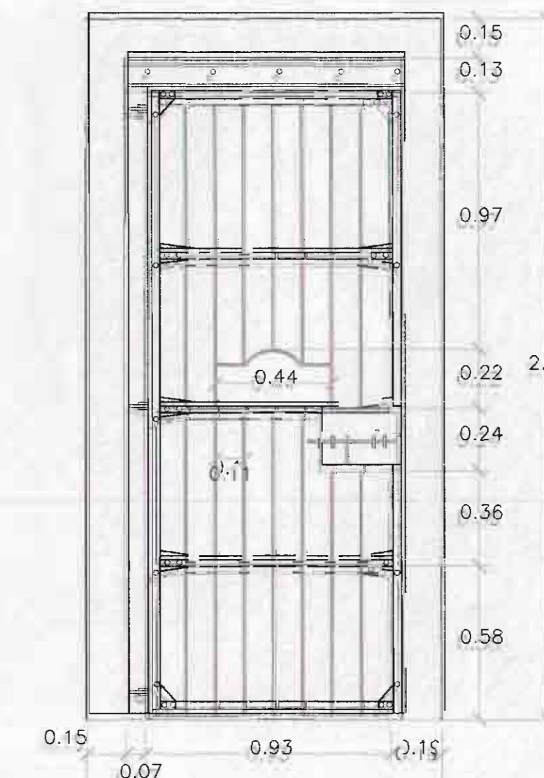
DETALLE DE PORTON TIPO B' ESCALA 1:20
