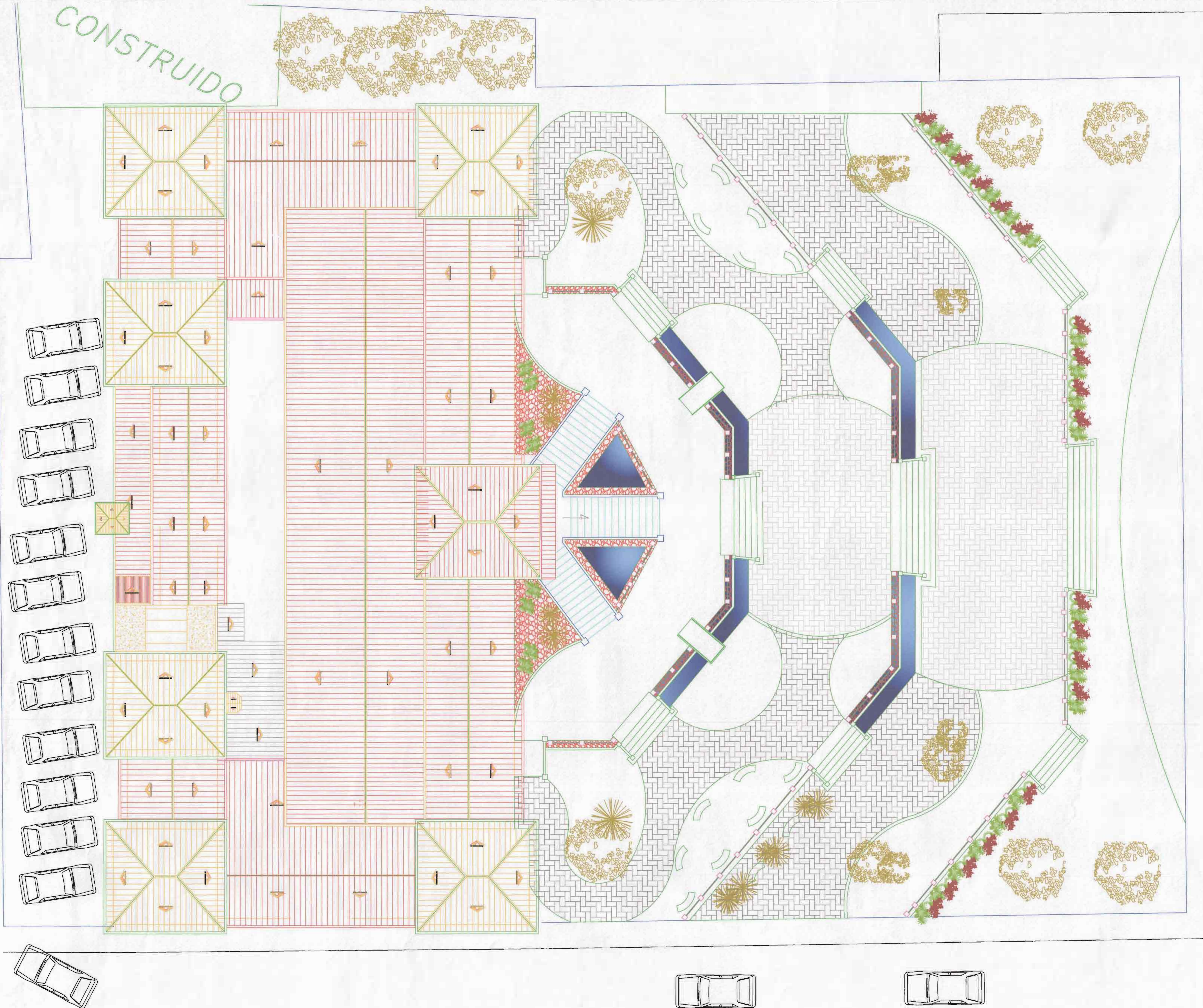
PLANTA DE PLAZOLETA EN CONJUNTO ESC 1:100
