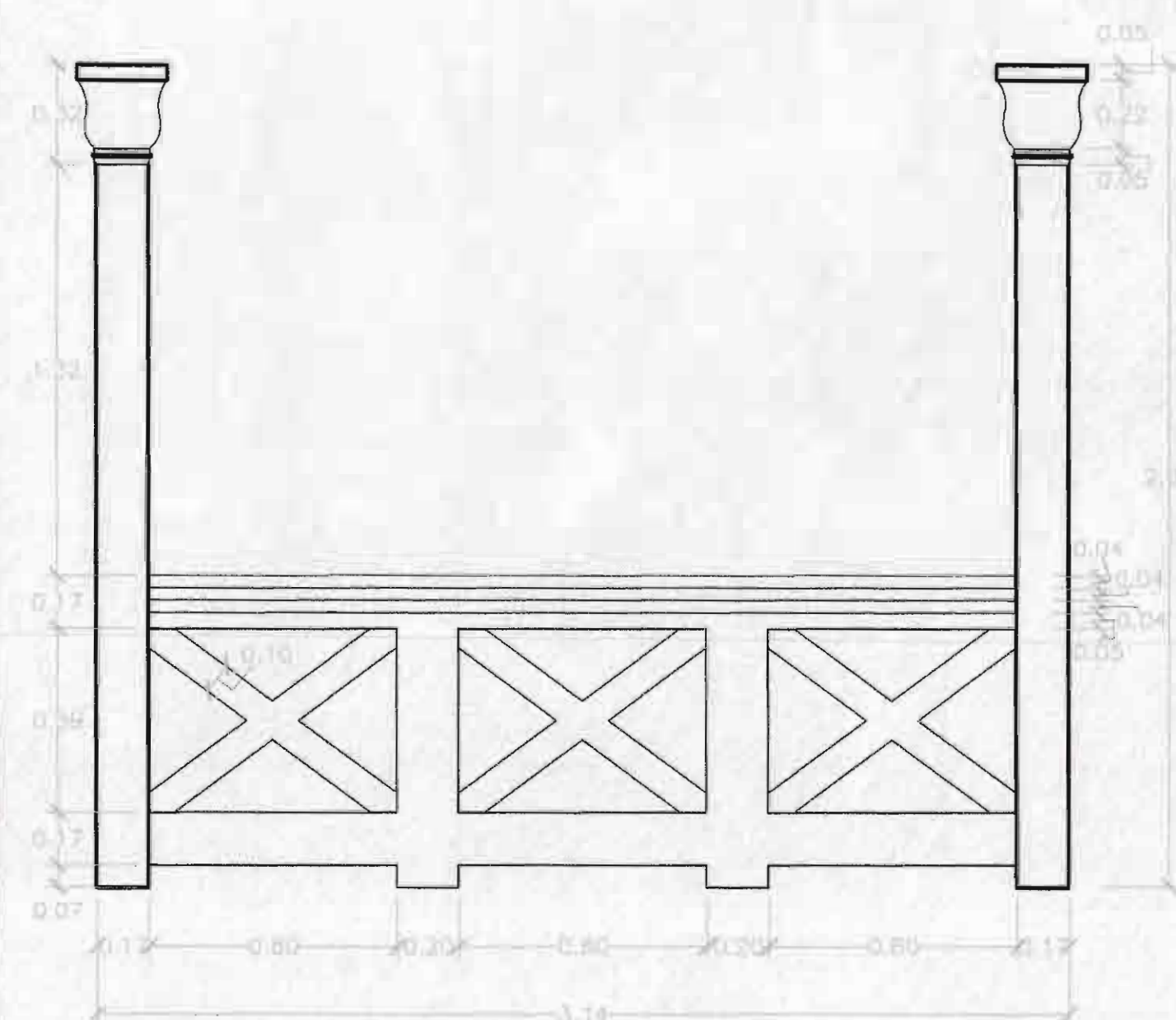
DETALLE DE BARANDA ESCALA 1:20
