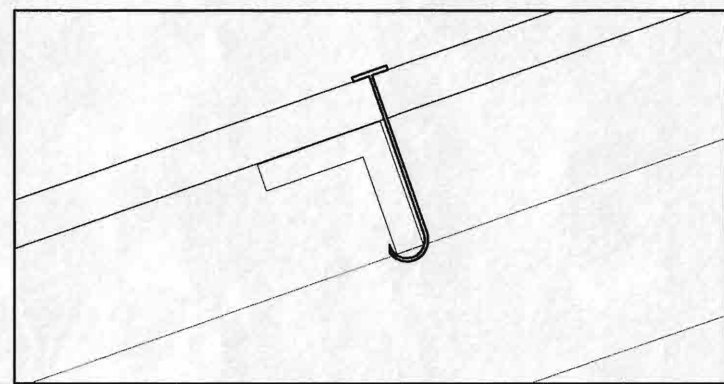
DETALLE DE ANCLAJE SIN ESCALA
