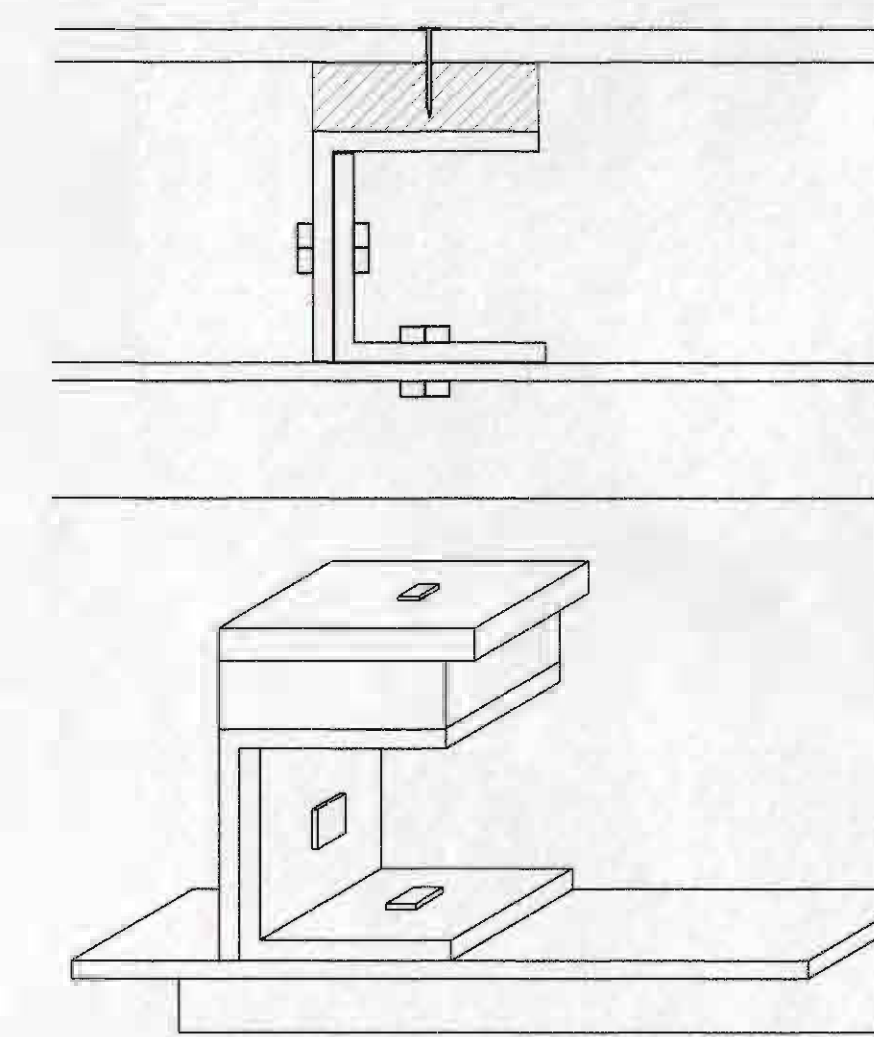
DETALLE DE ANGULARES
