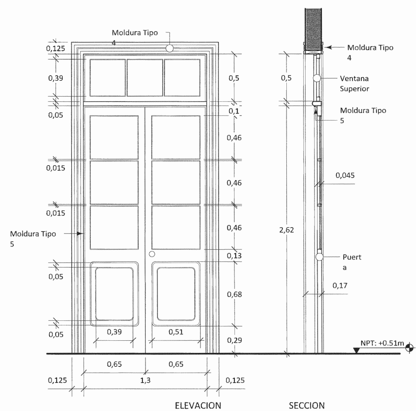
DETALLE DE PUERTA TIPICA Escala 1:25
