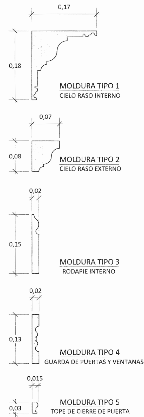
DETALLE DE MOLDURAS DE MADERA Escala 1:5
