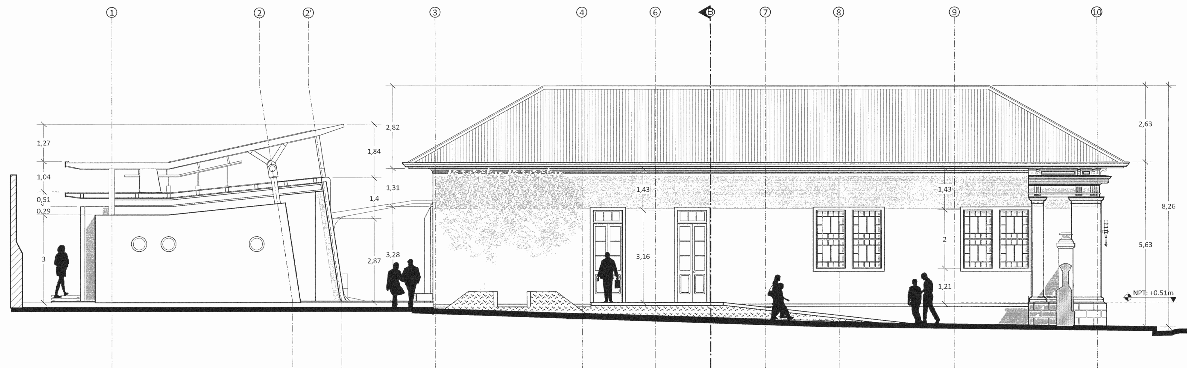
PROPUESTA - FACHADA OESTE Escala 1:75
