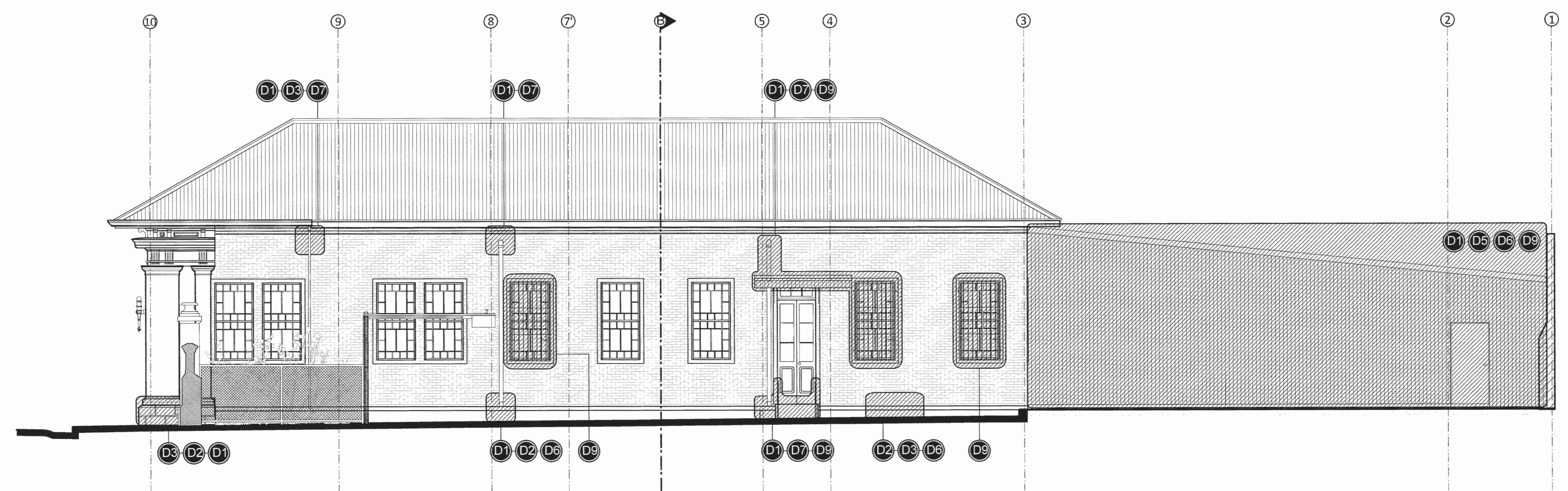
ACTUAL FACHADA ESTE / CONSIGNA DE DAÑOS Escala 1:75
