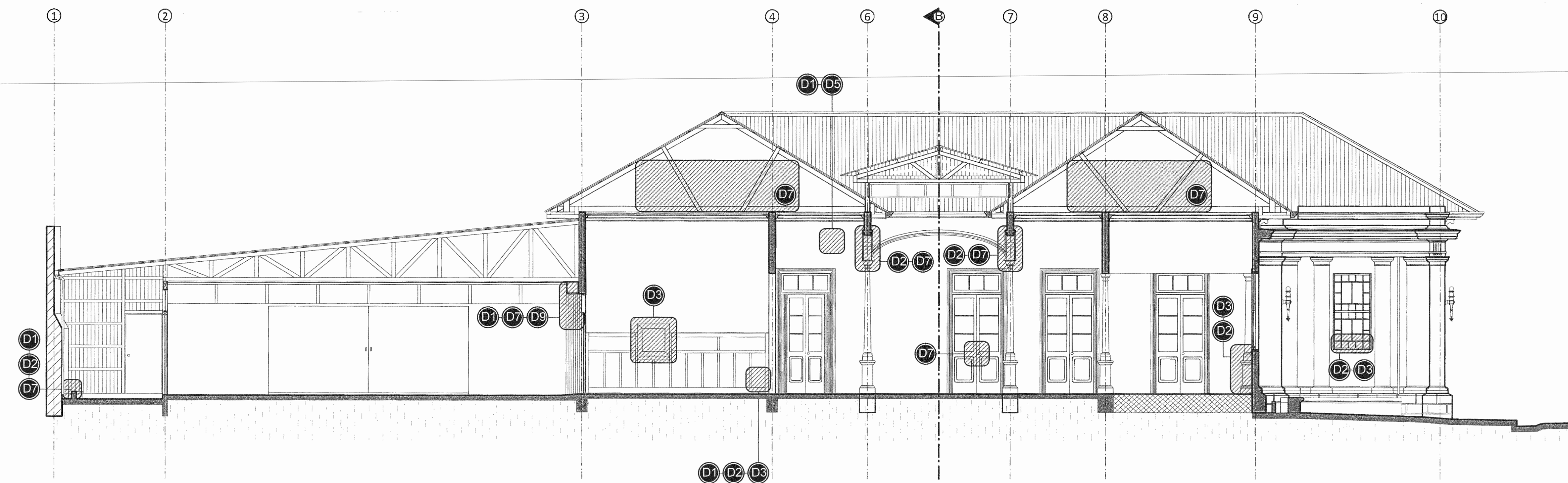
ACTUAL CORTE A - A / CONSIGNA DE DAÑOS Escala 1:75
