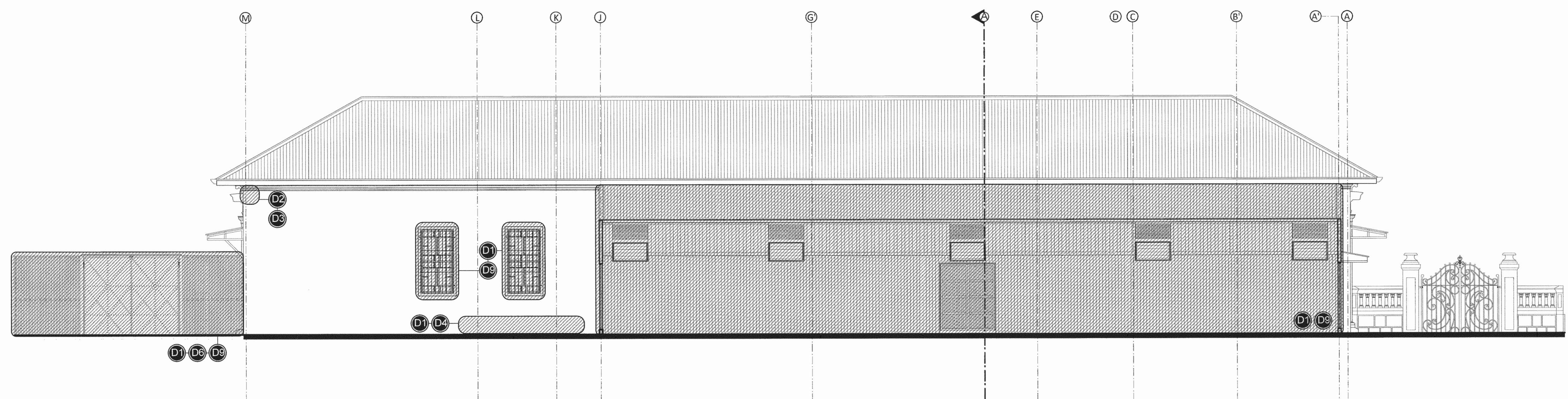
ACTUAL FACHADA - CORTE NORTE / CONSIGNA DE DAÑOS Escala 1:75
