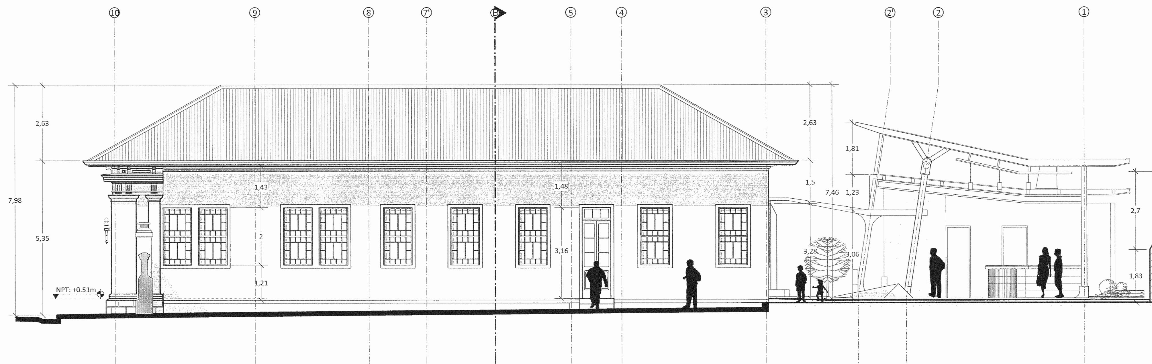
PROPUESTA - FACHADA ESTE Escala 1:75
