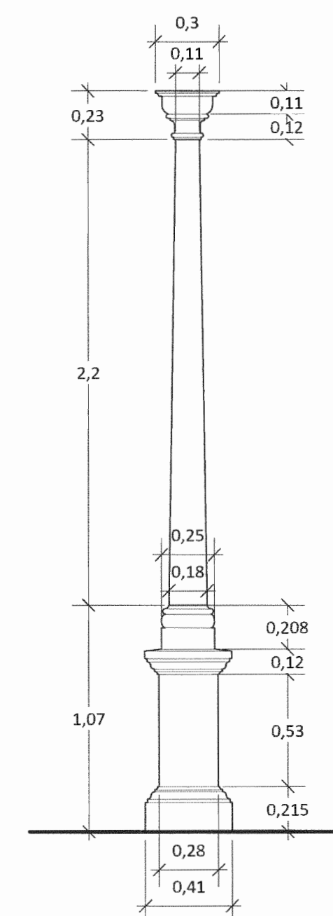
DETALLE DE COLUMNA TIPICA Escala 1:25
