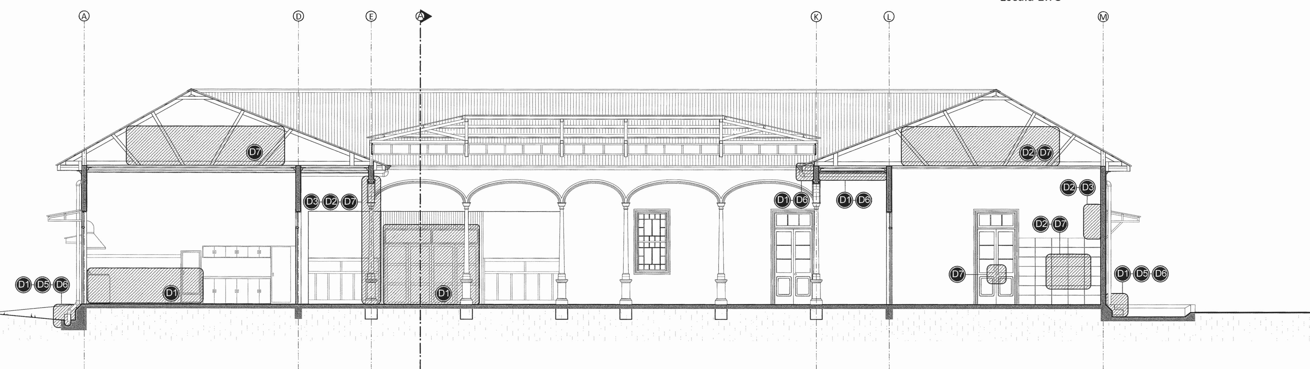
ACTUAL CORTE B - B / CONSIGNA DE DAÑOS Escala 1:75
