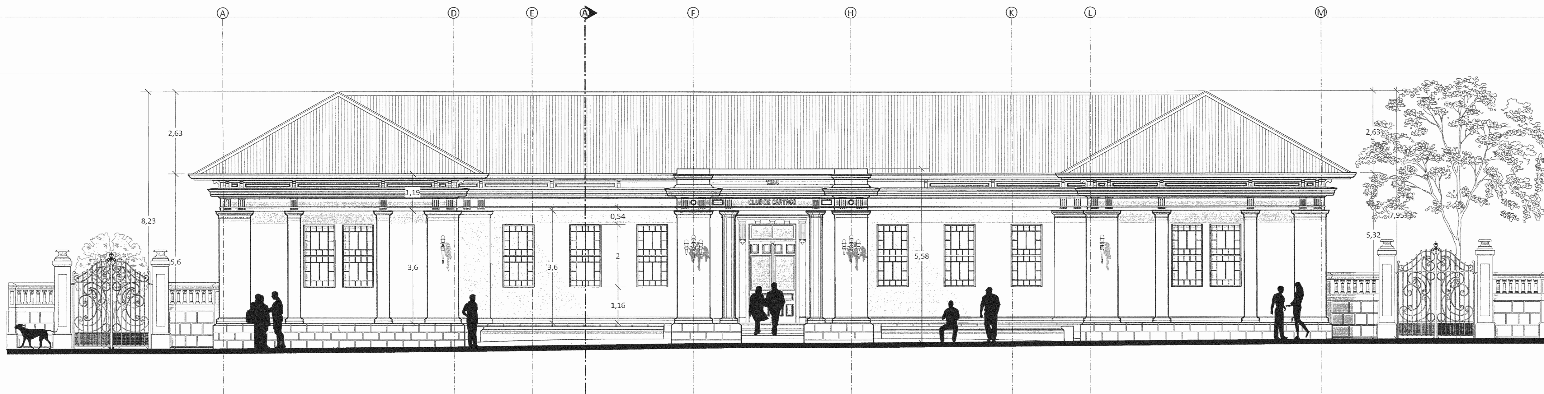
PROPUESTA - FACHADA PRINCIPAL Escala 1:75
