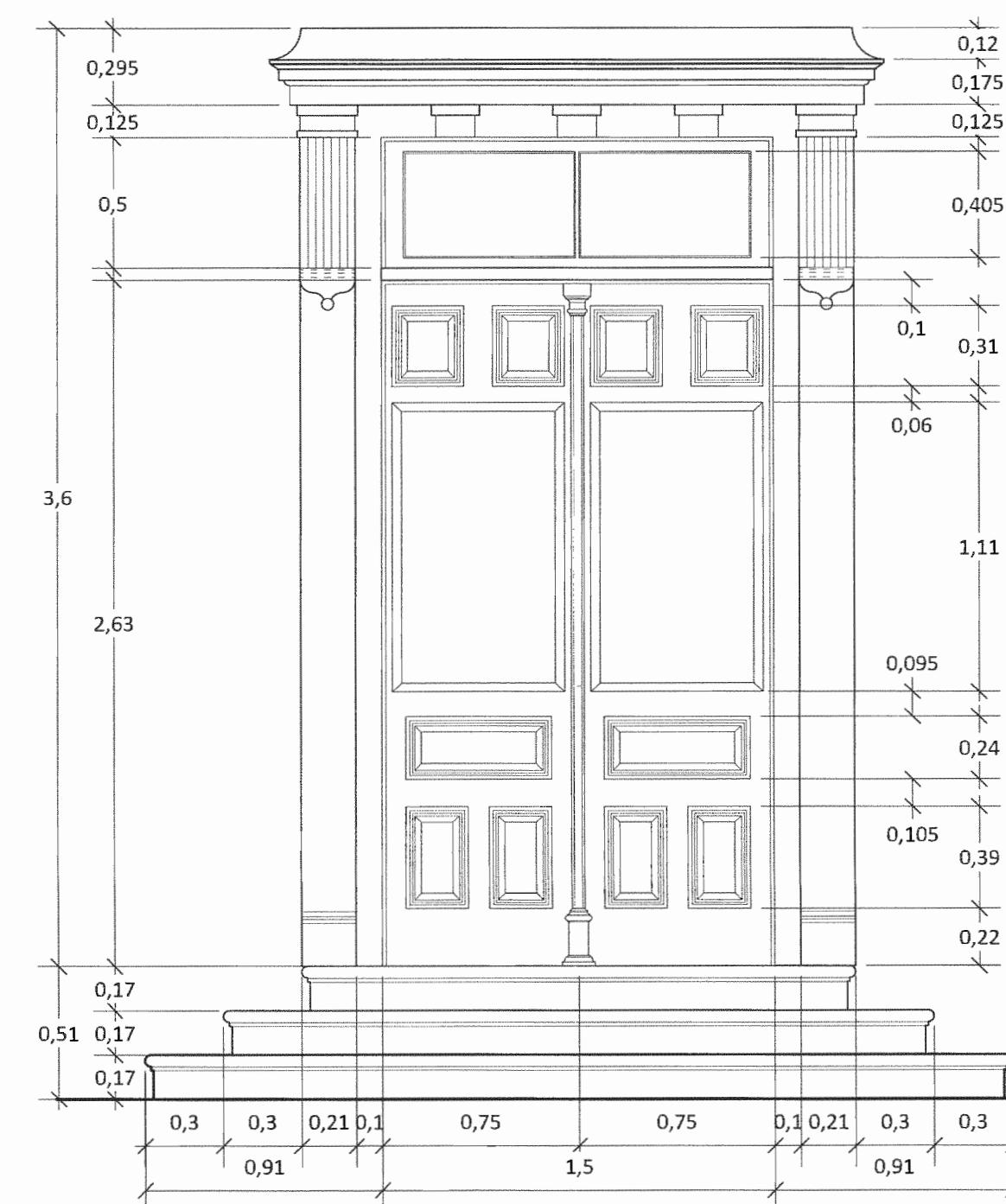
DETALLE DE PUERTA PRINCIPAL Escala 1:25
