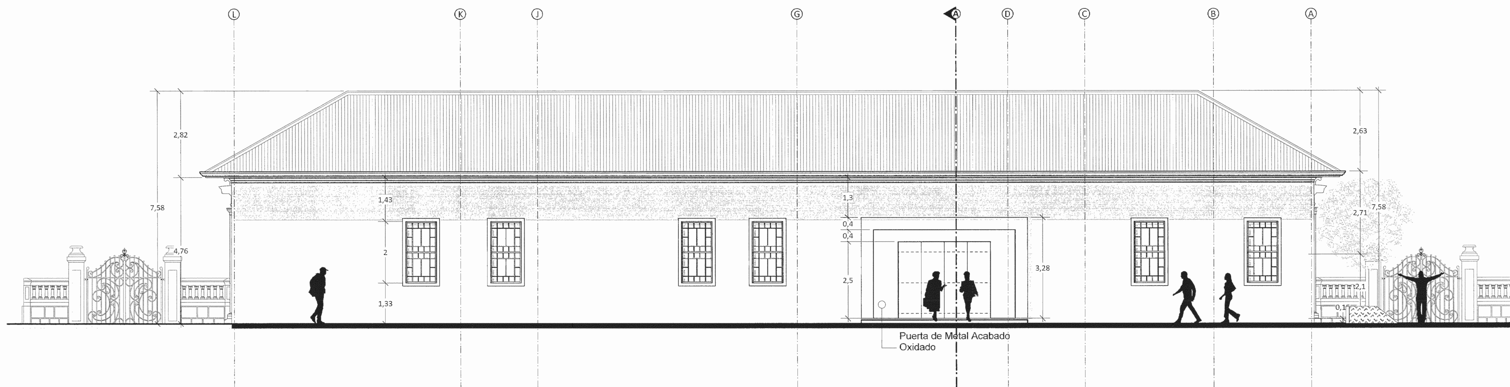
PROPUESTA - FACHADA NORTE Escala 1:75
