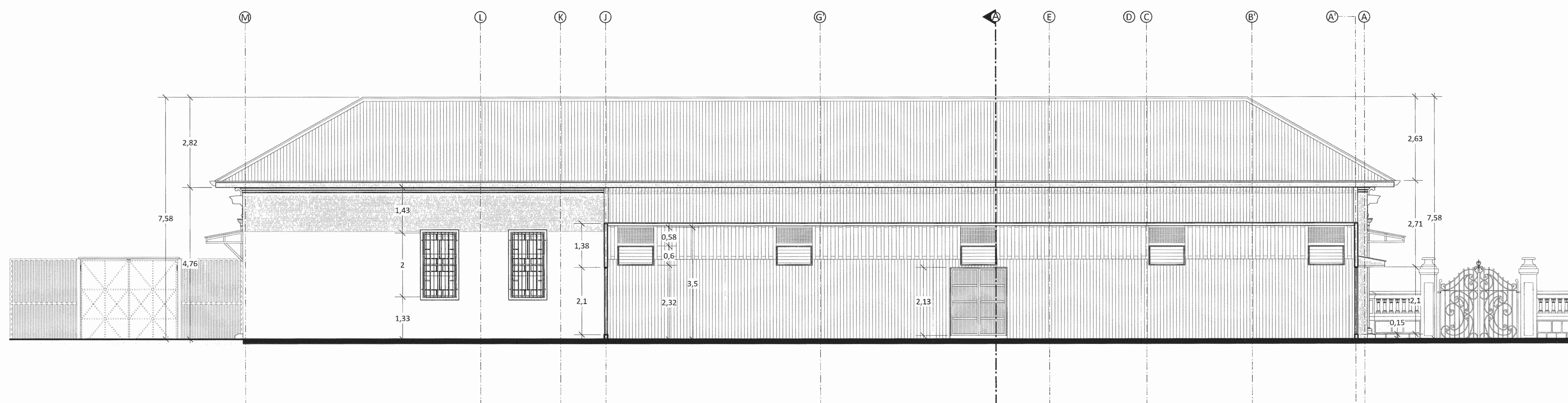
ACTUAL FACHADA - CORTE NORTE Escala 1:75
