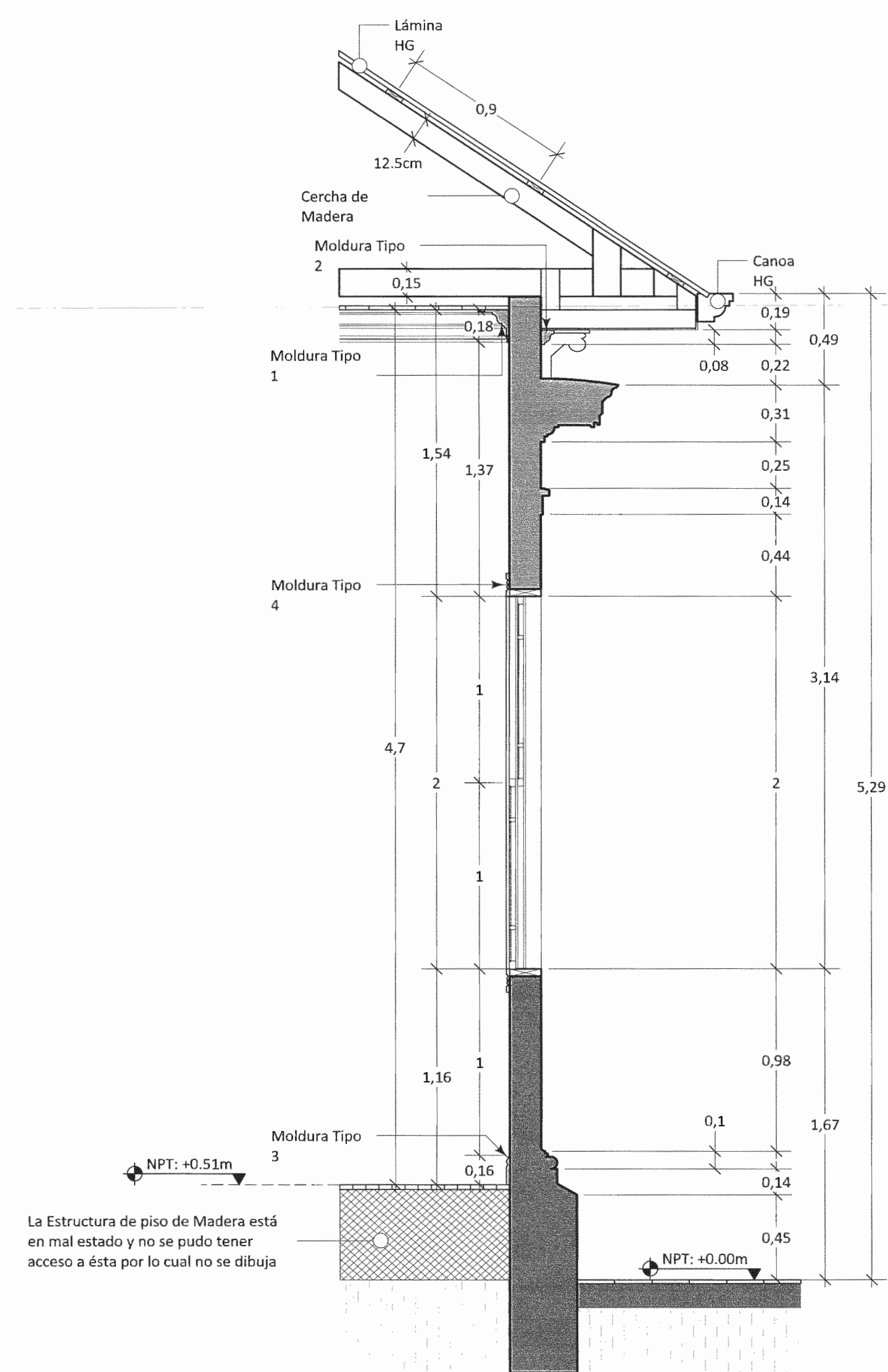
DETALLE 1 Escala 1:25
