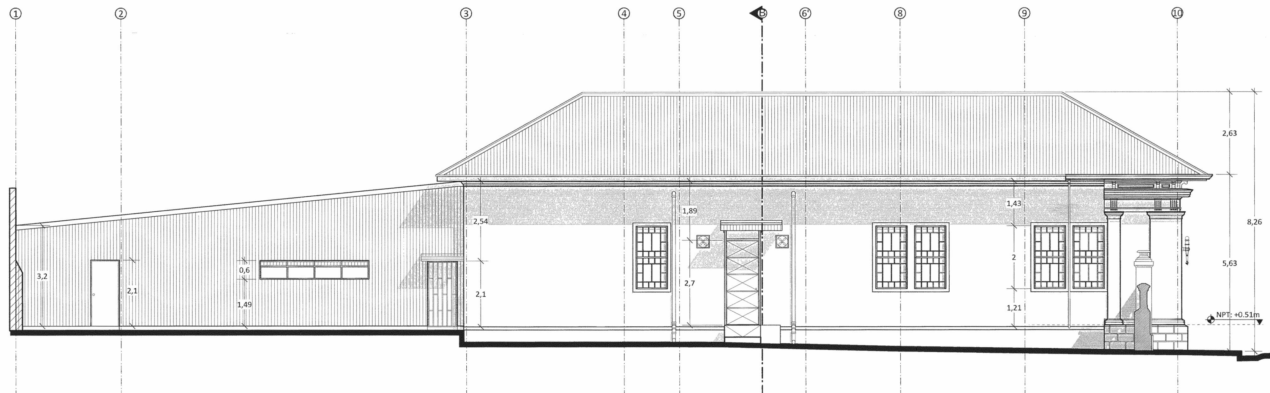
ACTUAL FACHADA OESTE Escala 1:75
