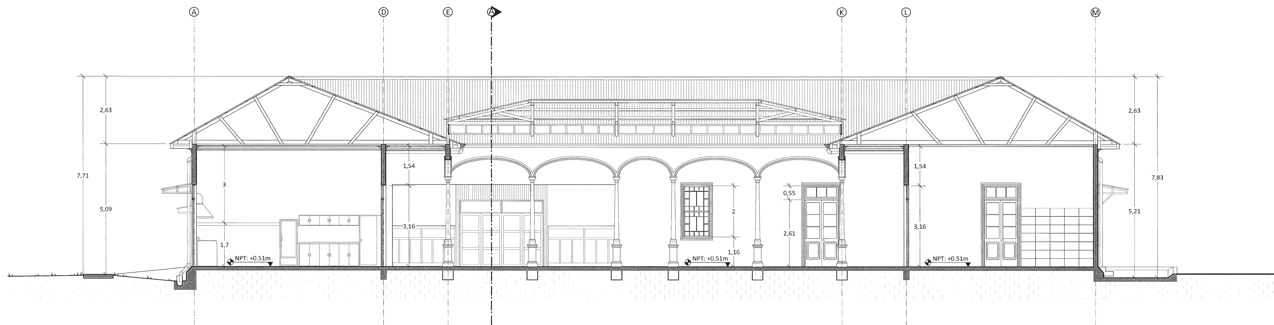
ACTUAL CORTE B - B Escala 1:75
