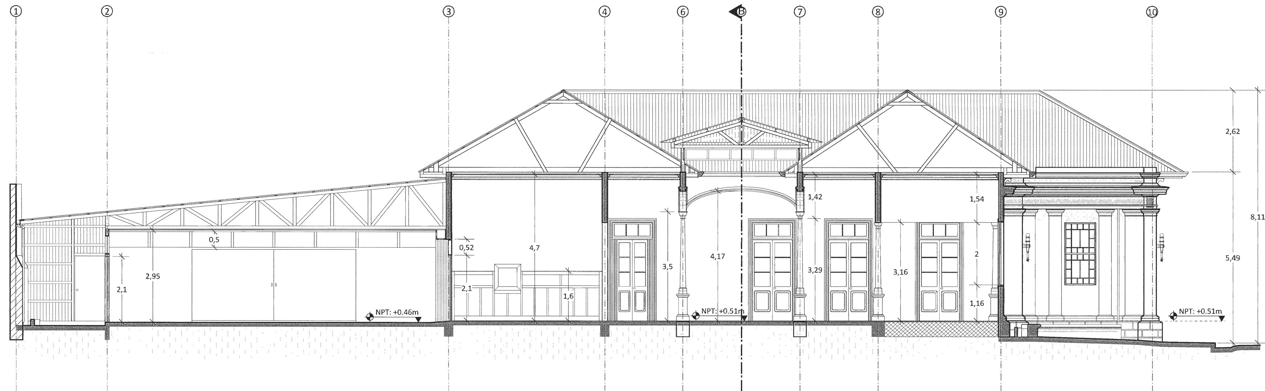
ACTUAL CORTE A - A Escala 1:75
