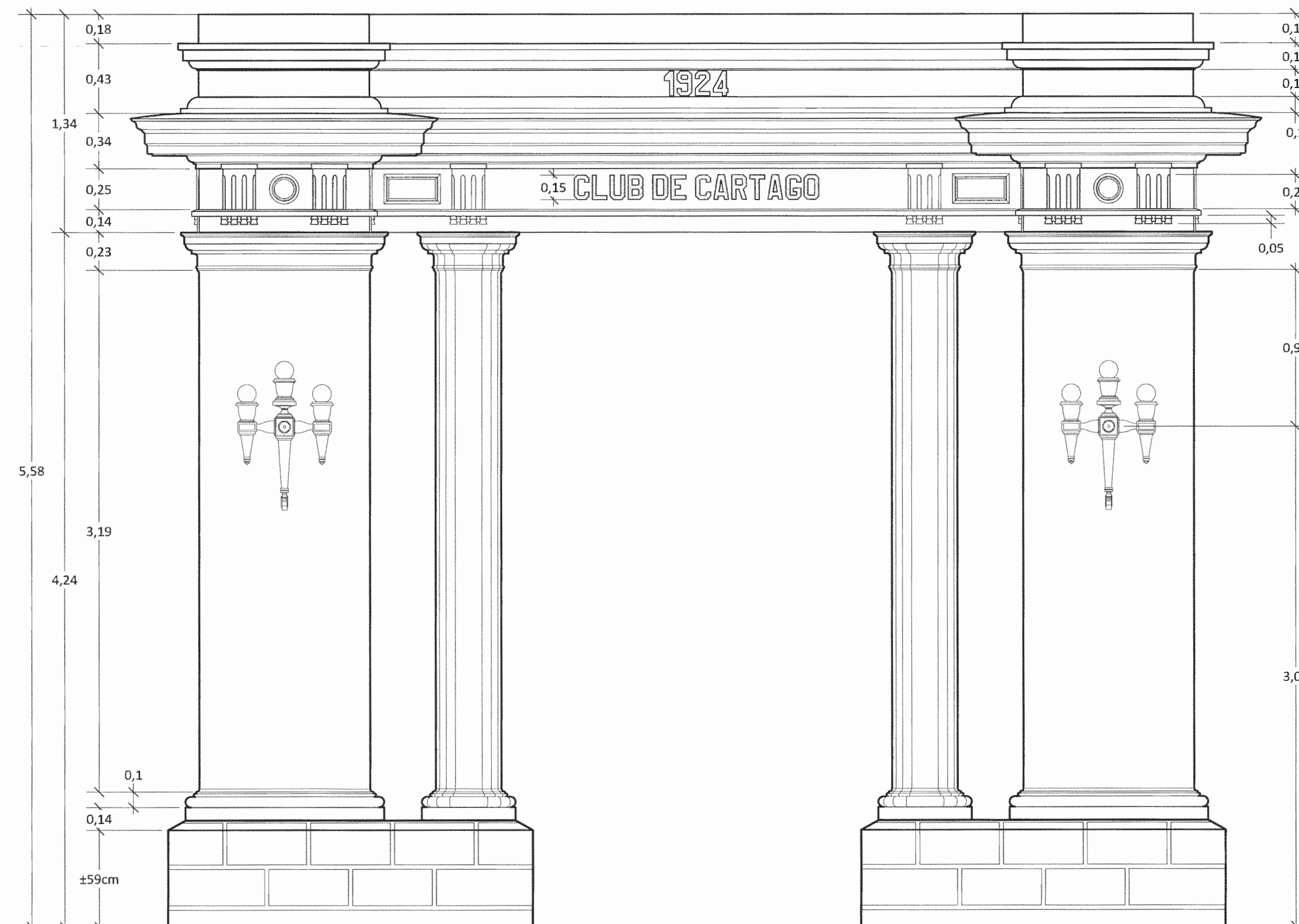
DETALLE ELEVACION DE PORTICO Escala 1:25
