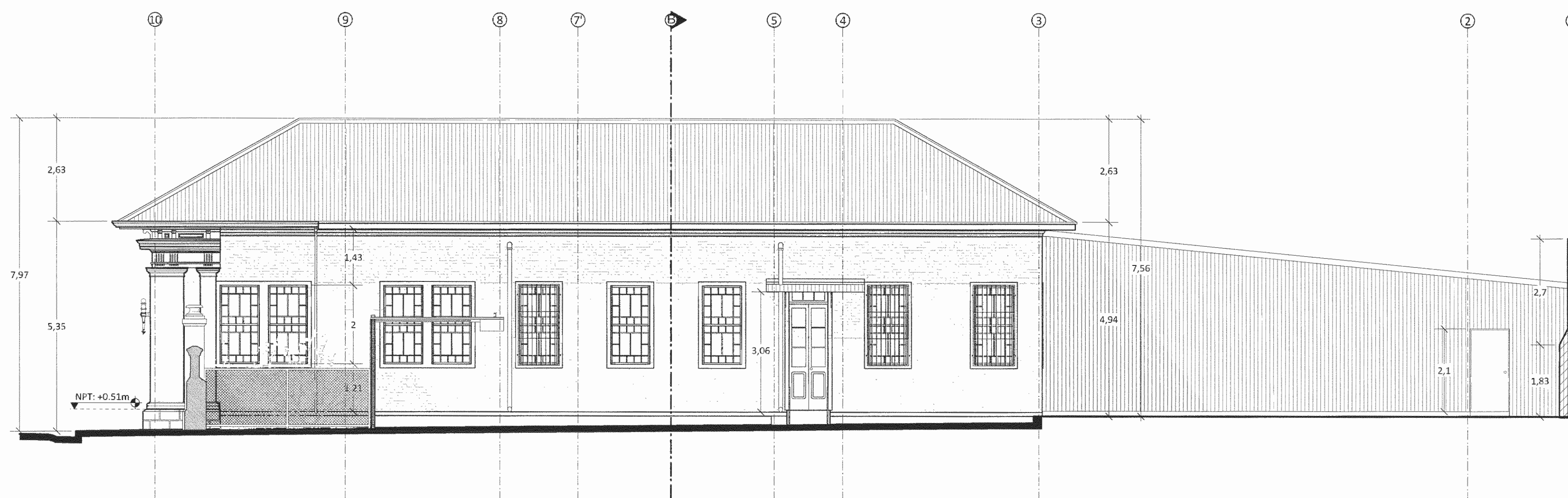
ACTUAL FACHADA ESTE Escala 1:75
