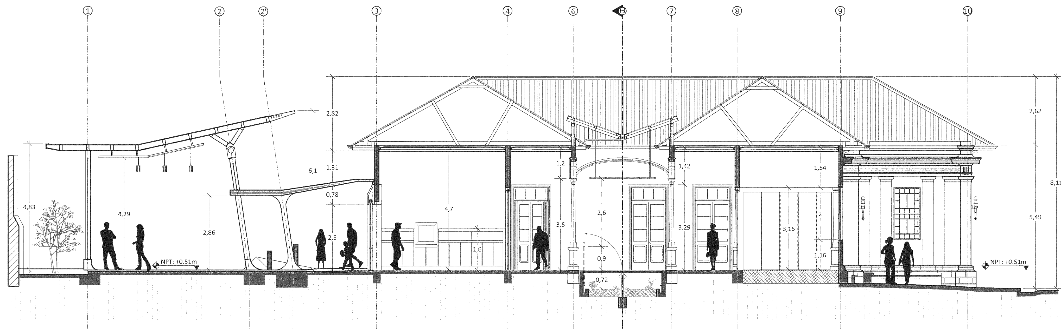
PROPUESTA - CORTE A - A Escala 1:75
