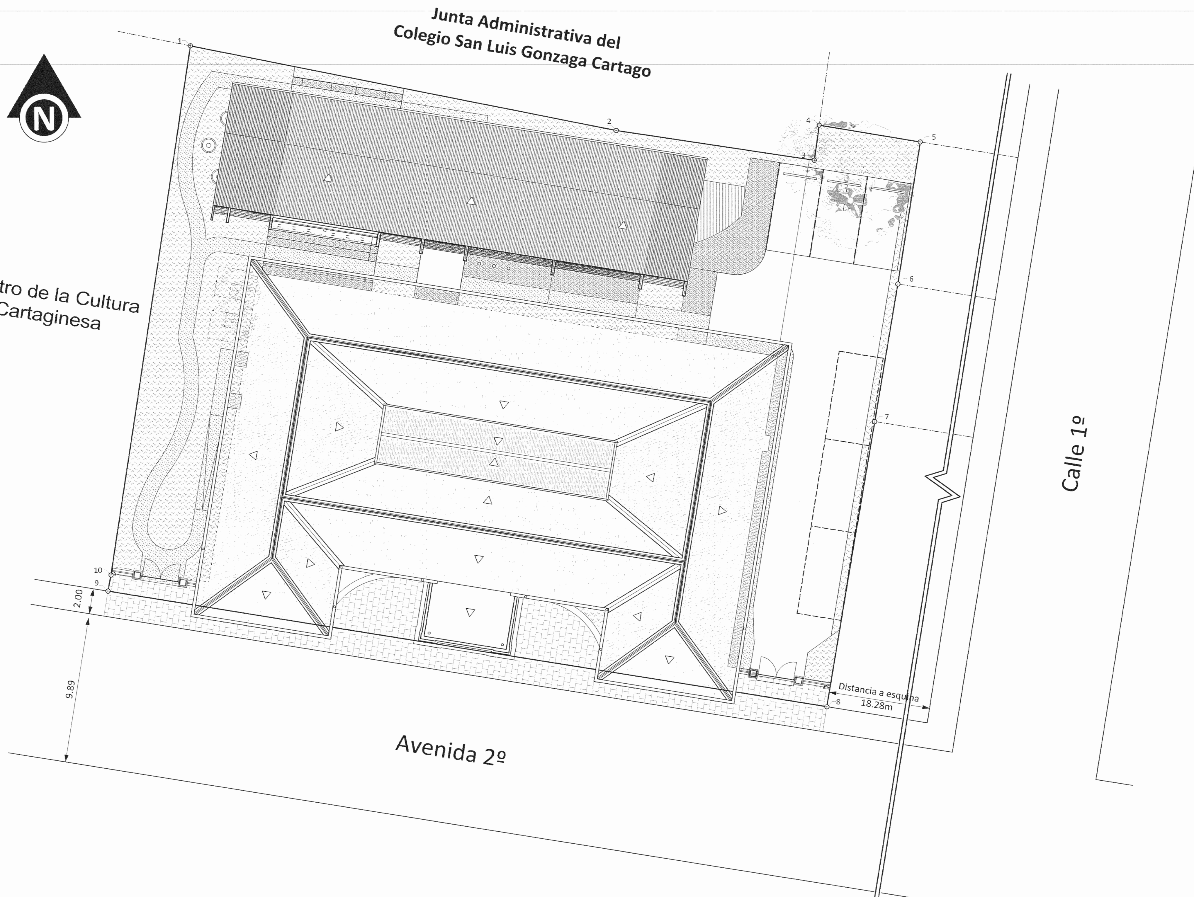
PROPUESTA - PLANTA DE CONJUNTO Escala 1:150
