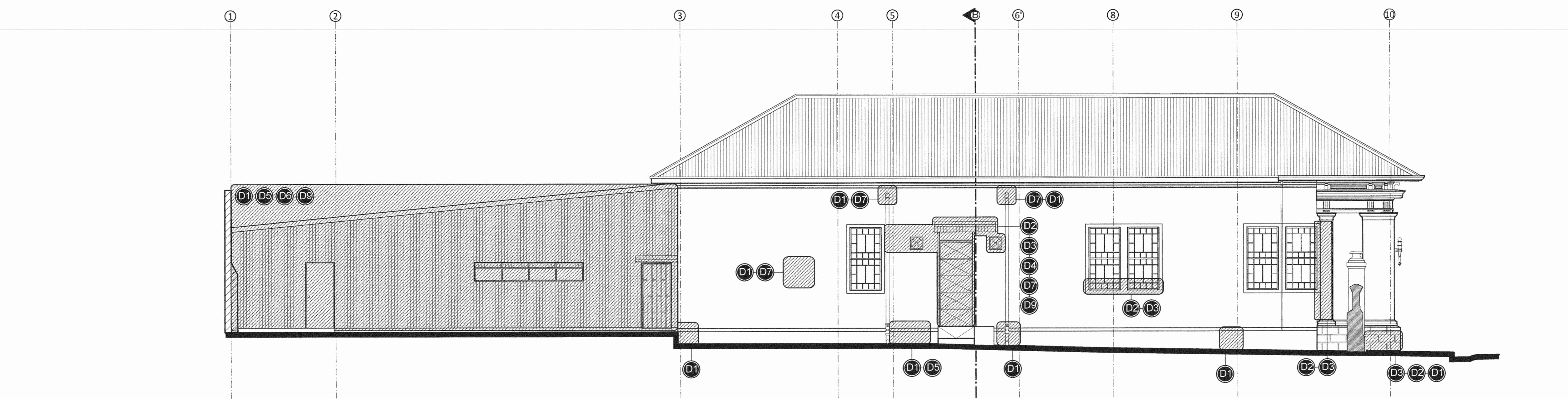
ACTUAL FACHADA OESTE / CONSIGNA DE DAÑOS Escala 1:75
