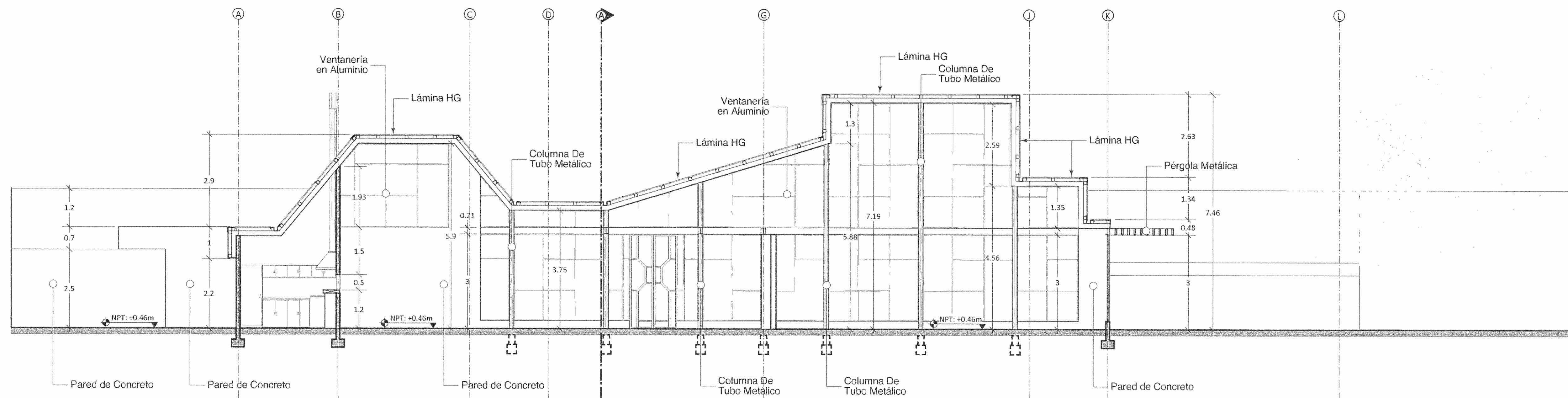
PROPUESTA - CORTE C - C Escala 1:75
