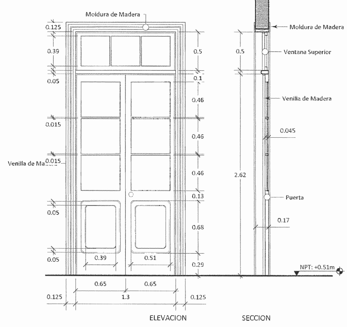
DETALLE DE PUERTA TIPICA Escala 1:25
