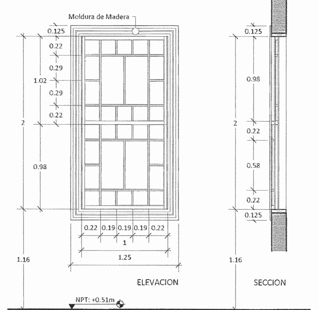
DETALLE DE VENTANA TIPICA Escala 1:25
