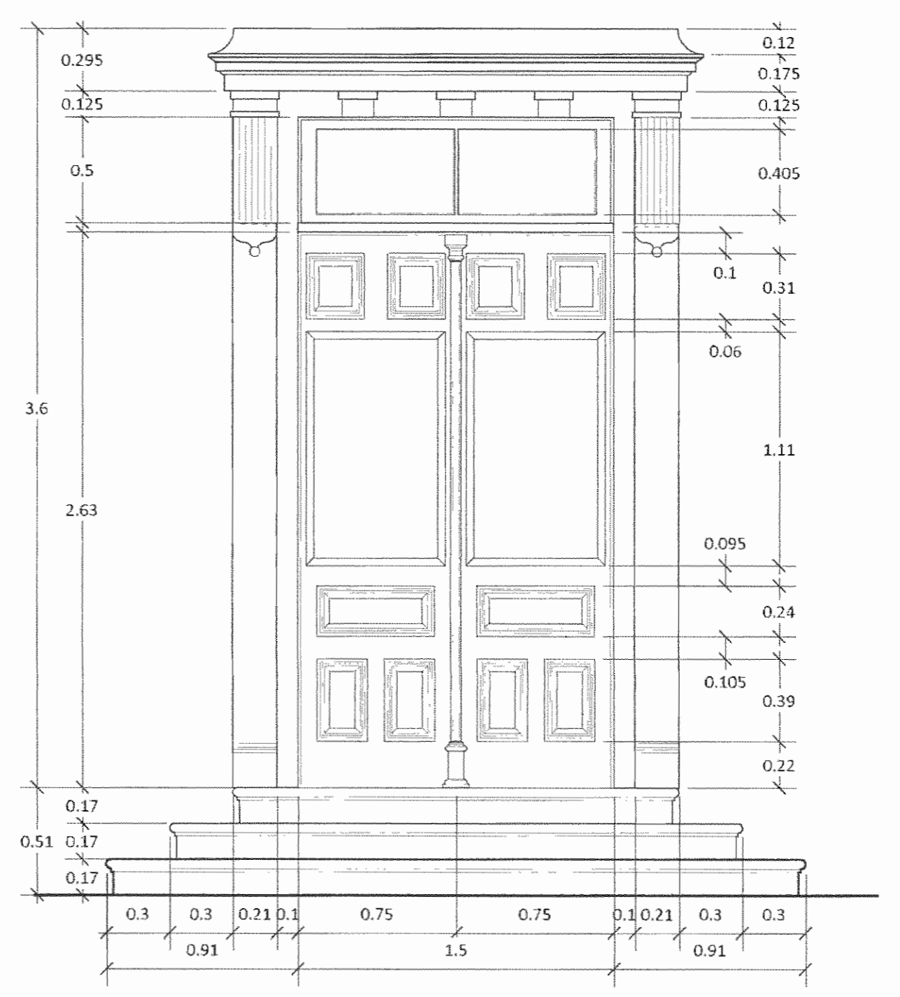
DETALLE DE PUERTA PRINCIPAL Escala 1:25
