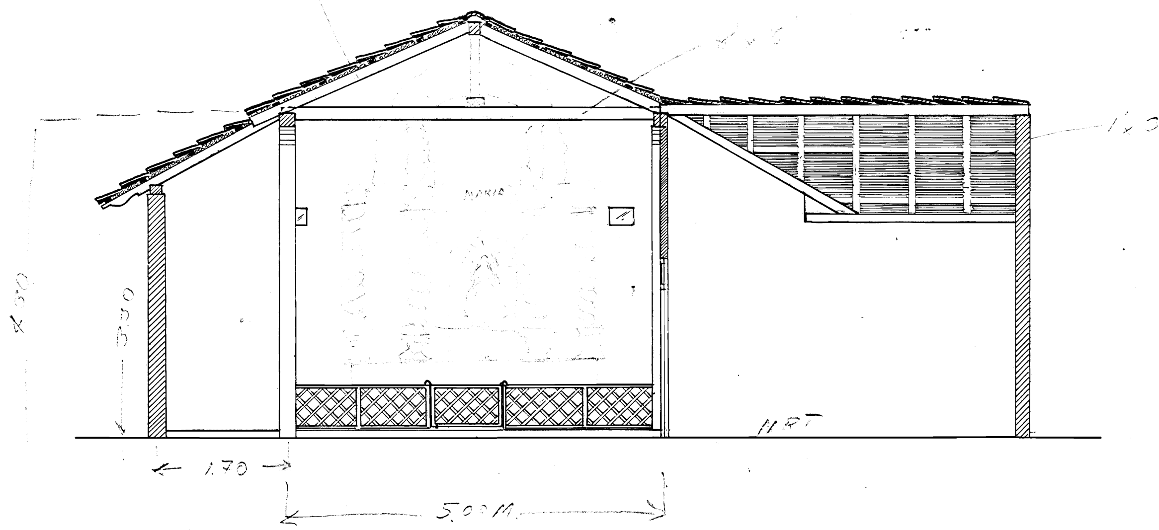
CORTE TRANSVERSAL B-B
