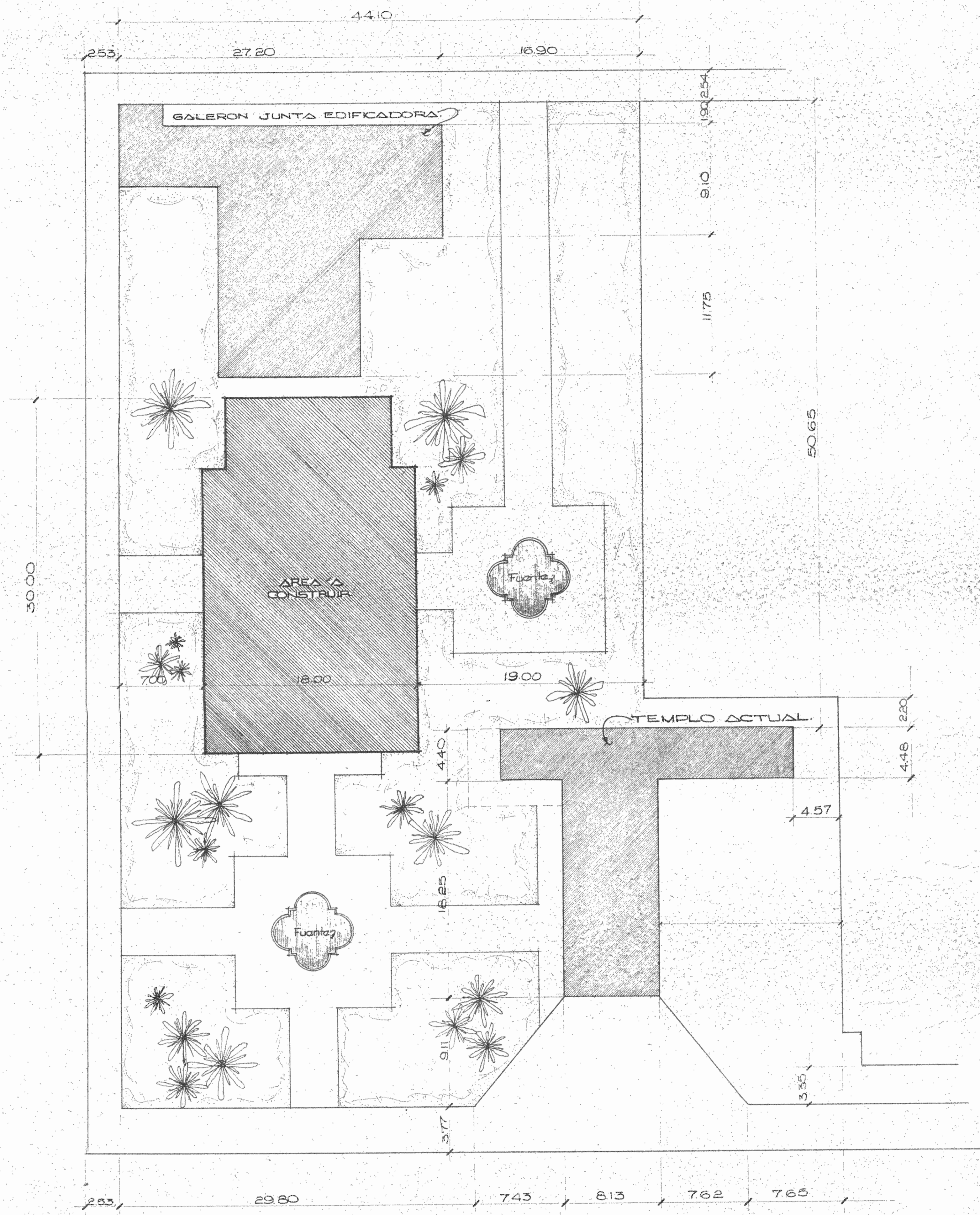
PLANTA DE CONJUNTO. ESC: 1:200
