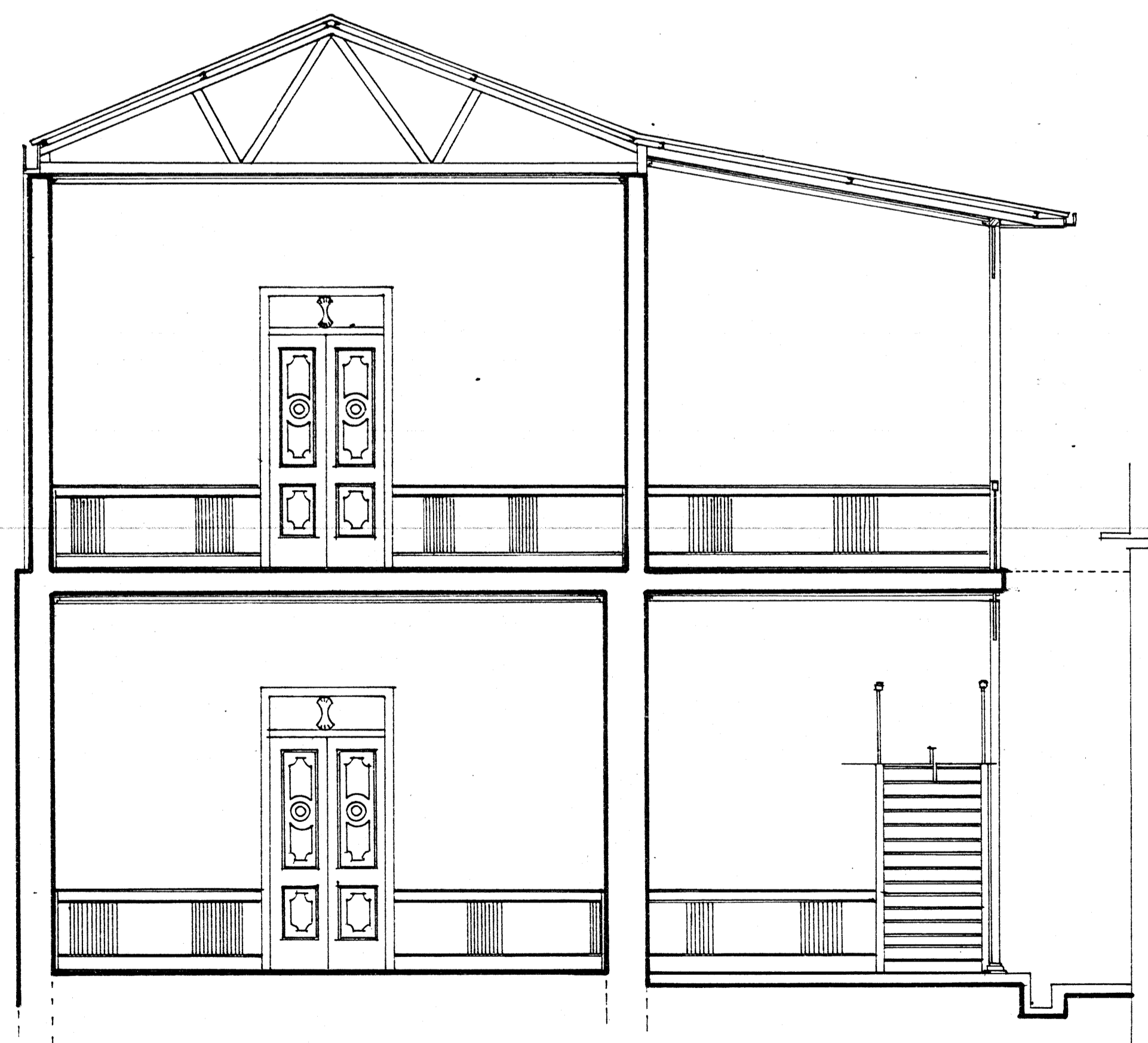
CORTE 4-4 ESC. 1:50
