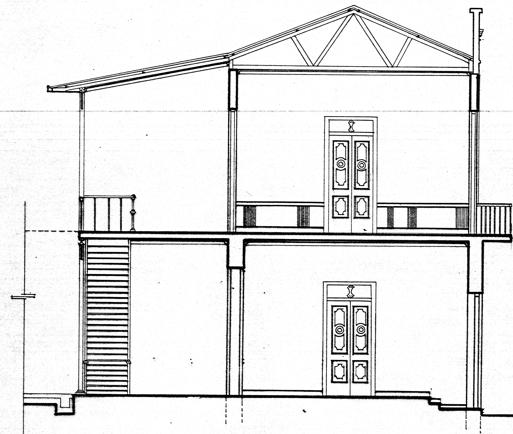
CORTE 2-2 ESC. 1:50
