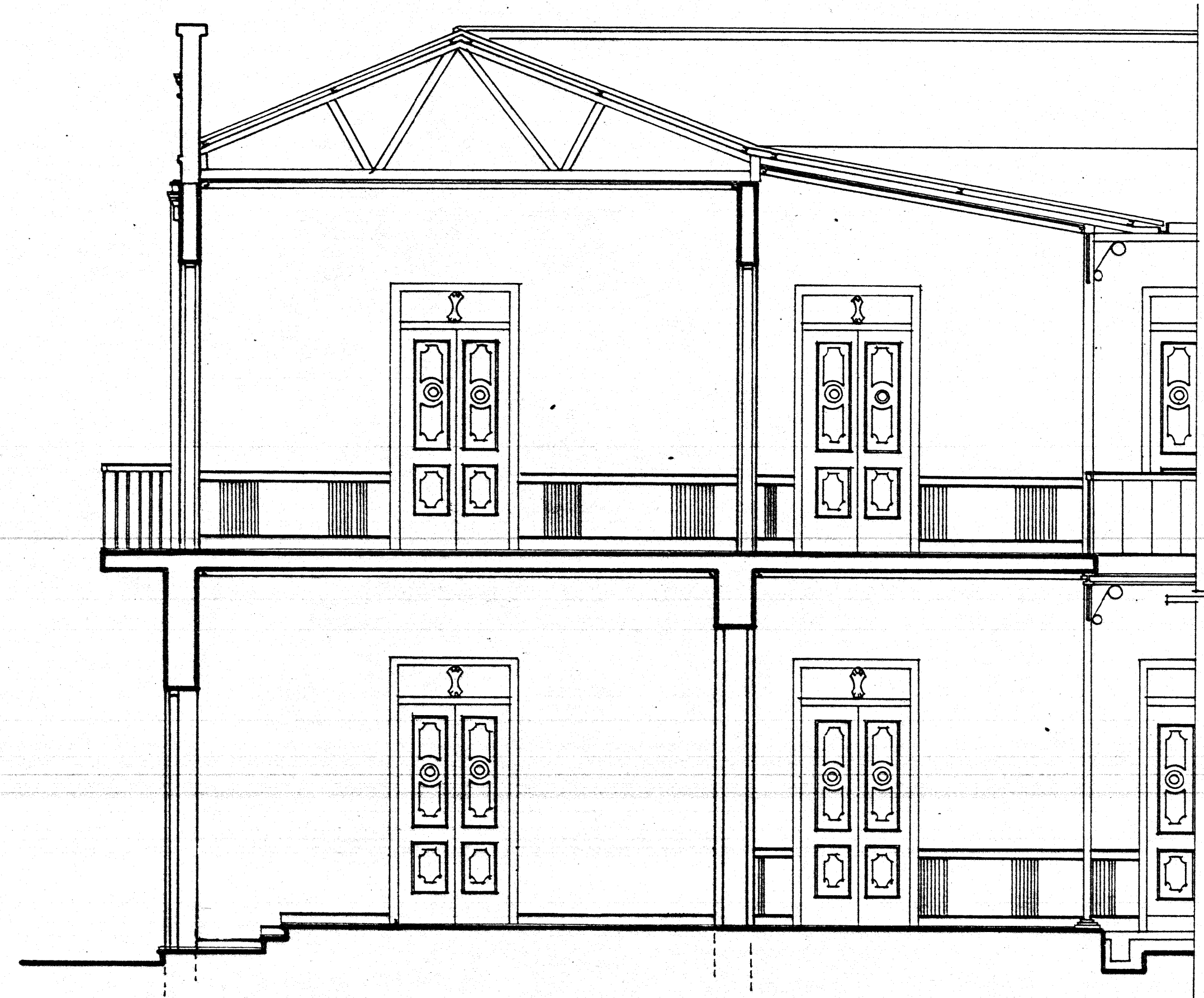
CORTE 3-3 ESC. 1:50
