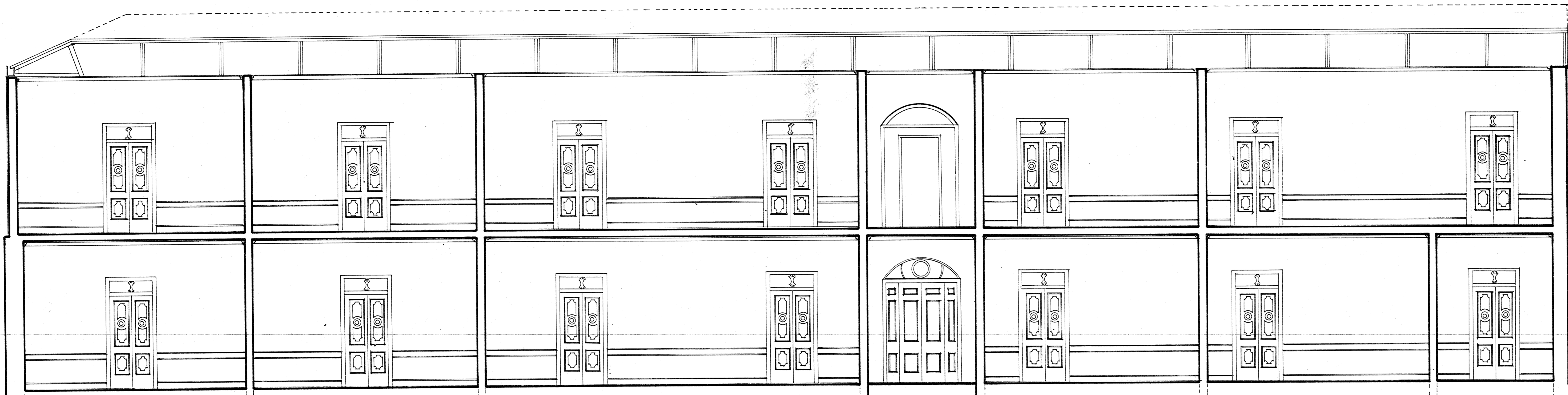
SECCION GG ESC. 1:50
