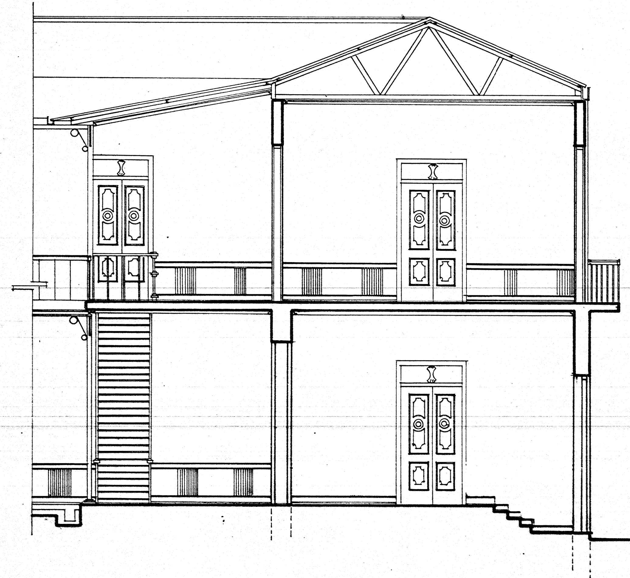
CORTE 5-5 ESC. 1:50
