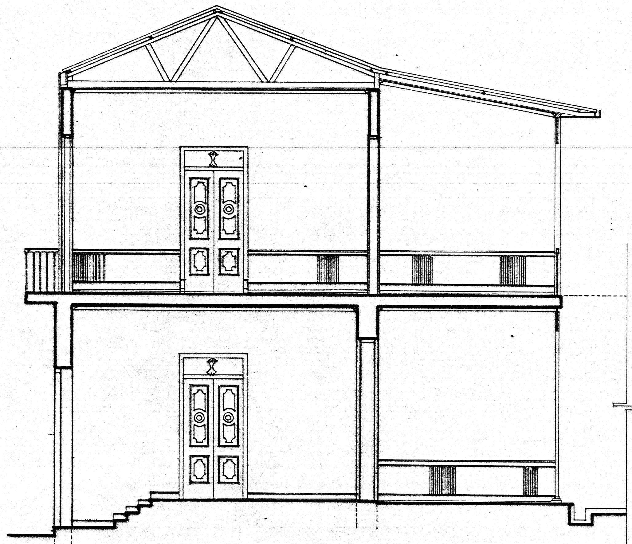
CORTE 6-6 ESC. 1:50
