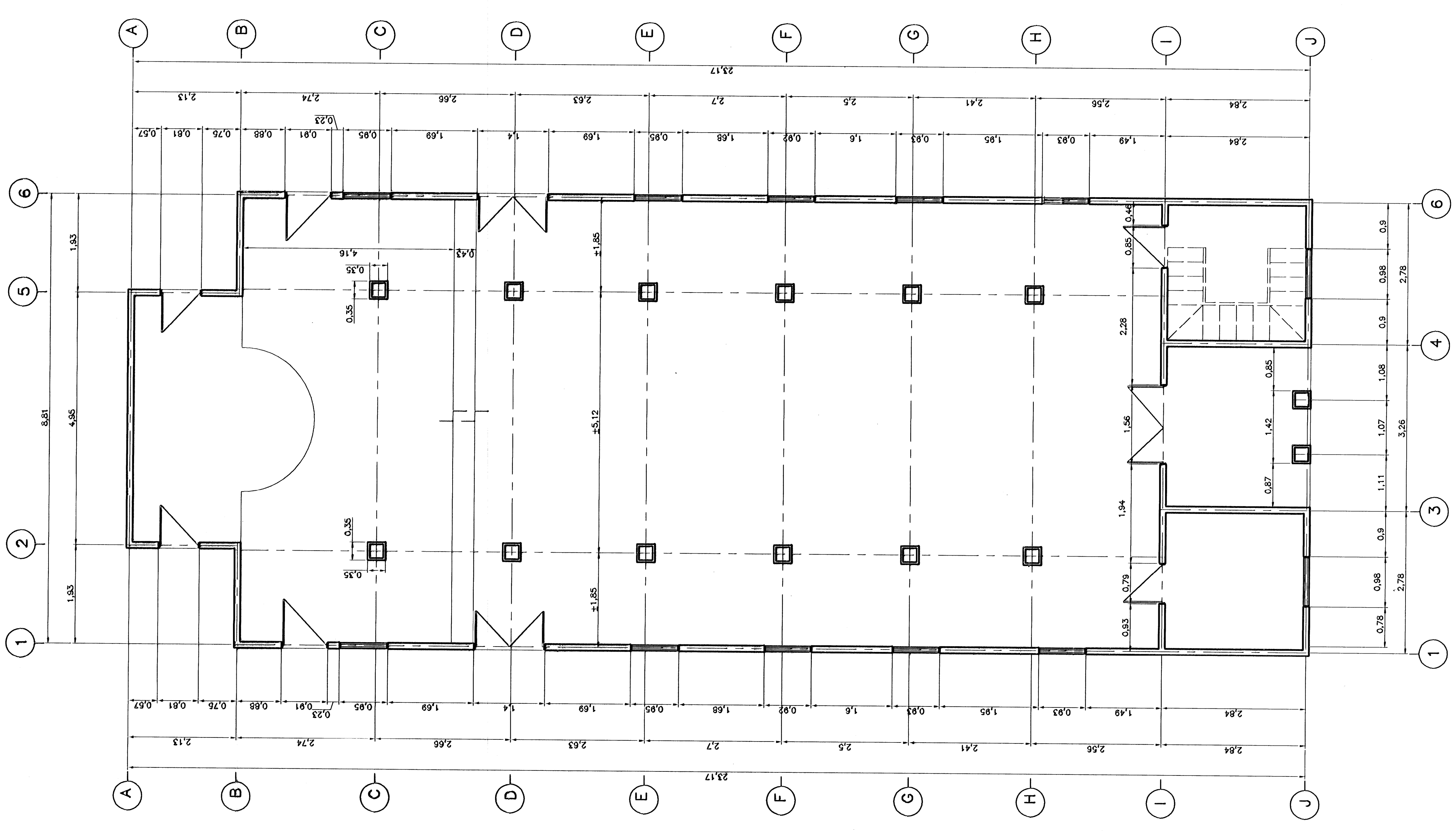
PLANTA DE DISTRIBUCION ARQUITECTONICA ESC. 1:50
