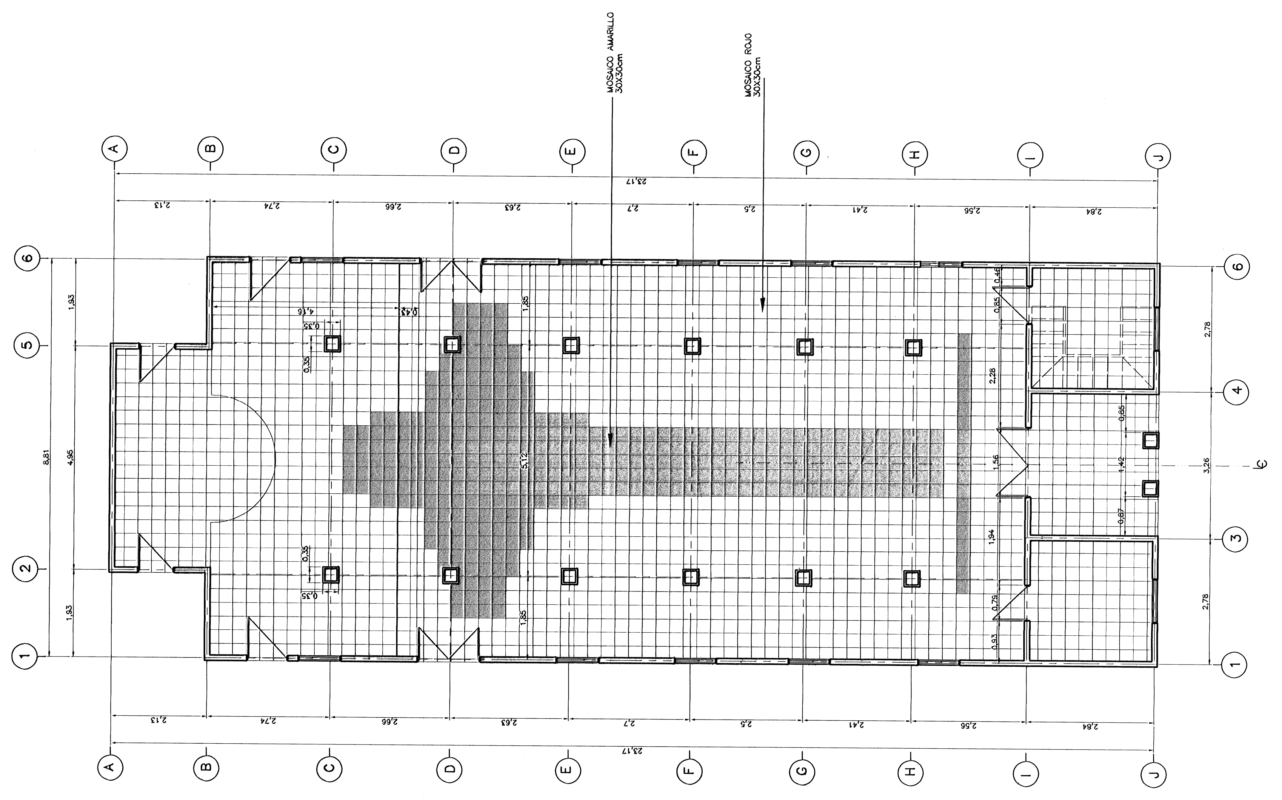
PLANTA DE DISEÑO DE PISO ESC. 1:50
