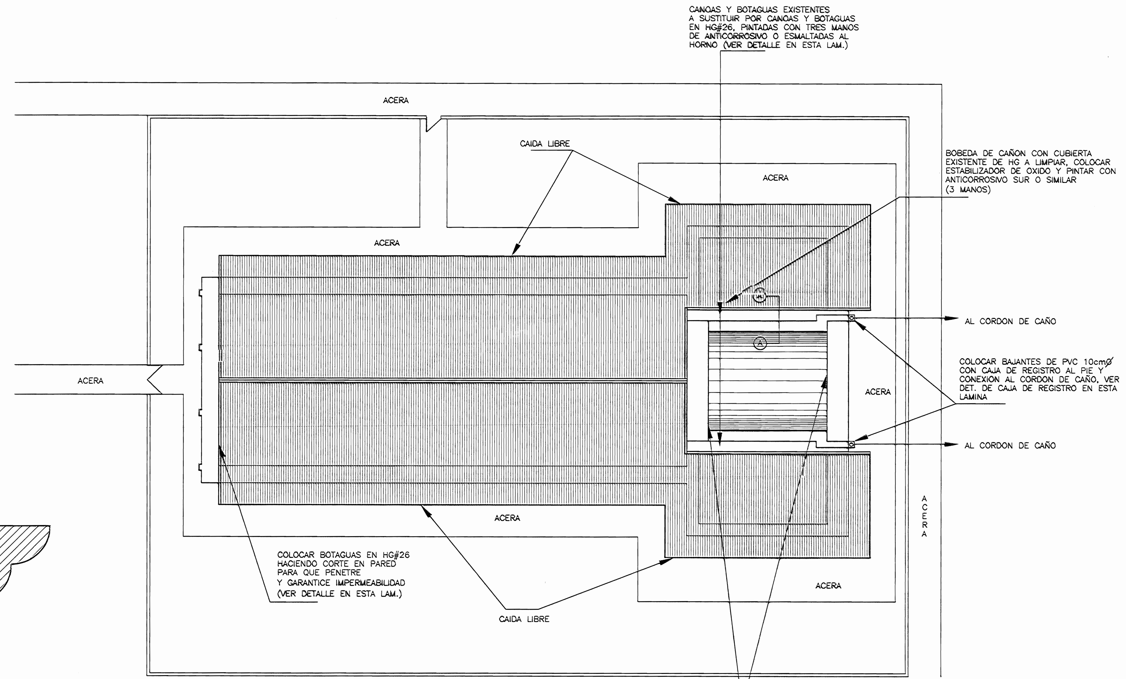
PLANTA DE TECHOS Y EVACUACION PLUVIAL ESC. 1 : 125
