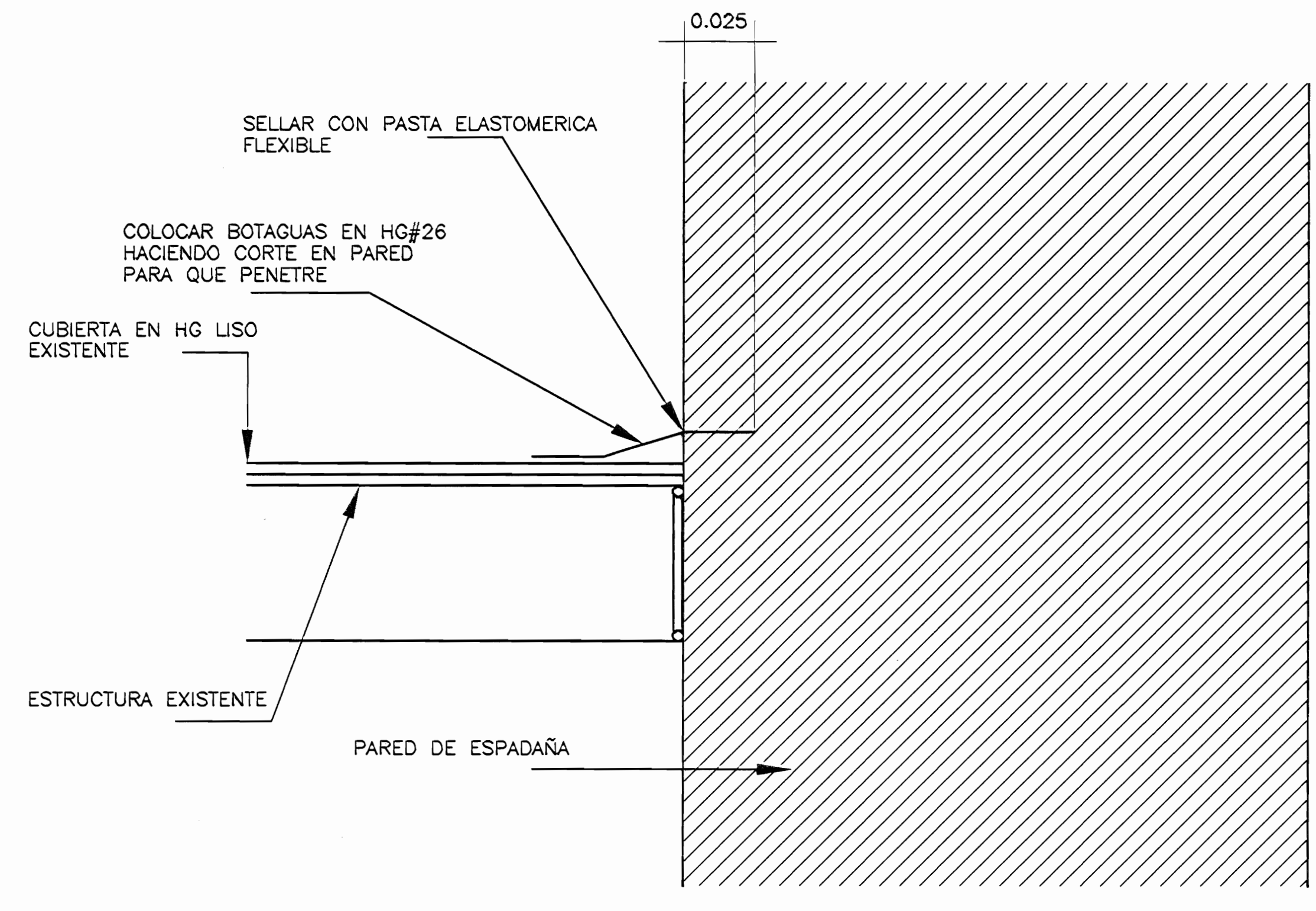
DETALLE DE COLOCACION DE BOTAGUAS ESC. 1 : 10
