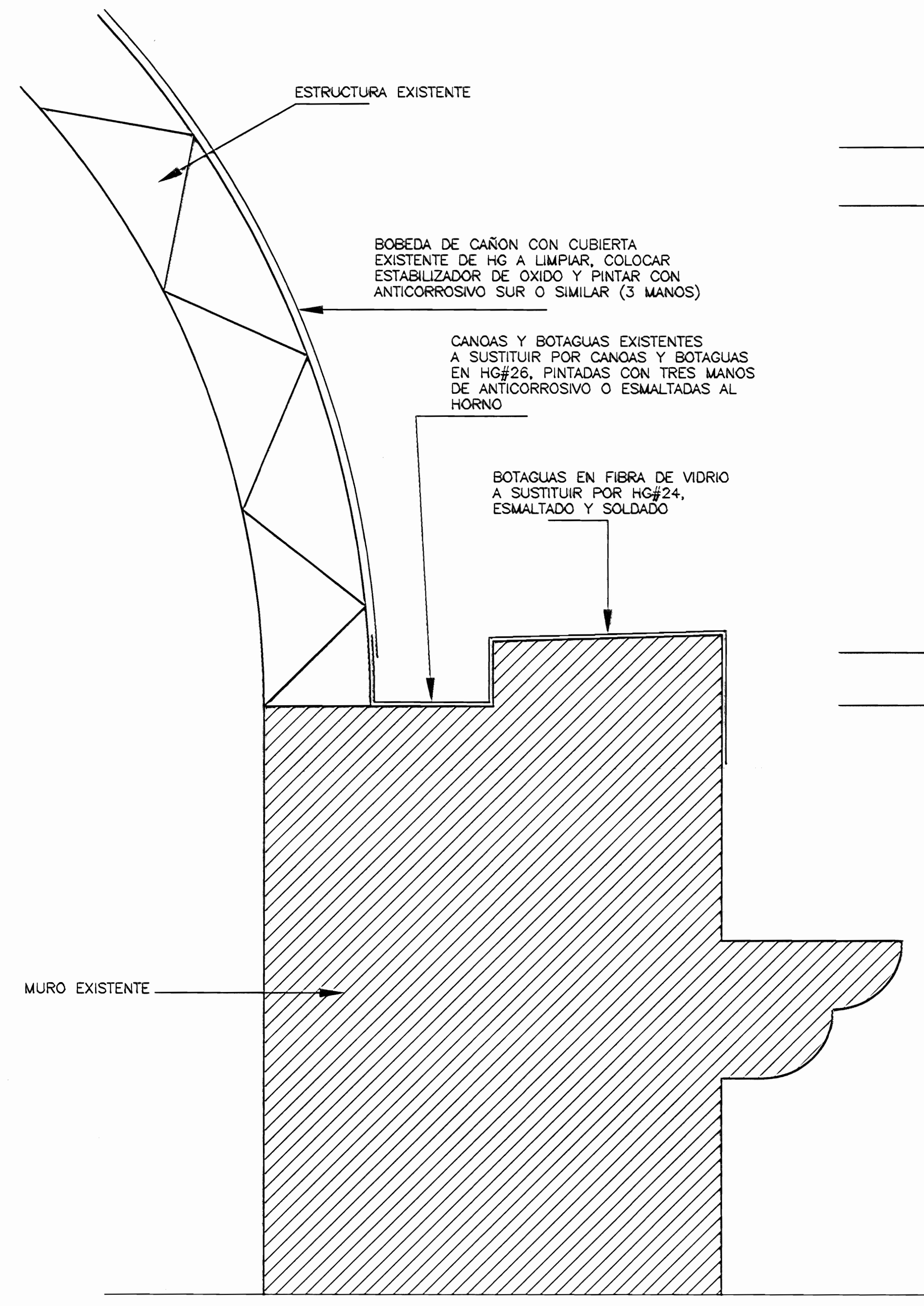
SECCION A-A DETALLE DE BOTAGUAS Y CANOA DE LA BOBEDA DE CAÑON ESC. 1 : 10
