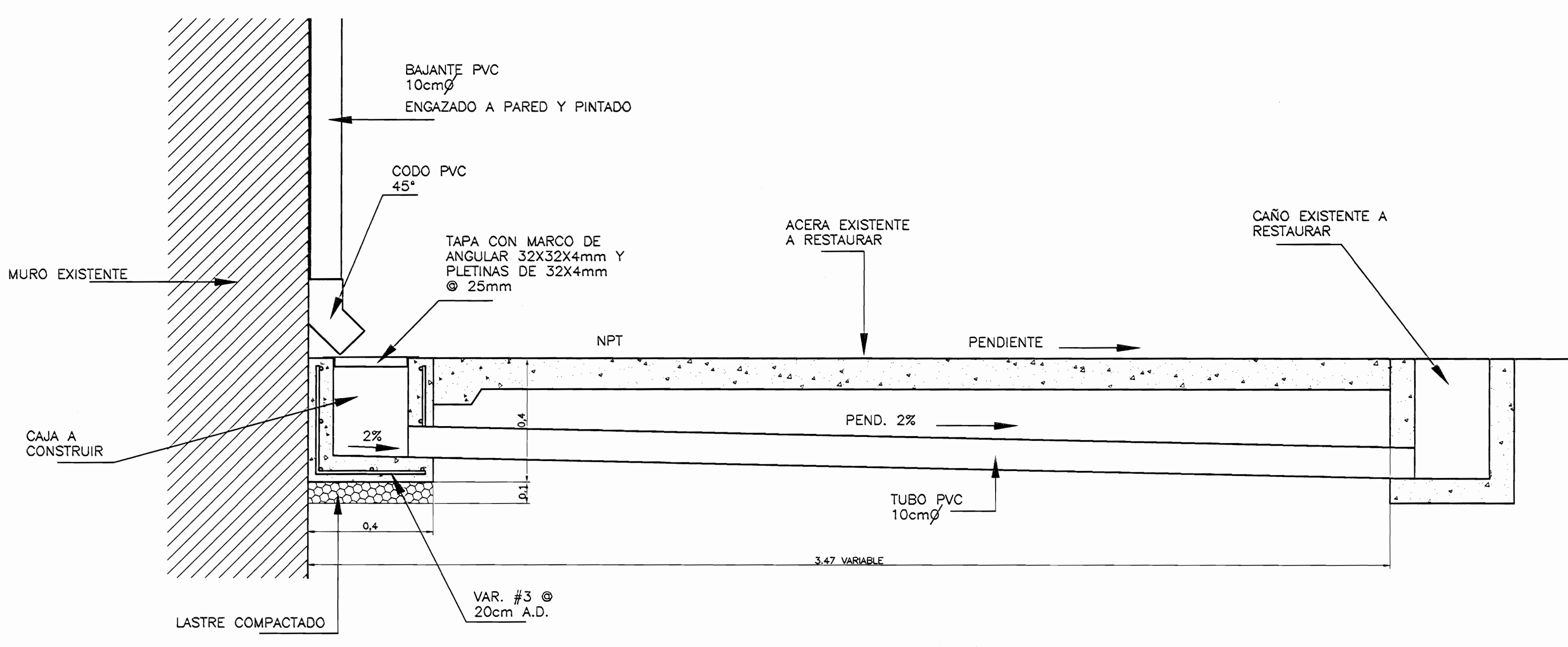
DETALLE CAJA DE REGISTRO PLUVIAL ESC. 1 : 10
