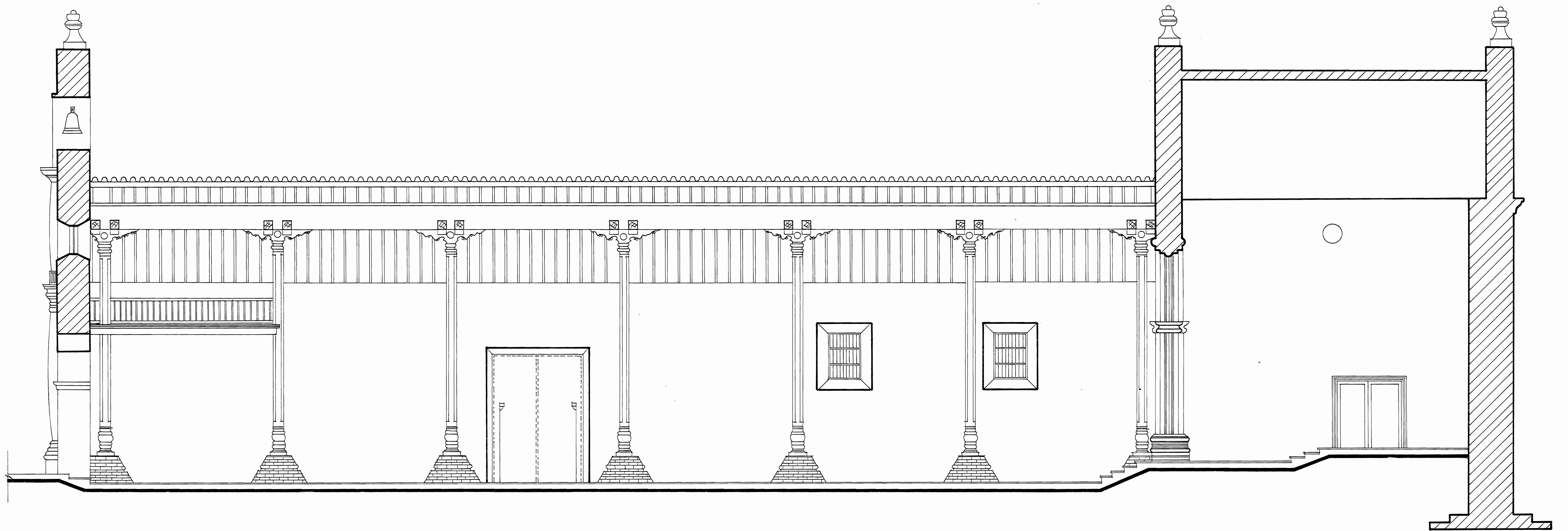
SECCION LONGITUDINAL IGLESIA DE SAN BLAS - NICOYA ESC. 1:50
