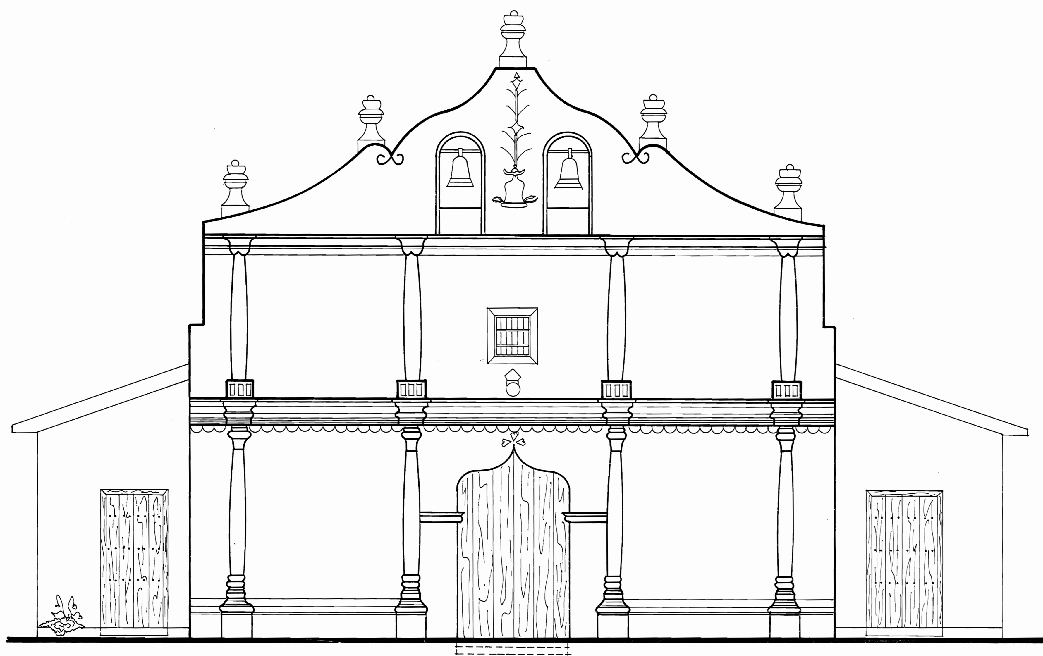
ELEVACION PRINCIPAL IGLESIA DE SAN BLAS-NICOYA ESC. 1: 50
