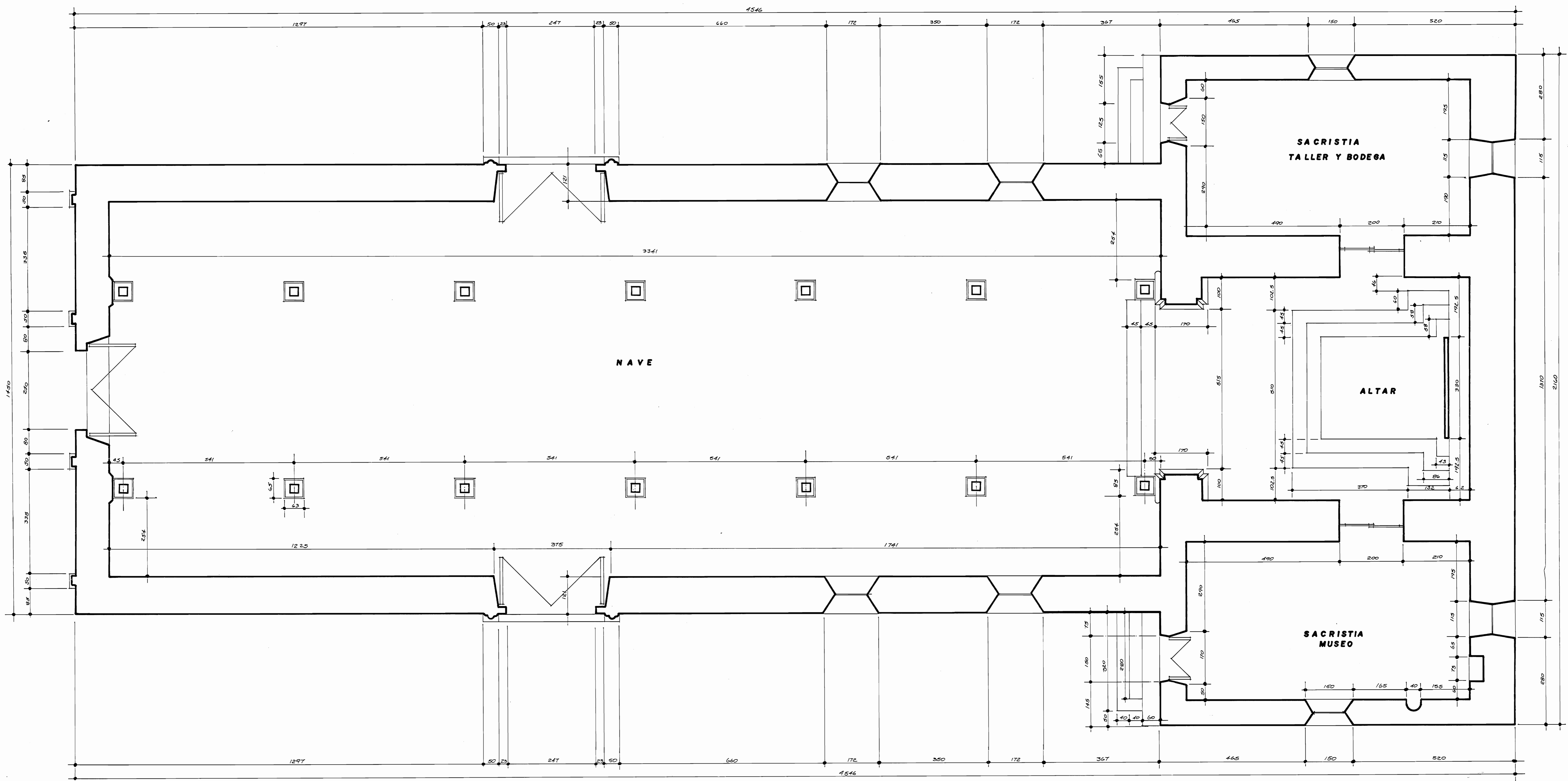
PLANTA ARQUITECTONICA IGLESIA DE SAN BLAS - NICOYA ESC. 1:50
