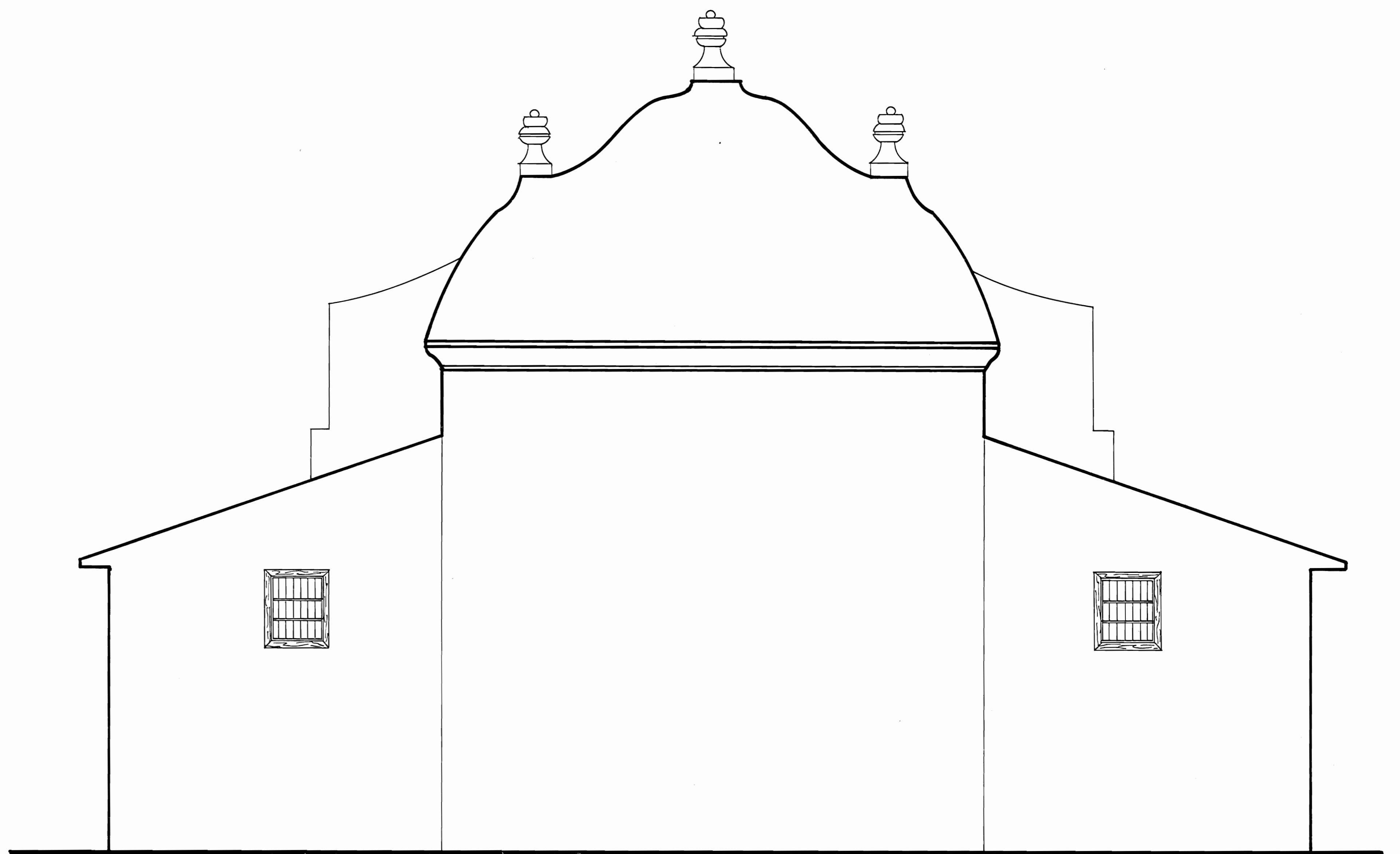
ELEVACION POSTERIOR IGLESIA DE SAN BLAS-NICOYA ESC. 1: 50
