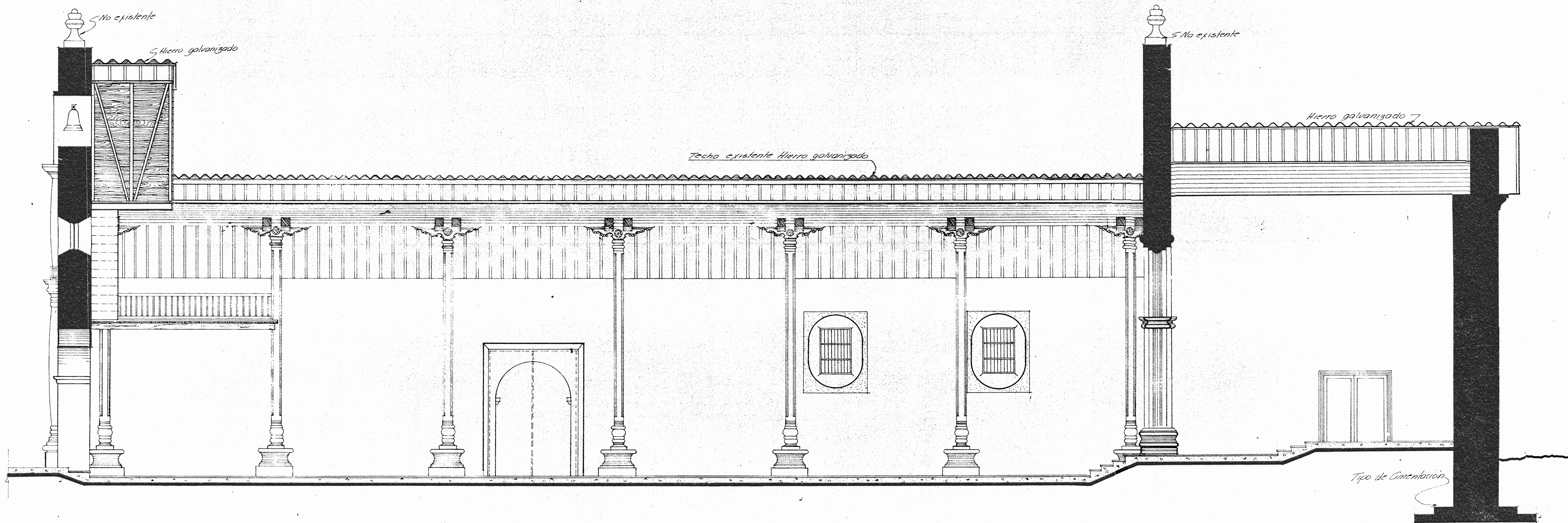
SECCION LONGITUDINAL "EXISTENTE" Escala 1:50
