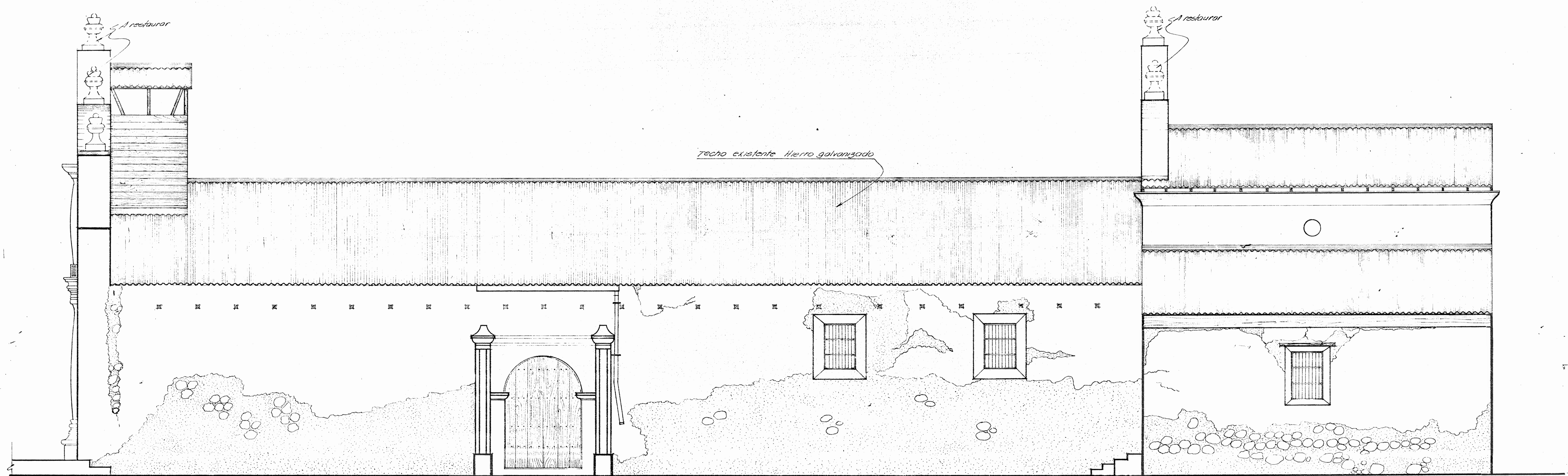
ELEVACION SUR "EXISTENTE" Escala 1:50
