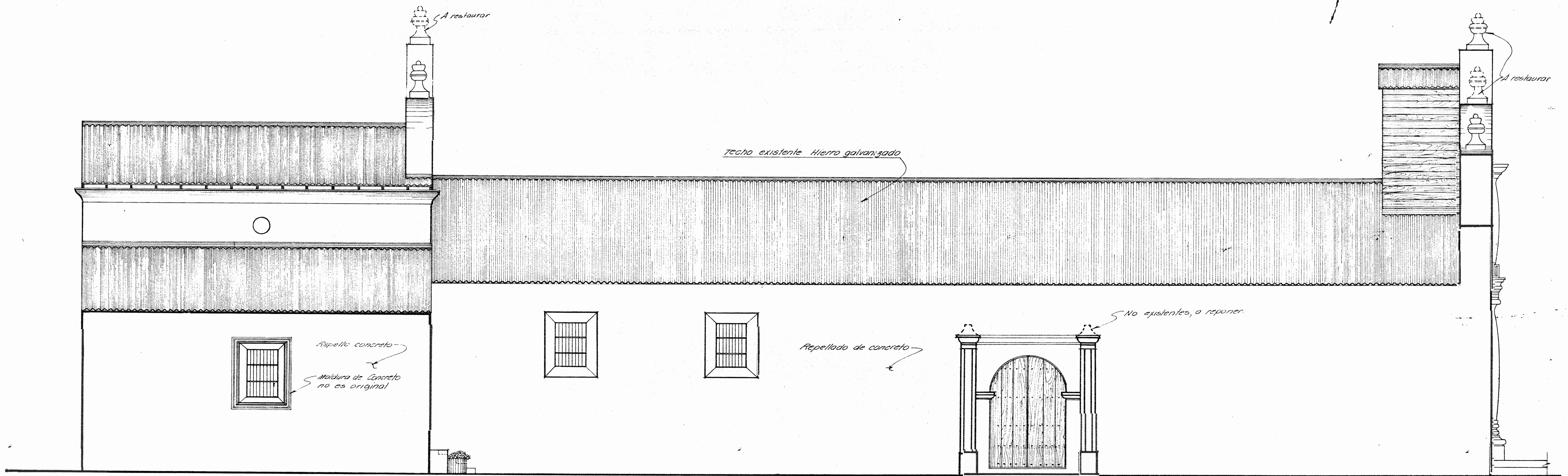
ELEVACION NORTE "EXISTENTE" Escala 1:50
