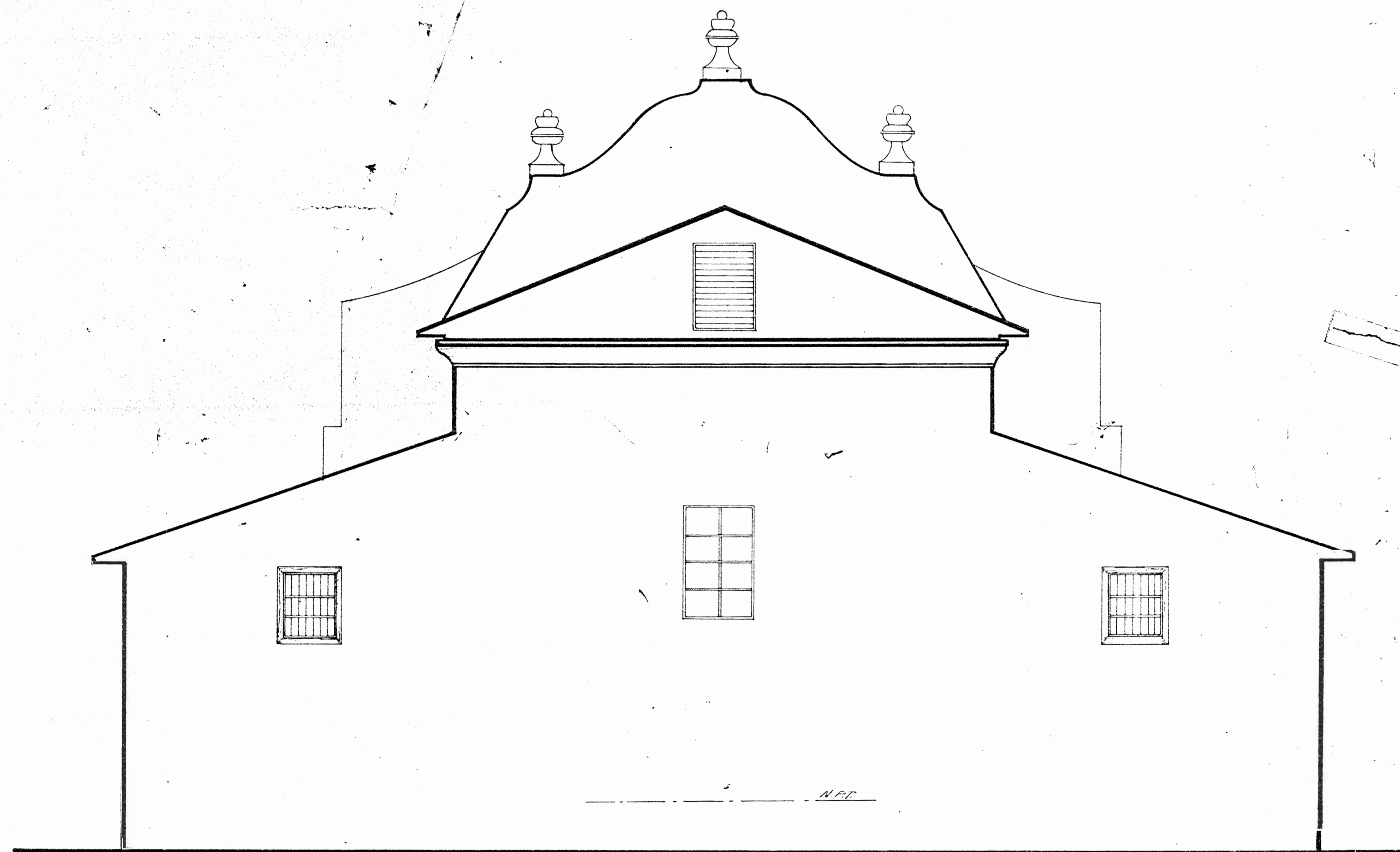
ELEVACION POSTERIOR "EXISTENTE" Escala 1:50
