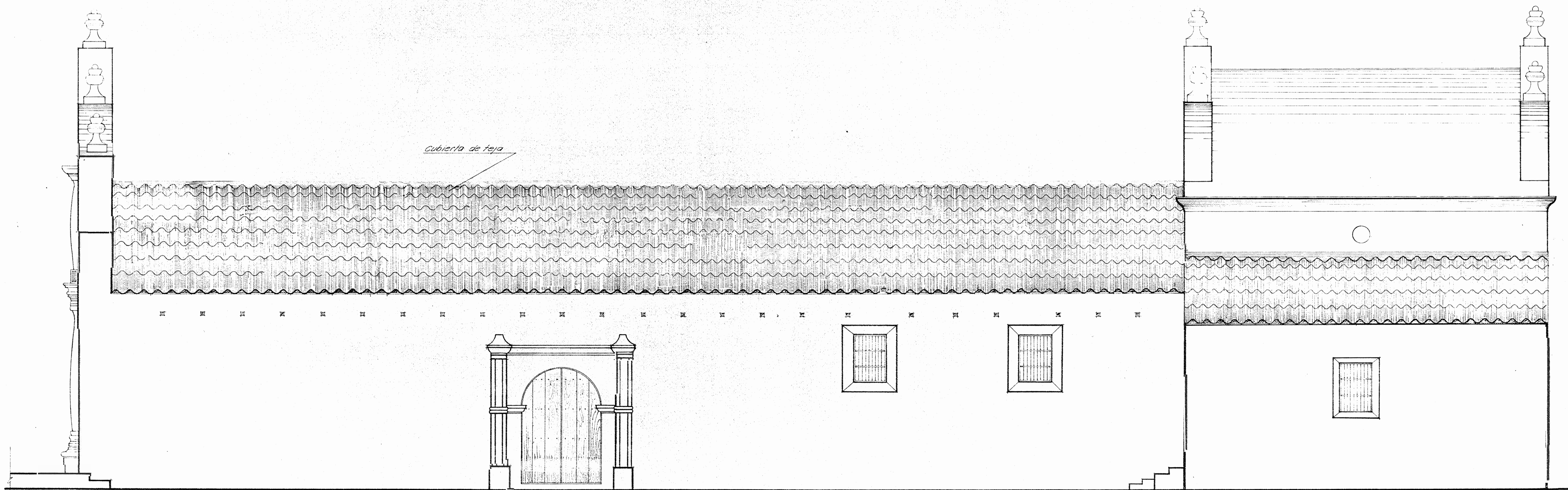
ELEVACION SUR "RESTAURADA" Escala 1:50
