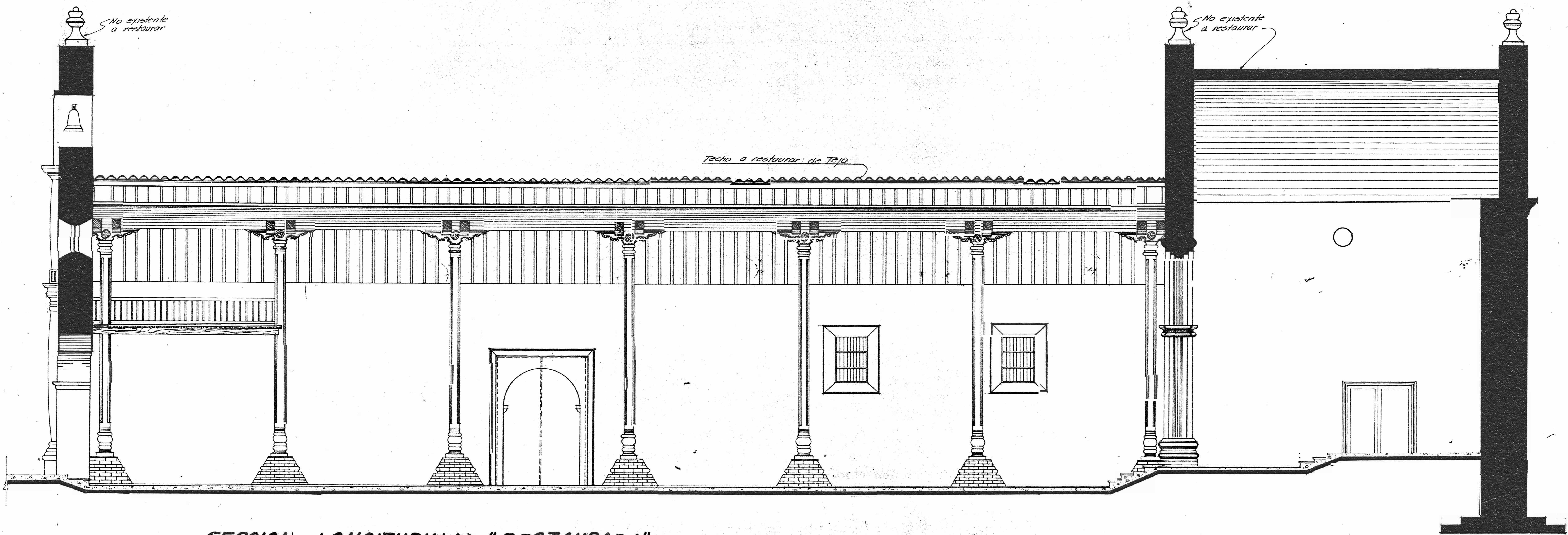
SECCION LONGITUDINAL "RESTAURADA" Escala 1:50
