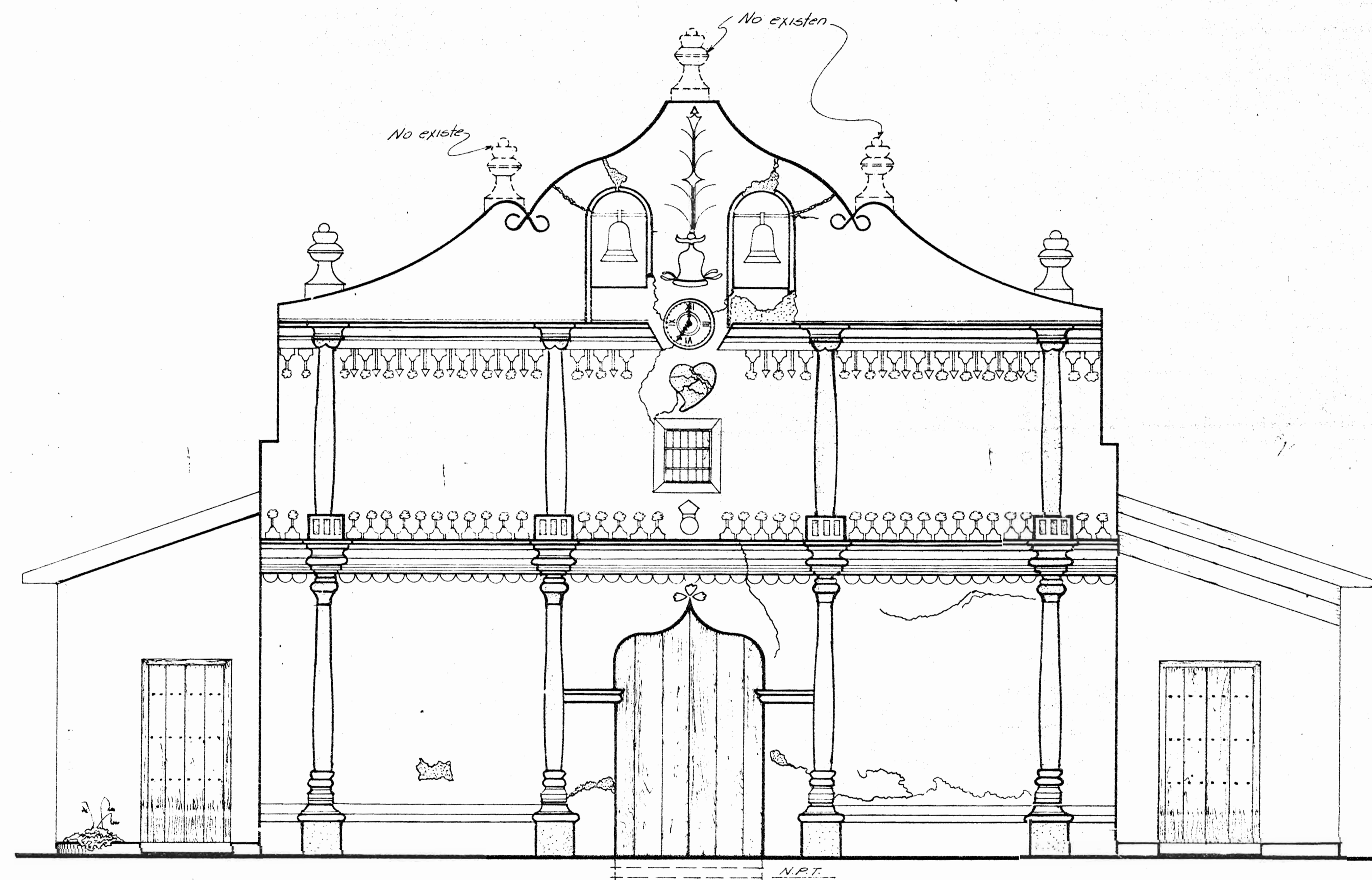
ELEVACION PRINCIPAL "EXISTENTE" Escala 1:50
