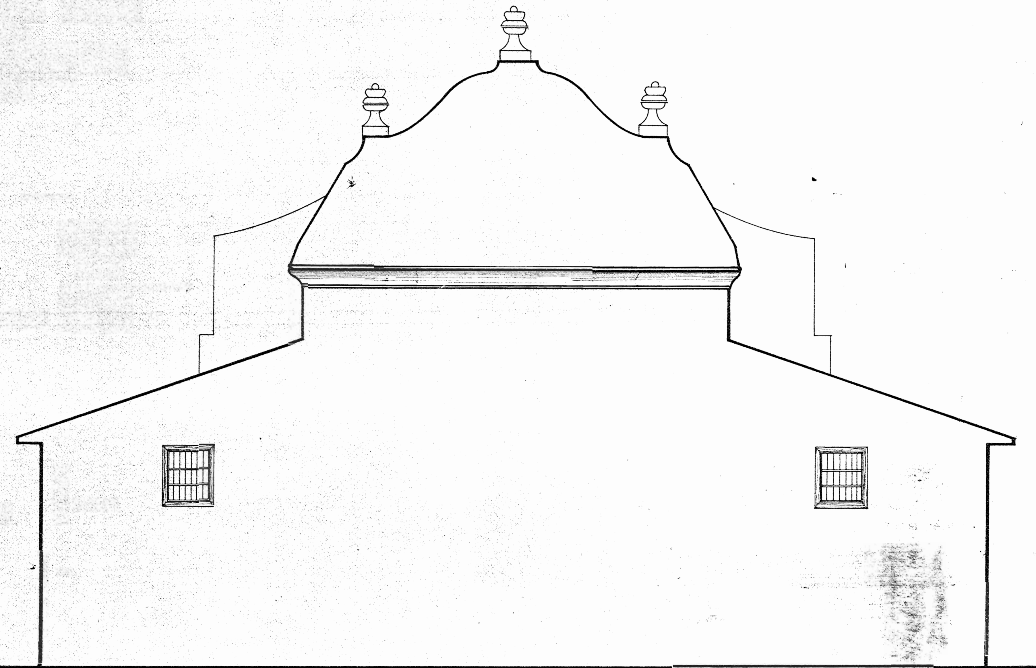
ELEVACION POSTERIOR "RESTAURADA" Escala 1:50
