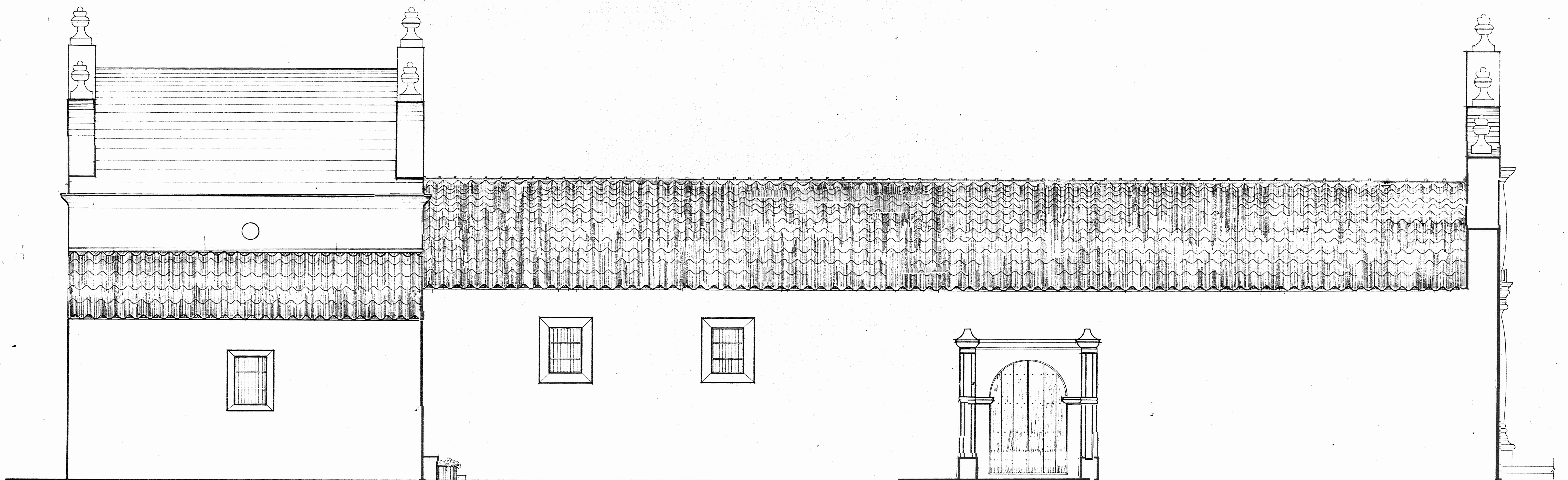
ELEVACION NORTE "RESTAURADA" Escala 1:50
