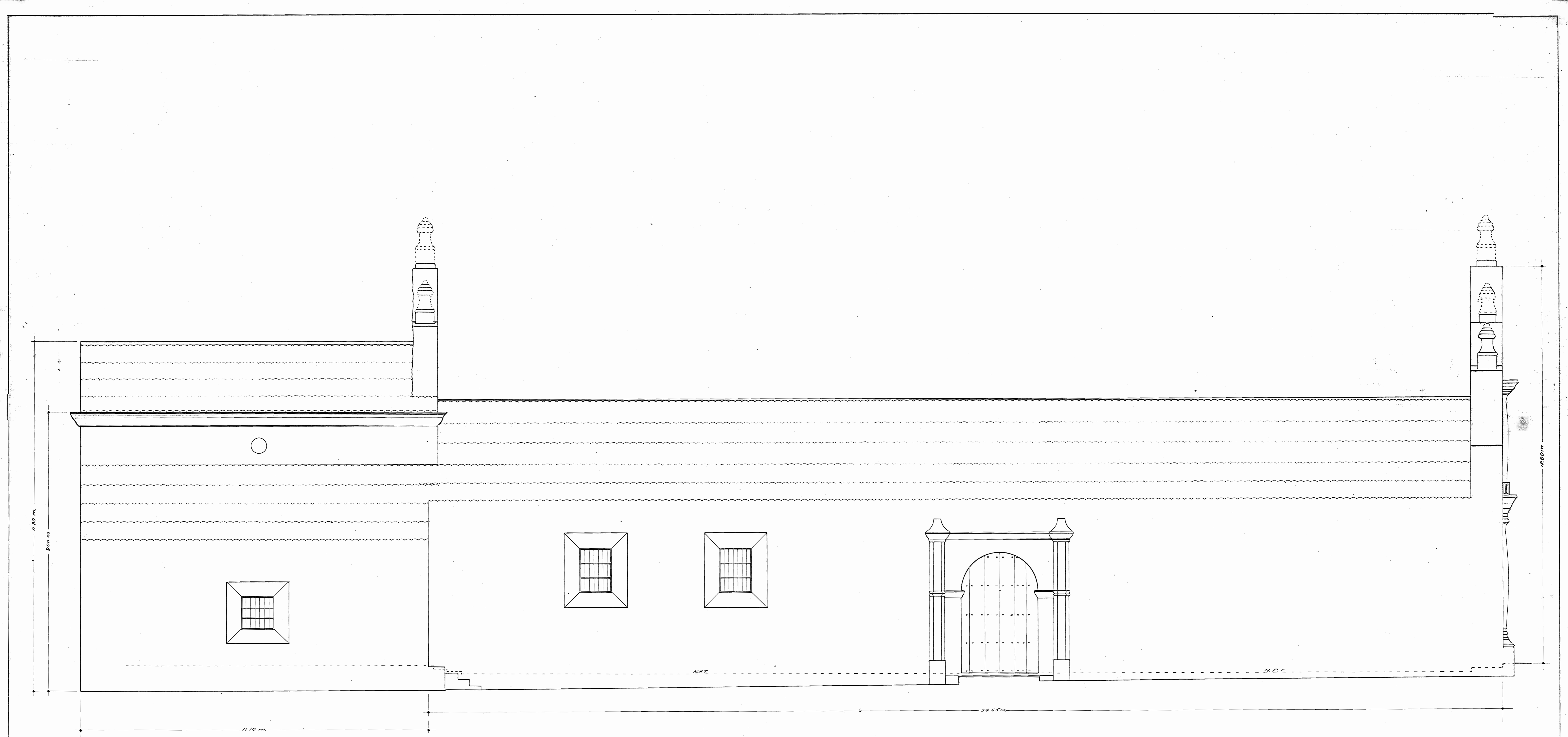
FACHADA NORTE Escala 1:50
