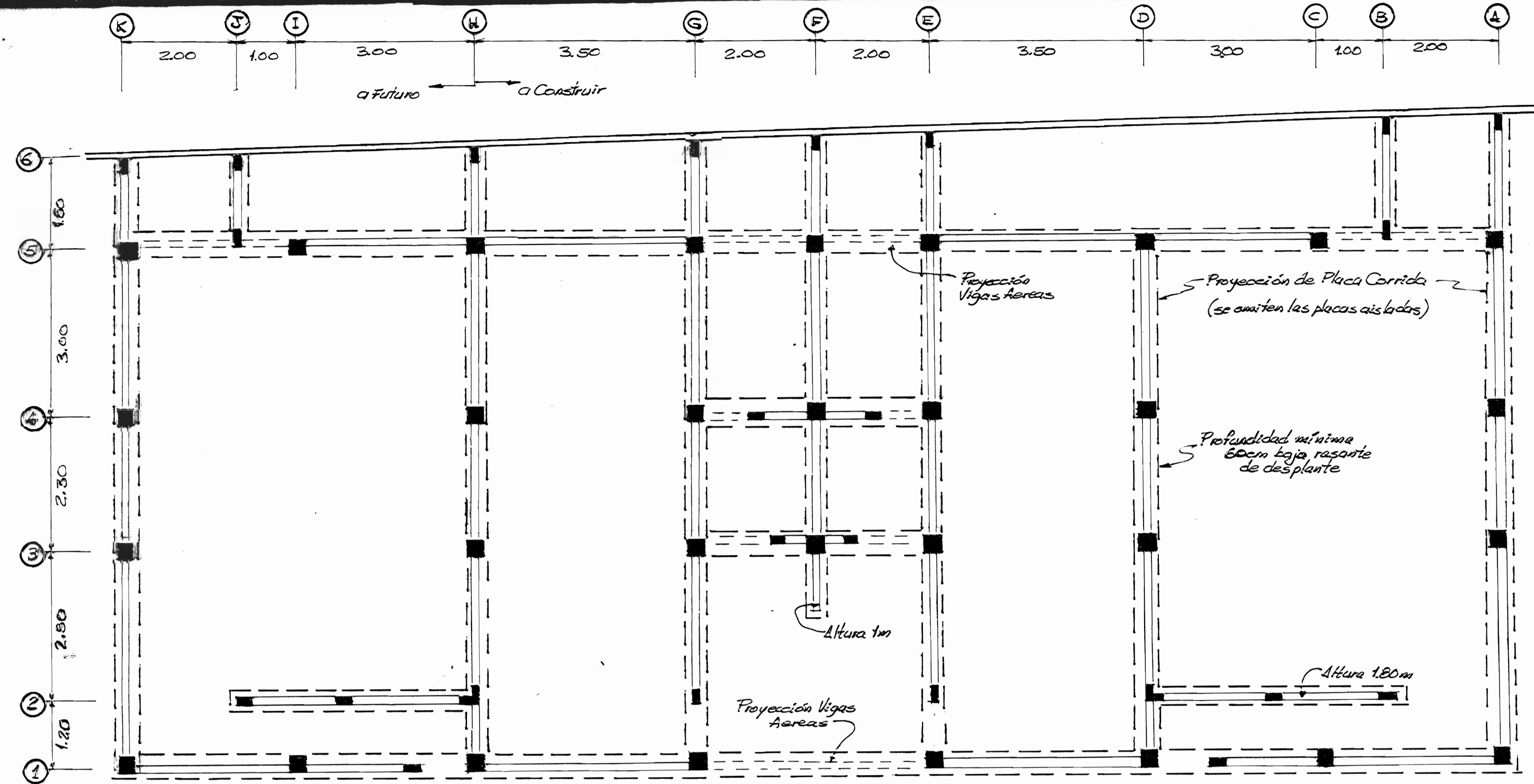
CIENTOS Y COLUMNAS (Ejes Estructurales)
