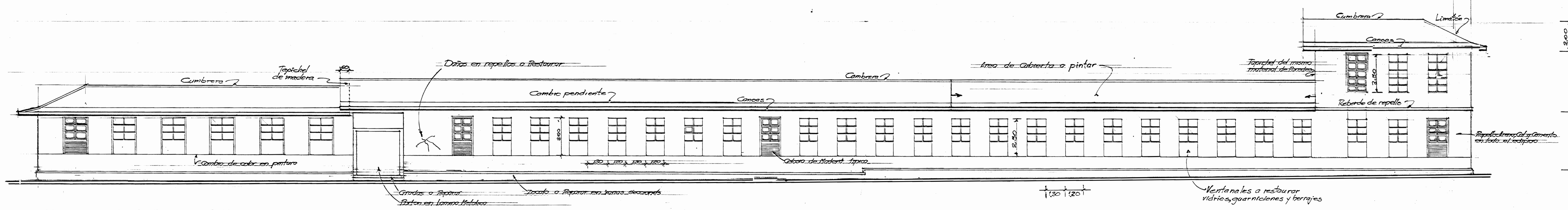
FACHADA ÉSTE PABELLON 3 Esc. 1:100
