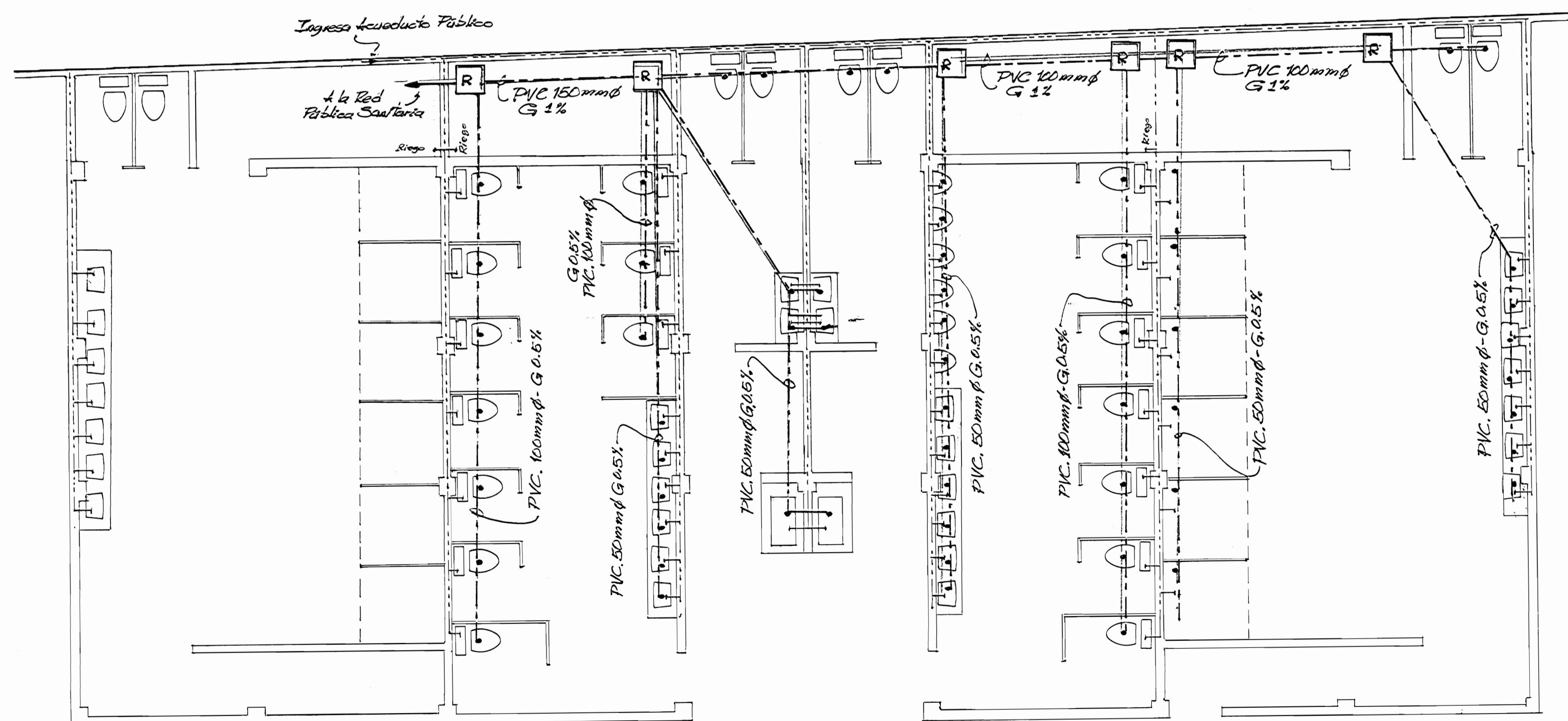
INSTALACION MECANICA
