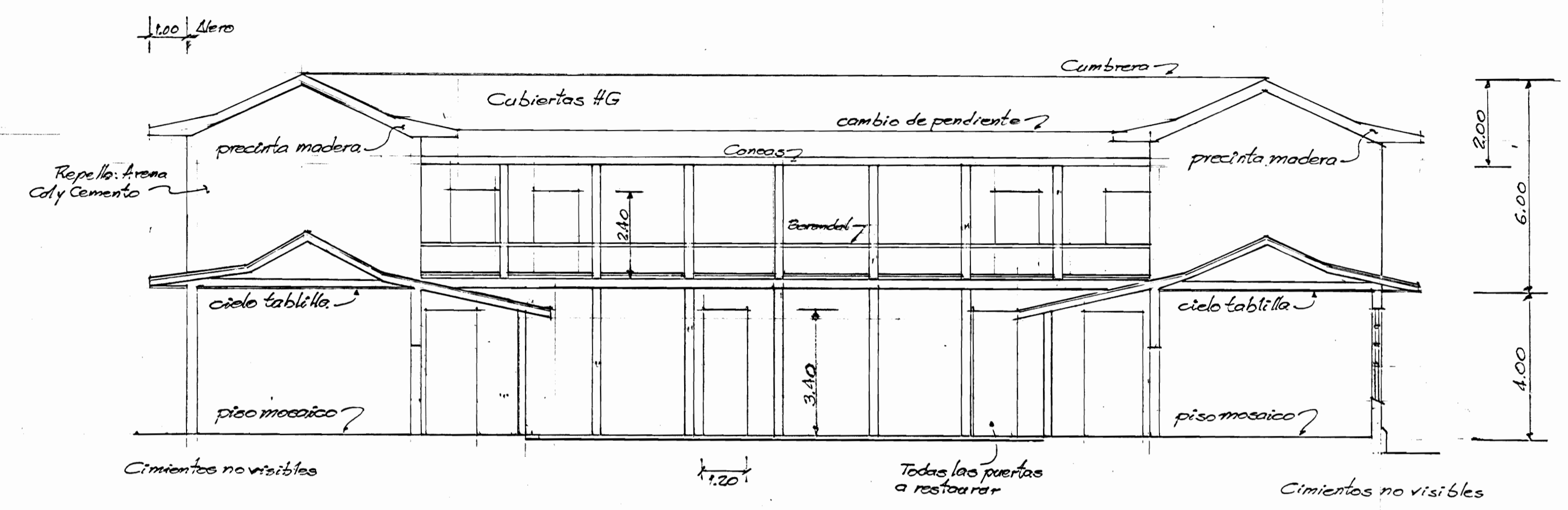
FACHADA SUR PABELLON 2 Esc. 1:100
