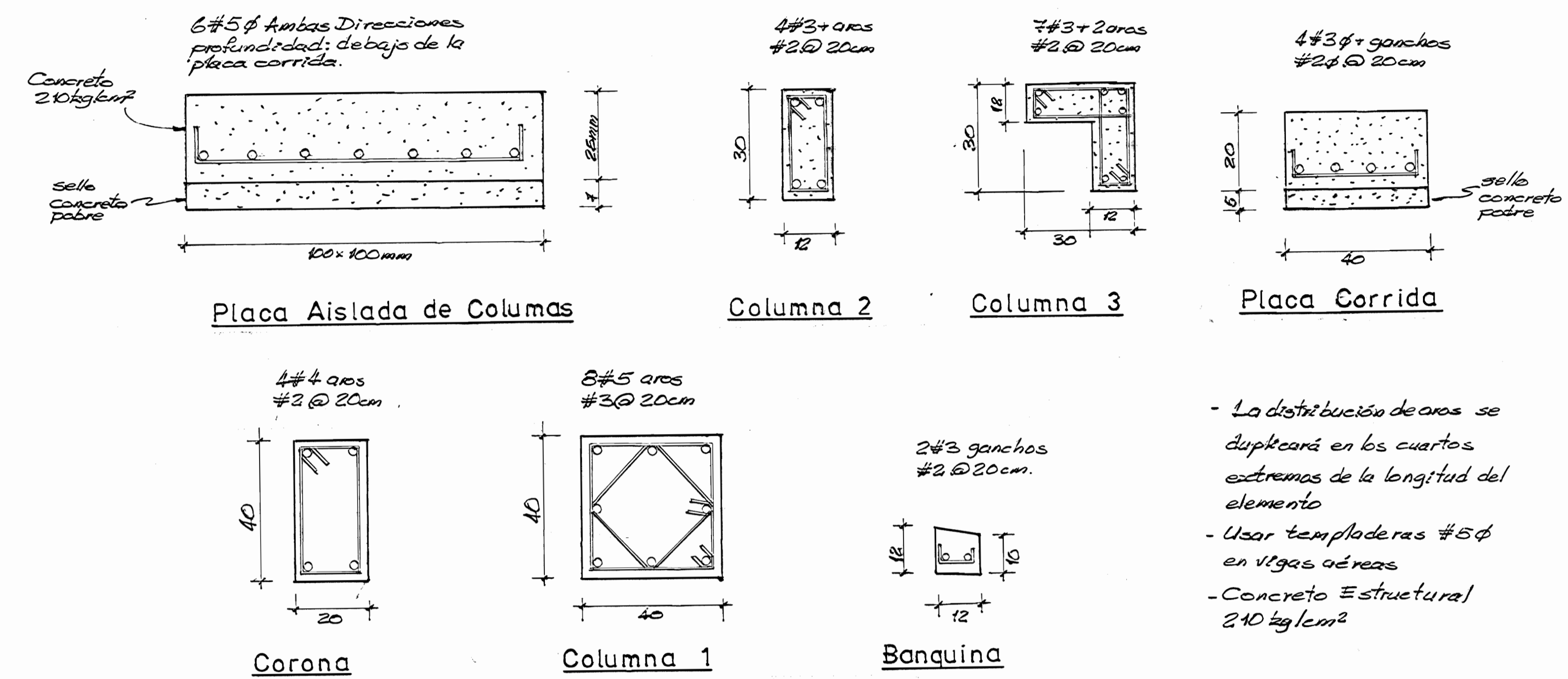
SECCIONES ESTRUCTURALES
