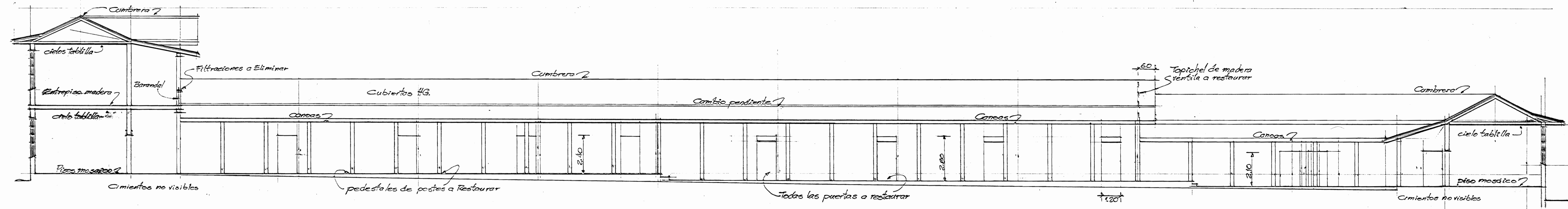
CORTE Y FACHADA OESTE PABELLON 3 Esc. 1:100
