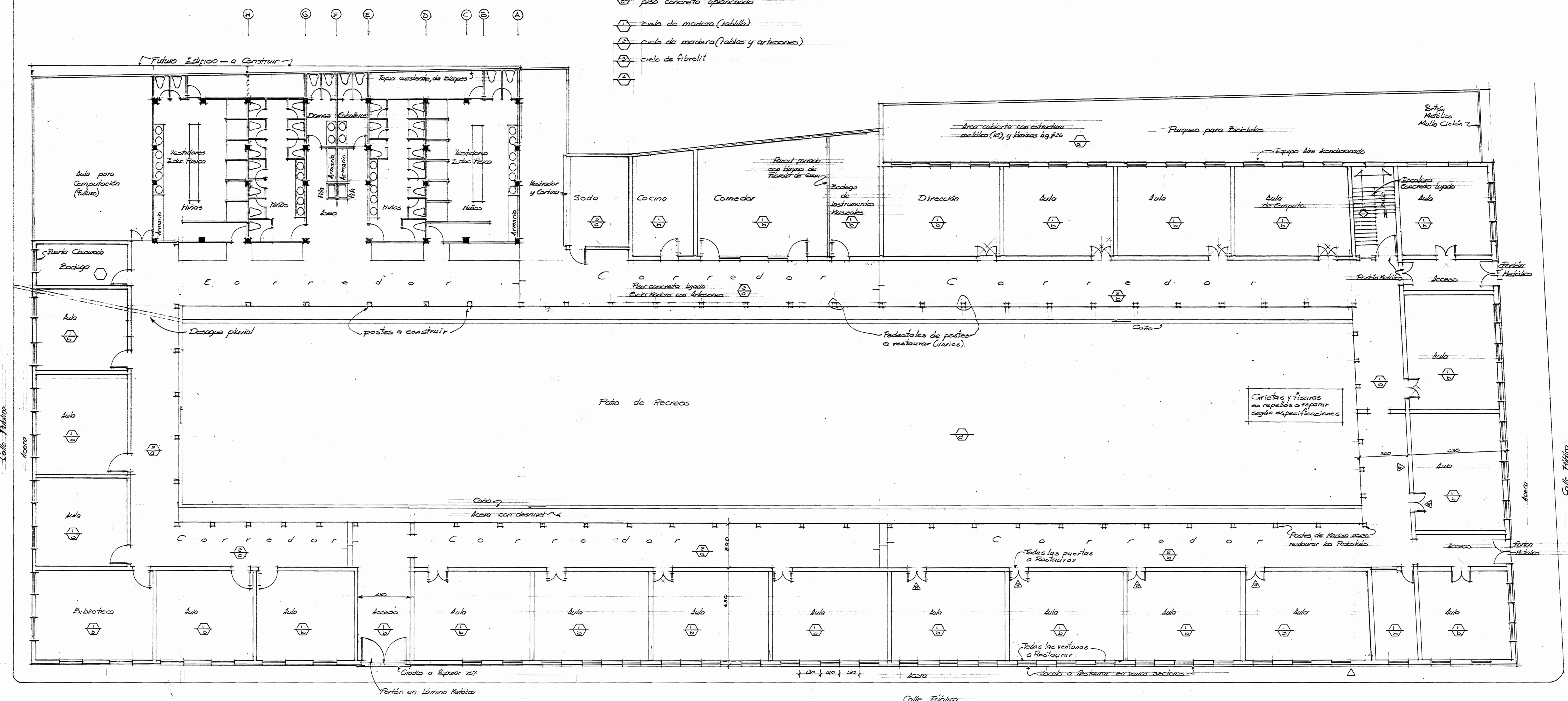
Planta Principal Existente Mostrando Sanitarias y Vestidores a Construir ESC 1:100
