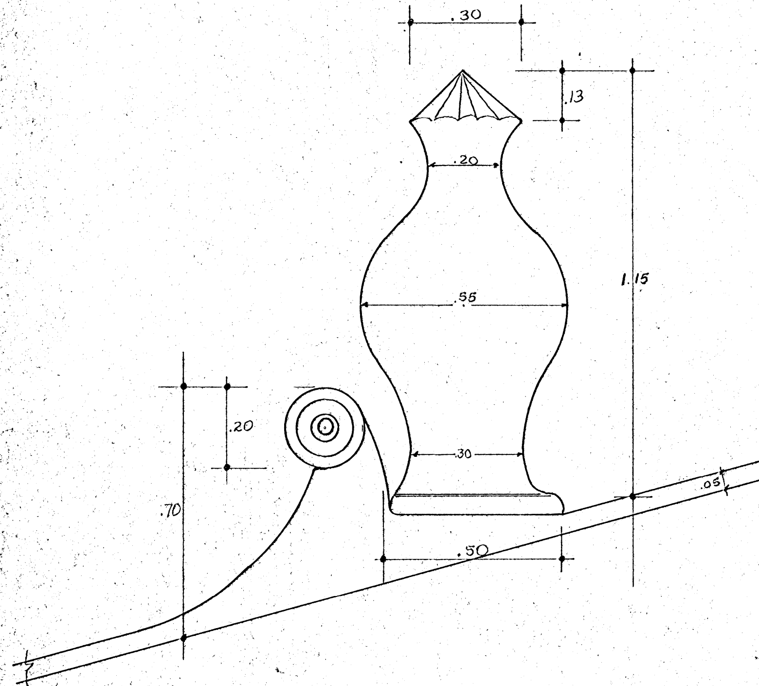
DET. DE ADORNO EN FACHADA Esc 1:10
