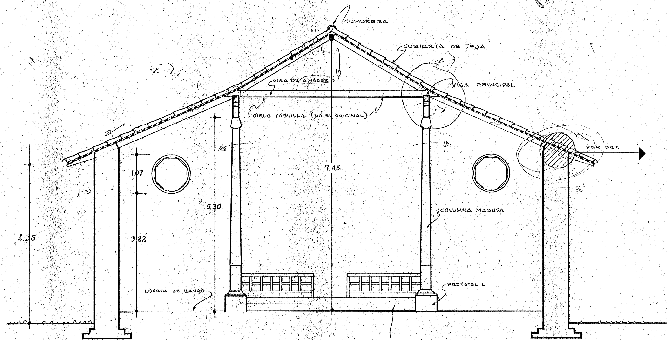
SECCION POR B-B Esc 1:50
