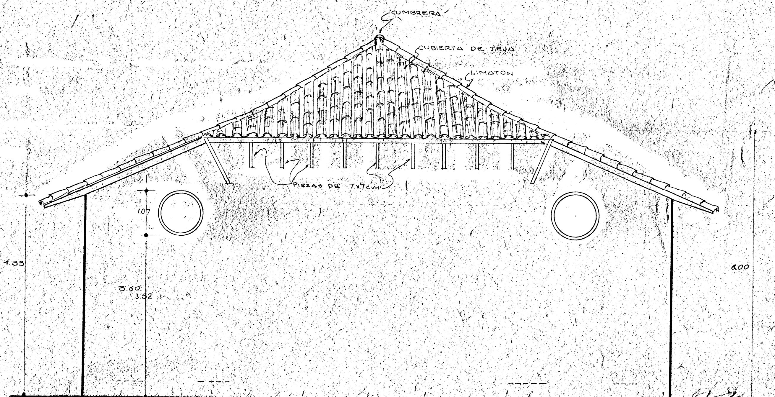
FACHADA POSTERIOR Escala 1/50
