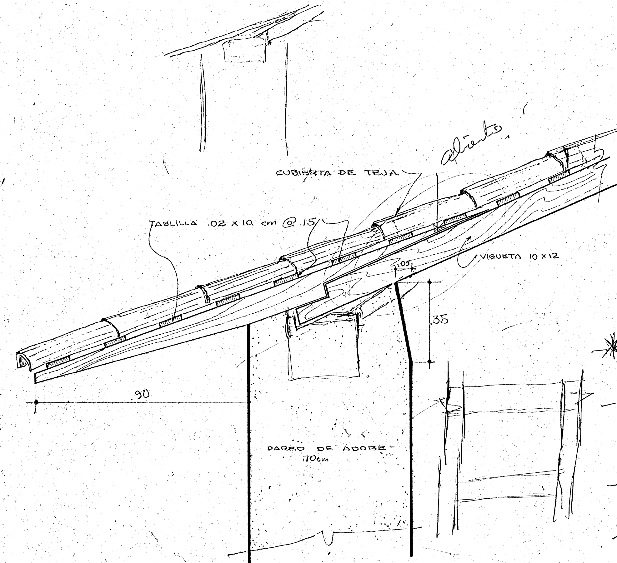
DET. DE UNION DE ALERO Y VIGUETA Esc 1:10
