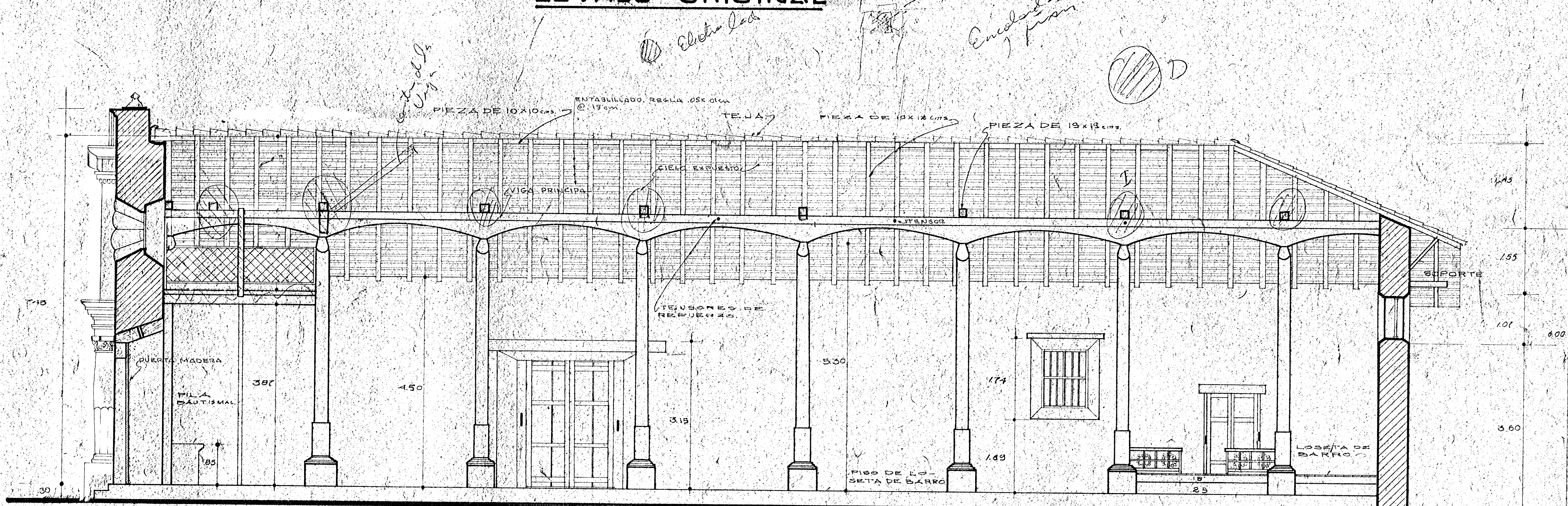
CORTE POR C-C Escala 1/50
