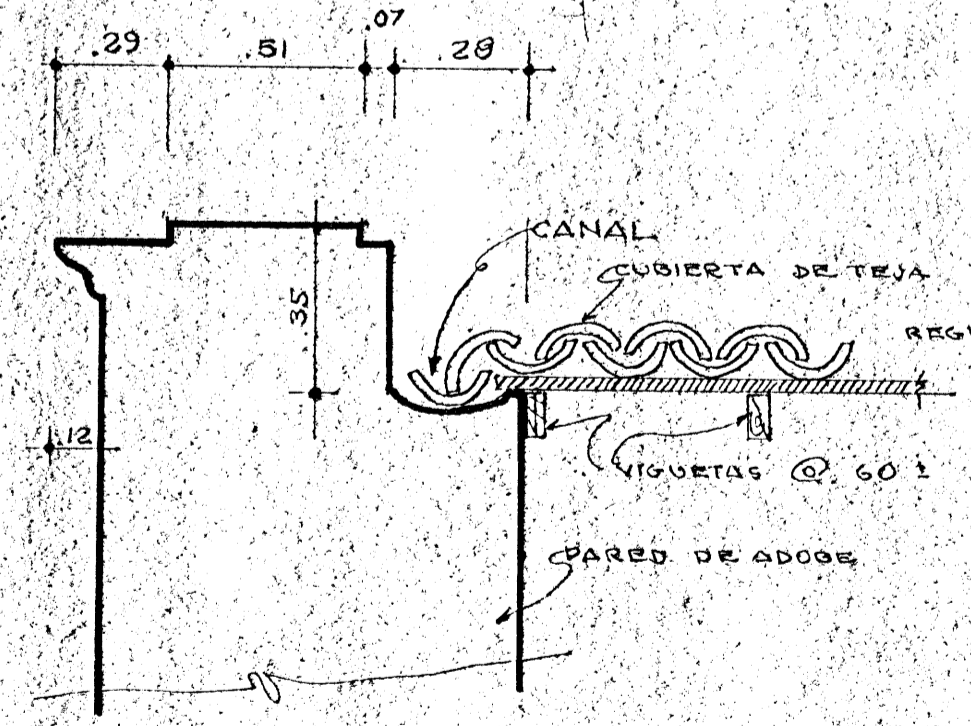
SECCION 1-1 DET. DE PARED Ene 1:20
