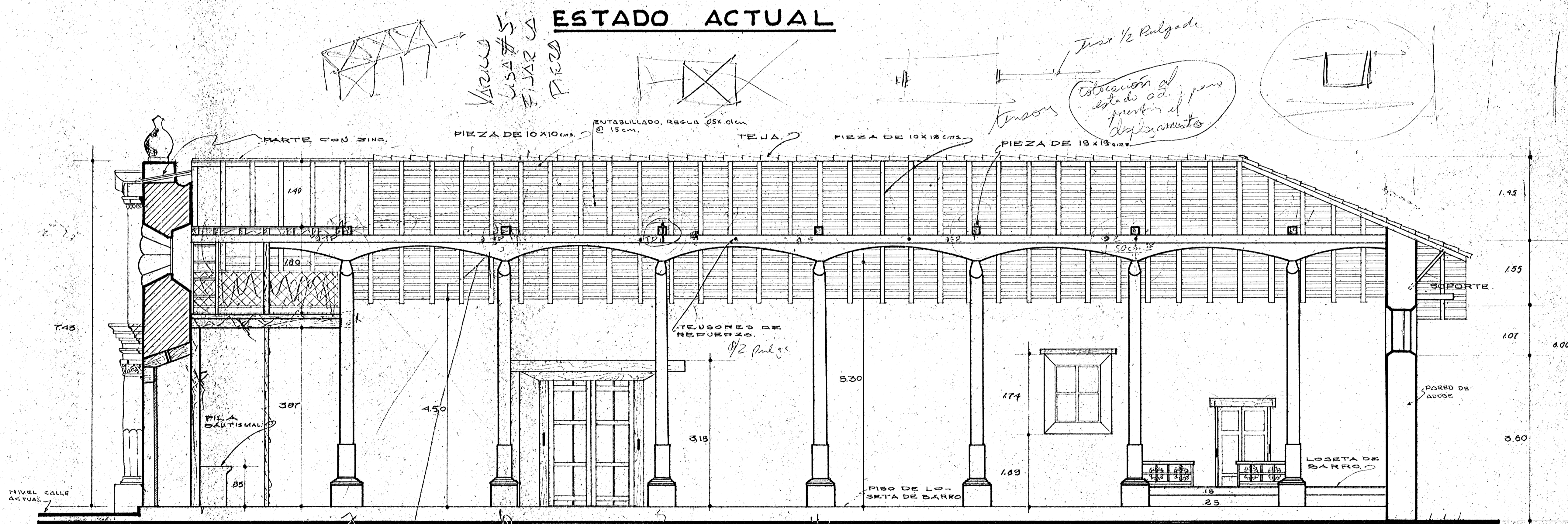
CORTE POR C-C. escala 1:50
