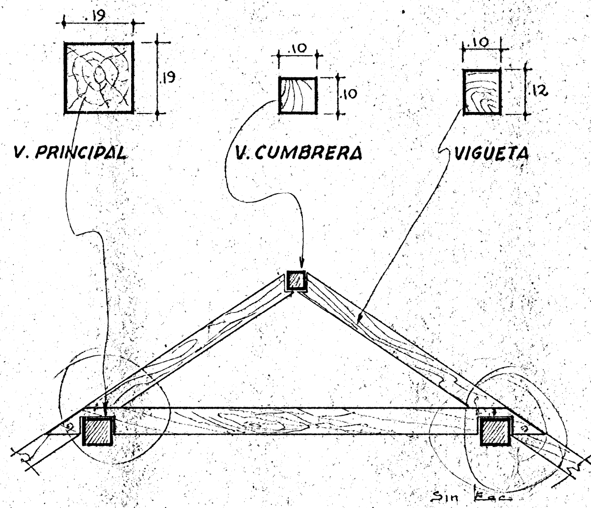
DET. DE VIGAS Y VIGUETAS DE MADERA
