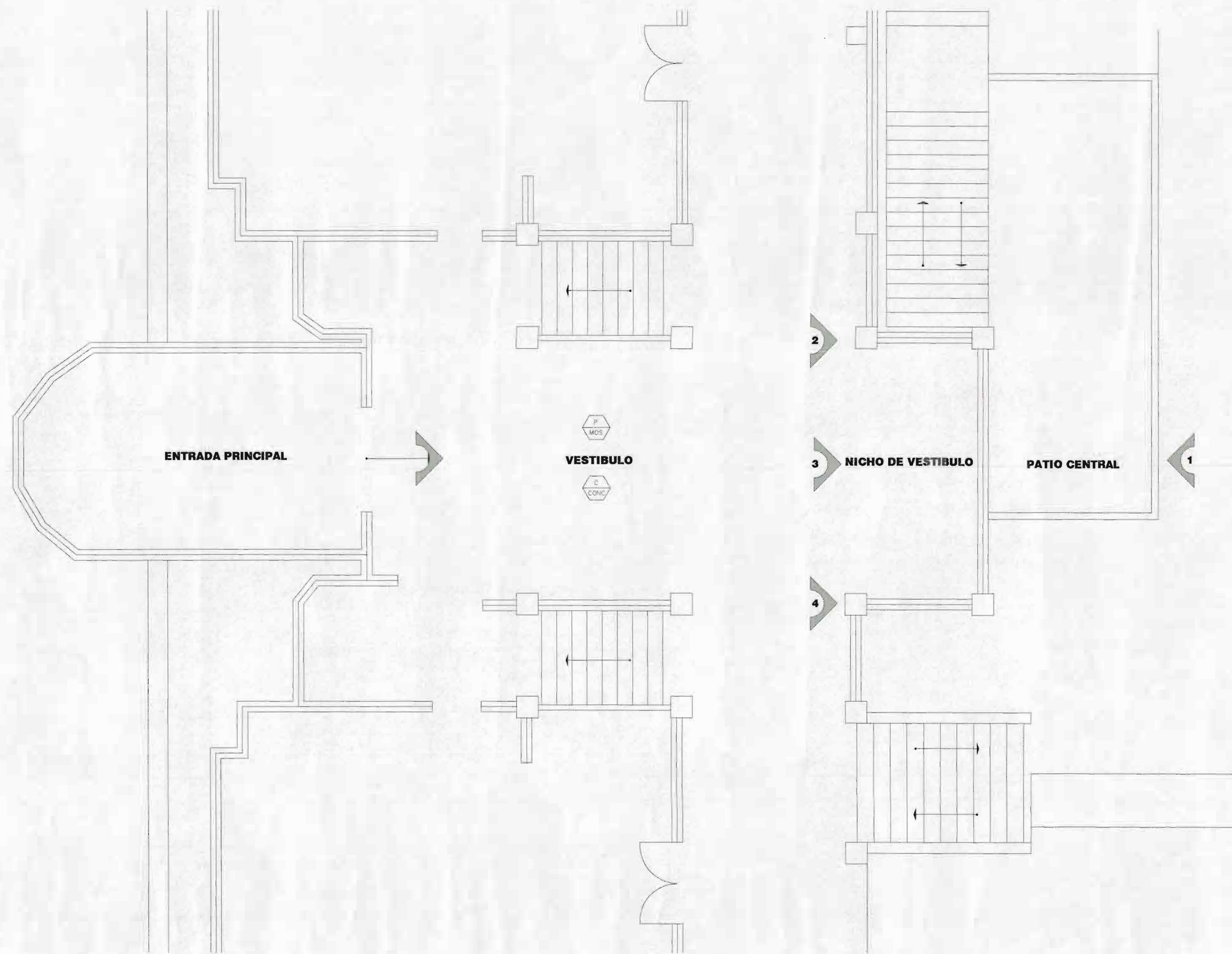
PLANTA ARQUITECTONICA DEL VESTIBULO
