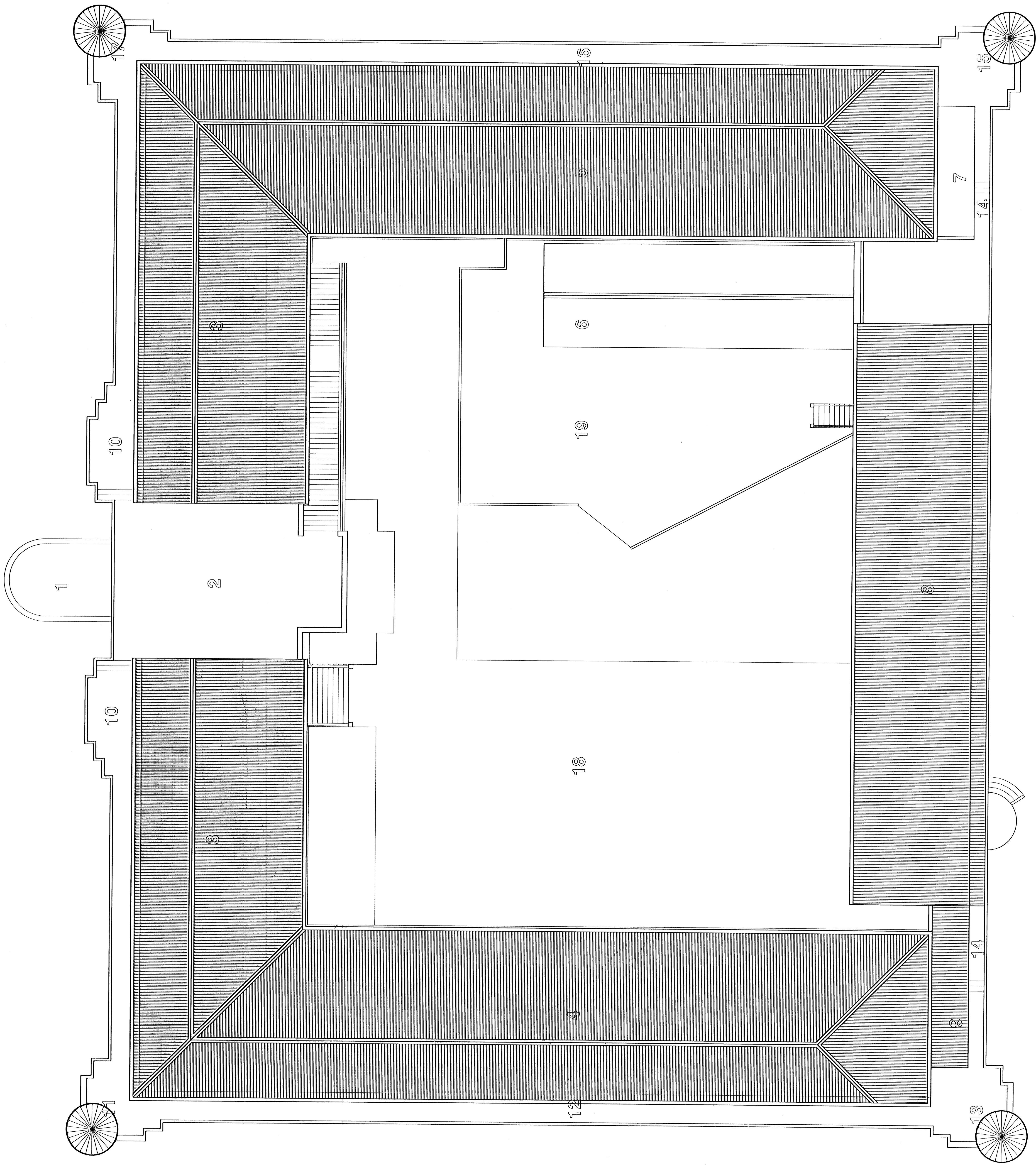
PLANTA DE TECHOS ESC. 1 : 100
