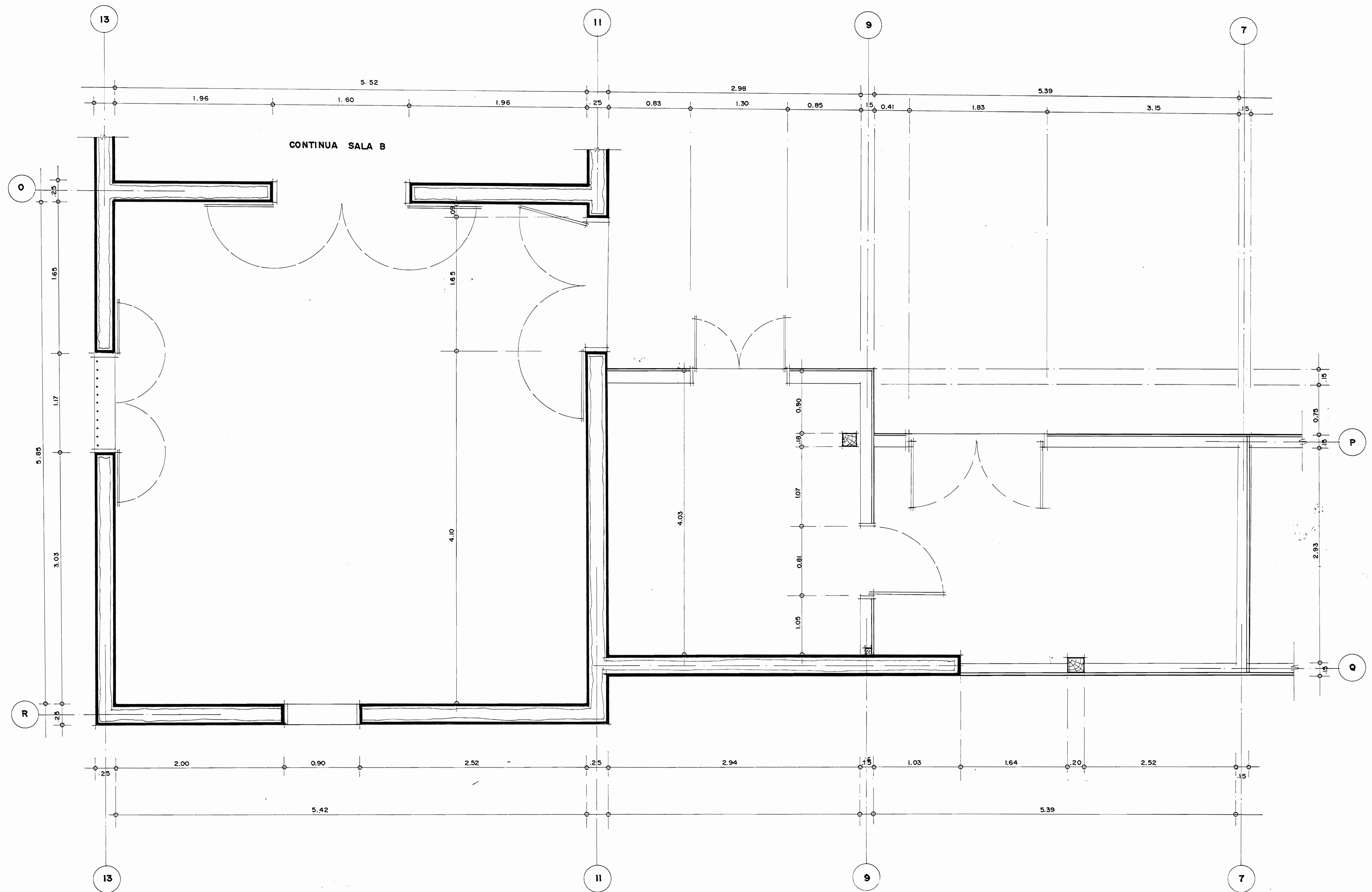
PLANTA MUSEOGRAFICA SALA C, ORATORIO Y SACRISTIA GIRADO 90° A LA DERECHA
