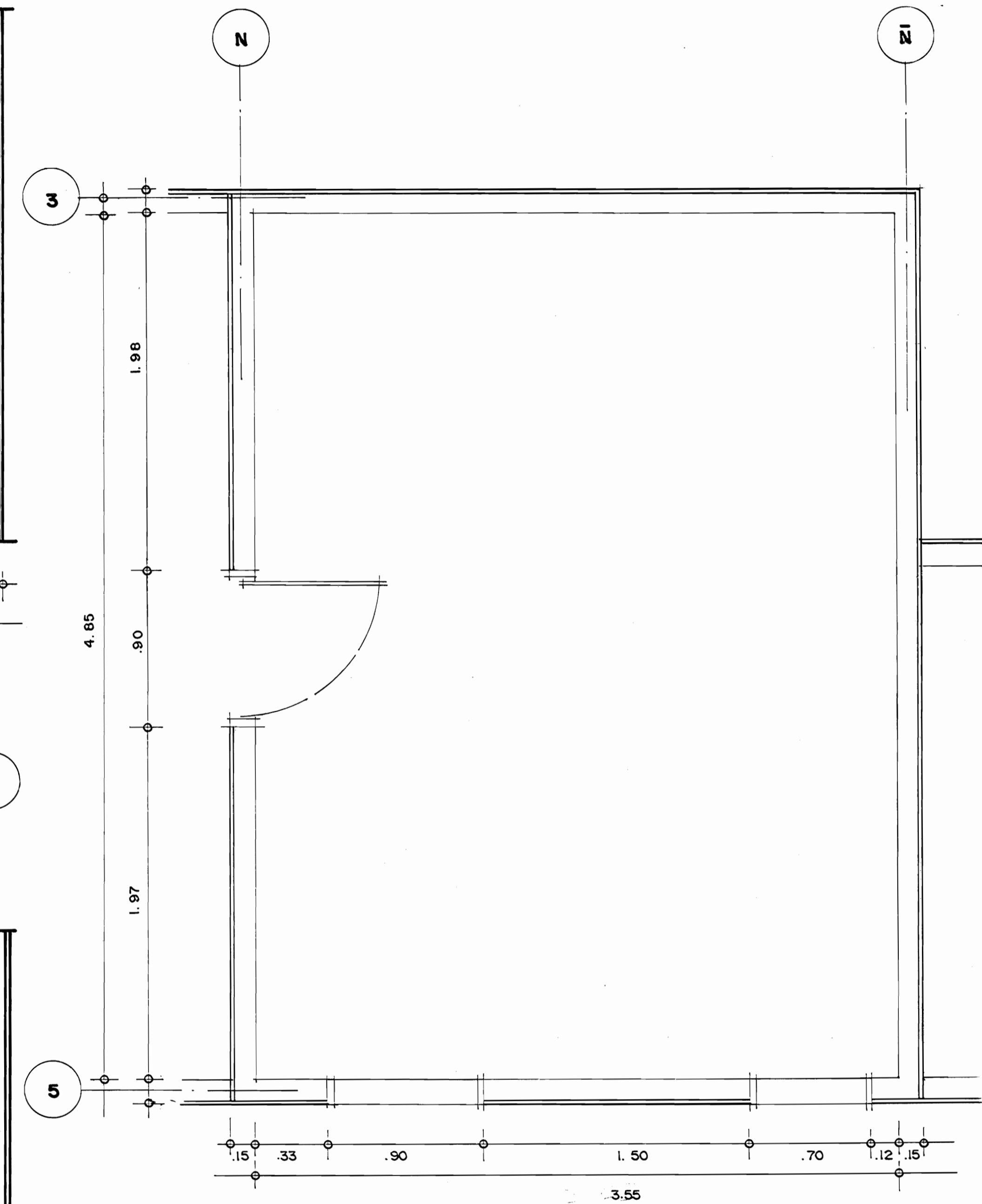
PLANTA MUSEOGRAFICA SALA E
