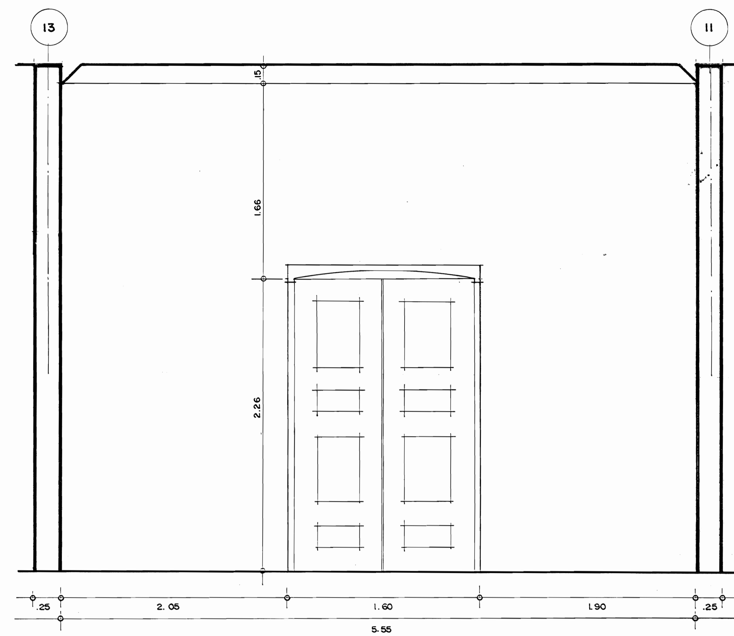
PLANO MUSEOGRAFICO OESTE
