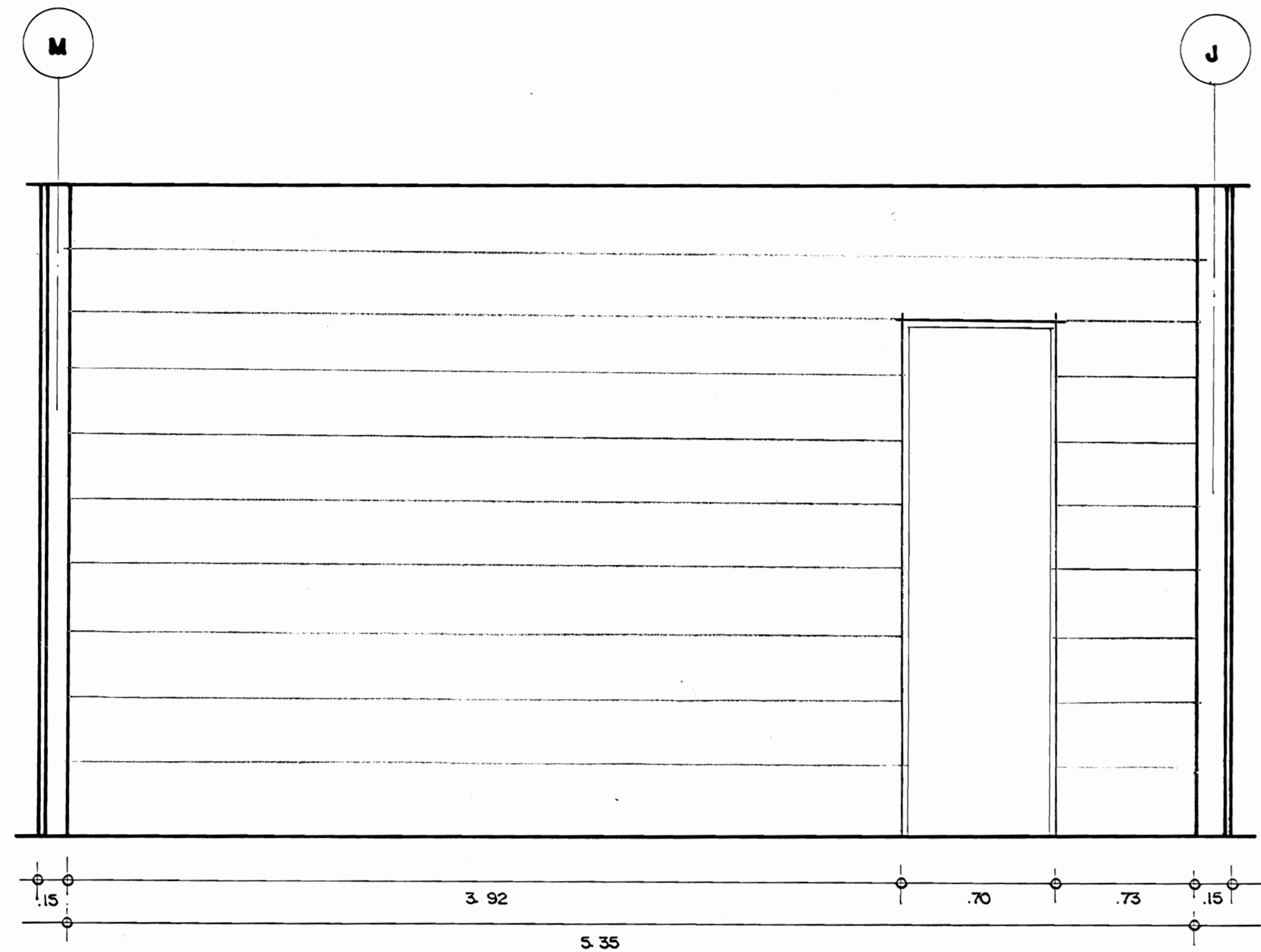
PLANO MUSEOGRAFICO SUR
