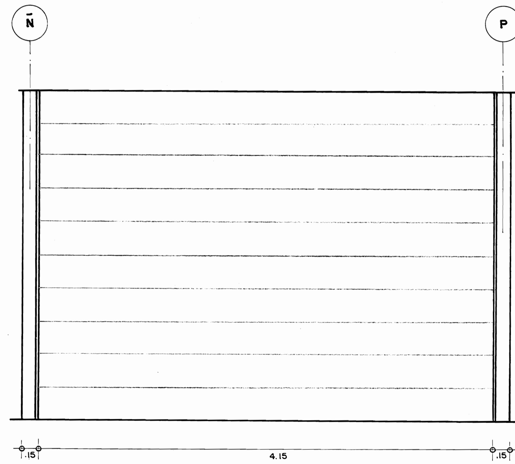
PLANO MUSEOGRAFICO NORTE
