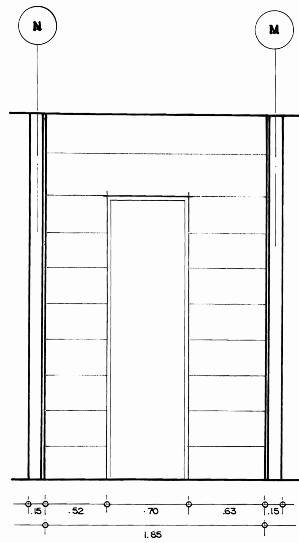
PLANO MUSEOGRAFICO SUR
