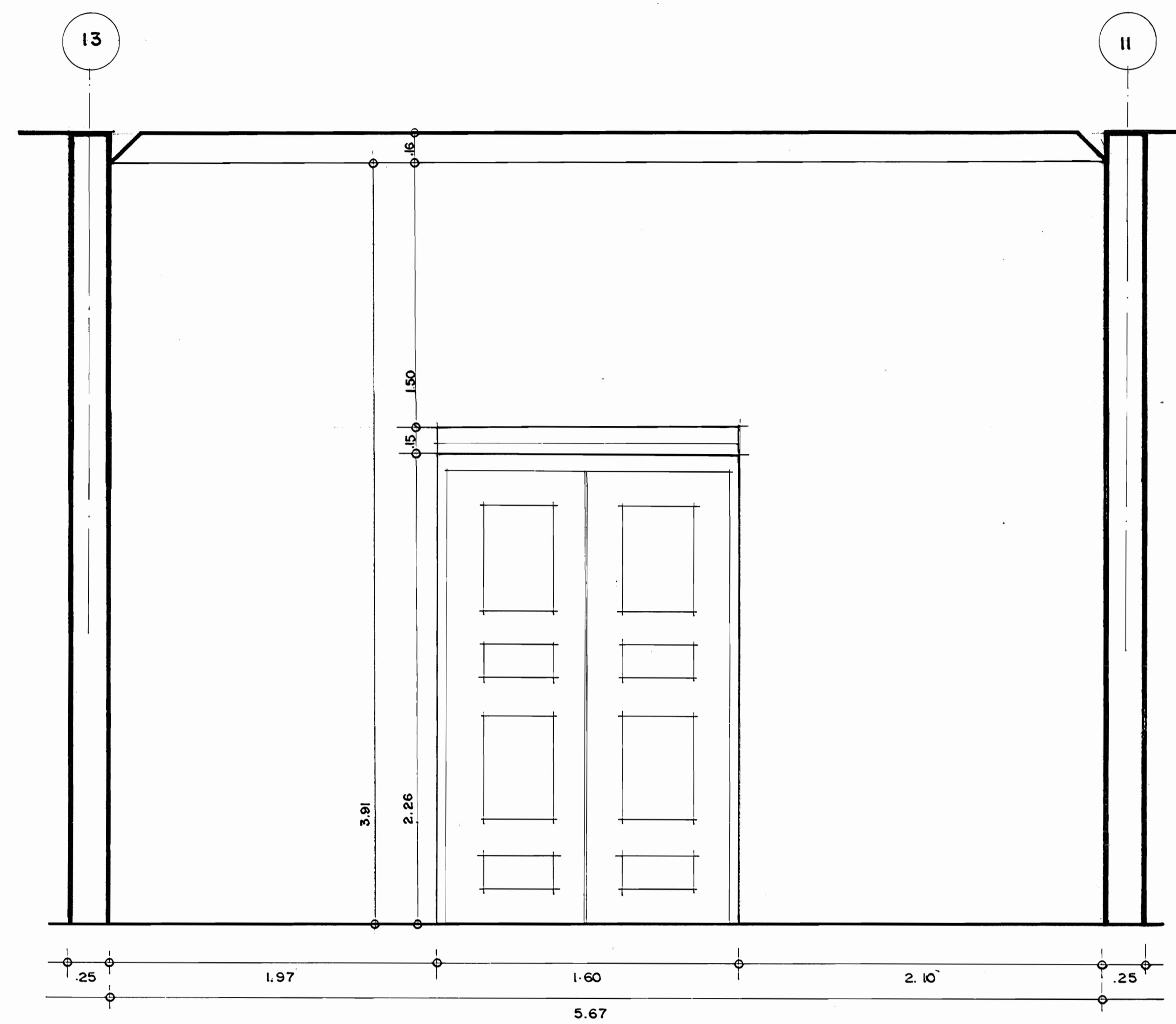
PLANO MUSEOGRAFICO OESTE
