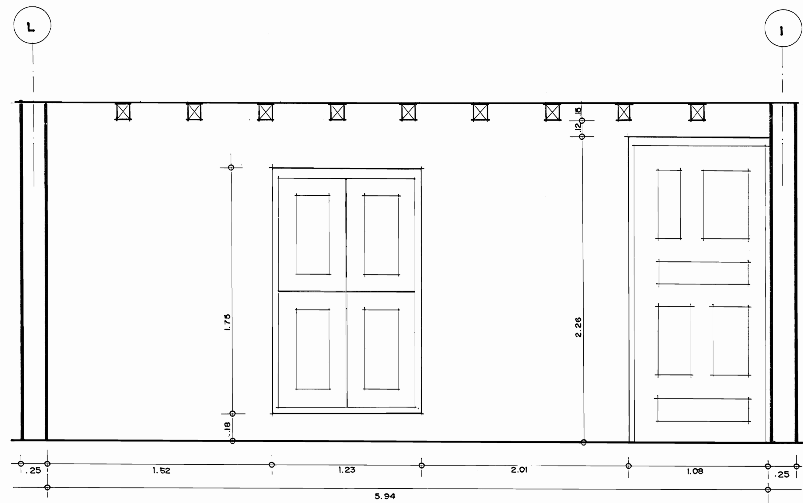
PLANO MUSEOGRAFICO SUR
