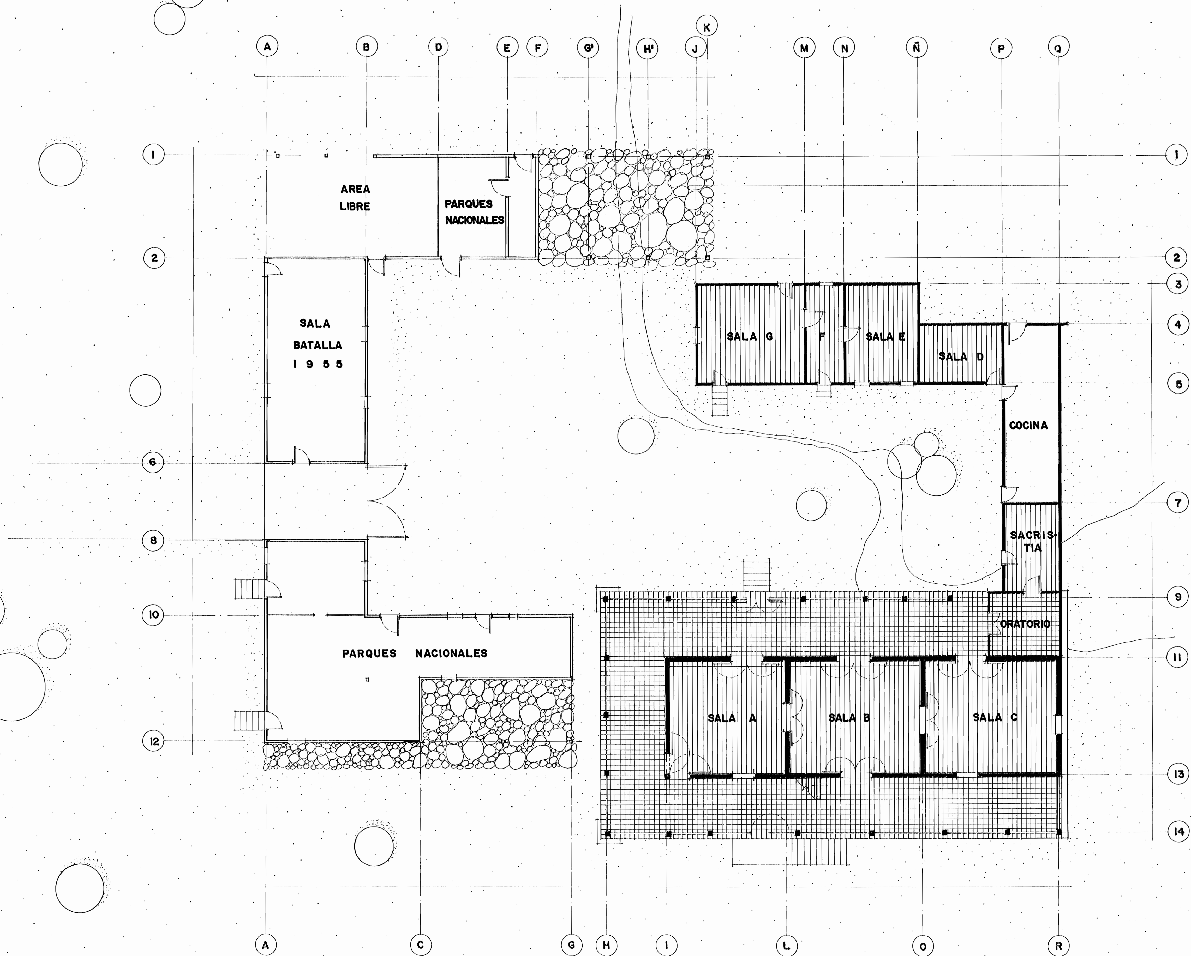
PLANTA DE CONJUNTO ESCALA 1:100
