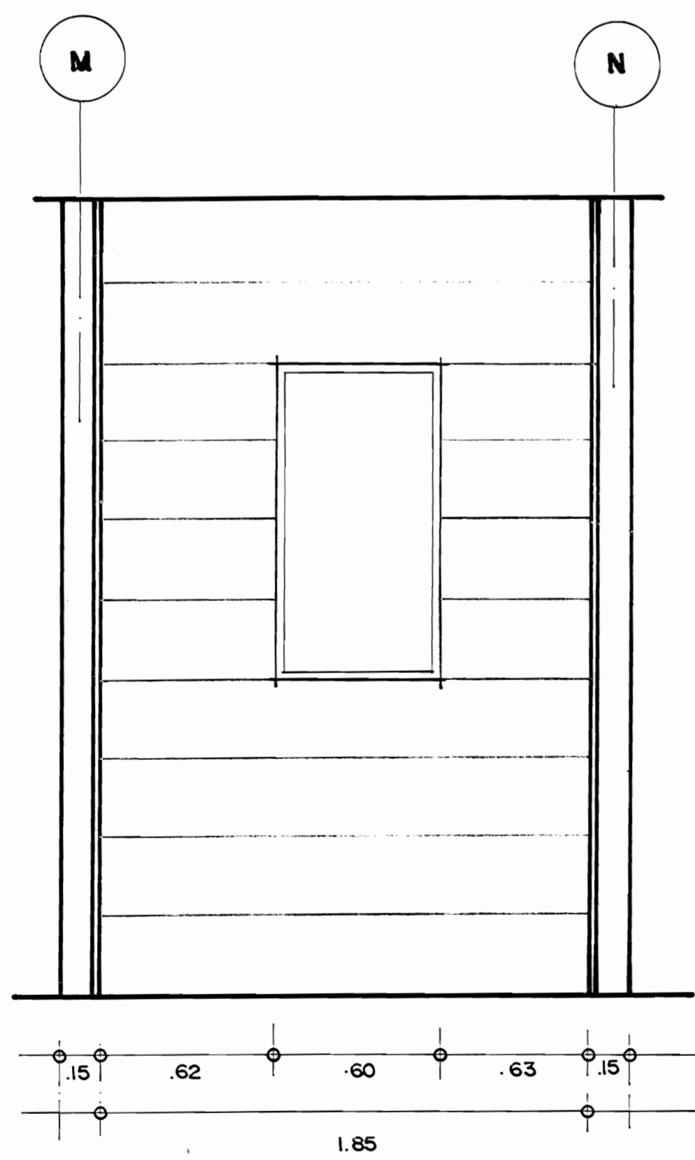
PLANO MUSEOGRAFICO NORTE
