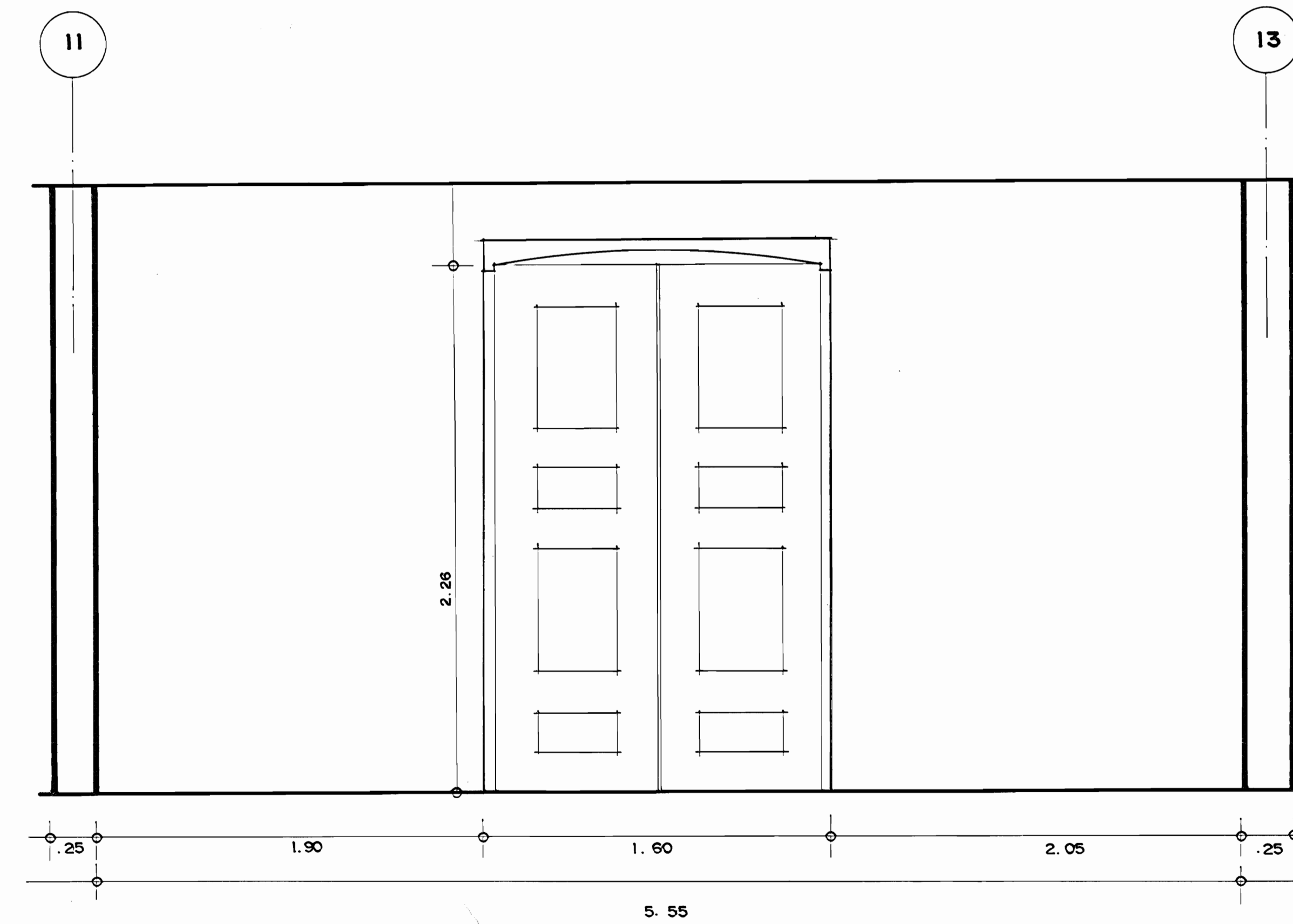
PLANO MUSEOGRAFICO ESTE
