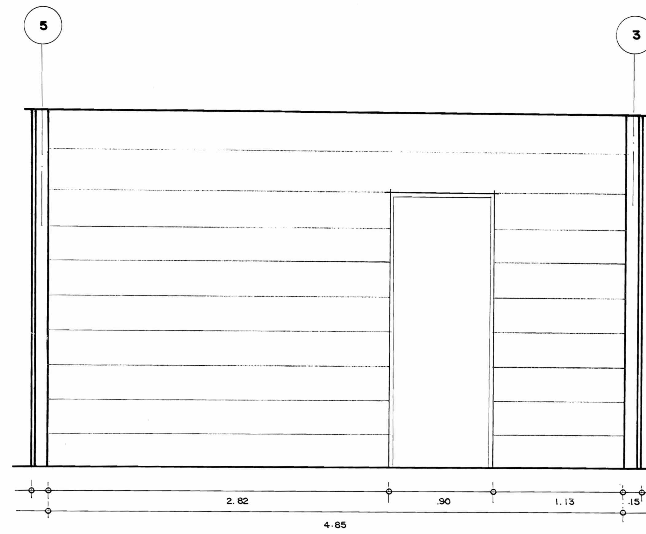
PLANO MUSEOGRAFICO OESTE
