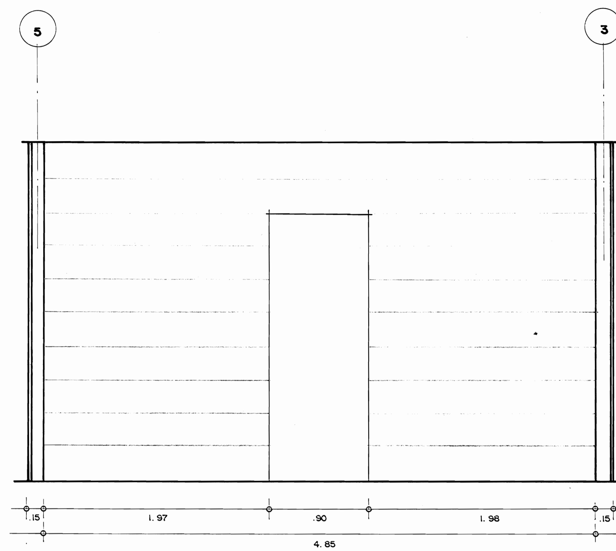
PLANO MUSEOGRAFICO OESTE
