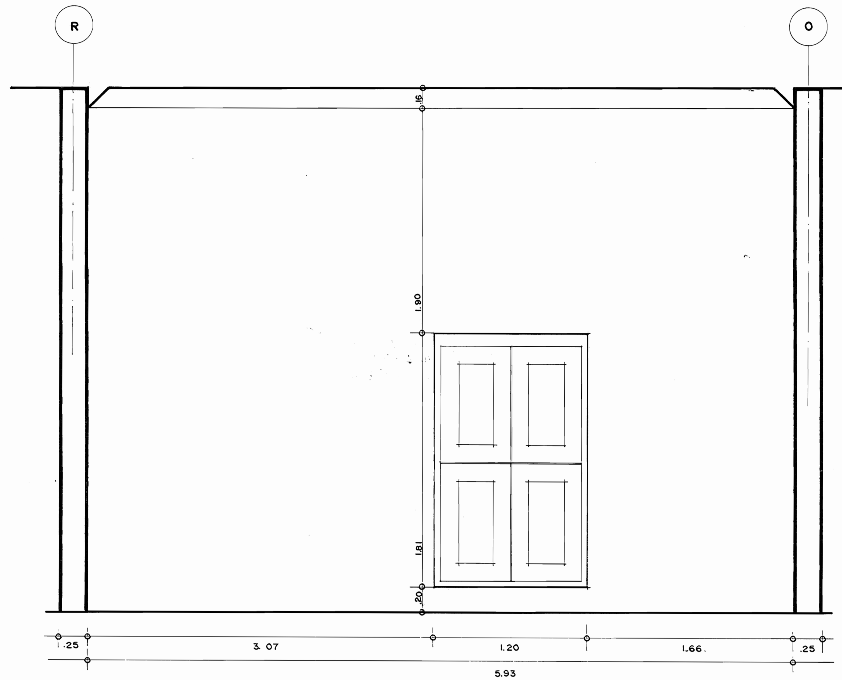
PLANO MUSEOGRAFICO SUR
