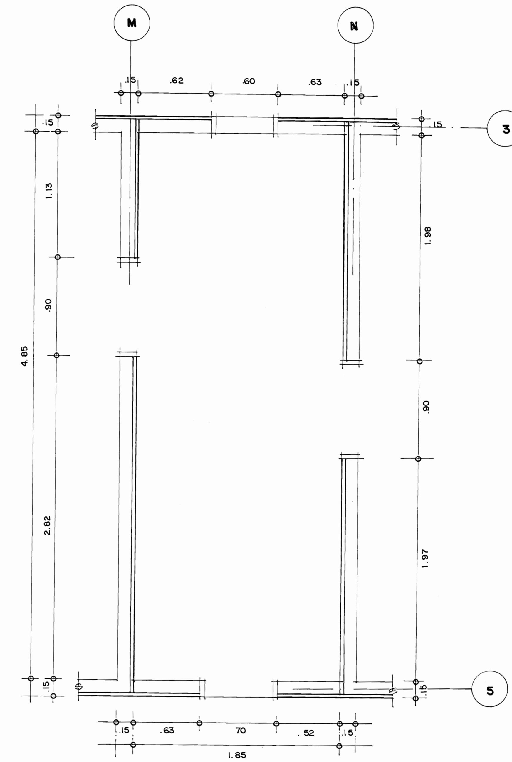
PLANTA MUSEOGRAFICA SALA F
