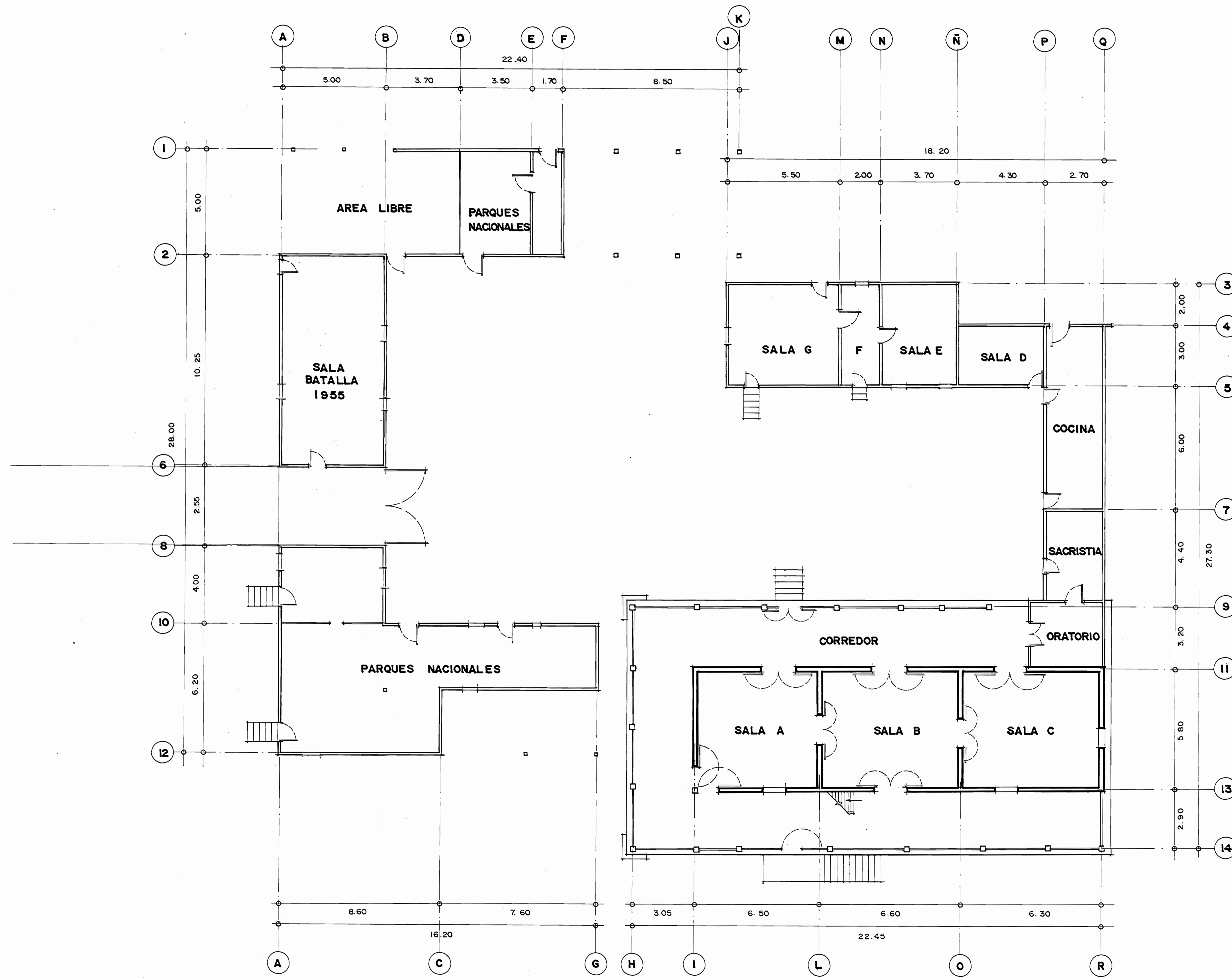
PLANTA DE CONJUNTO ESCALA 1:100
