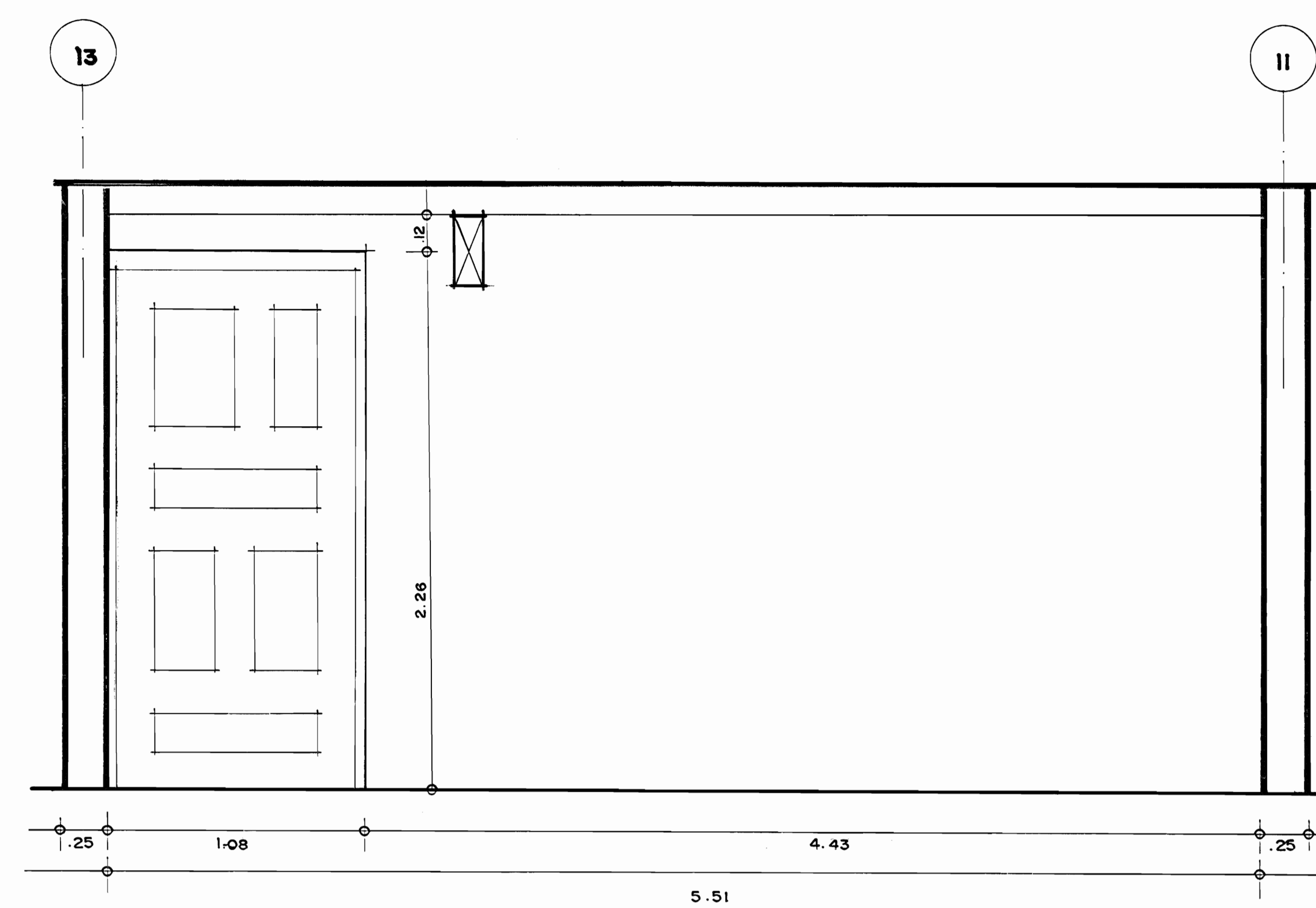
PLANO MUSEOGRAFICO OESTE
