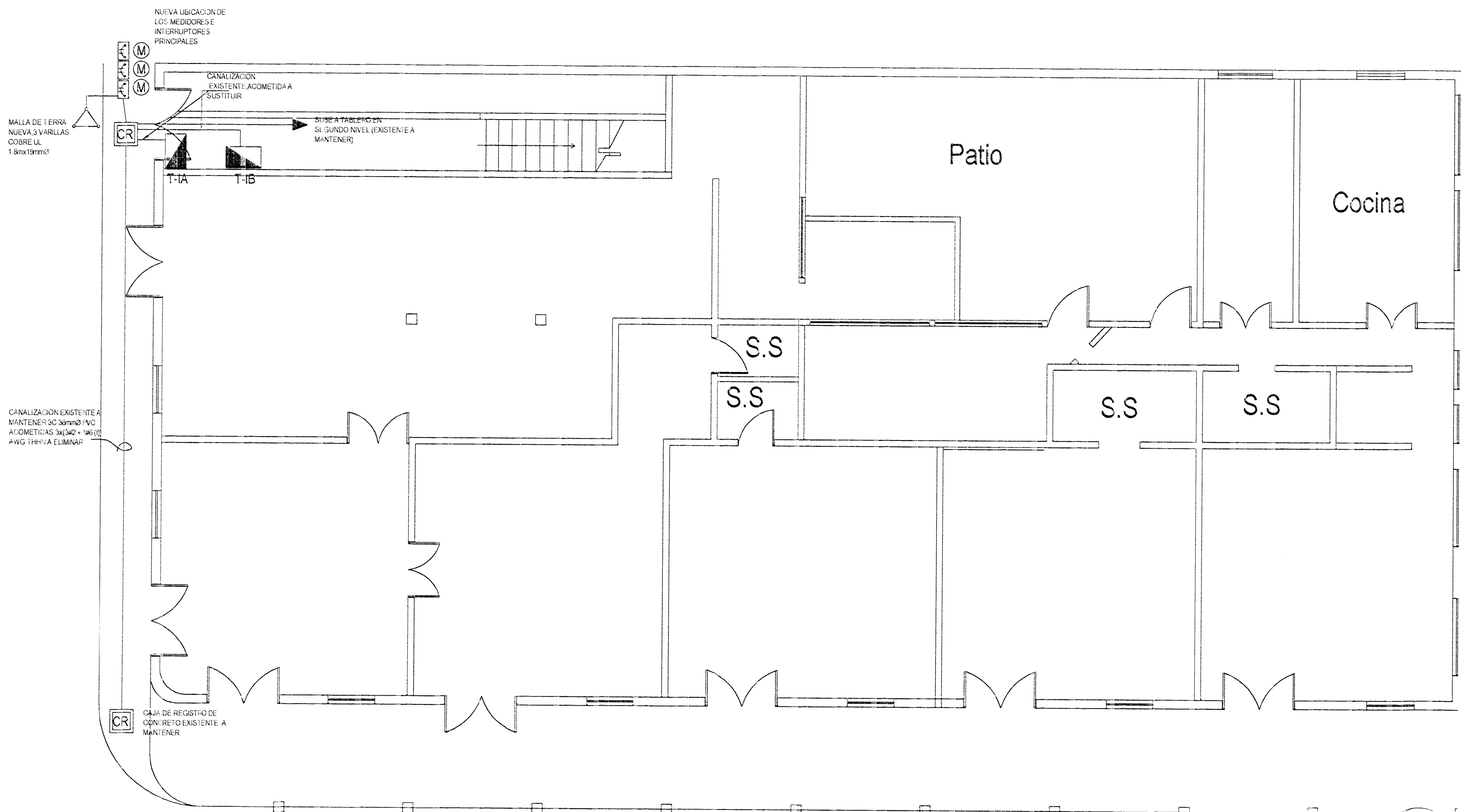
PLANTA DE DISTRIBUCION DE REUBICACION DE ACOMETIDA ELECTRICA
