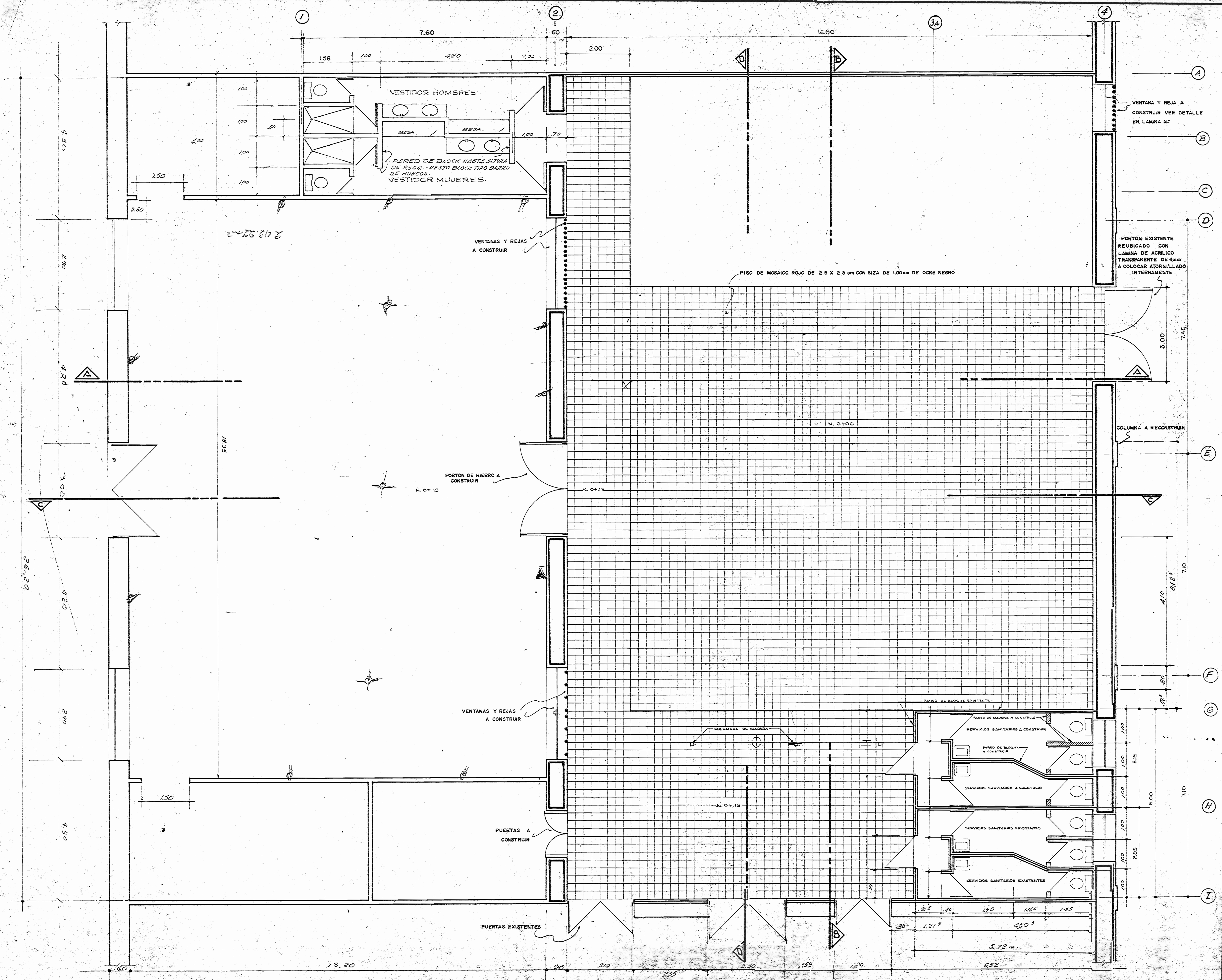
PLANTA ARQUITECTONICA PROPUESTA. ESCALA 1:50
