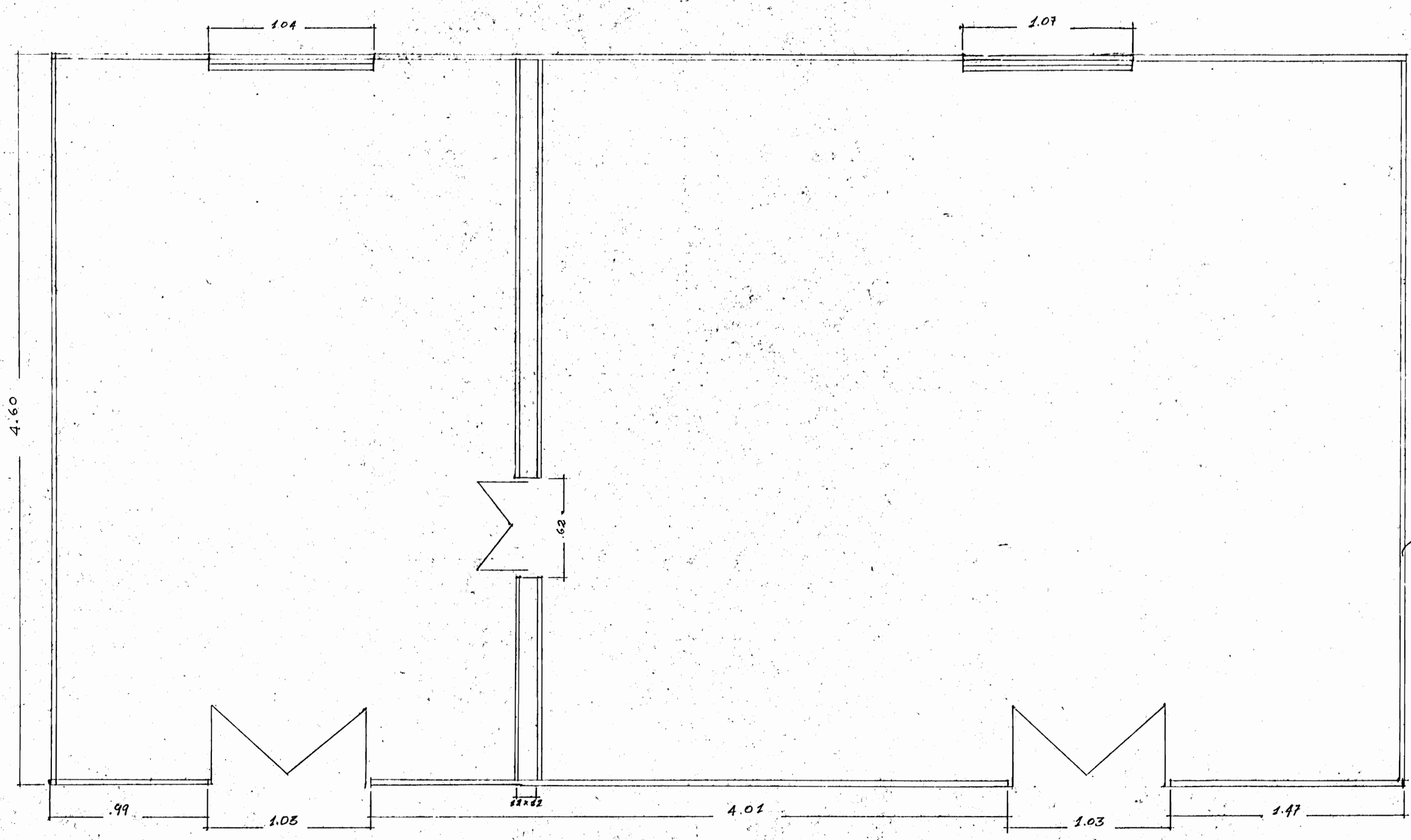
CASA DE REFUGIO EN OJO DE AGUA PEREZ ZELEDÓN DISTRIBUCIÓN ACTUAL ESC: 1:20
