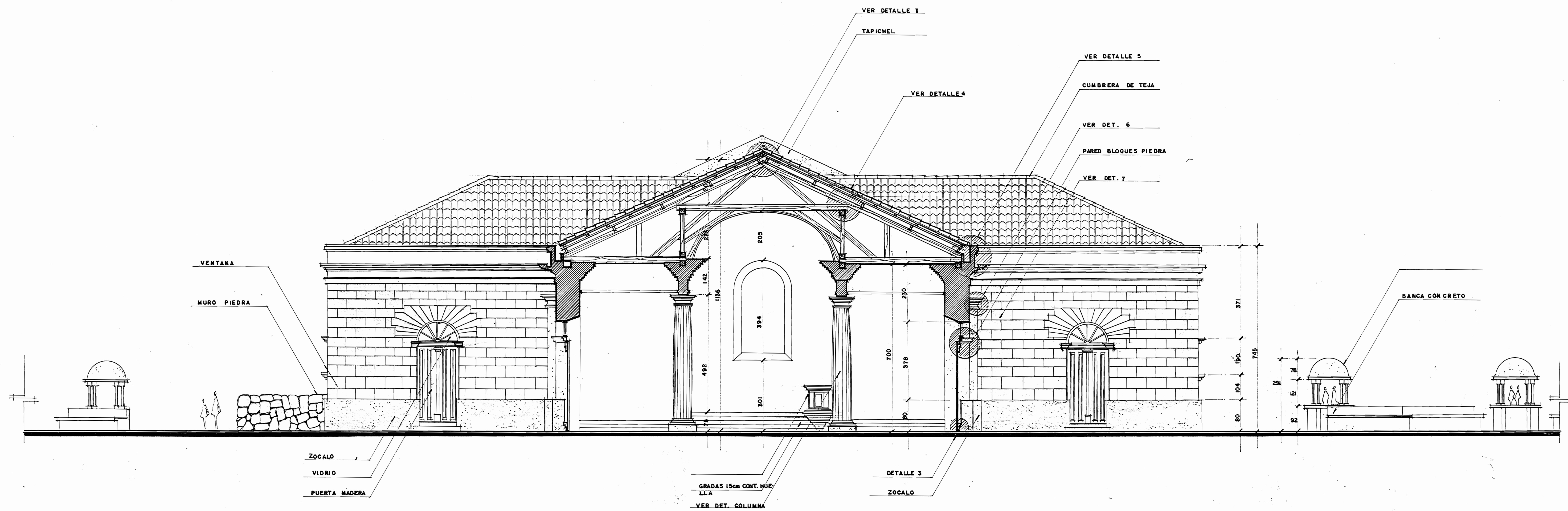
CORTE TRANSVERSAL ESTE ESC. 1:75
