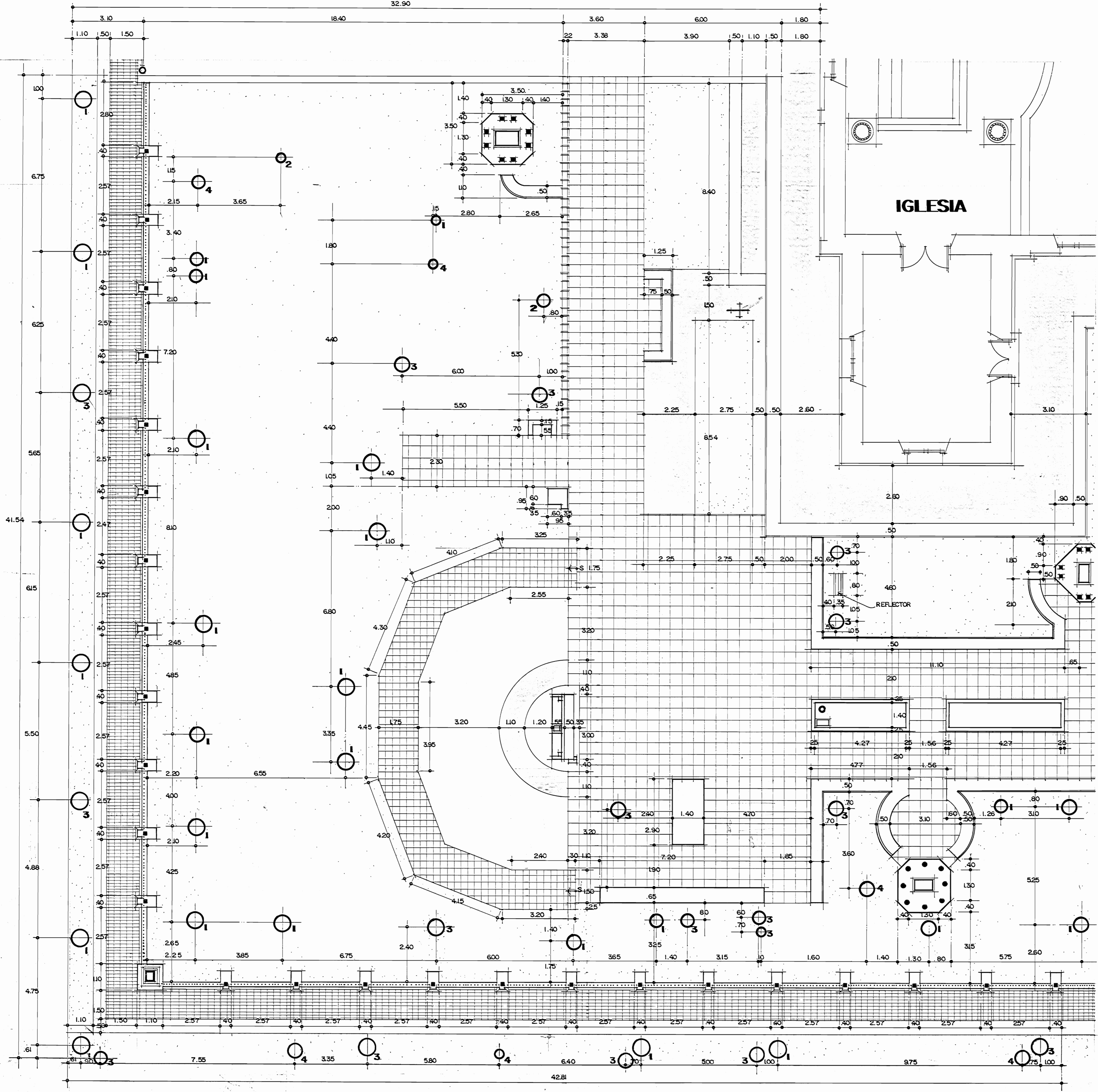
PLANTA SECTOR NORESTE
