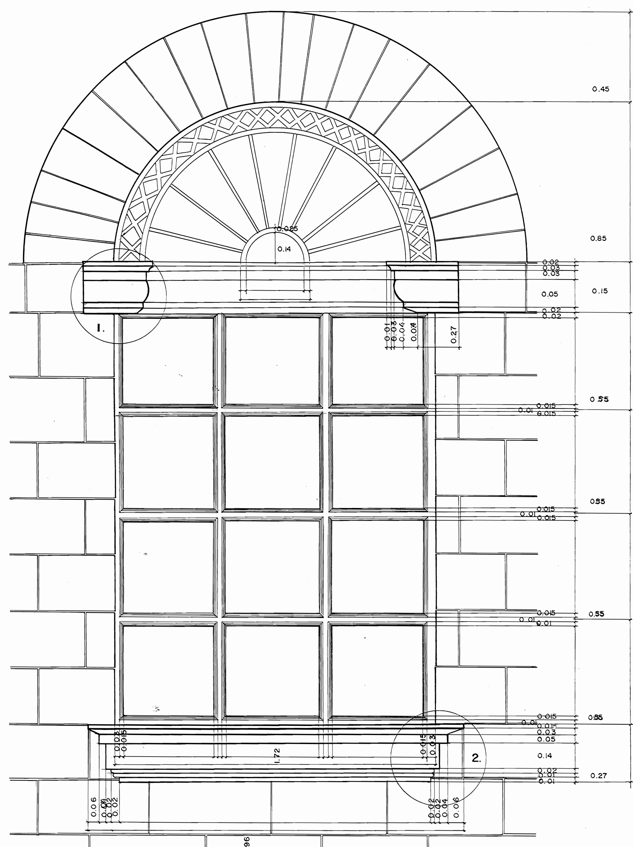
VENTANA CENTRAL _ FACHADA POSTERIOR. escala: 1:10.
