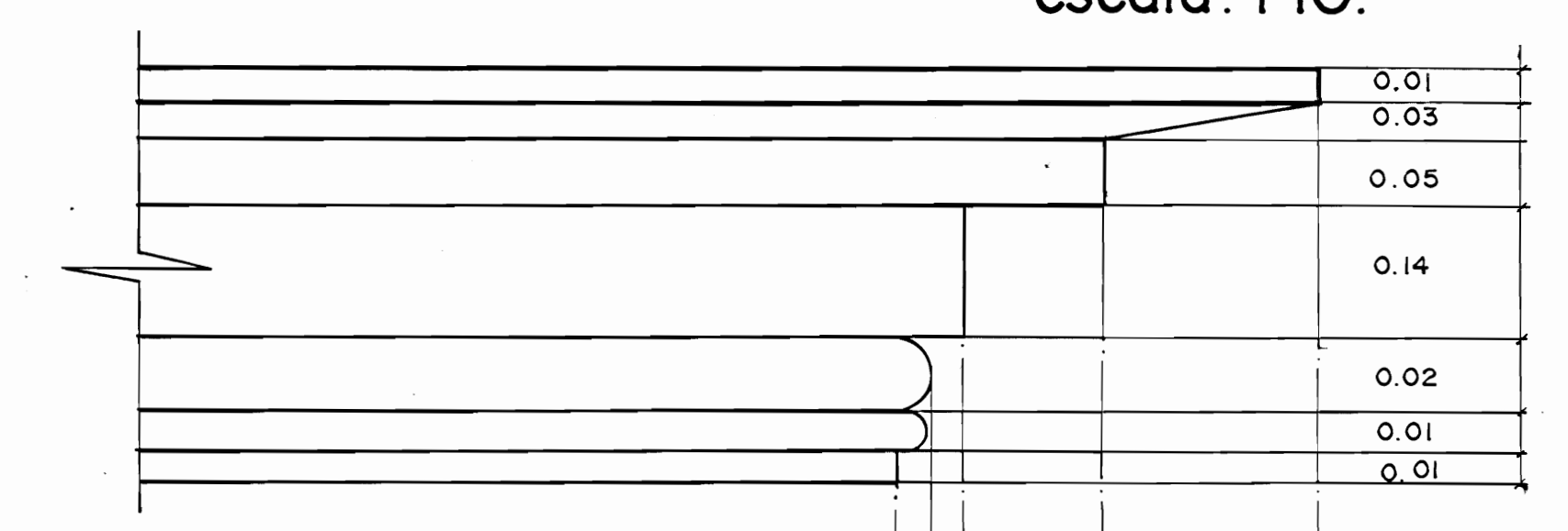
VERJA CENTRAL _ FACHADA POSTERIOR. escala: 1:10.
