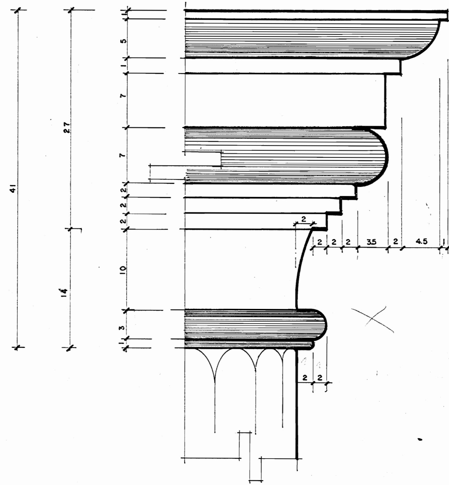
DETALLE COLUMNA ESC. 1:3
