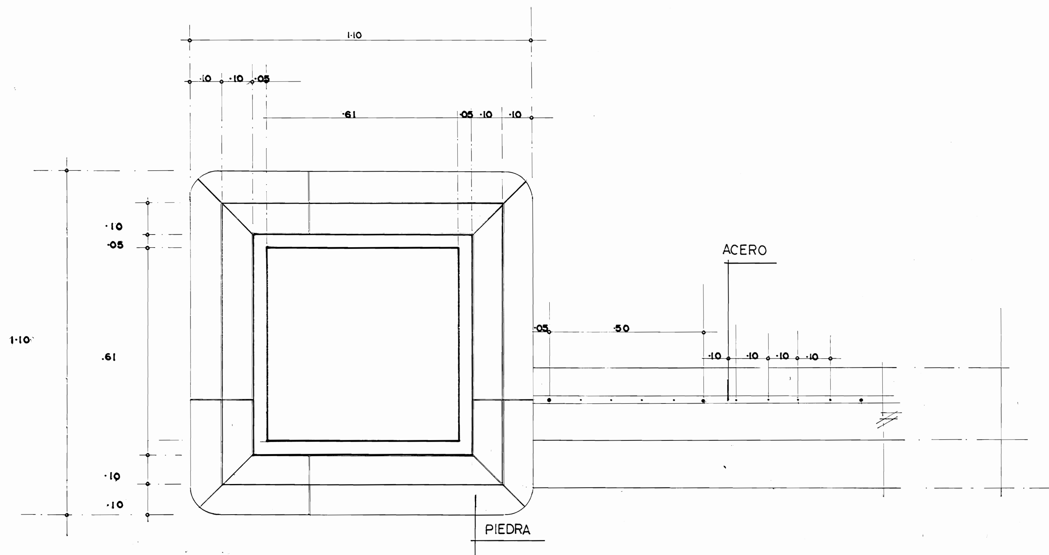
DETALLE DE COLUMNA EN EL MURO ①
