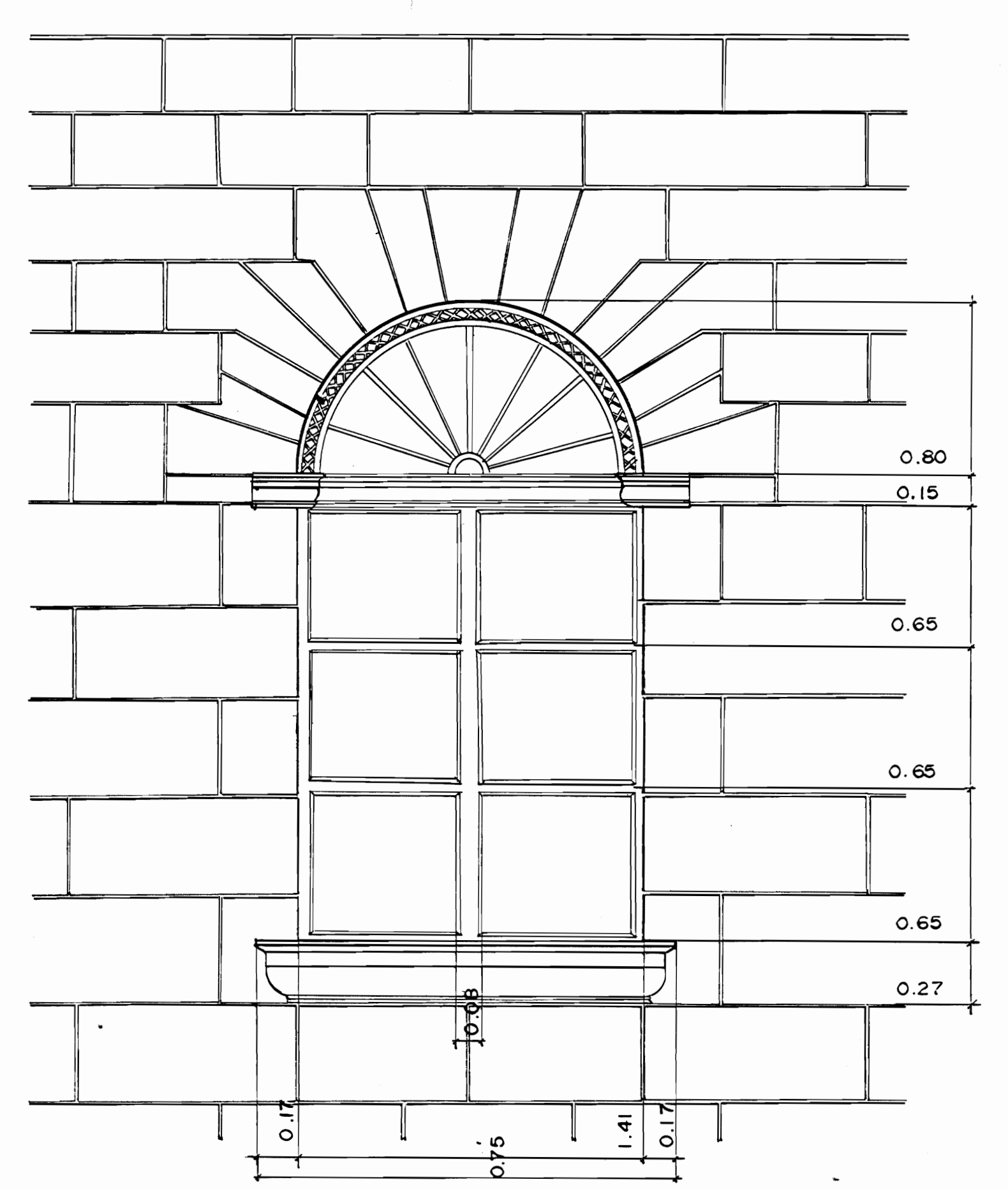
VENTANA LATERAL _ FACHADA POST. escala: 1:20.
