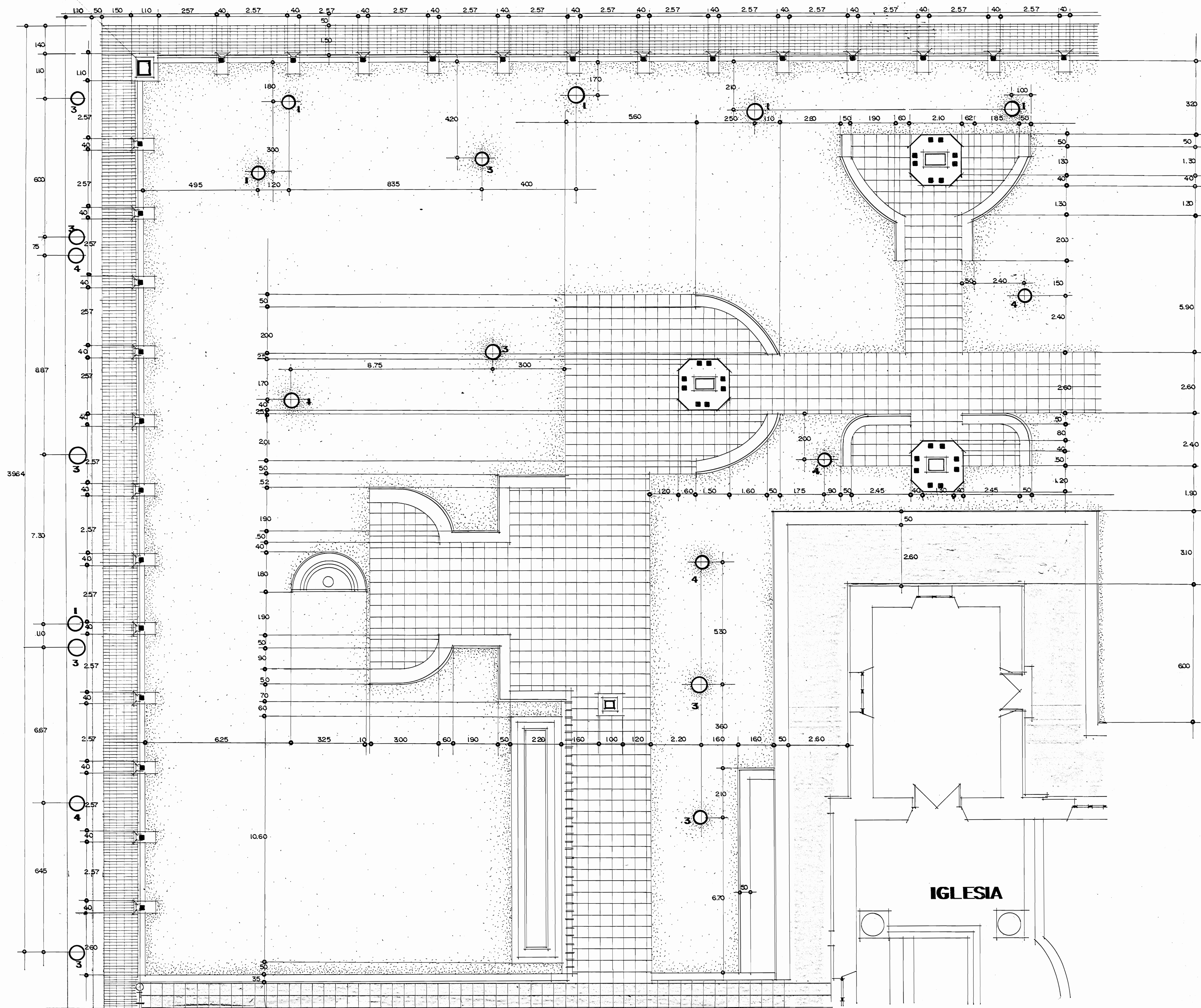
PLANTA SECTOR SURESTE
