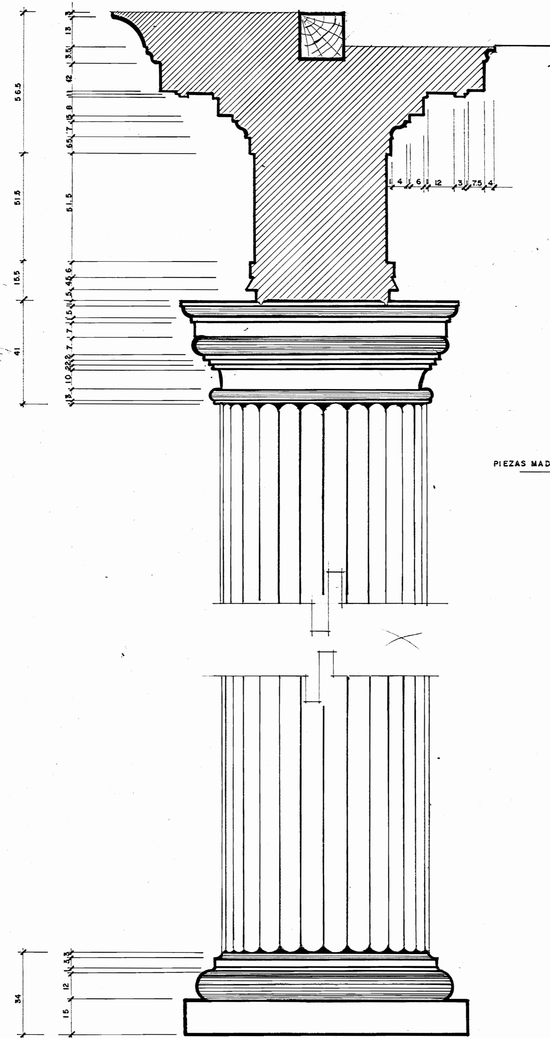
DETALLE DE COLUMNA ESC. 1:3
