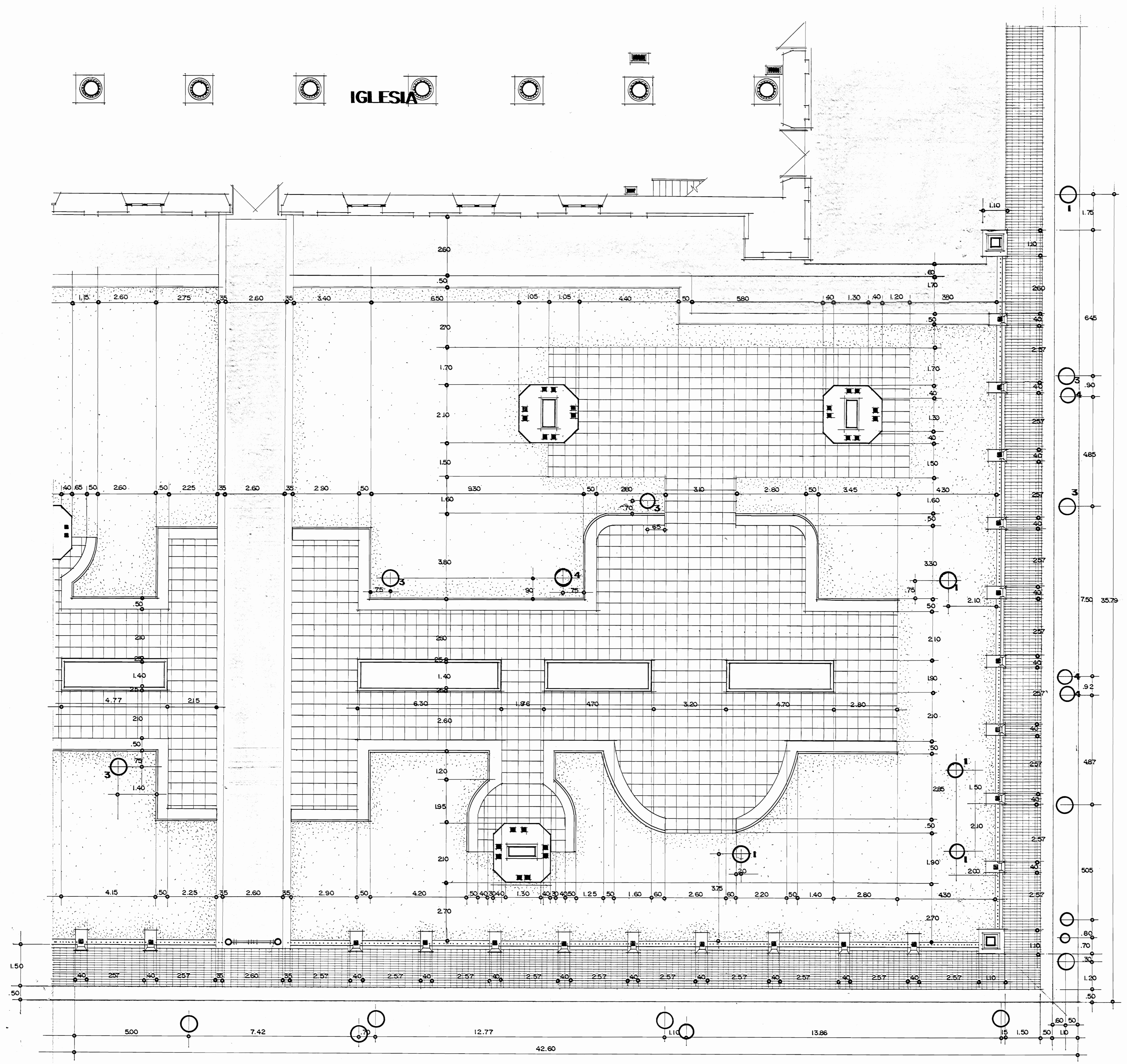
PLANTA SECTOR NOROESTE
