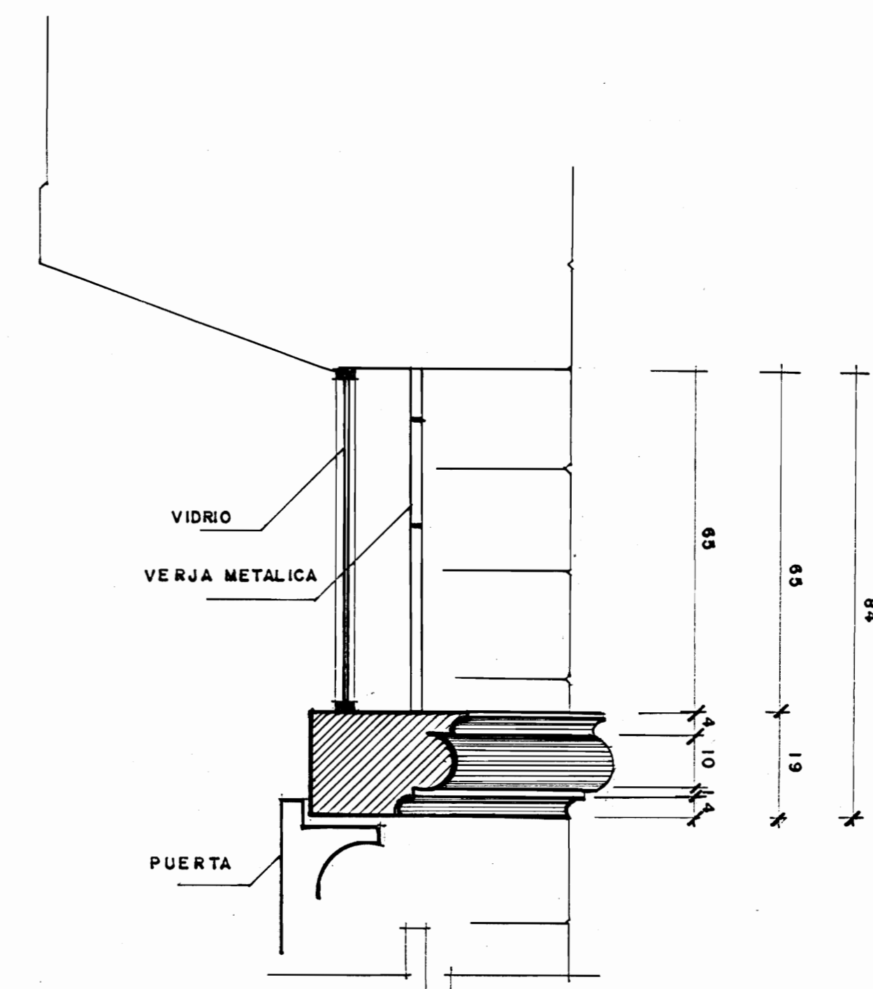
DETALLE 7 ESC. 1:10
