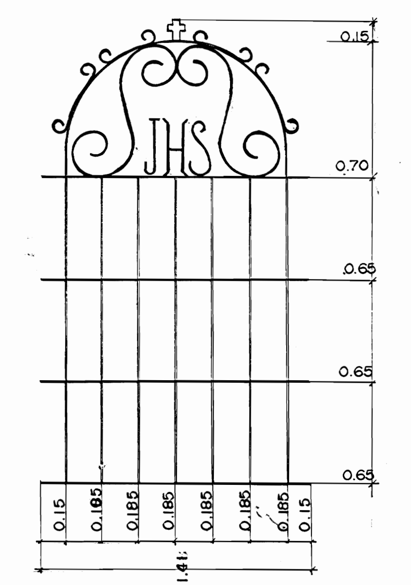
VERJA LATERAL _ FACHADA POST. escala: 1:20.
