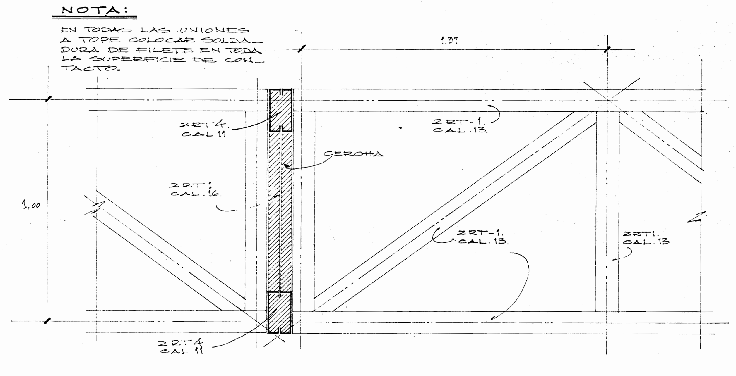
DET. DE VIGA AMERICANA ESC. = 1/10.
