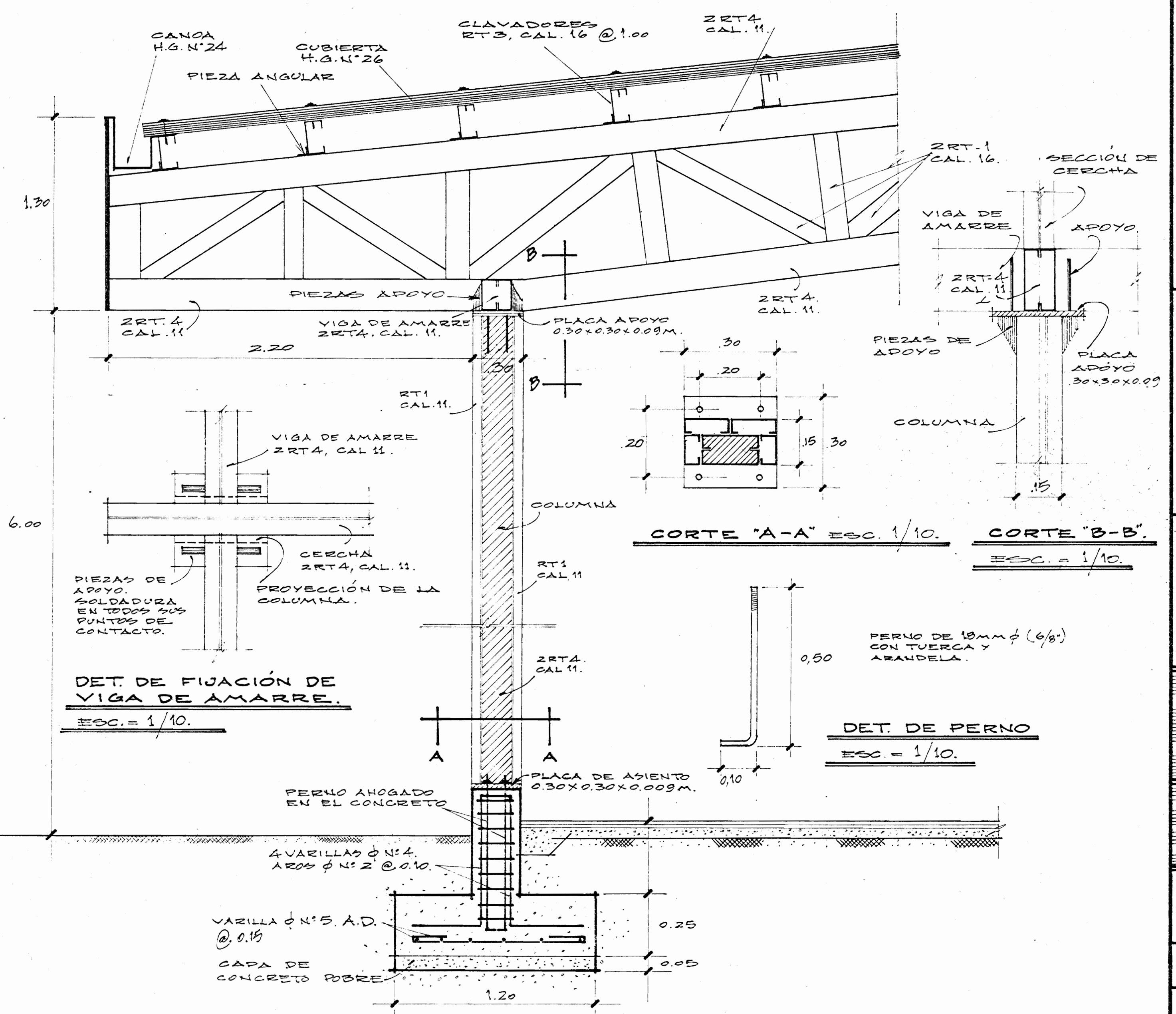
CORTE TÍPICO ESC. = 1/20.
