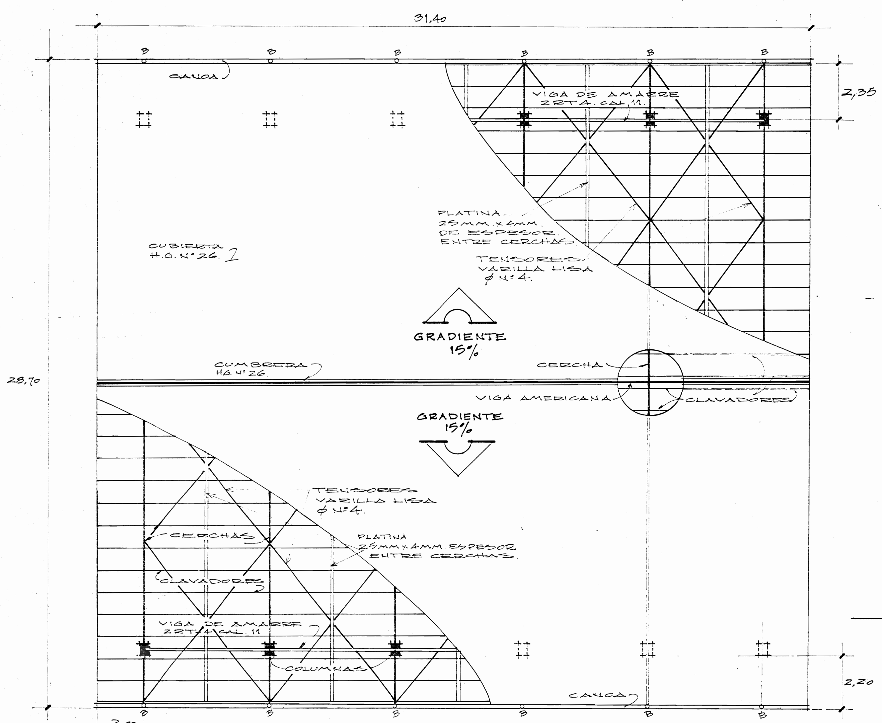
PLANTA DE TECHO ESC. = 1/100.
