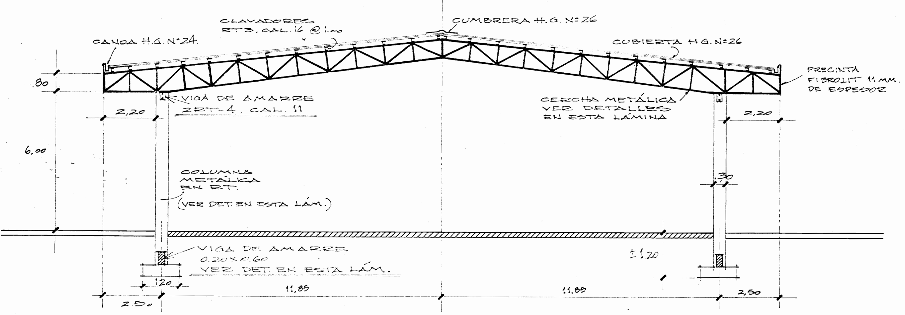
CORTE TRANSVERSAL ESC. = 1/100.
