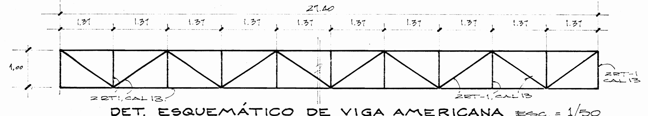
DET. ESQUEMÁTICO DE VIGA AMERICANA ESC. = 1/50.
