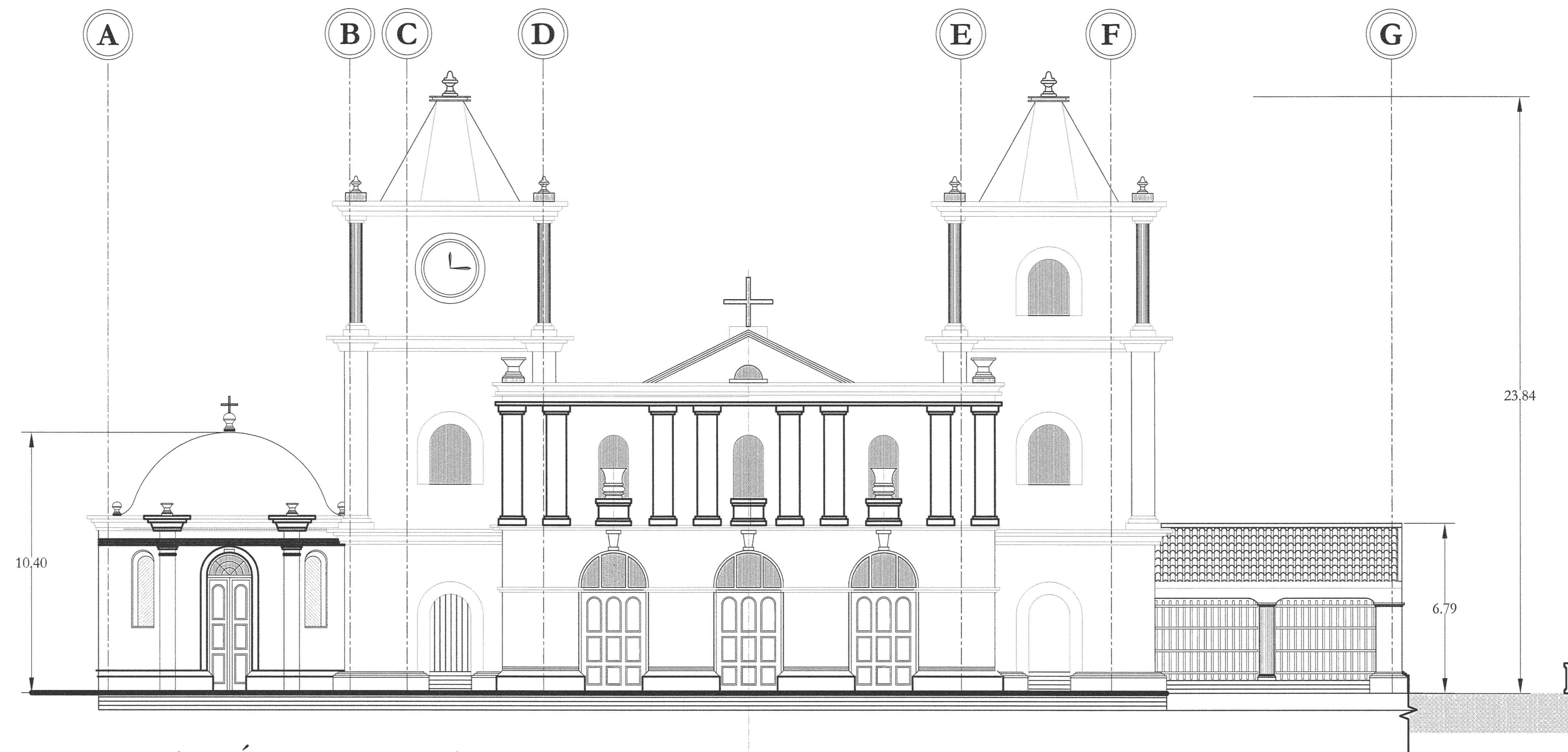
ELEVACIÓN PRINCIPAL esc. 1:100
