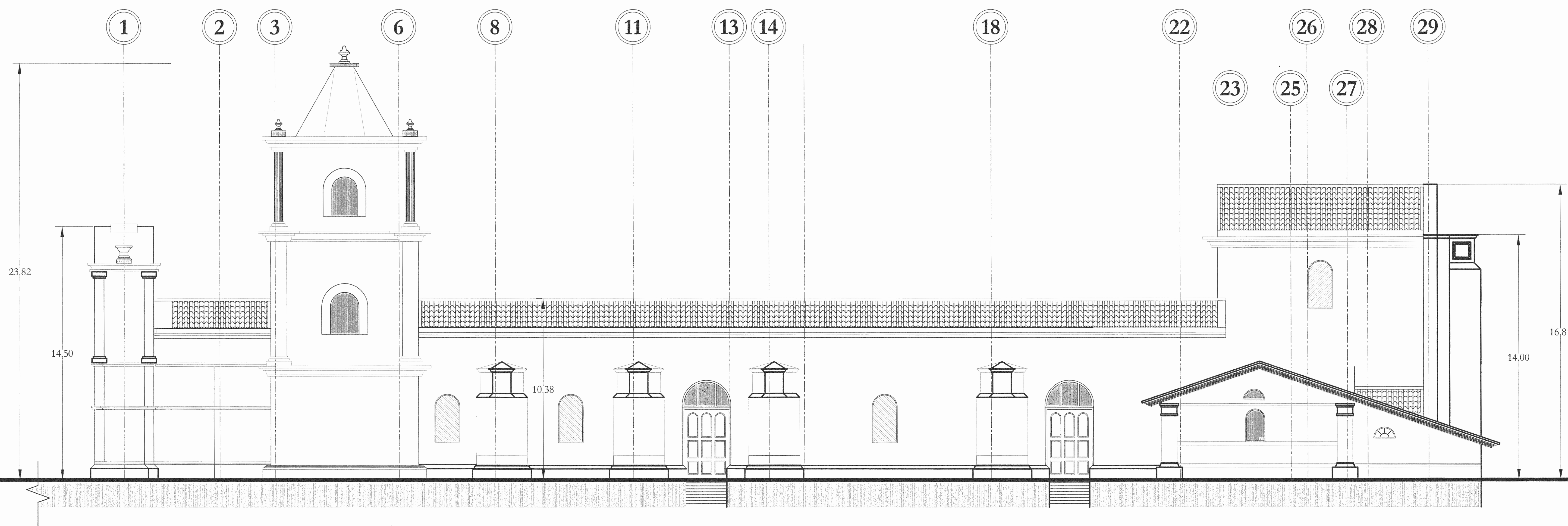
ELEVACIÓN NORTE esc. 1:100
