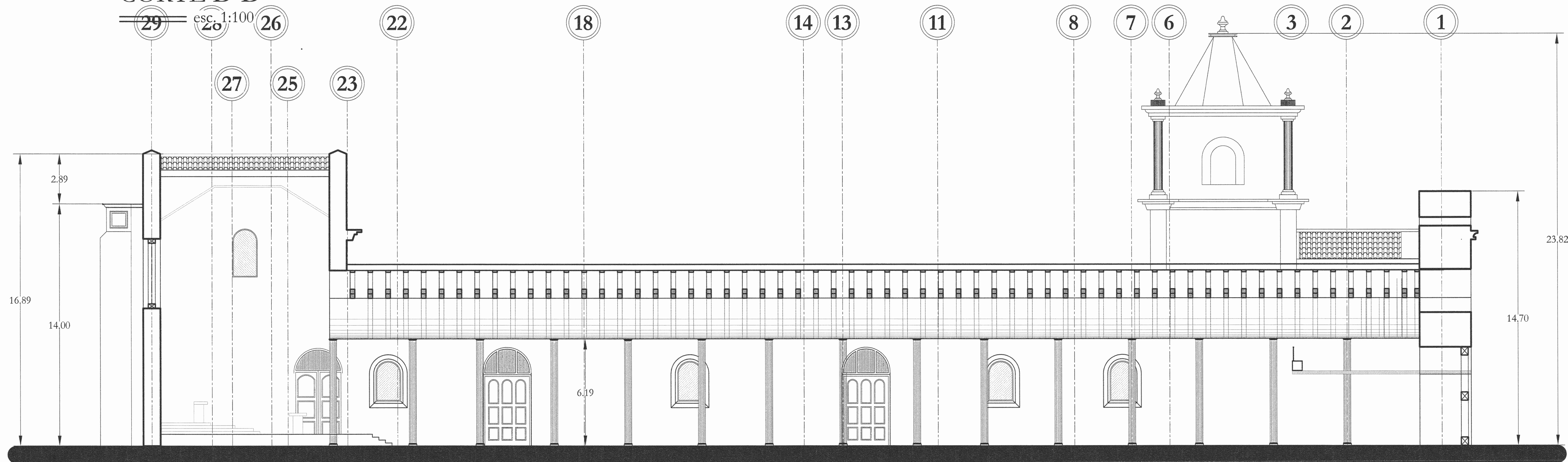
CORTE E-E
