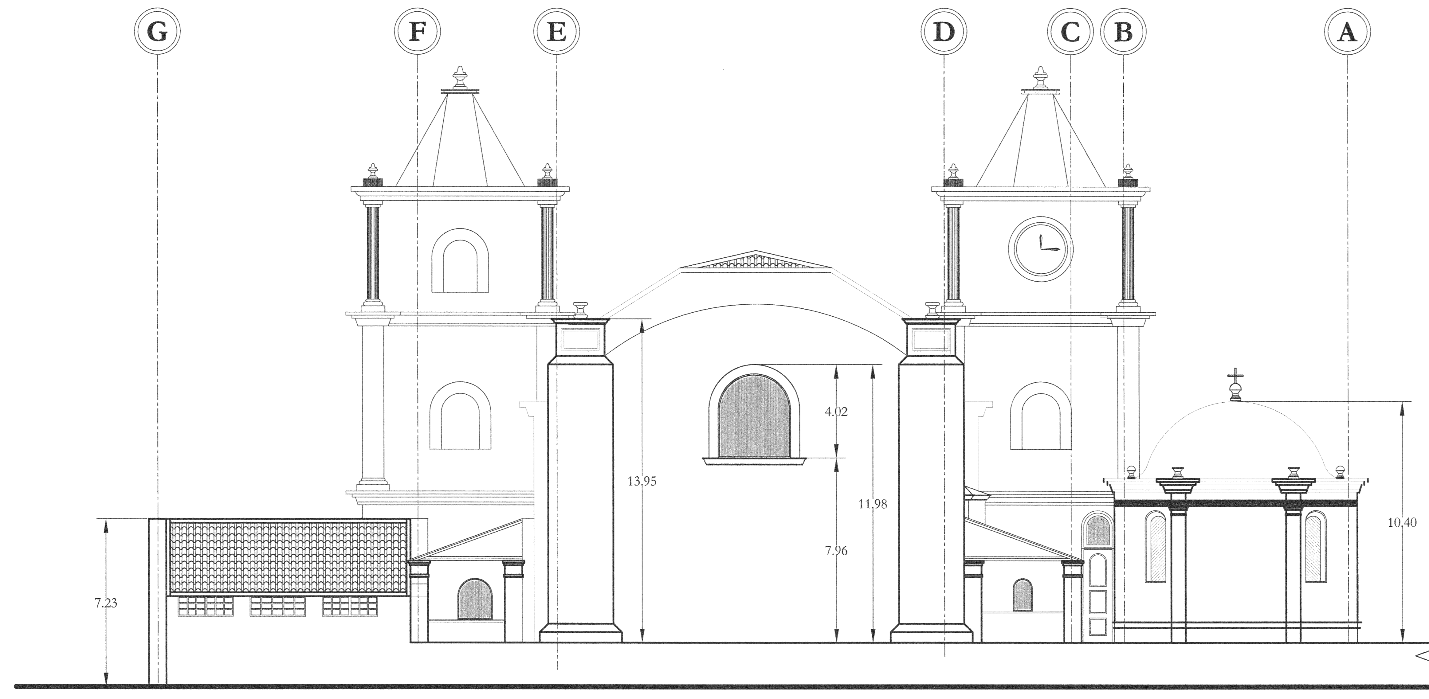
ELEVACIÓN POSTERIOR esc. 1:100
