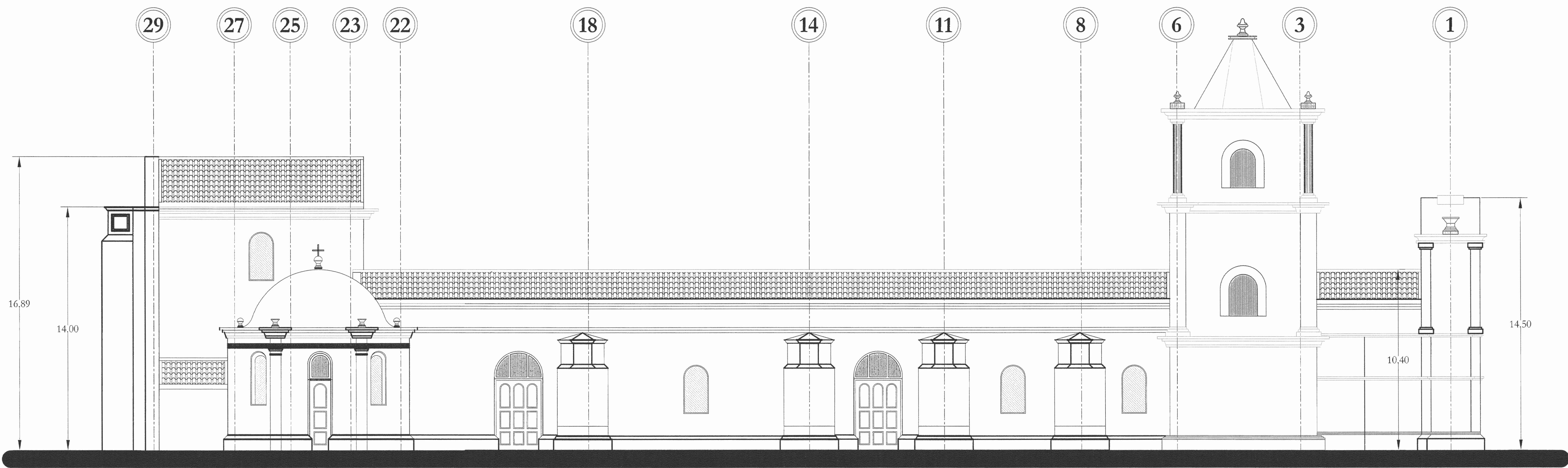
ELEVACIÓN SUR esc. 1:100
