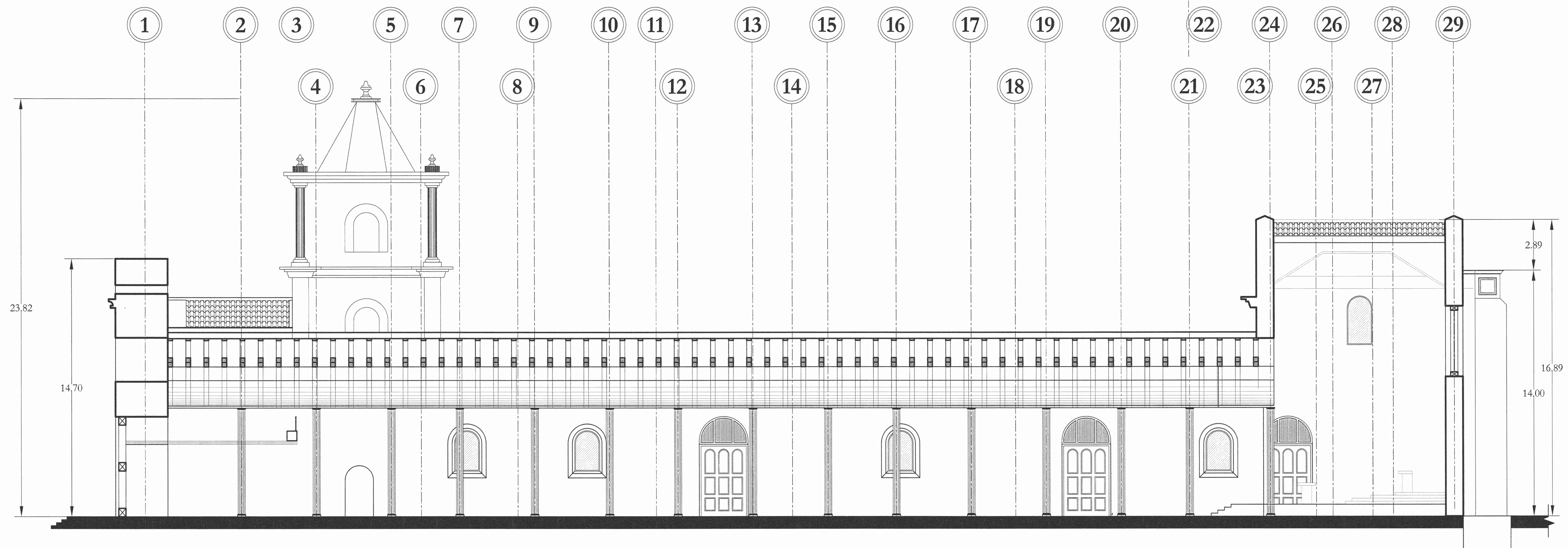
CORTE D-D
