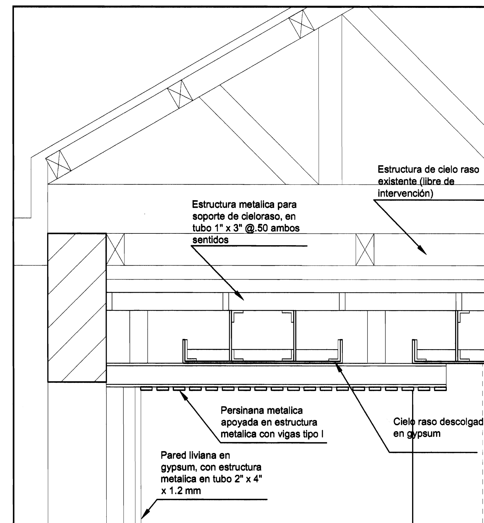
DETALLE 3 ESCALA 1/20
