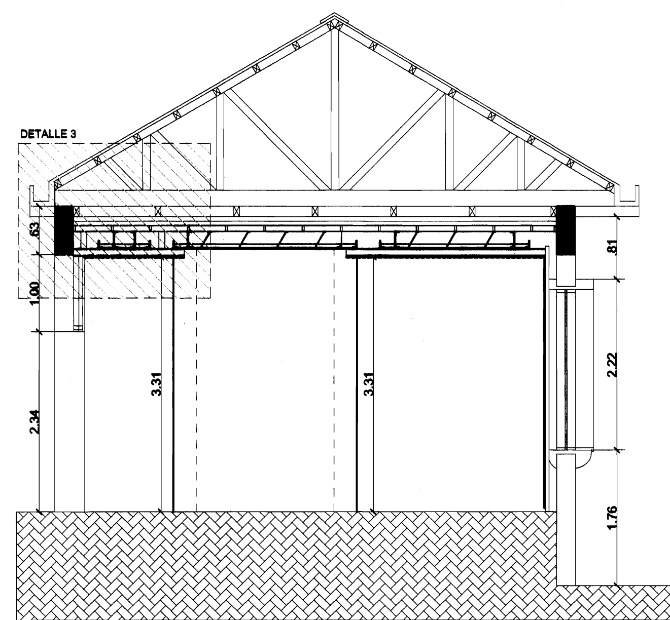
CORTE TRANSVERSAL C-C' ESCALA 1/50
