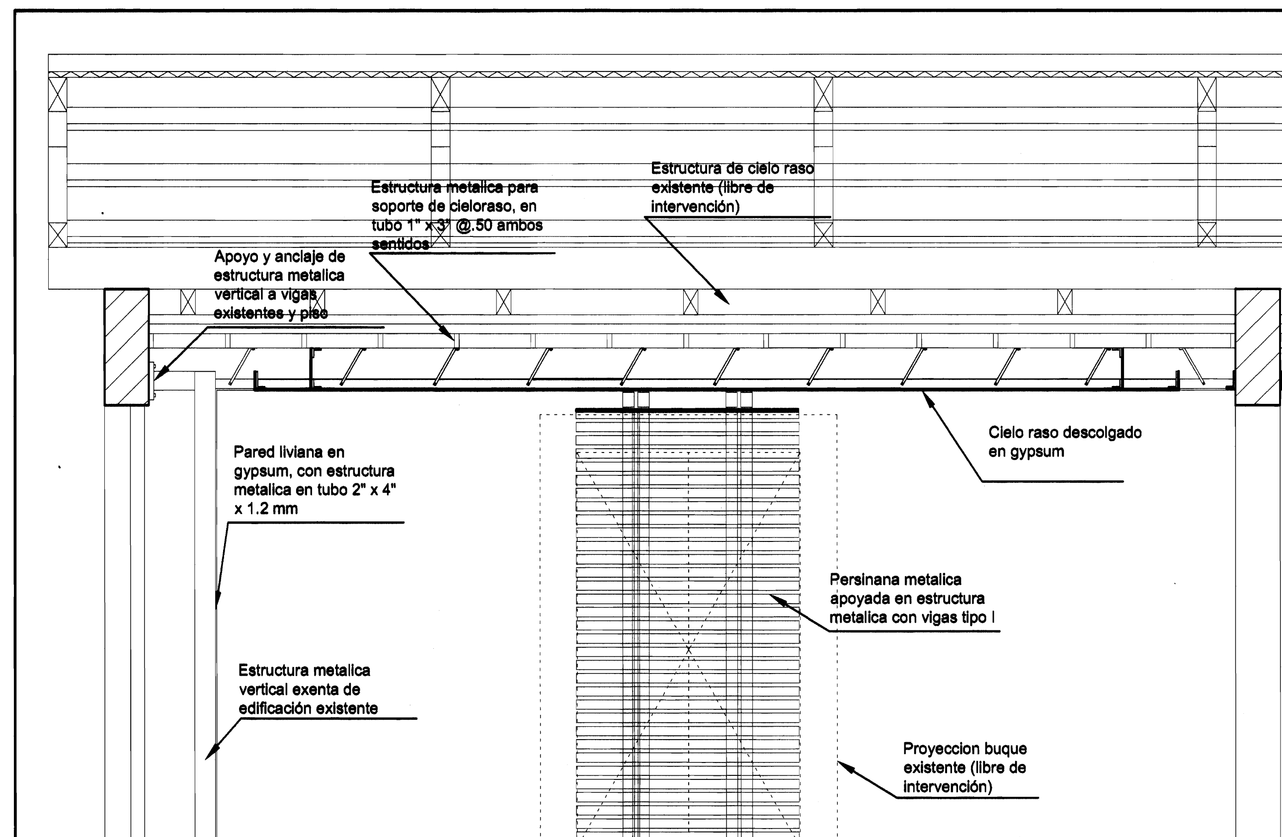
DETALLE 2 ESCALA 1/20
