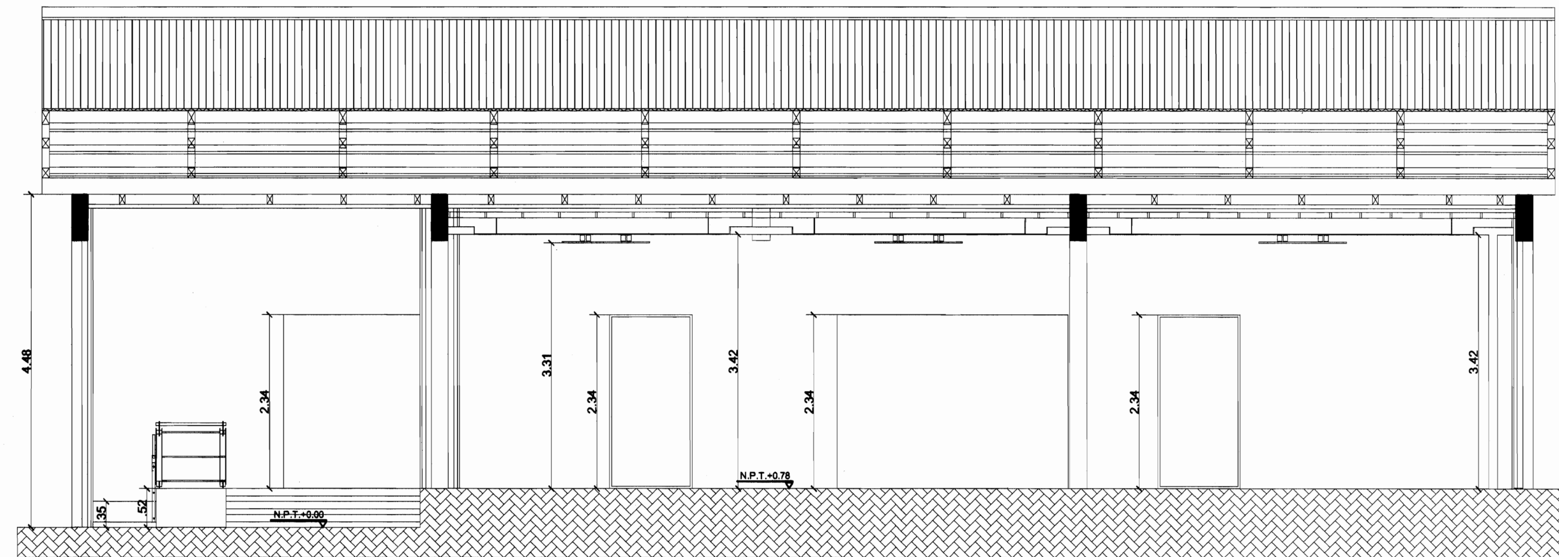
CORTE LONGITUDINAL A-A' ESCALA 1/50
