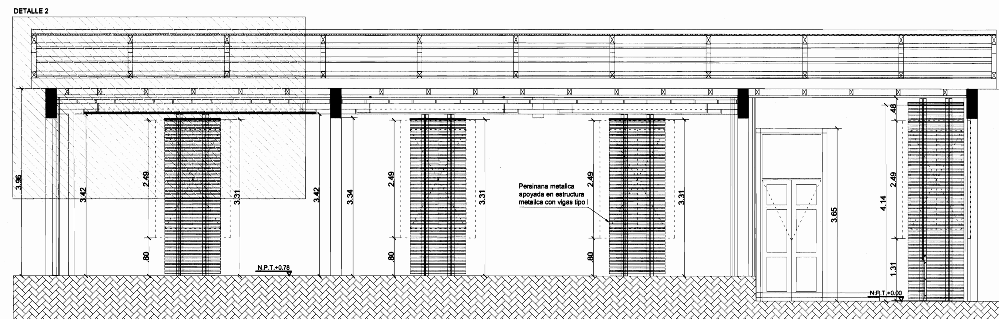
CORTE LONGITUDINAL B-B' ESCALA 1/50
