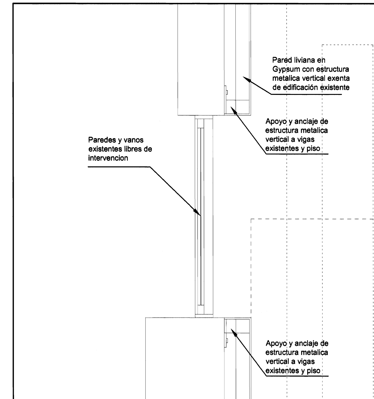
DETALLE 1 ESCALA 1/20
