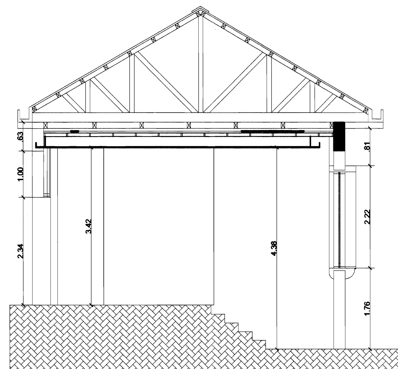
CORTE TRANSVERSAL D-D' ESCALA 1/50
