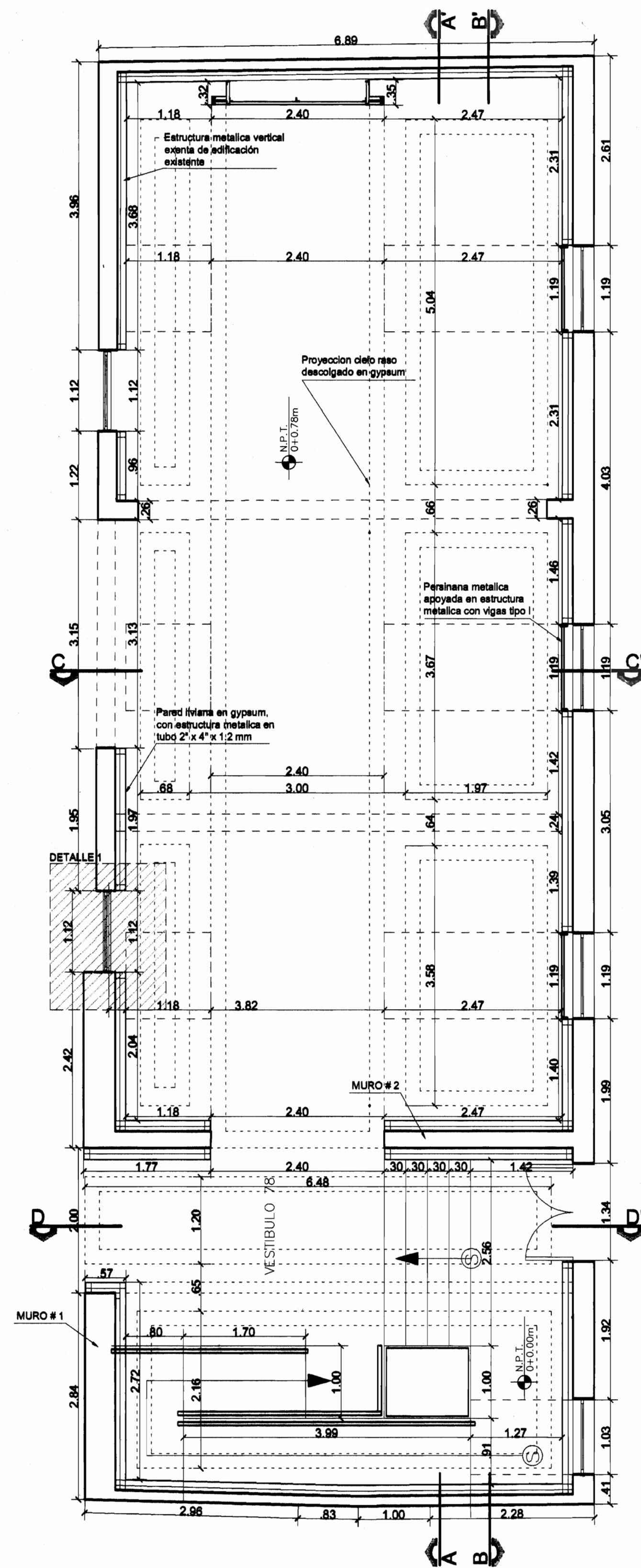
PLANTA DE DISTRIBUCION BINGO MIL COLORES (PATRIMONIO NACIONAL) ESCALA 1/50
