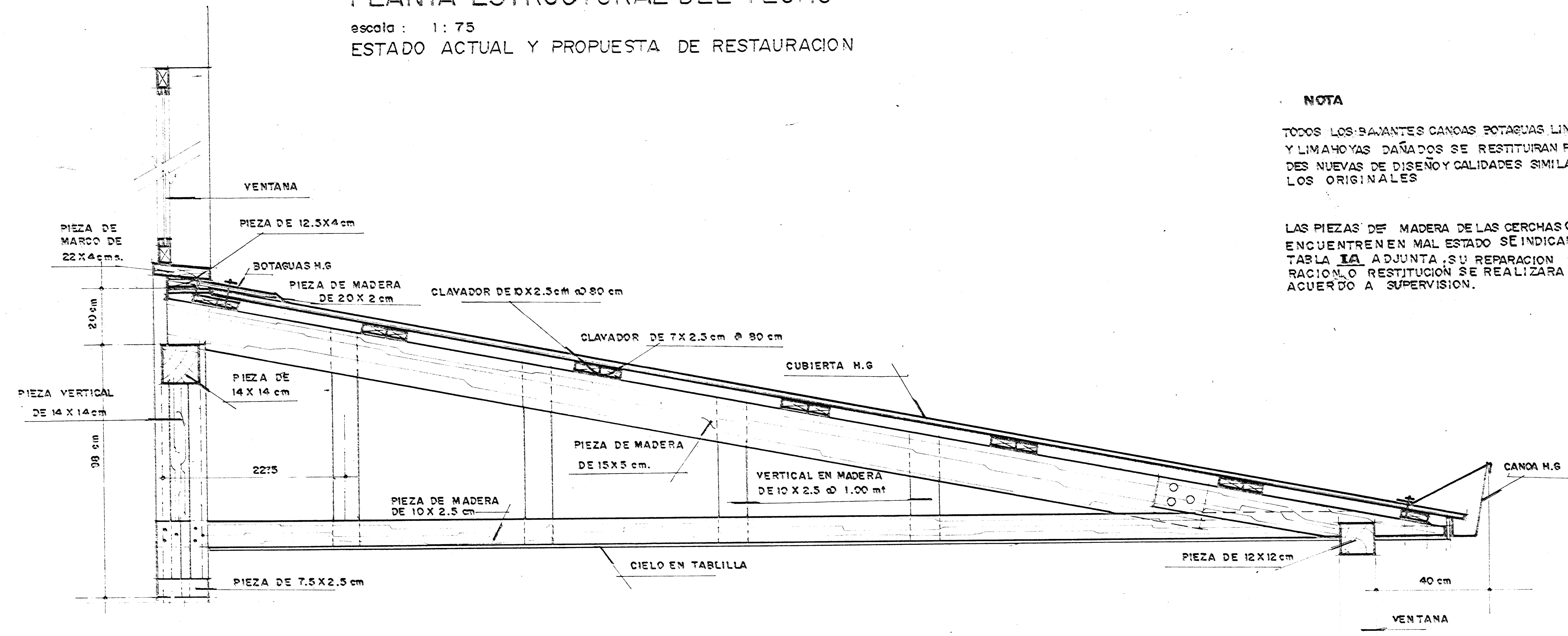
CORTE POR I-I escala : 1 : 10
