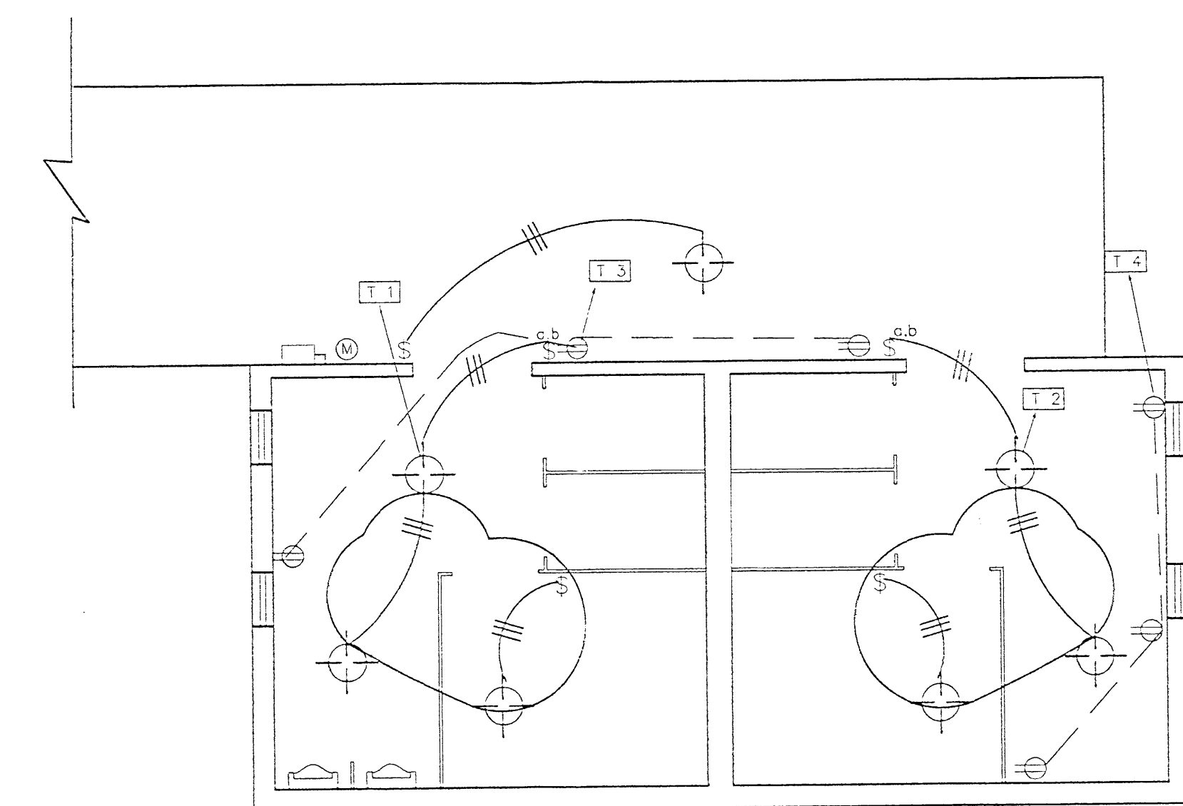
PLANTA ELECTRICA ESC. 1 : 50
