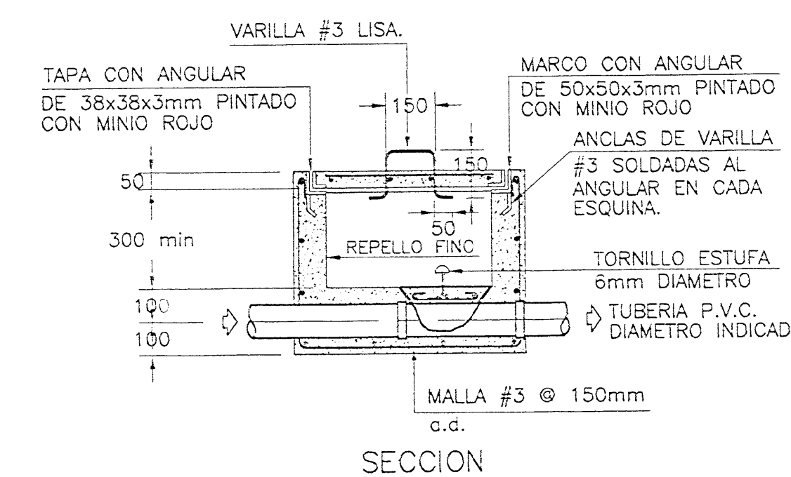
DETALLE DE CAJA DE REGISTRO PARA AGUAS NEGRAS ESC. 1 : 20
