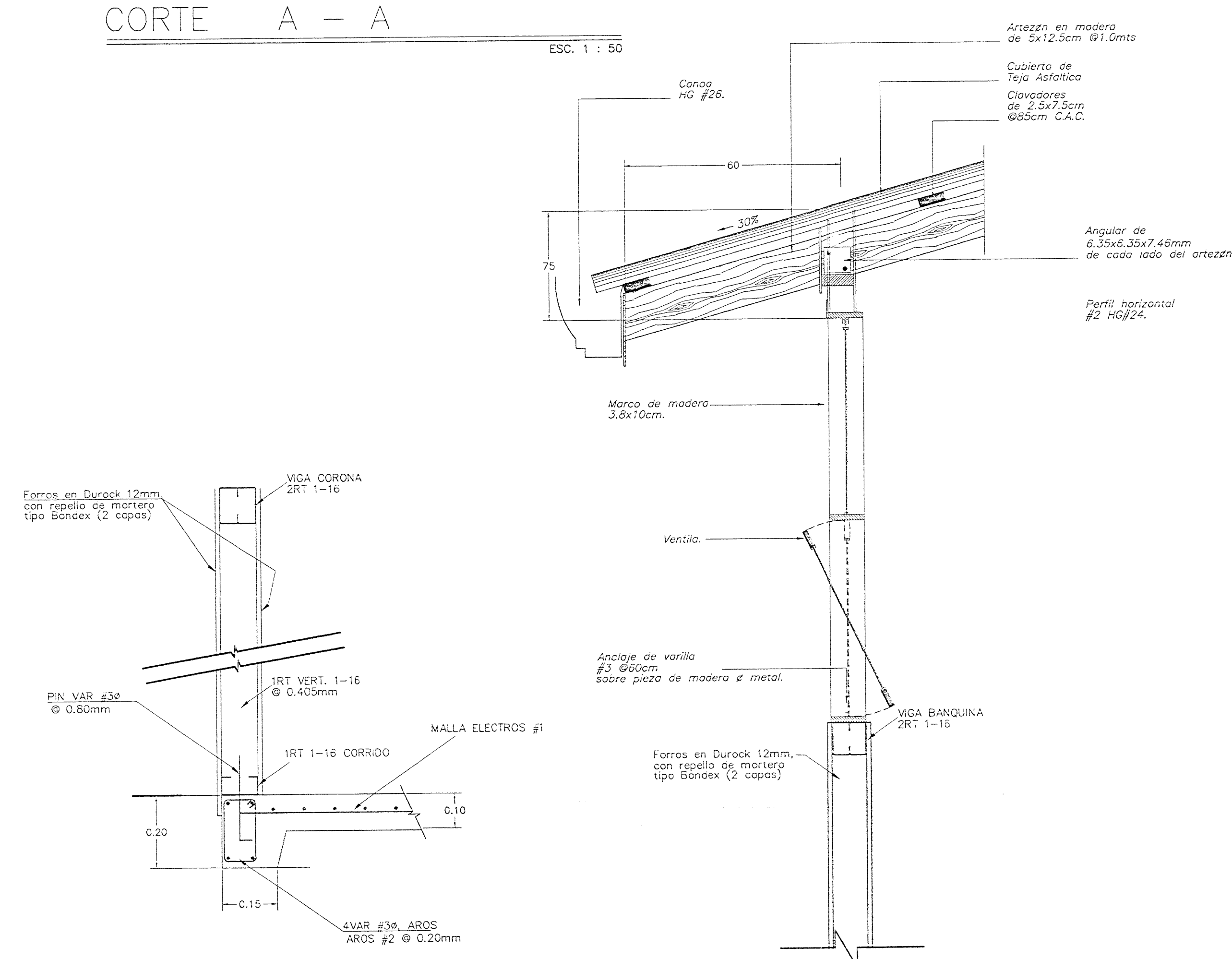
DETALLE DE PARED TIPICO ESC. 1:20
