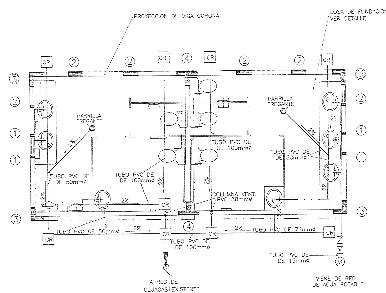
PLANTA DE CIMENTOS ESC. 1 : 50
