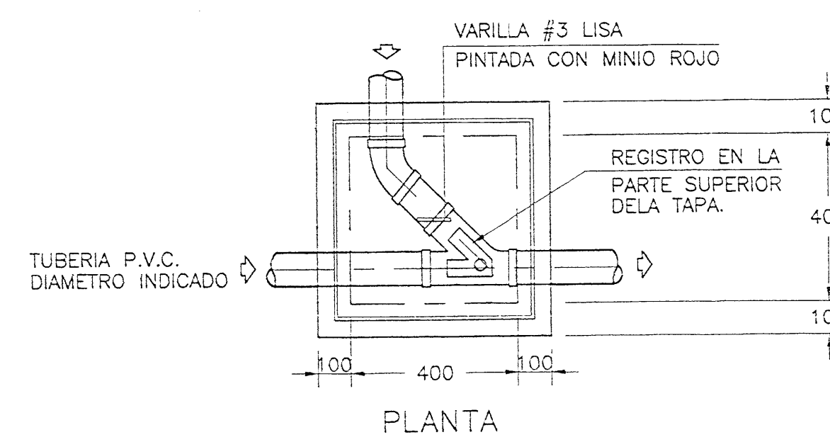
PLANTA
