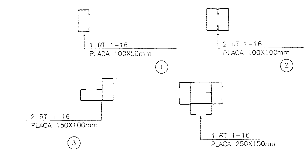
DETALLE DE MOCHETAS ESC. 1 : 20
