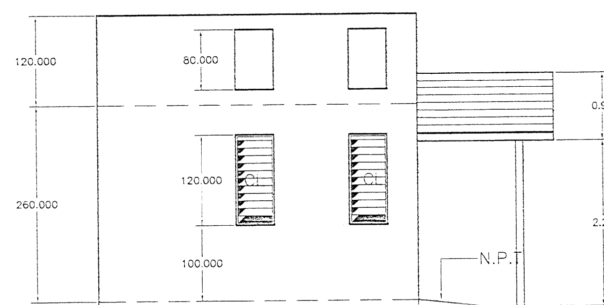
ELEVACION LATERAL DERACHA ESC. 1 : 50
