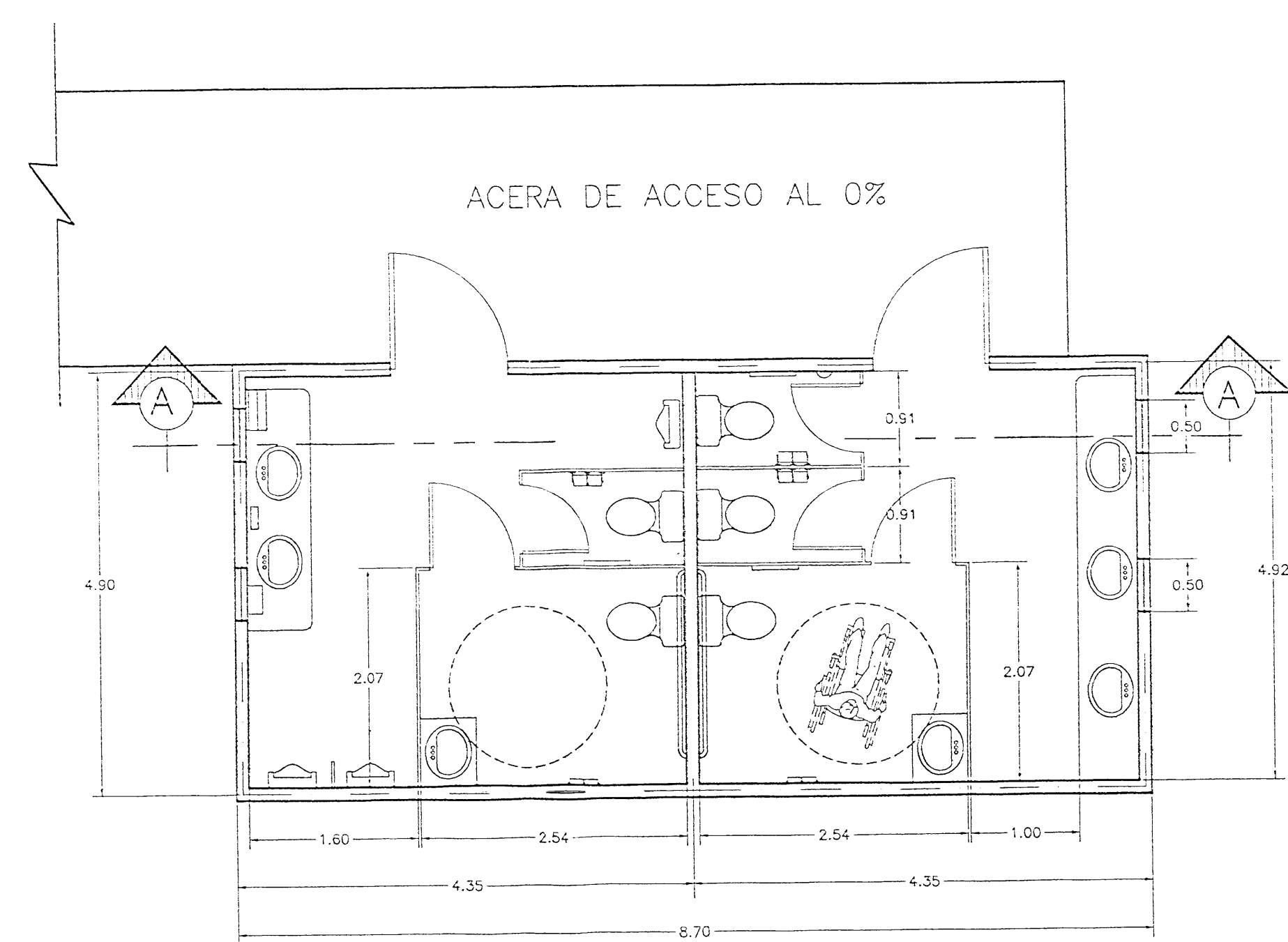
PLANTA DE DISTRIBUCION ESC. 1 : 50
