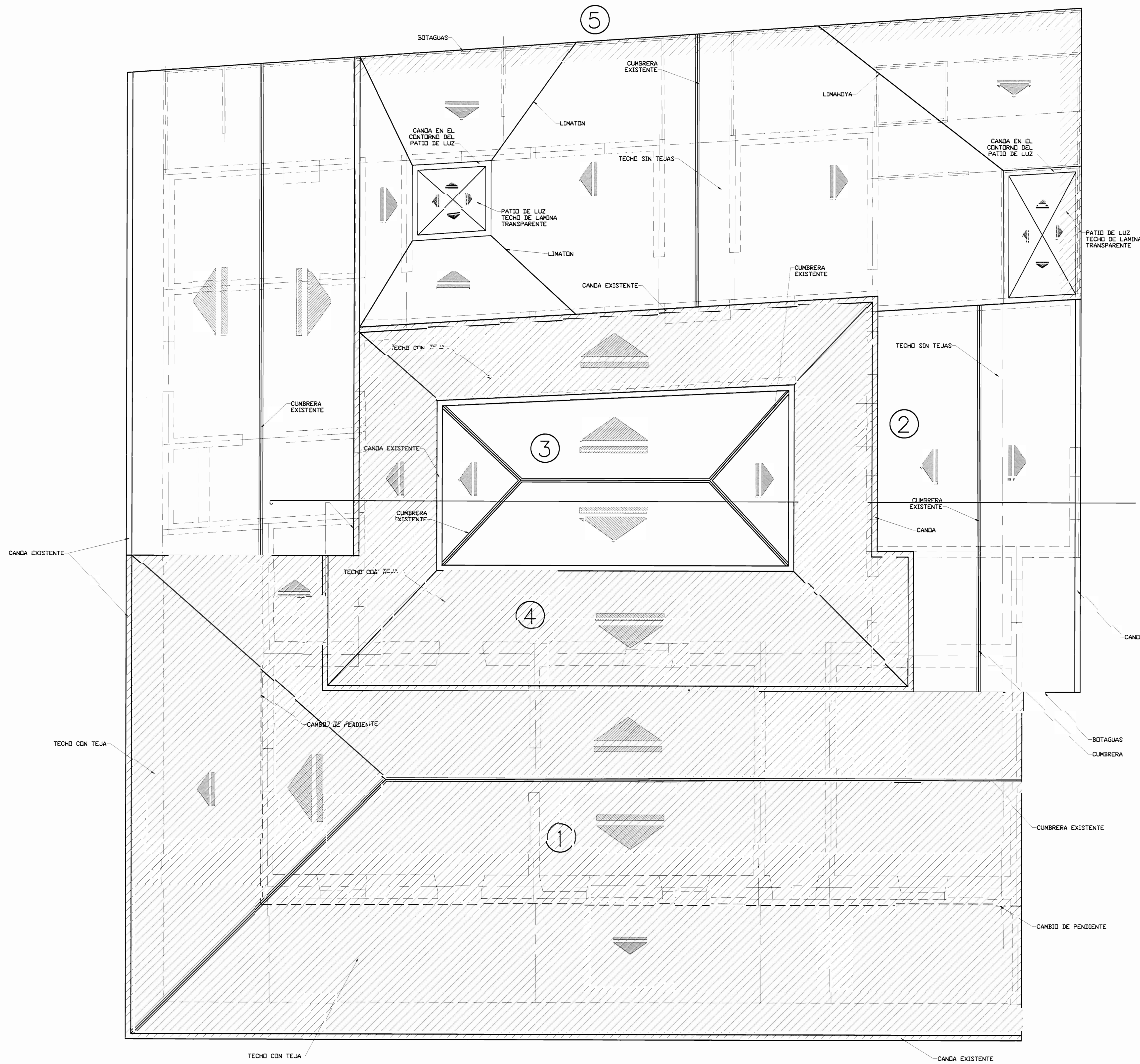
PLANTA DE TECHOS ESCALA 1:50
