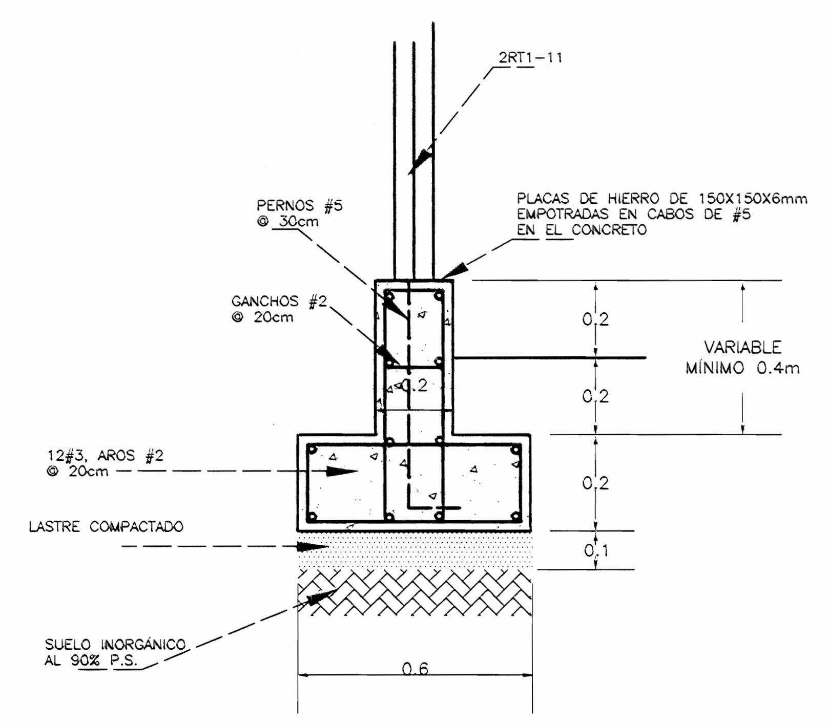
DETALLE PEDESTAL DE COLUMNA ESC. 1 : 10
