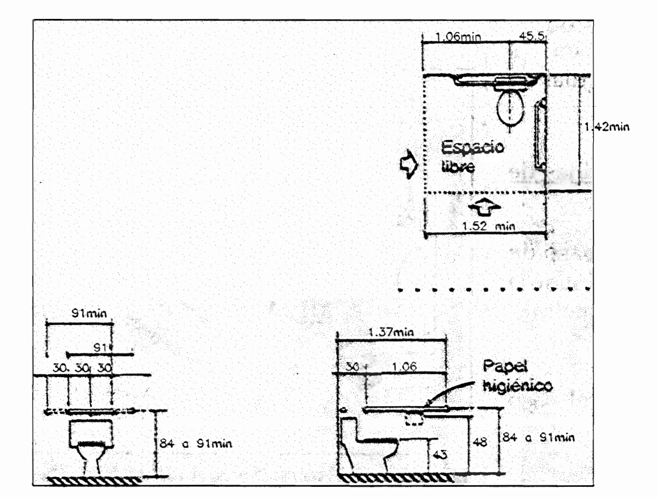
DETALLE BARRAS DE APOYO EN INODORO SIN ESC.
