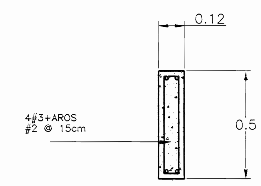
DETALLE TÍPICO DE COLUMNA ESC. 1 : 10
