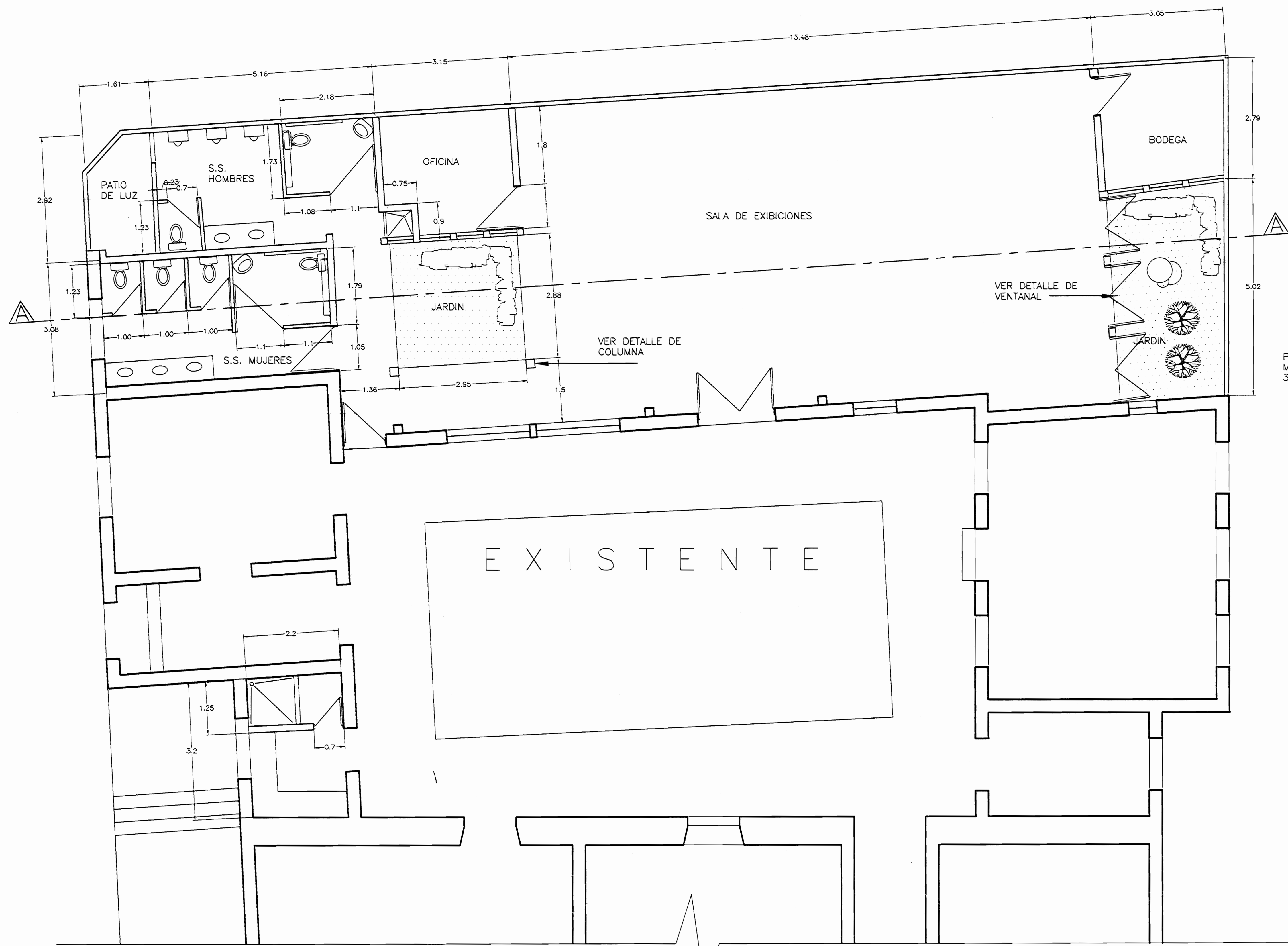
PLANTA DE DISTRIBUCIÓN ARQUITECTÓNICA PROPUESTA ESC. 1 : 50
