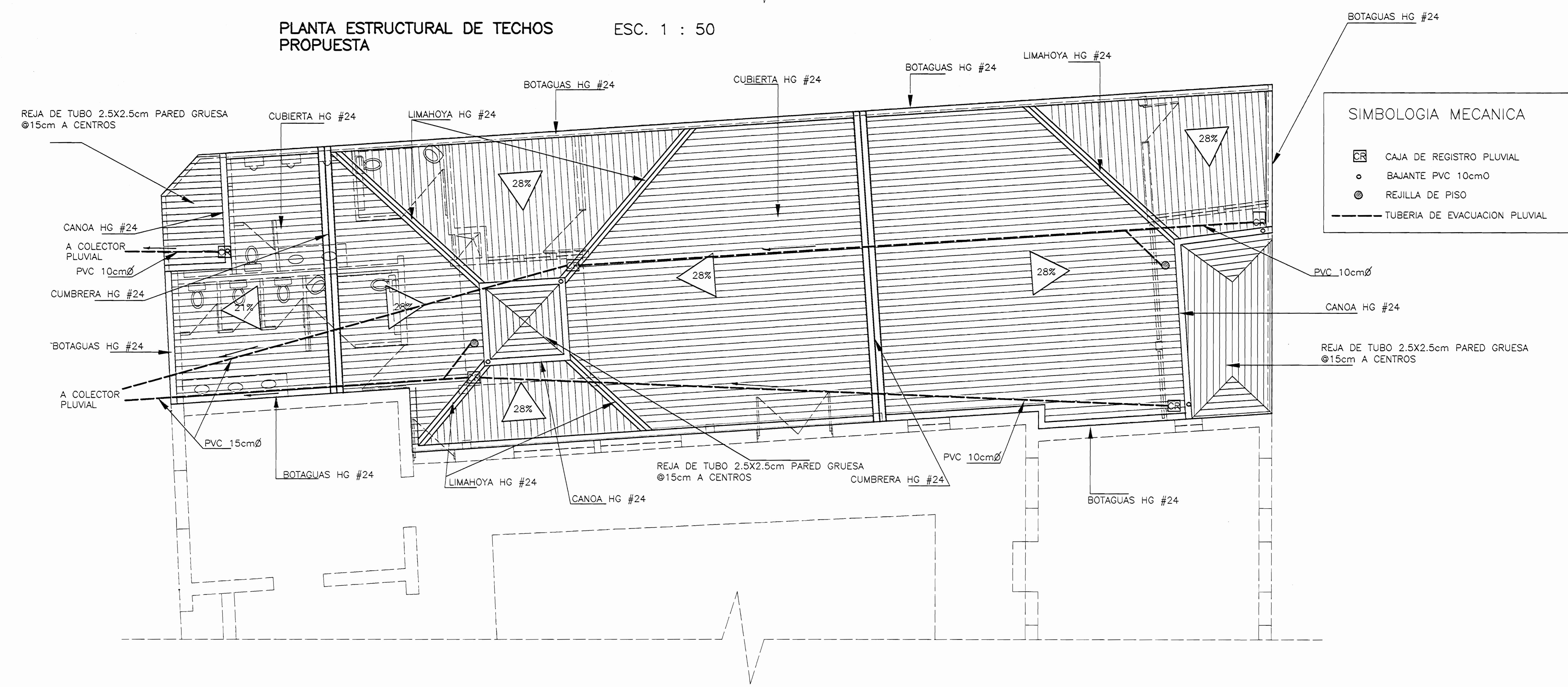
PLANTA DE CUBIERTAS Y EVACUACION PLUVIAL PROPUESTA ESC. 1 : 50
