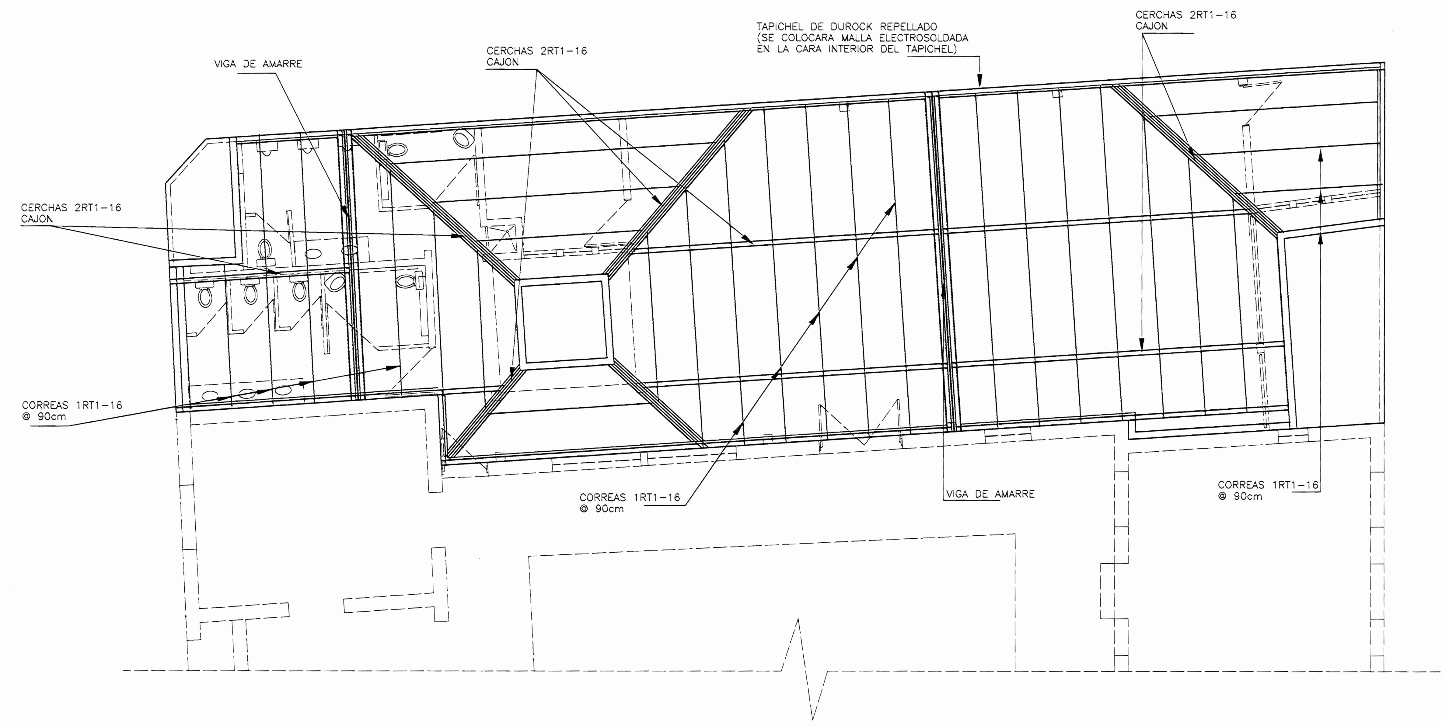
PLANTA ESTRUCTURAL DE TECHOS PROPUESTA ESC. 1 : 50
