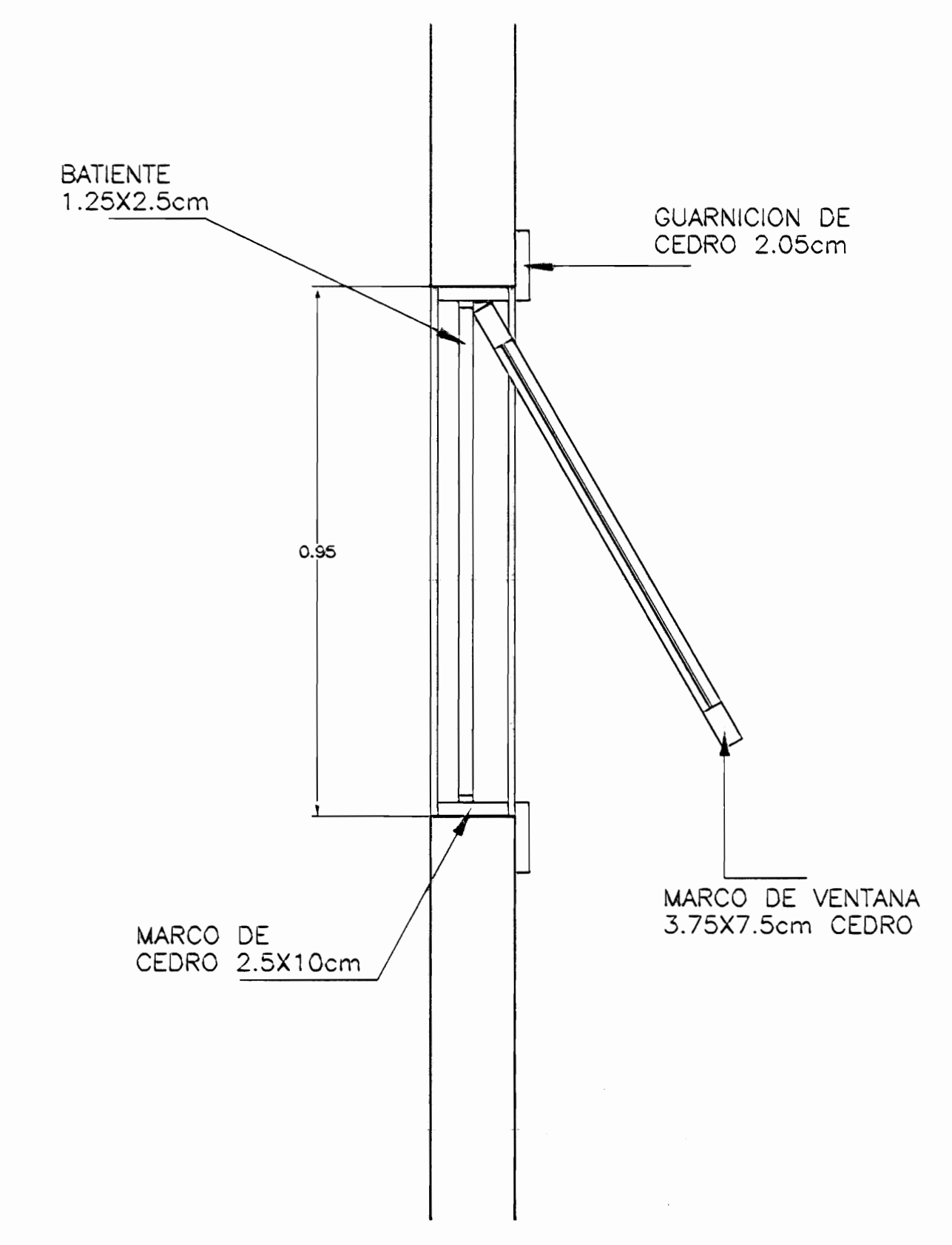
DETALLE DE VENTANA ESC. 1 : 10
