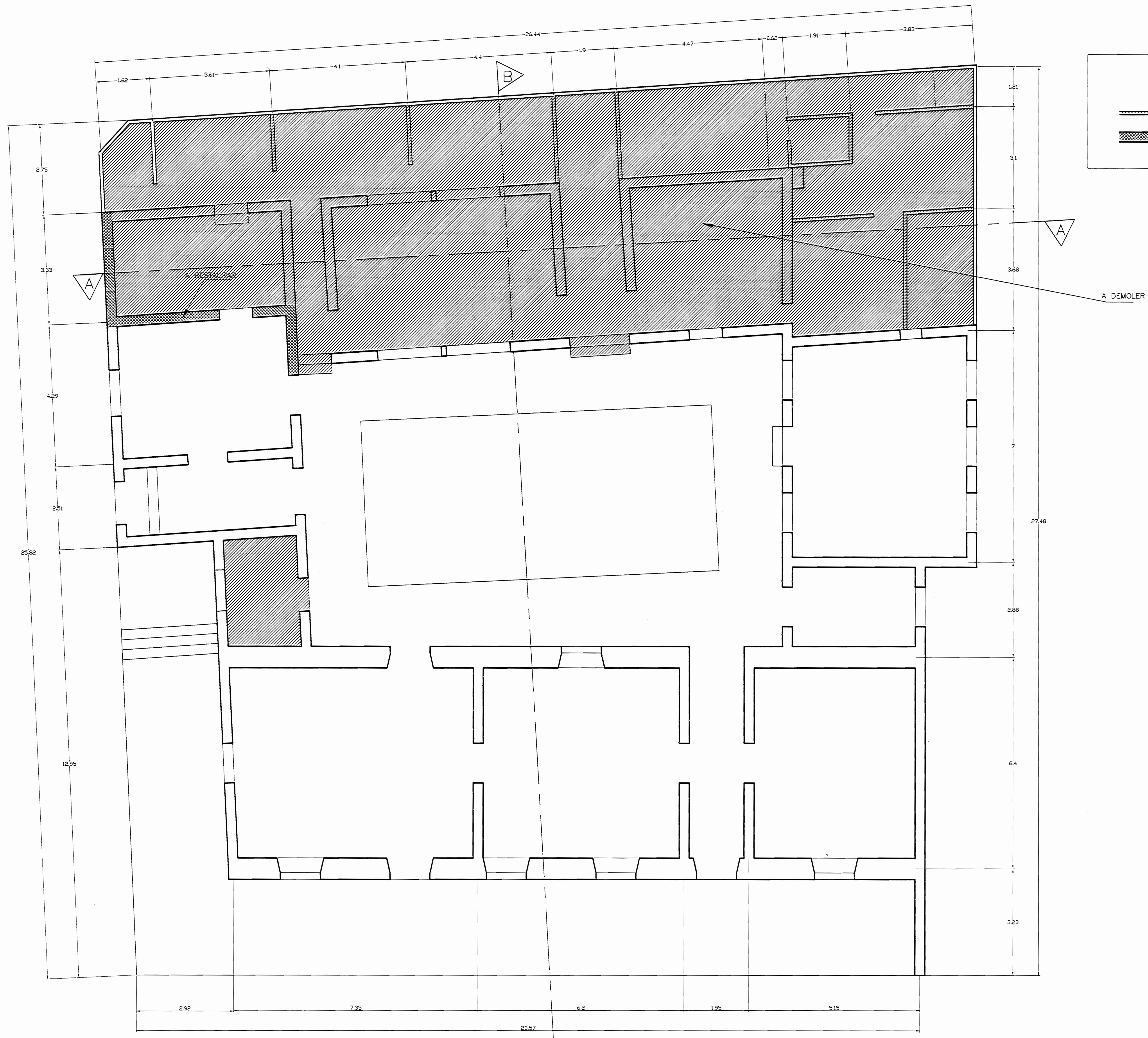
PLANTA DE DISTRIBUCIÓN ARQUITECTÓNICA ESTADO ACTUAL
