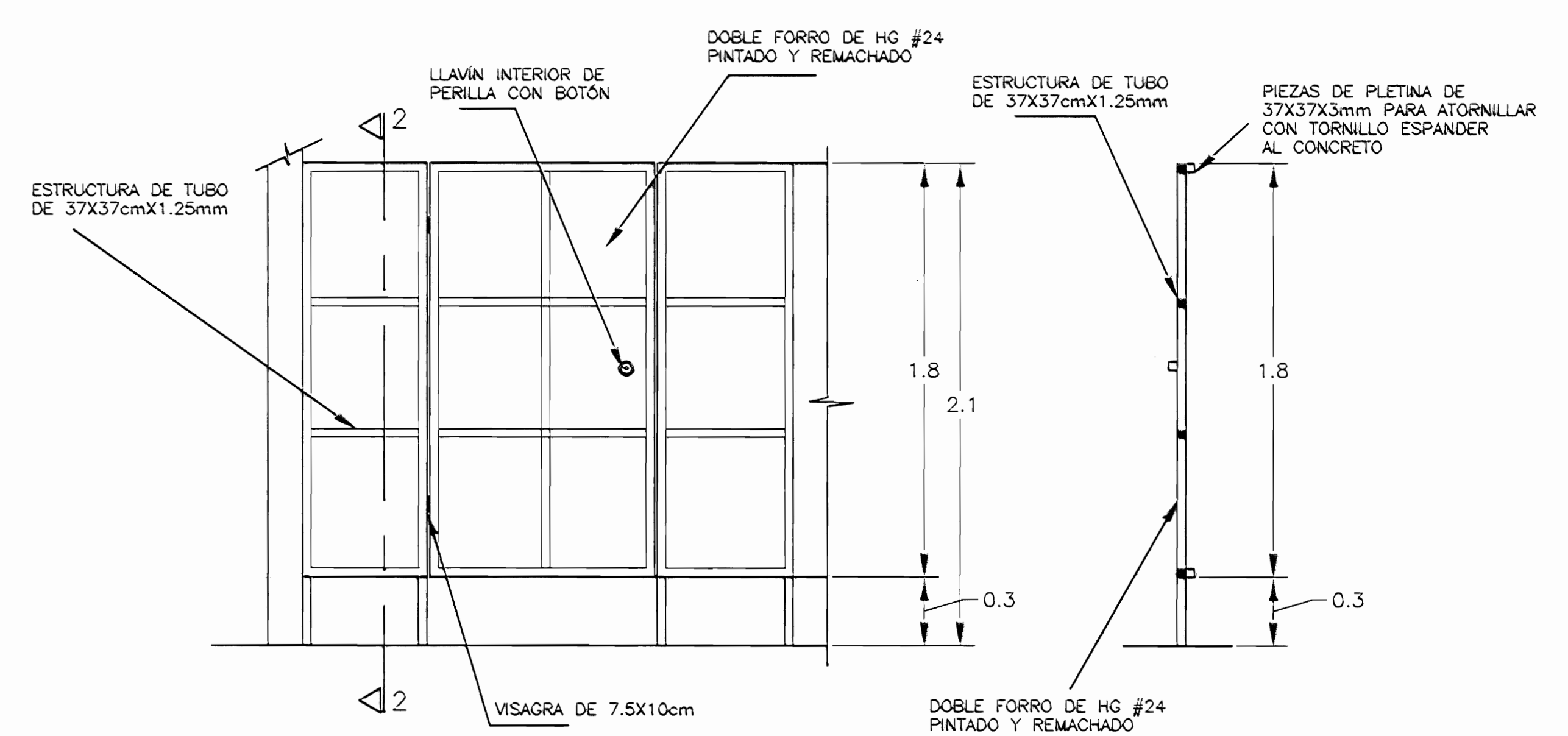
DETALLE TÍPICO DIVISION ENTRE SANITARIOS ESC. 1 : 20
