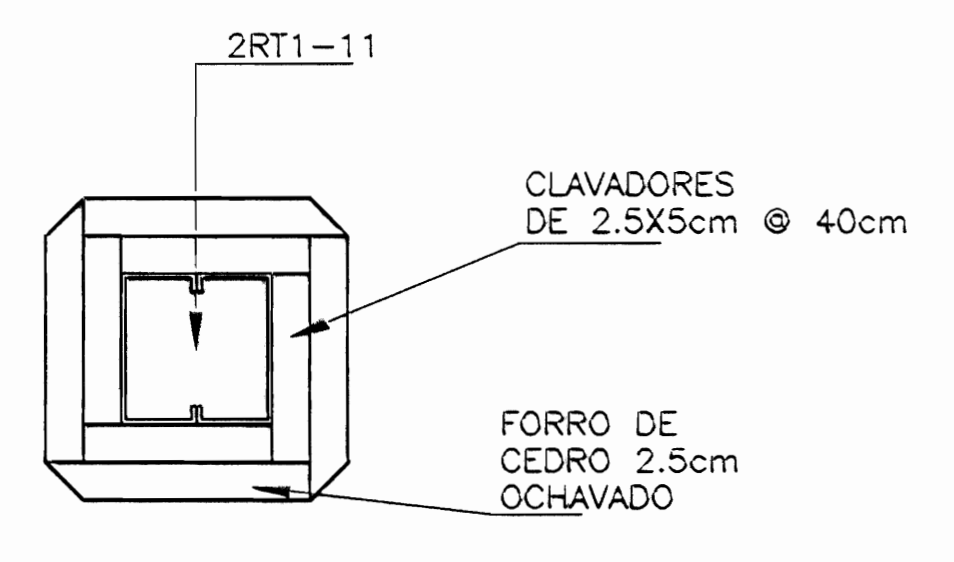
DETALLE DE COLUMNA SECCION 1 ESC. 1 : 20
