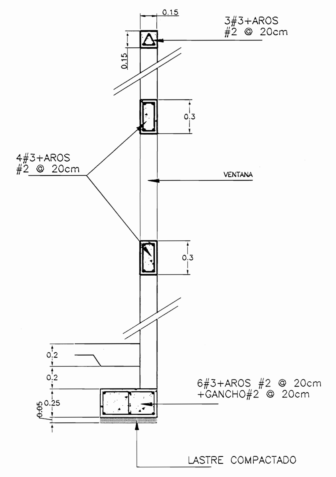
CORTE TÍPICO DE PARED ESC. 1 : 20
