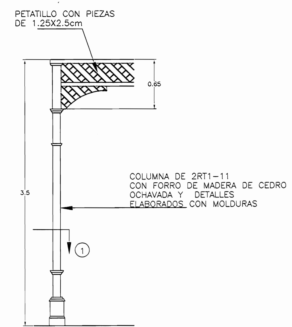
DETALLE DE COLUMNA ESC. 1 : 25
