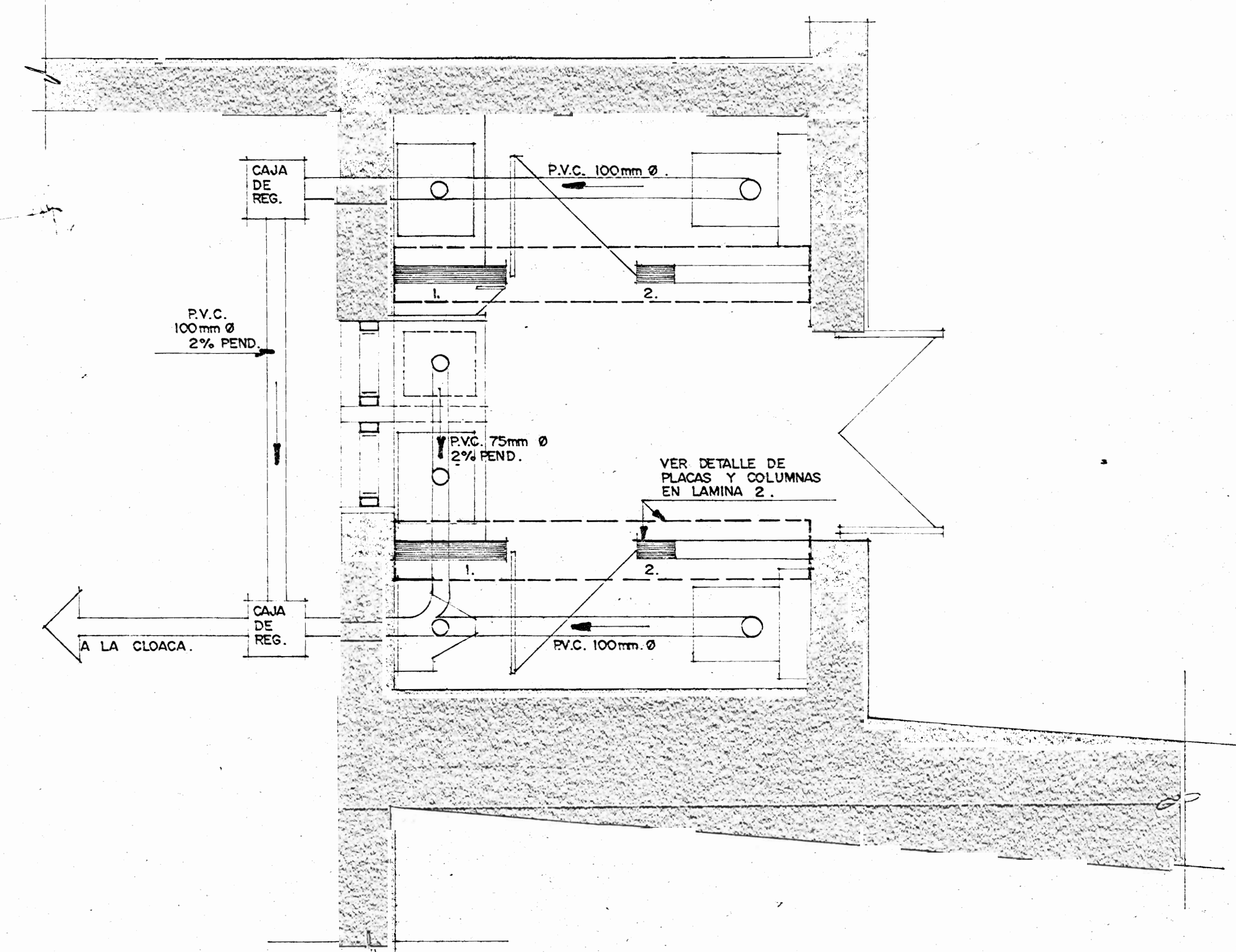
PLANTA DE CIMIENTOS, COLUMNAS E INSTALACIONES MECANICAS esc 1:20.
