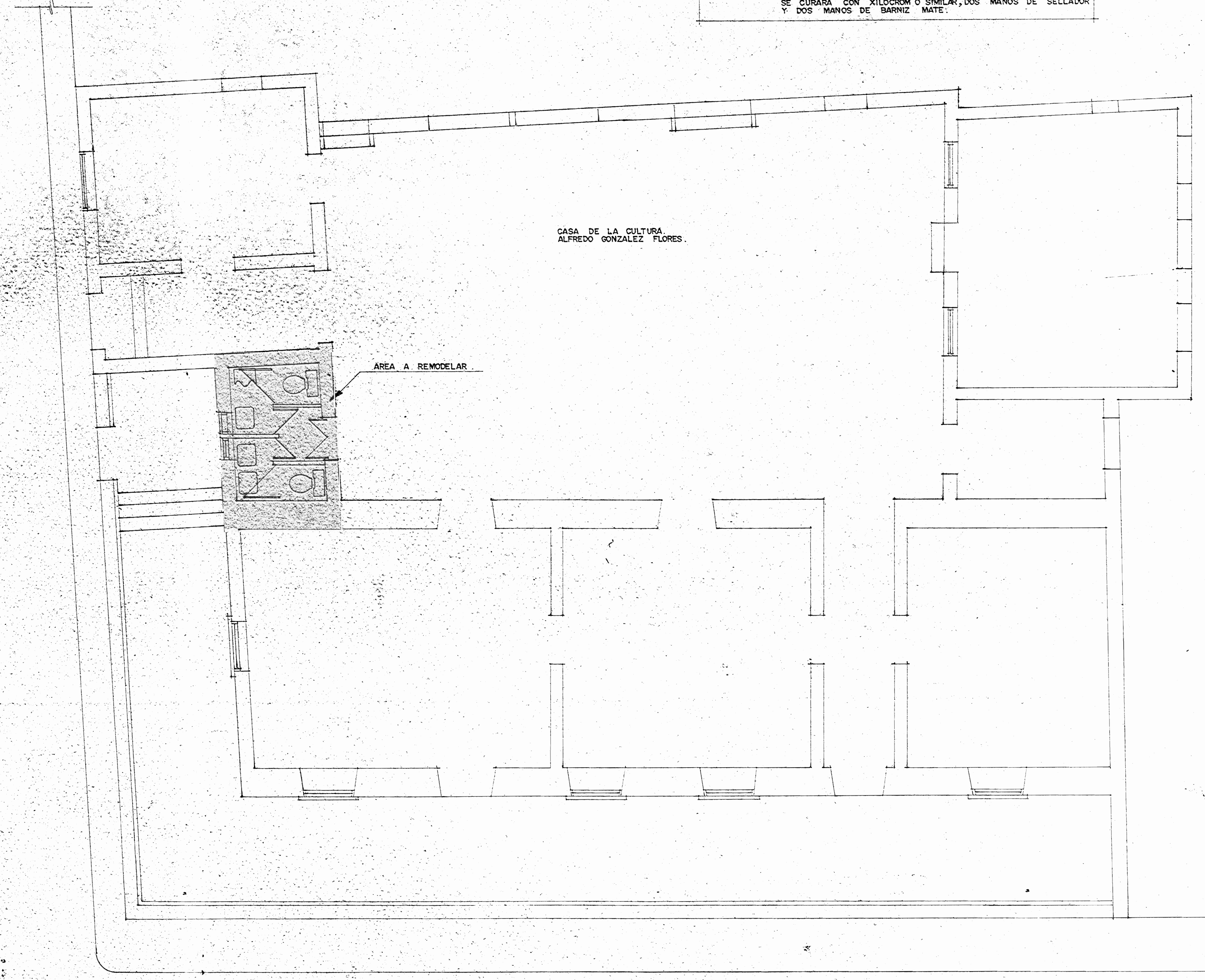
PLANTA DE DISTRIBUCION ARQUITECTONICA ESTADO ACTUAL esc. 1:50.
