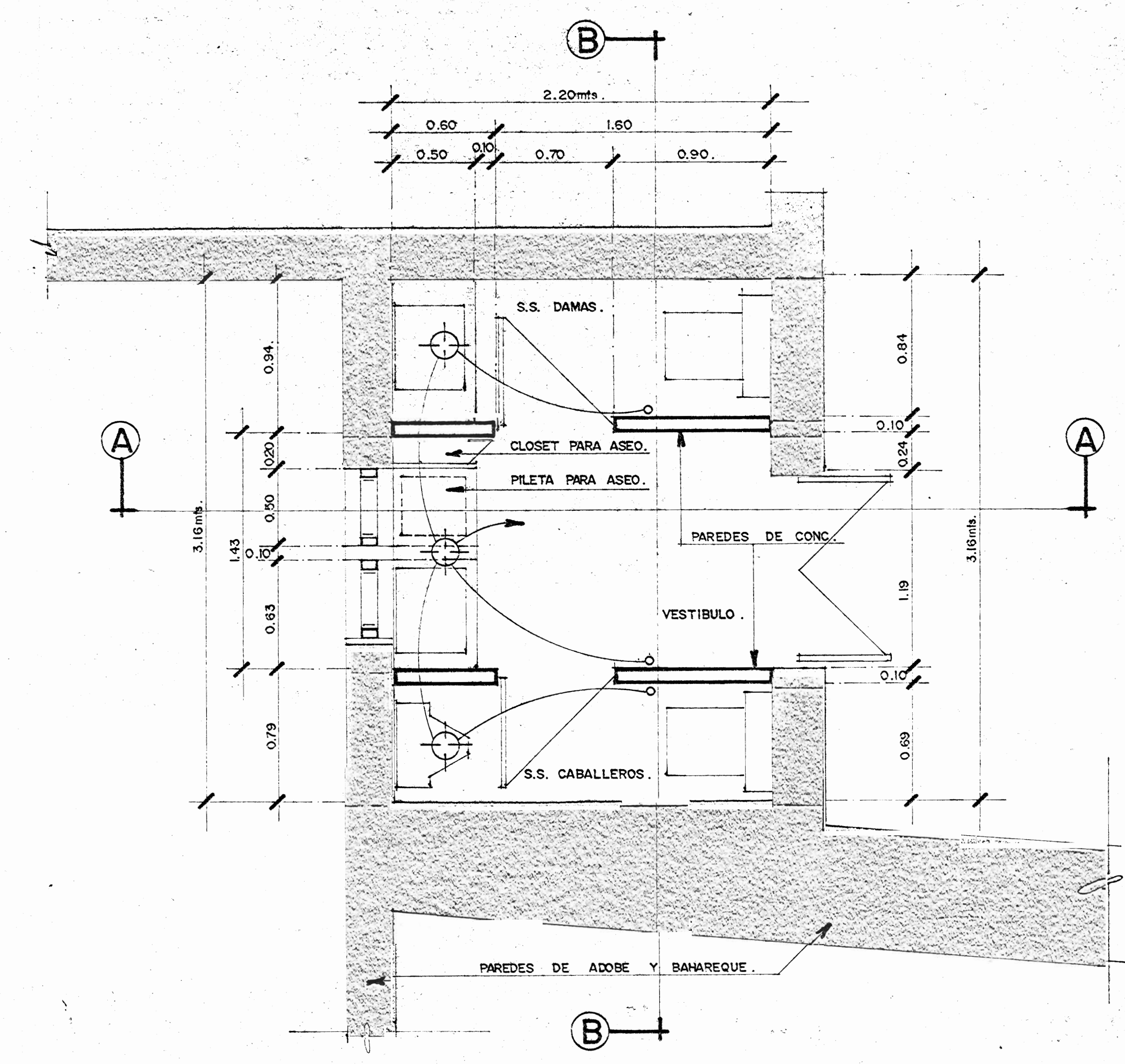
PLANTA DE DISTRIBUCION ARQUITECTONICA, ELECTRICA Y DE ACABADOS DEL AREA DE SERV. SANITARIOS -remodelacion.- esc. 1:20.
