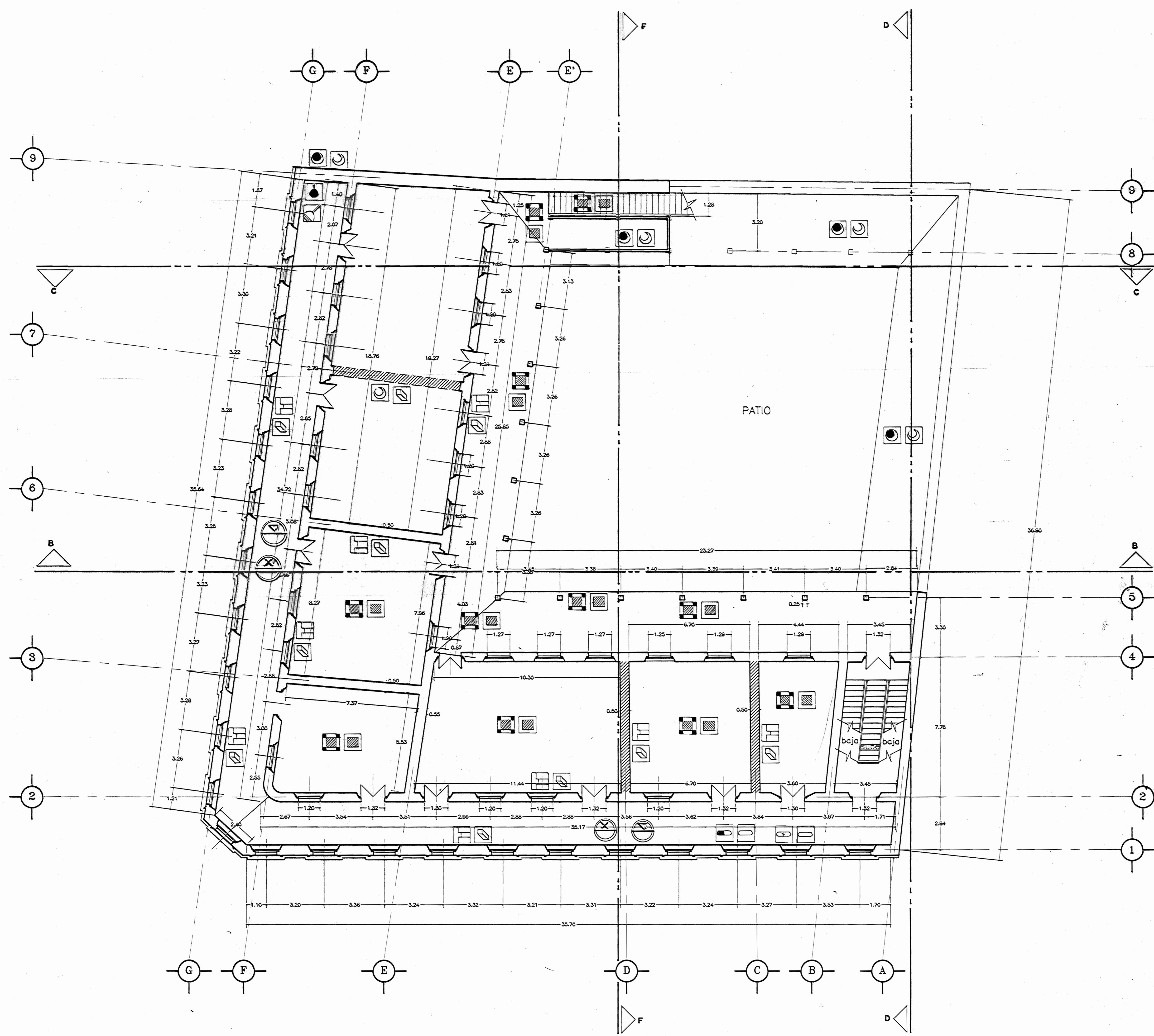
PLANTA ALTA ESTADO ACTUAL.
