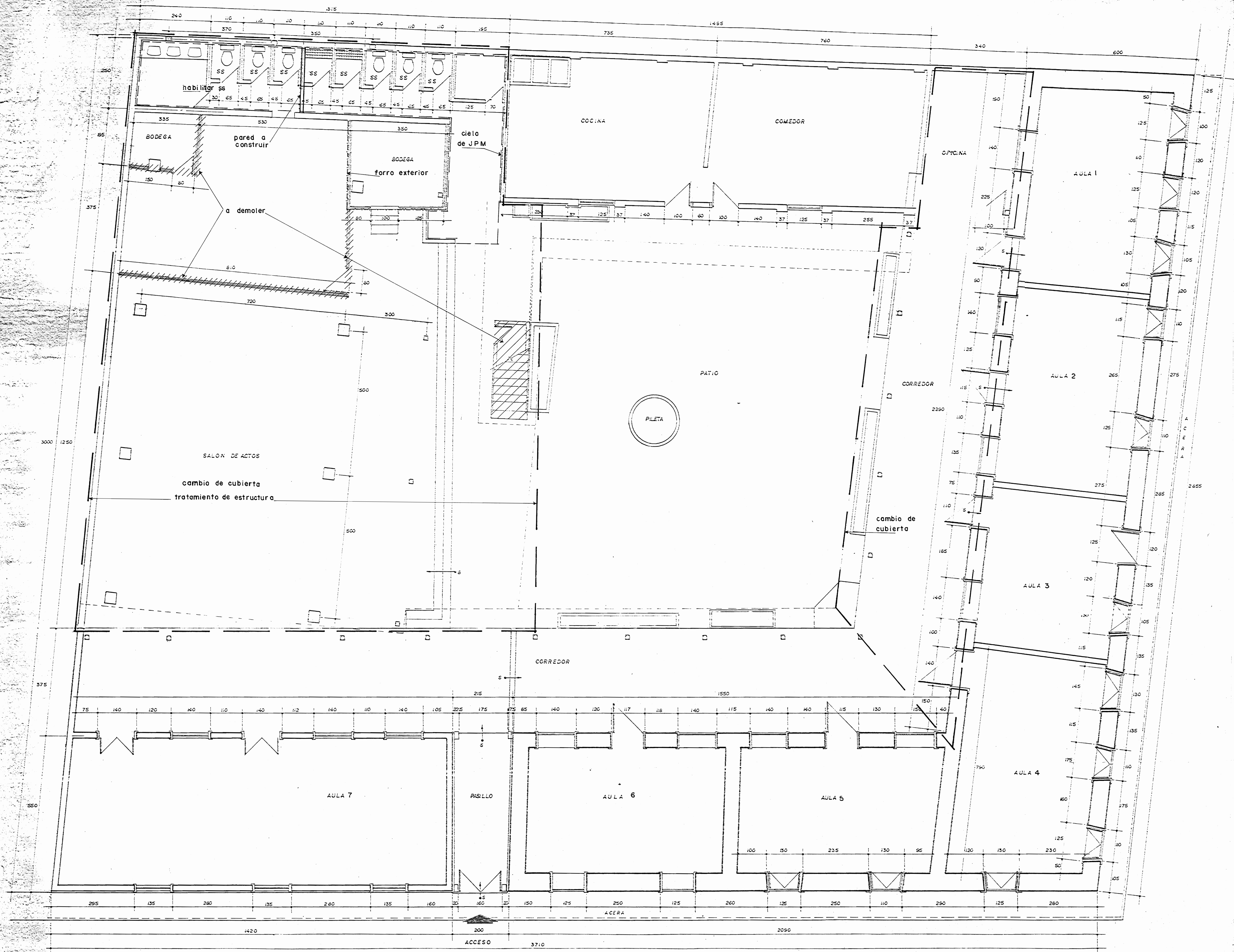
PLANTA DE DISTRIBUCION ARQUITECTONICA ESC. 1:50
