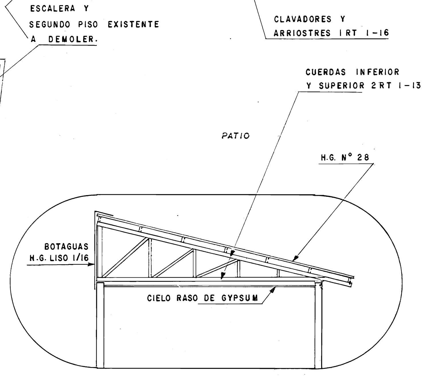
DETALLE DE ESTRUCTURA Y CUBIERTA QUE SUSTITUYE AREA DEMOLIDA 1:50
