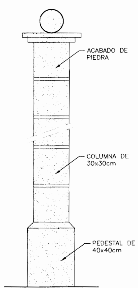
COLUMNA DE TAPIA ESCALA 1:20
