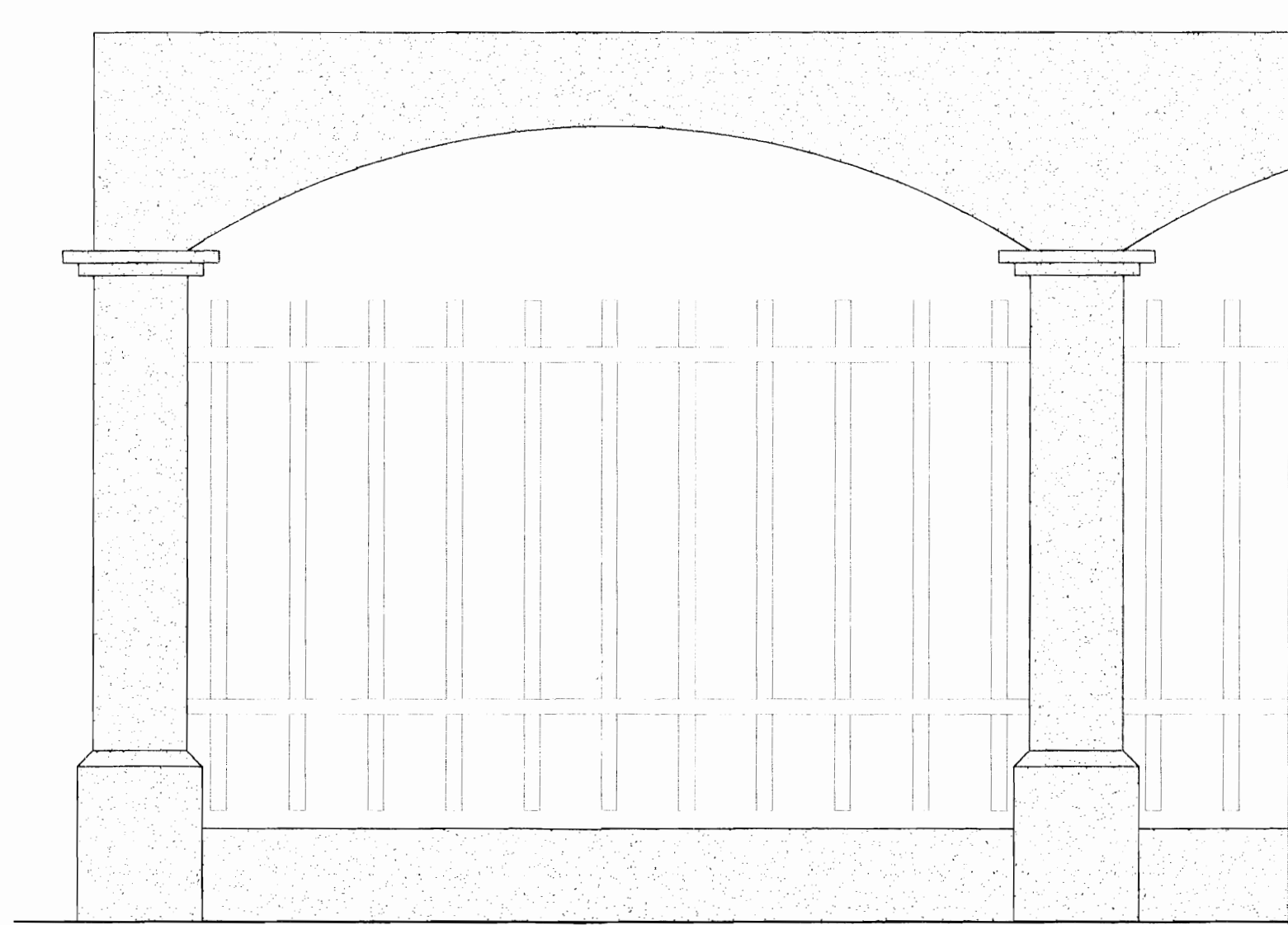
ELEVACION DE TAPIA ESCALA 1:20
