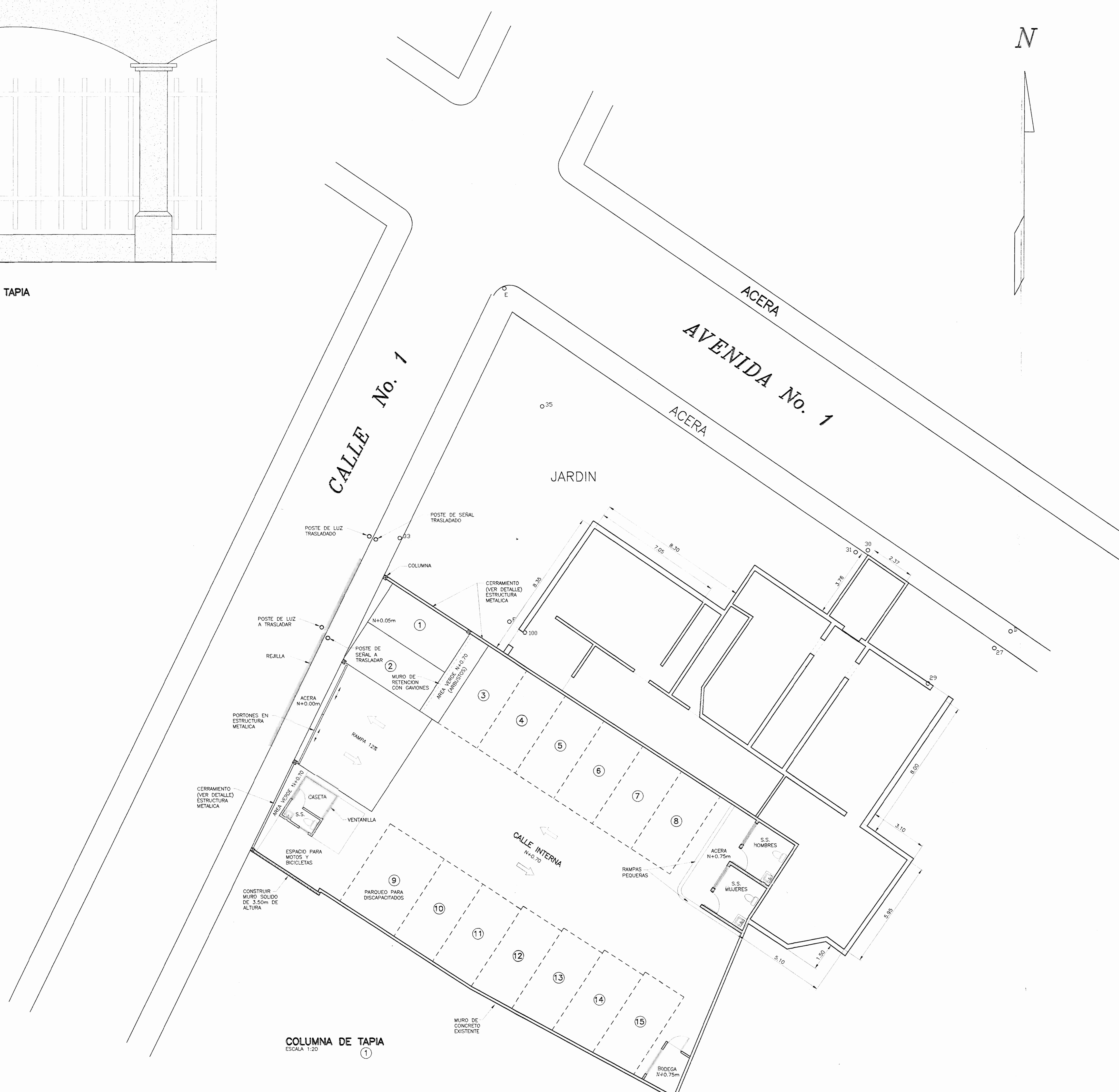
PLANTA DE PARQUEO ESCALA 1:100
