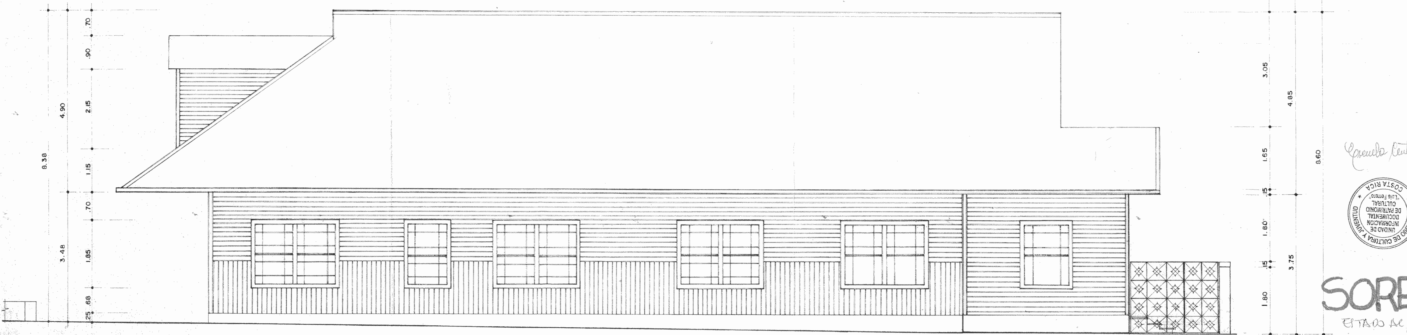
ELEVACION LATERAL OESTE ESC: 1/50
