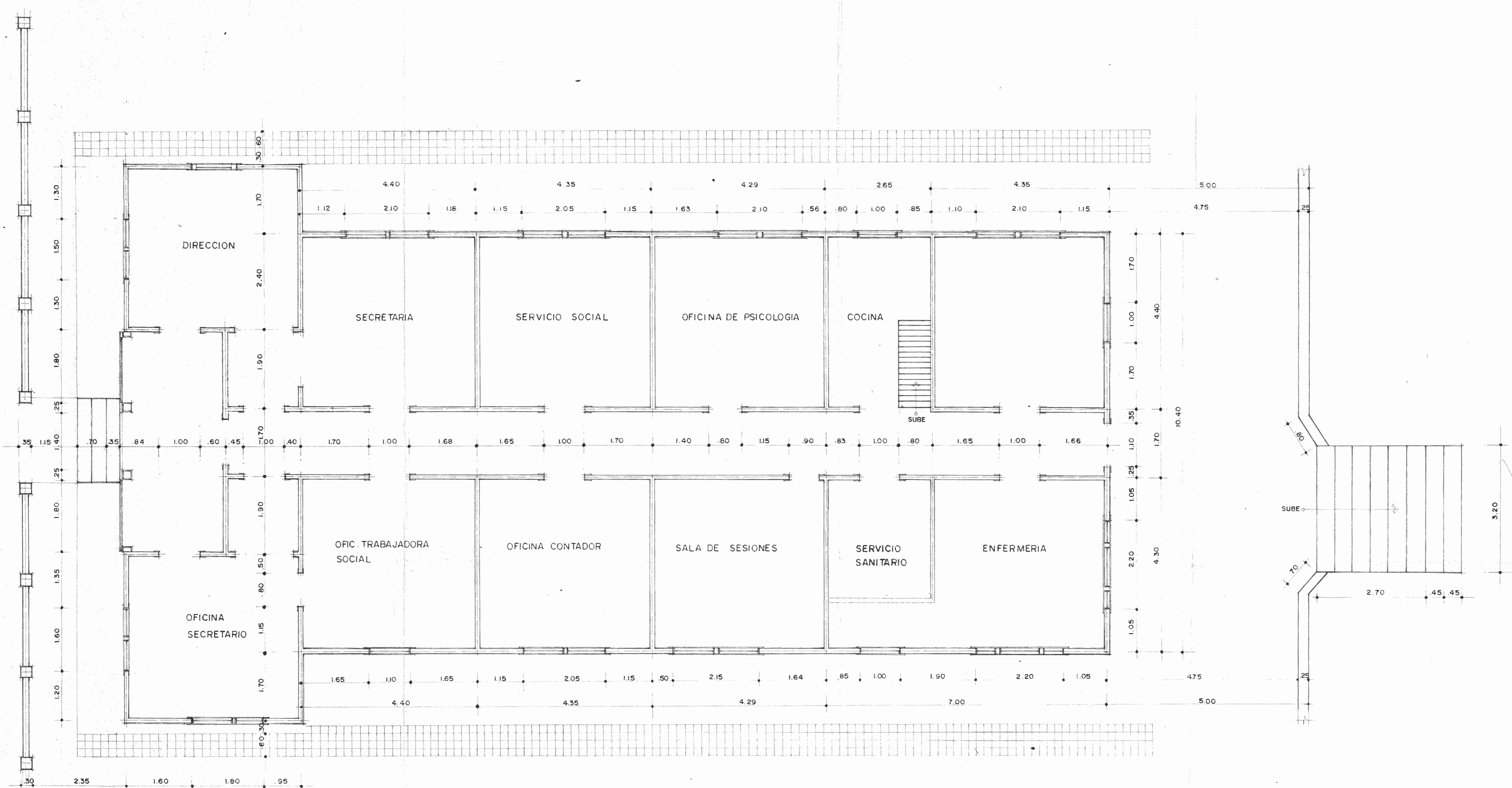
PLANTA DE DISTRIBUCION ARQUITECTONICA, ESC 1:50
