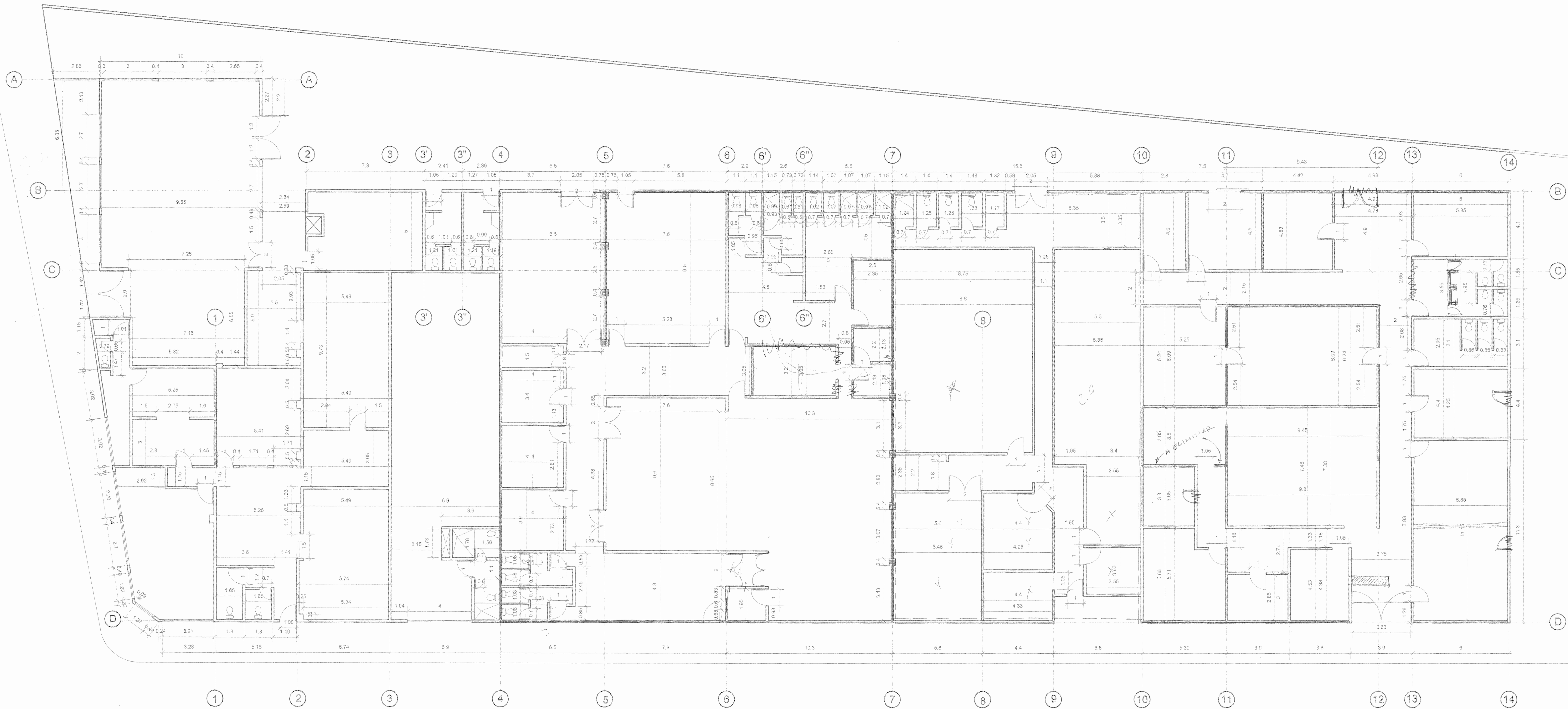
PLANTA DE DISTRIBUCION ARQUITECTONICA ACTUAL ESC: 1:100 CASA DEL ARTISTA.
