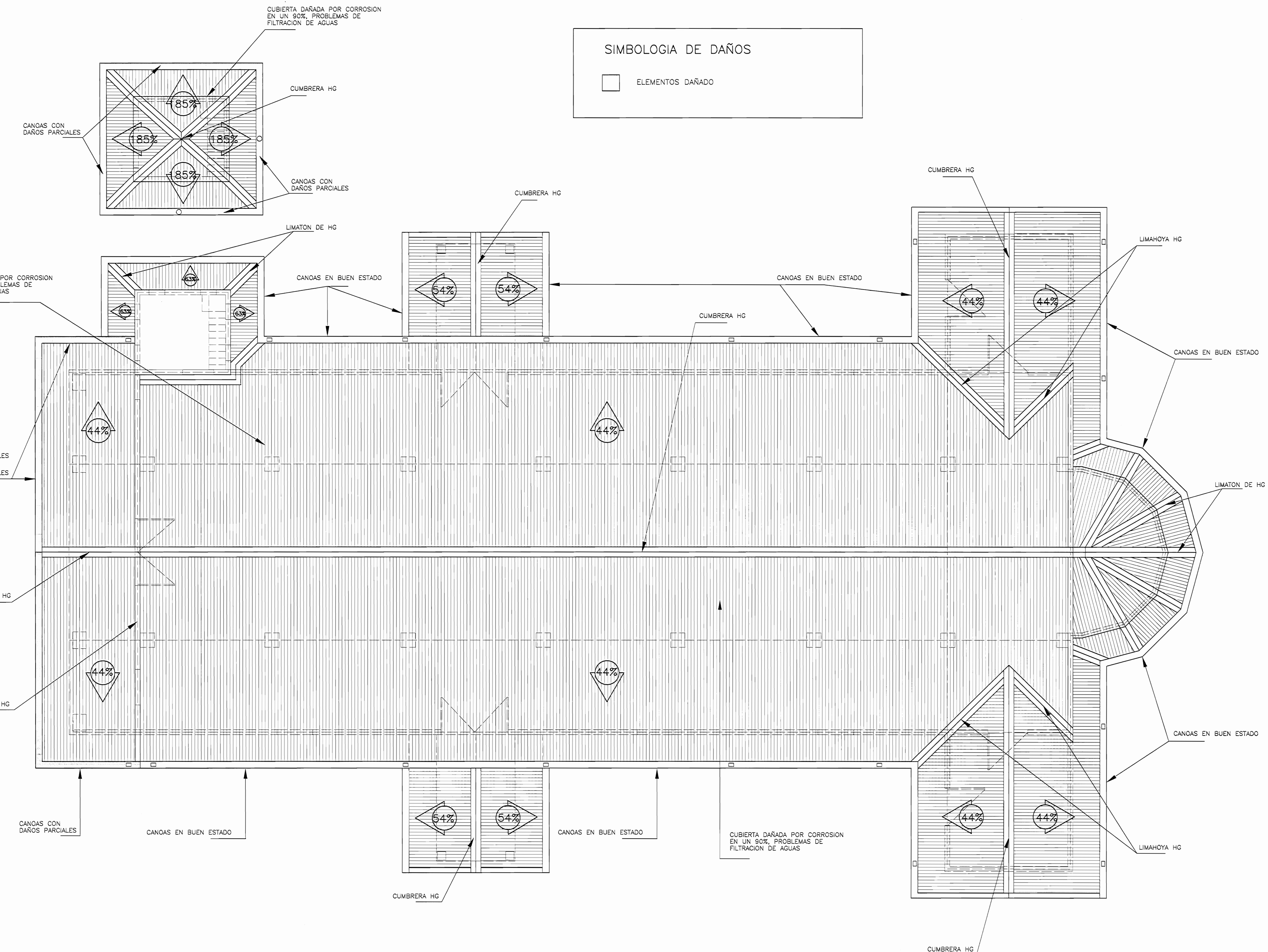
PLANTA DE CUBIERTAS Y EVACUACION PLUVIAL ESC. 1 : 50
