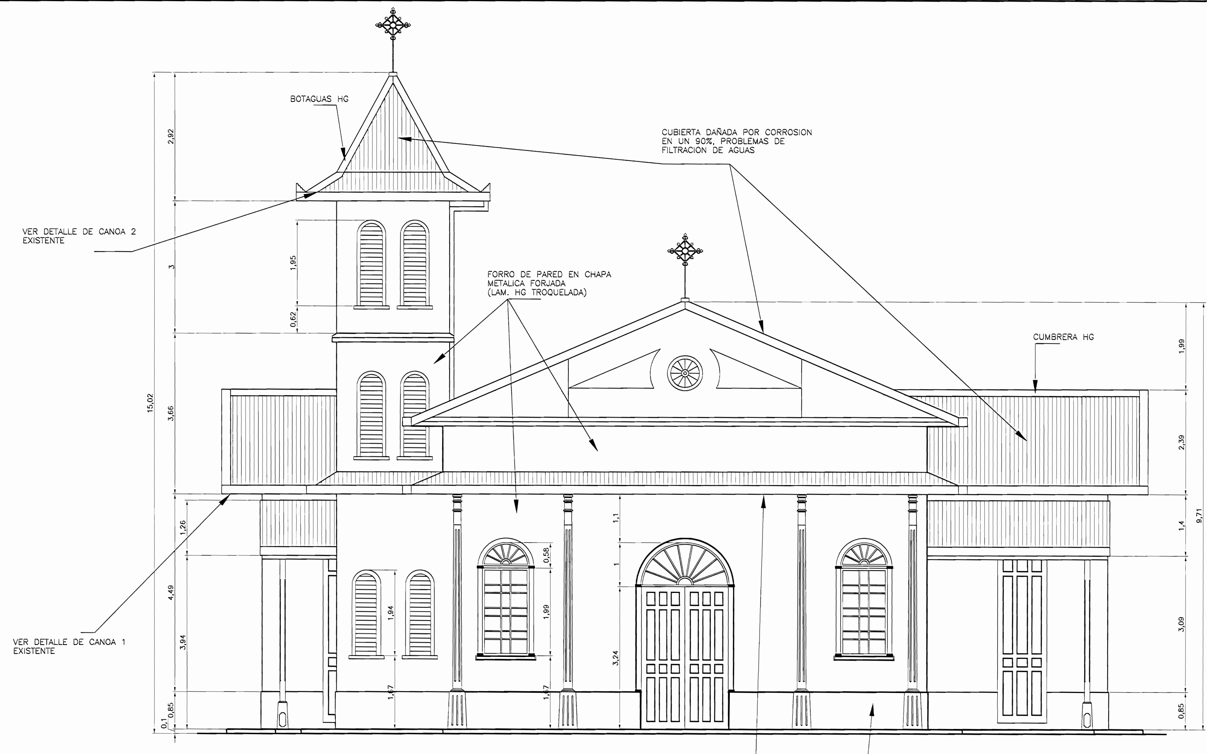
FACHADA OESTE ESC. 1 : 50
