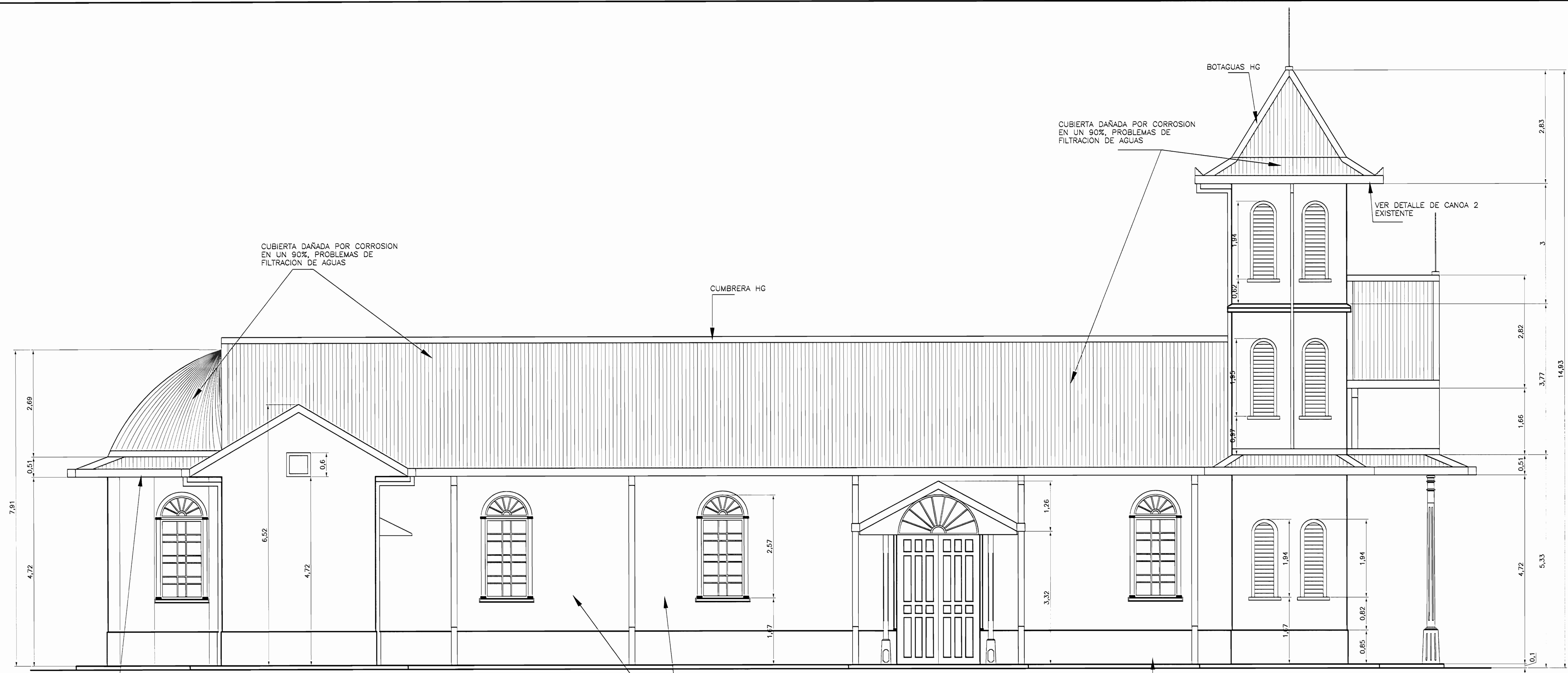
FACHADA NORTE ESC. 1 : 50
