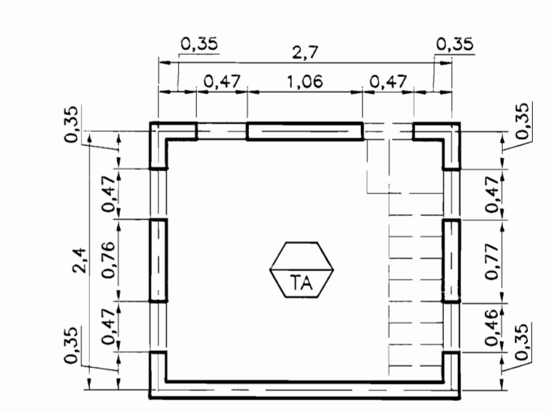
PLANTA MEZANINE, TORRE ESC. 1 : 50
