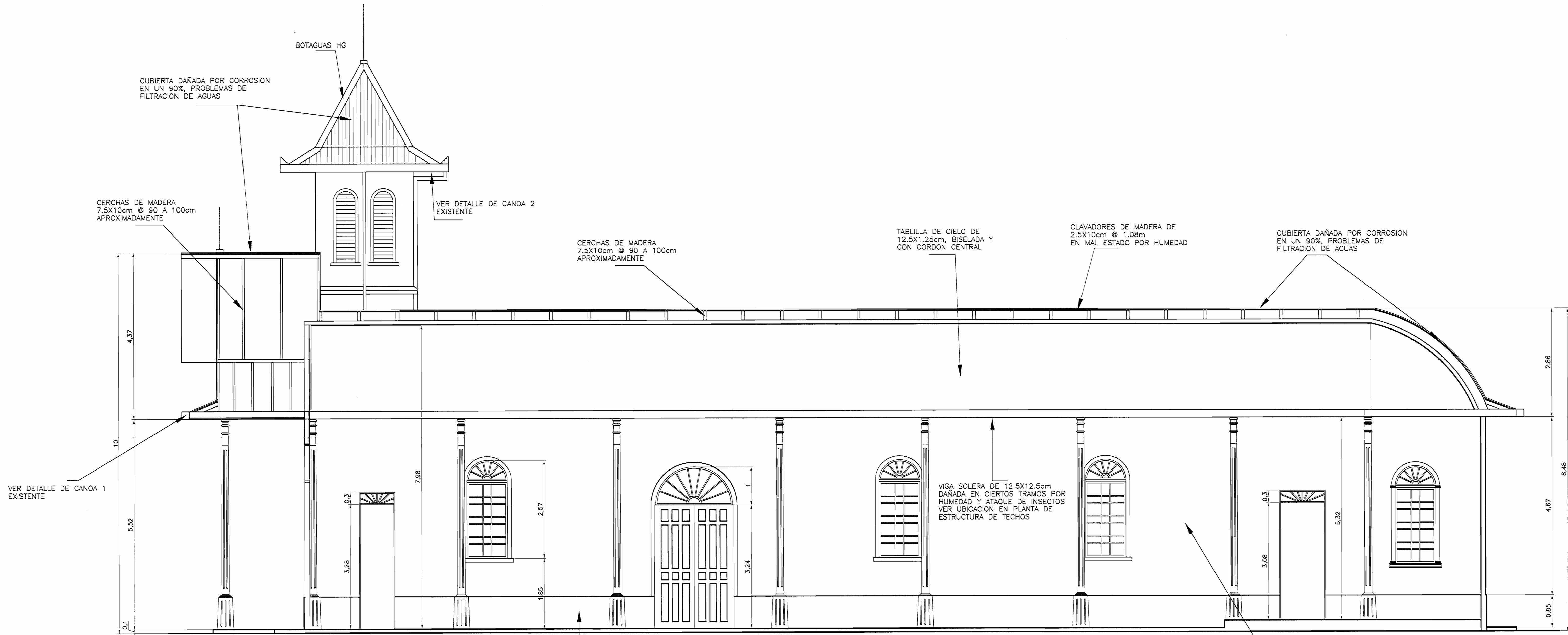
CORTE A-A ESC. 1 : 50
