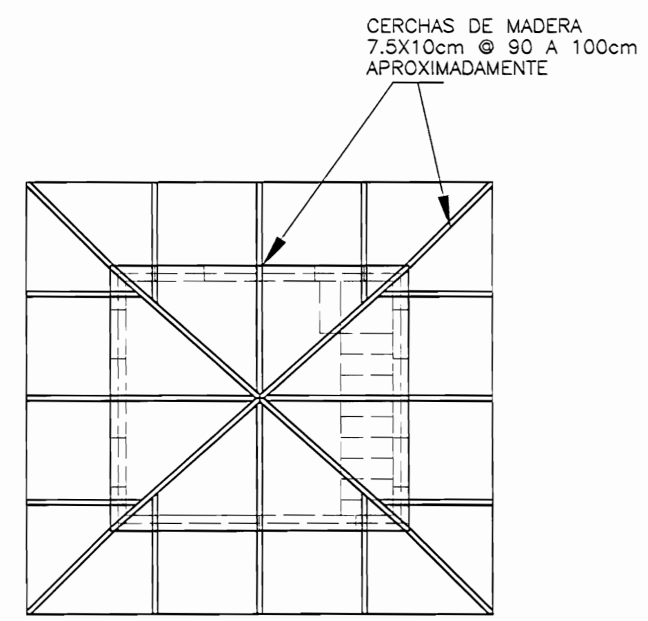
PLANTA DE ESTRUCTURA DE CERCHAS, TORRE ESC. 1 : 50
