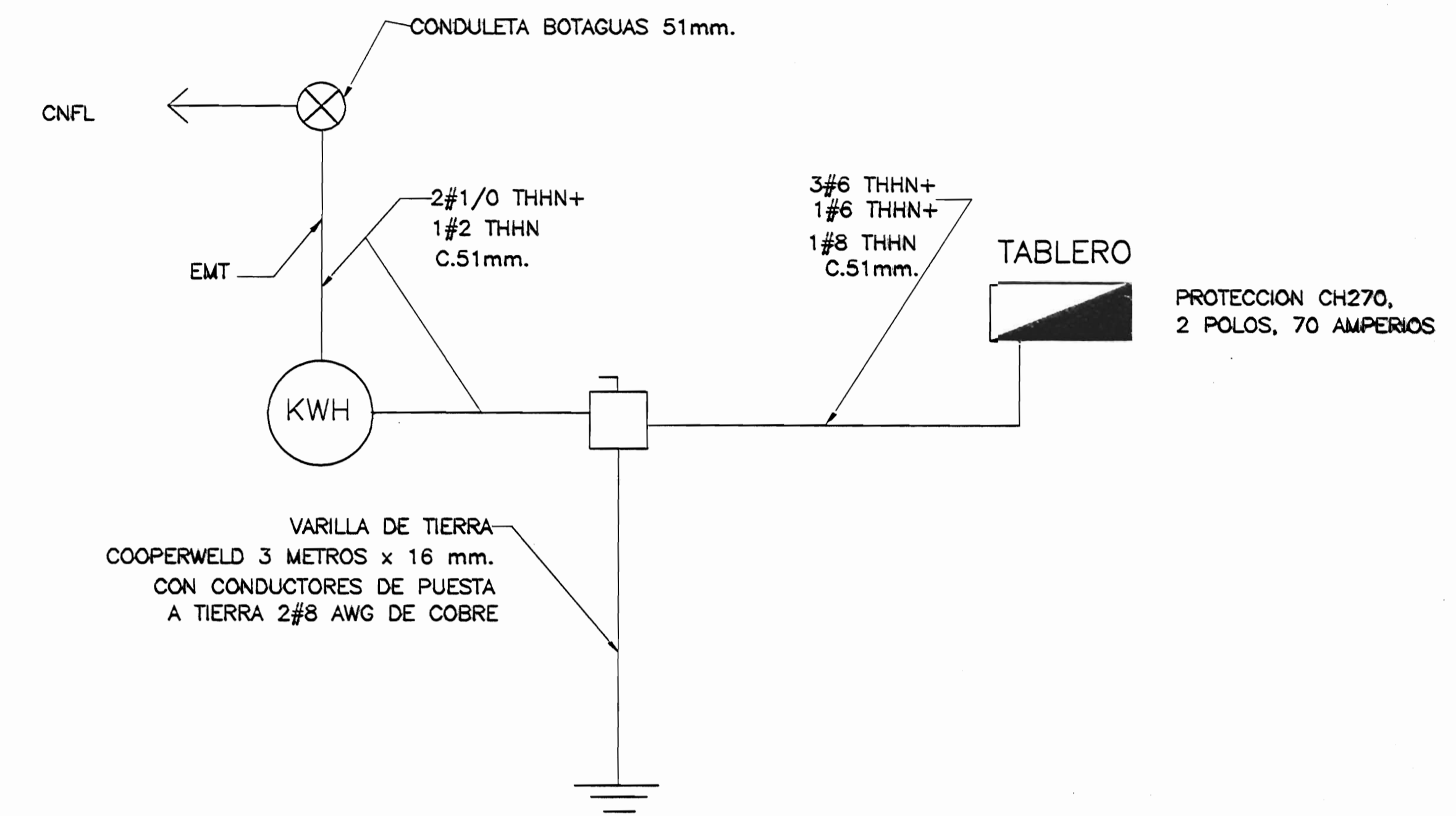
DIAGRAMA UNIFILAR ELECTRICO SIN ESCALA
