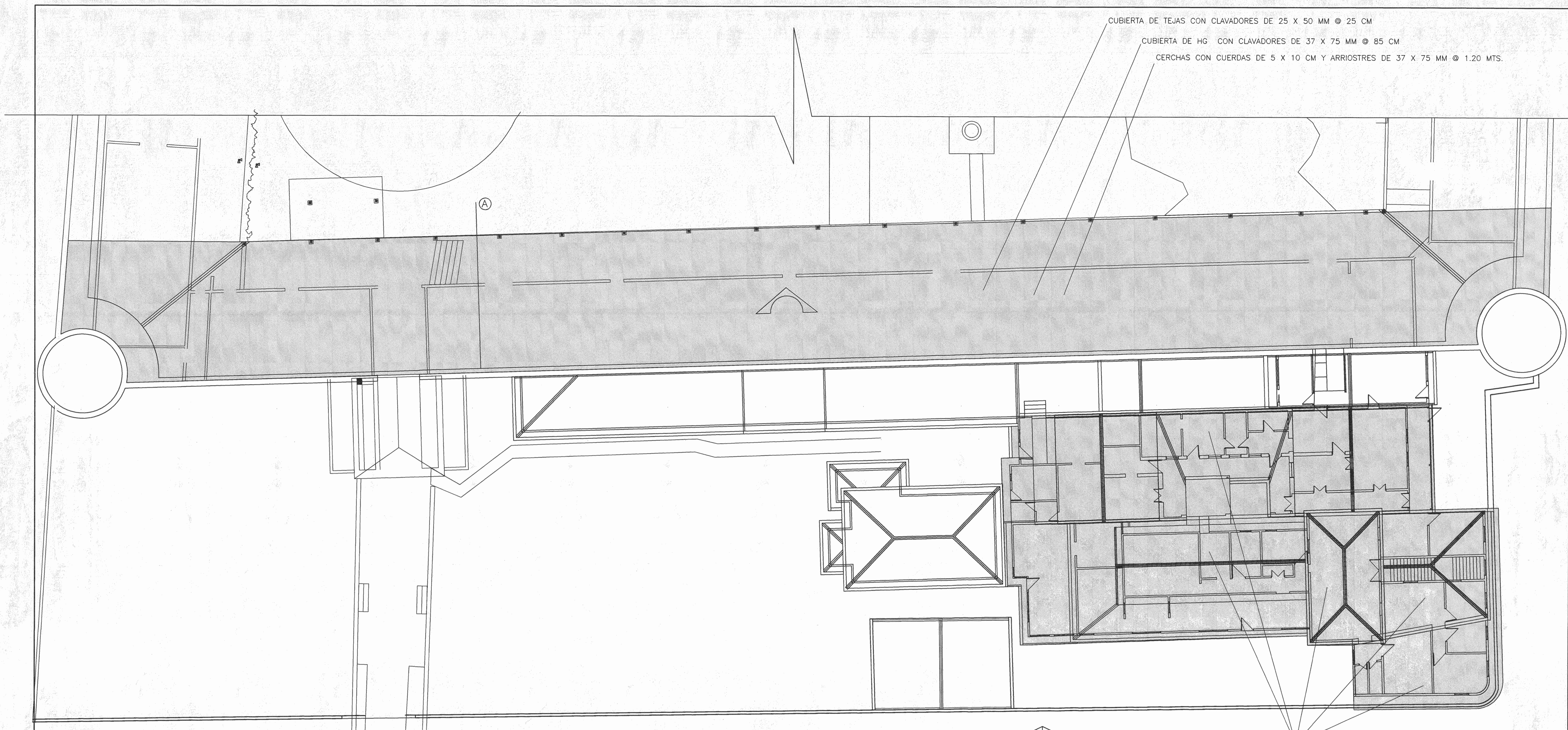
PLANTA DE TECHOS esc. 1:125
