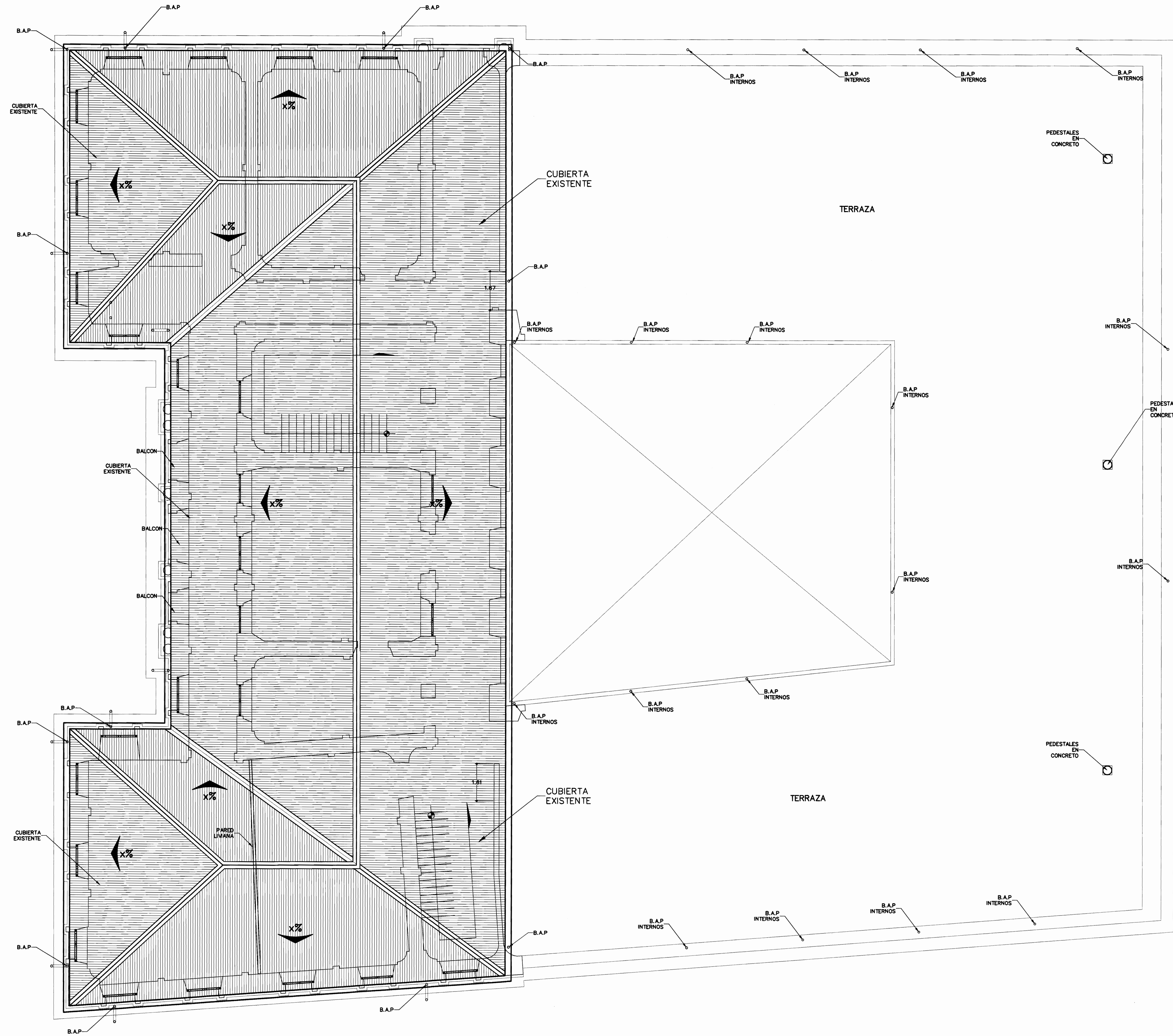
PLANTA DE TECHOS AZOTEA. ESCALA 1:75.
