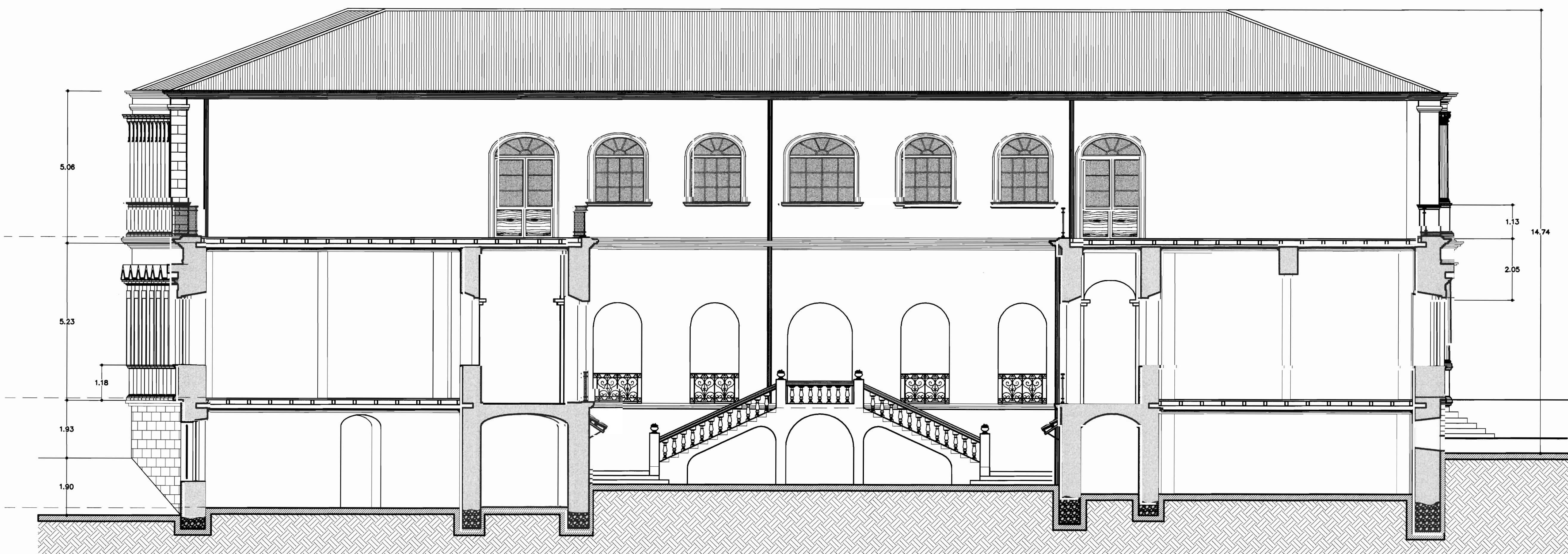
CORTE POR B-B. ESCALA 1:75.
