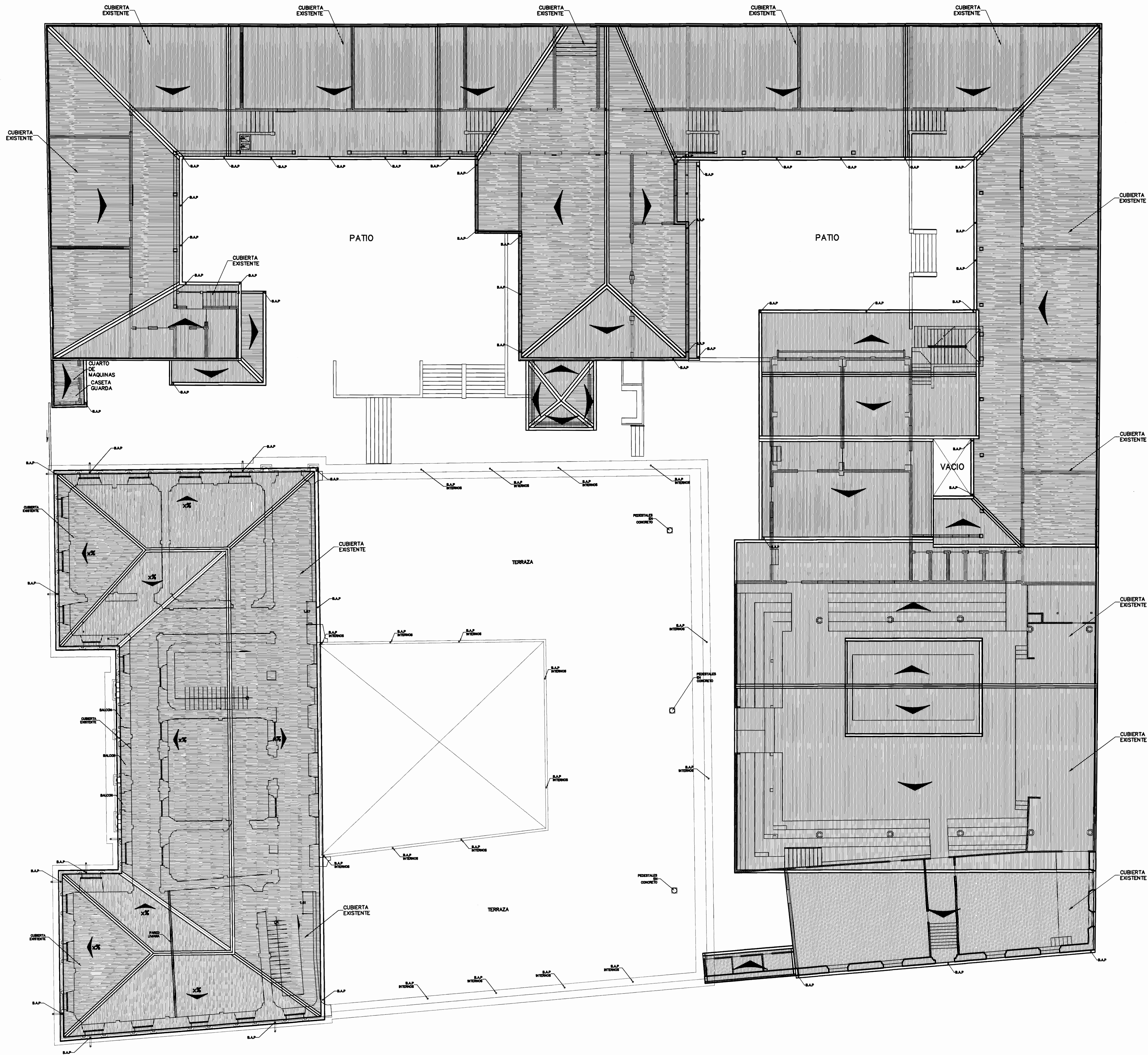
PLANTA CONJUNTO DE TECHOS. ESCALA 1:125.
