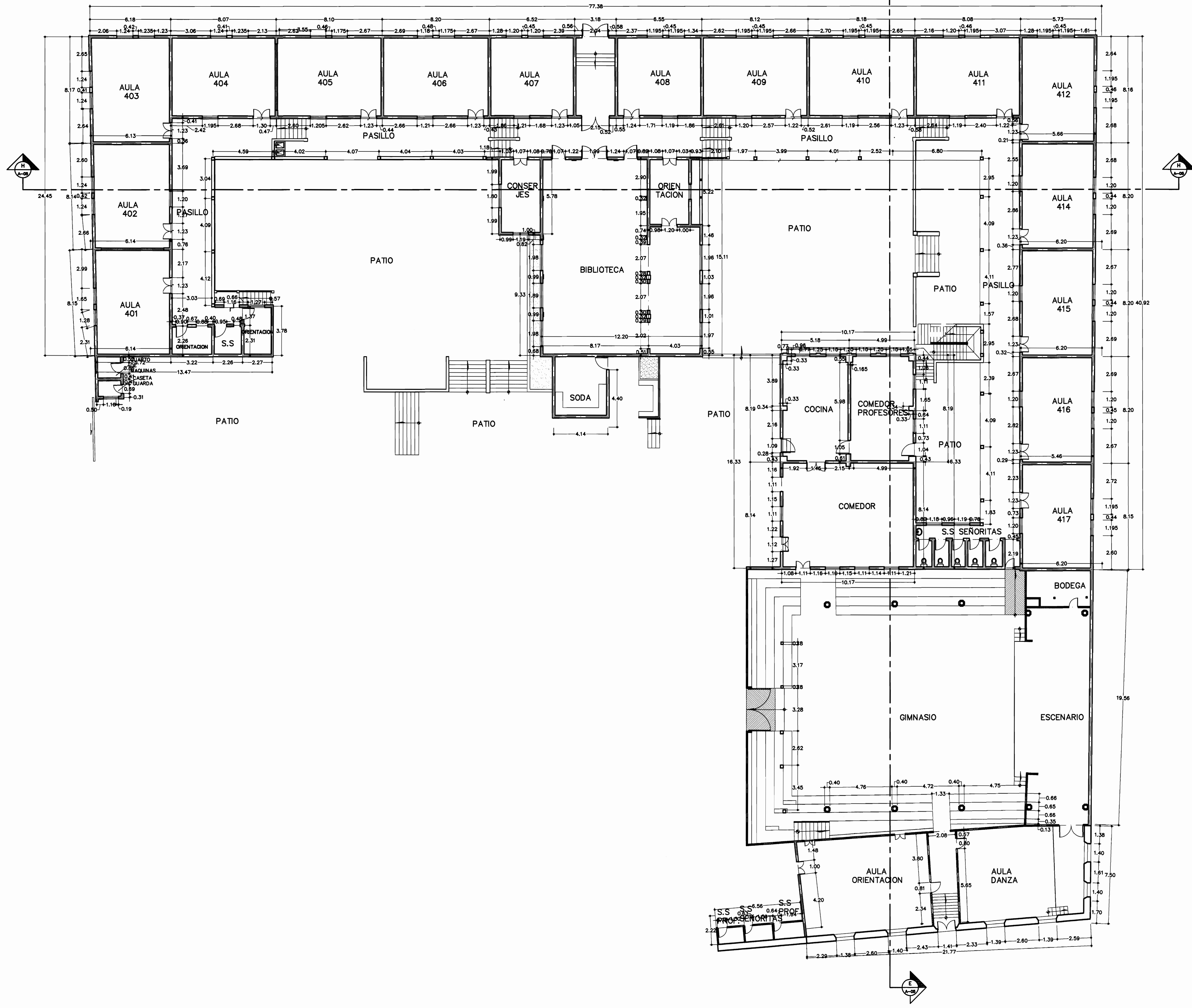
PLANTA ARQUITECTÓNICA ESCUELA. ESCALA 1:125.
