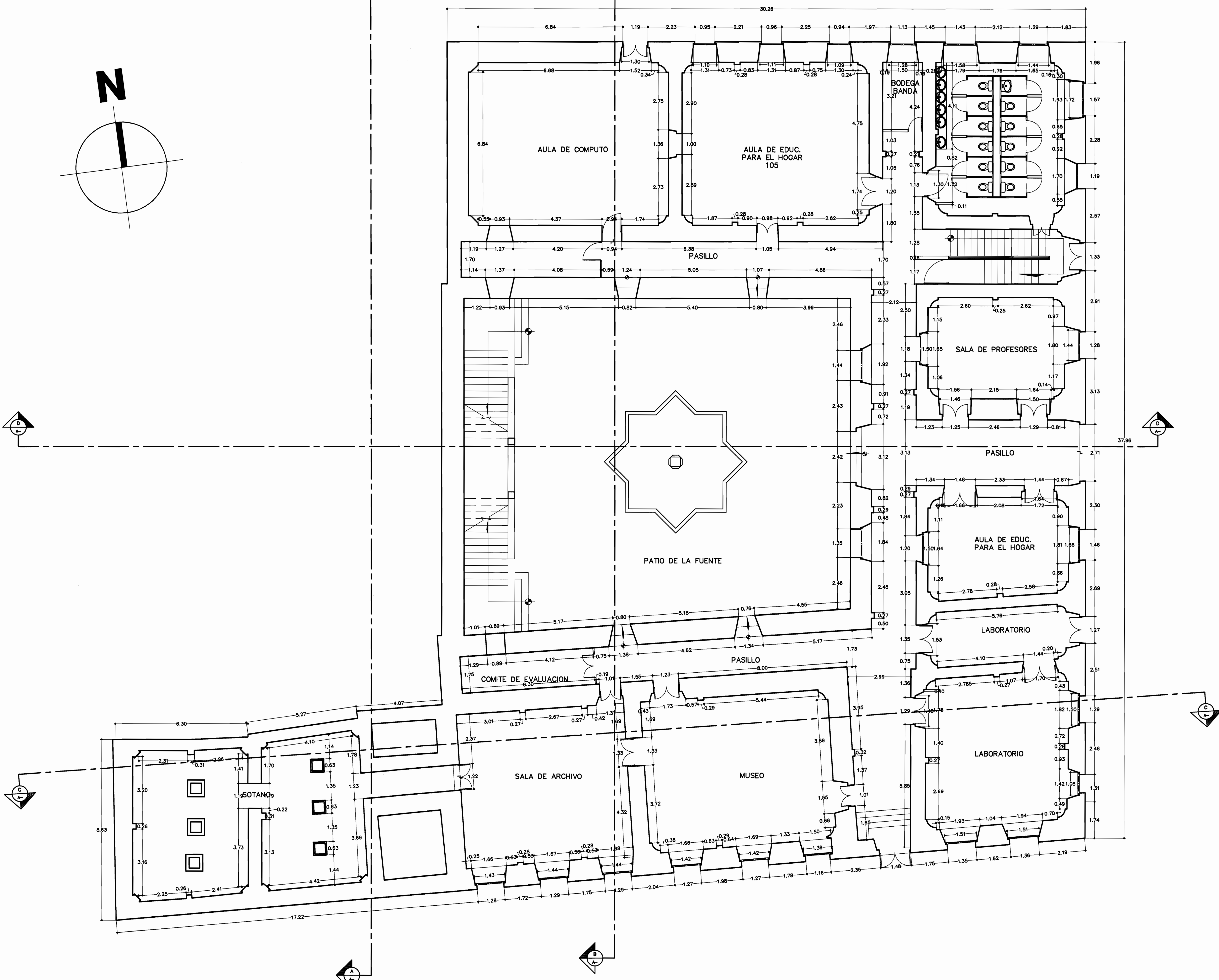
PLANTA ARQUITECTÓNICA SOTANO. ESCALA 1:75.
