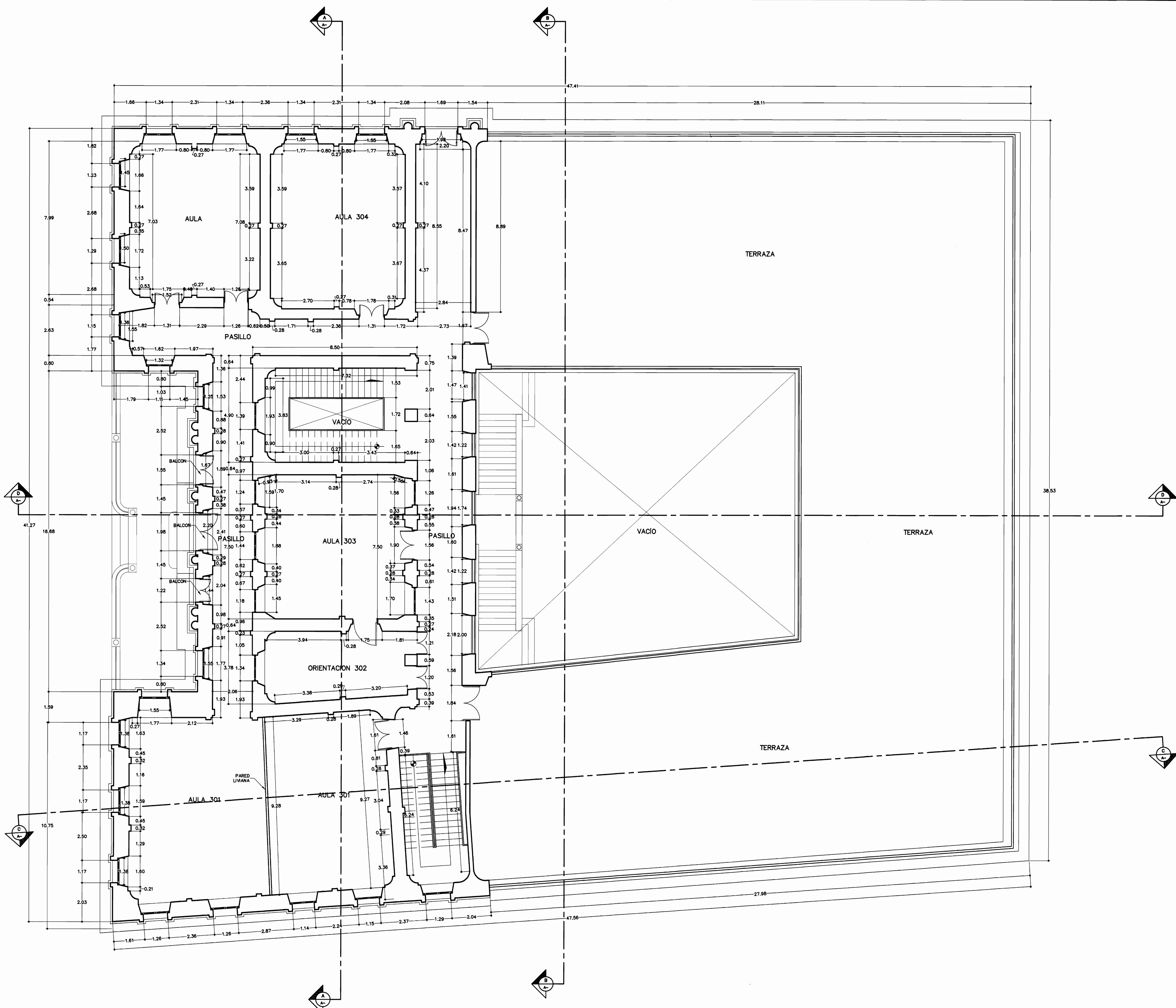
PLANTA ARQUITECTÓNICA SEGUNDO NIVEL. ESCALA 1:75.
