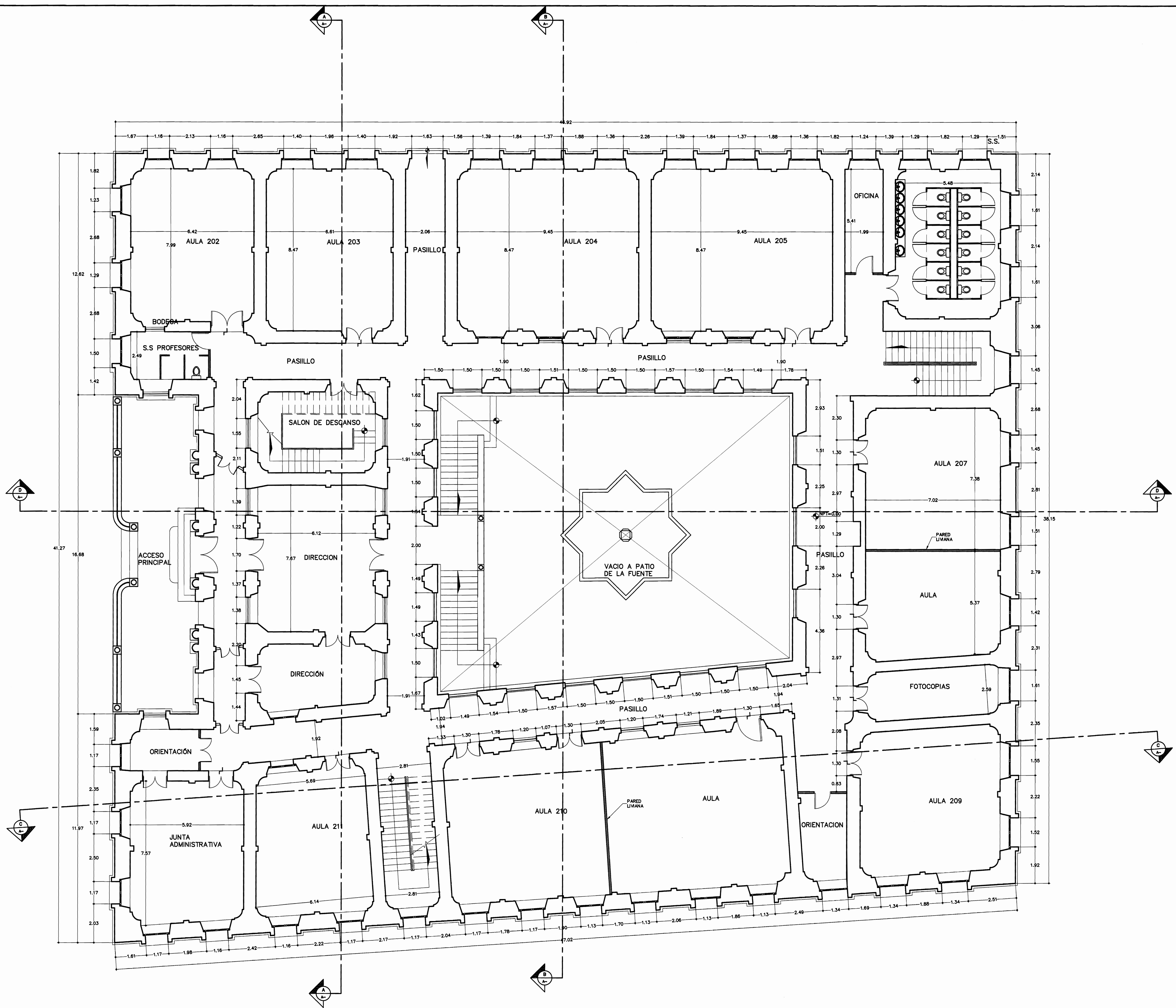
PLANTA ARQUITECTÓNICA PRINCIPAL. ESCALA 1:75.
