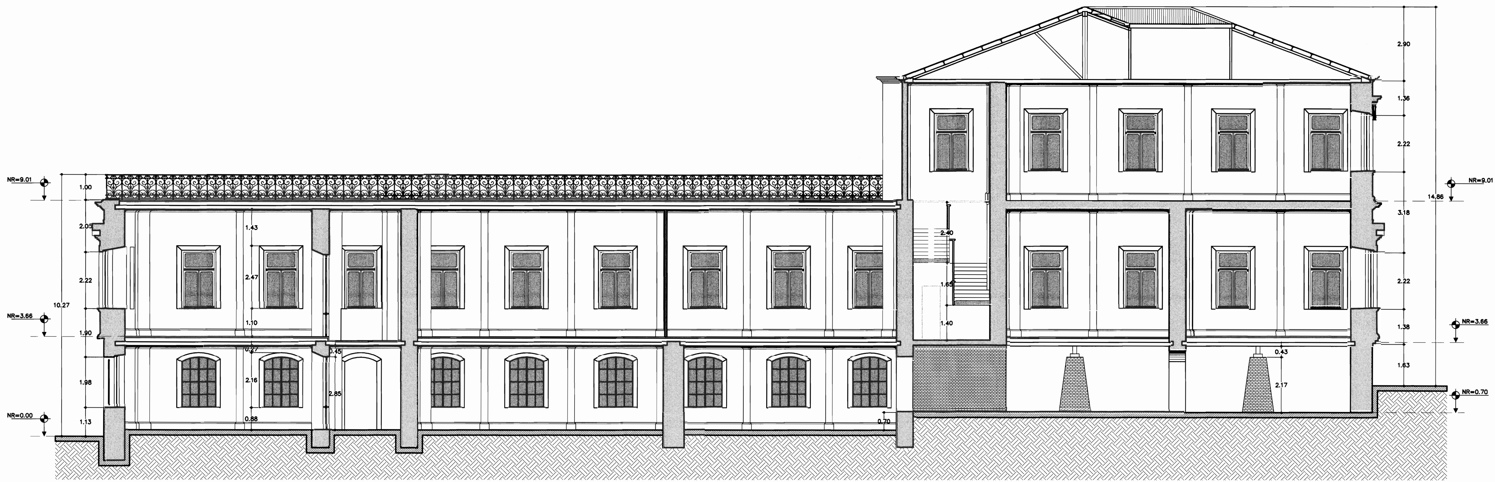
CORTE POR C-C. ESCALA 1:75.
