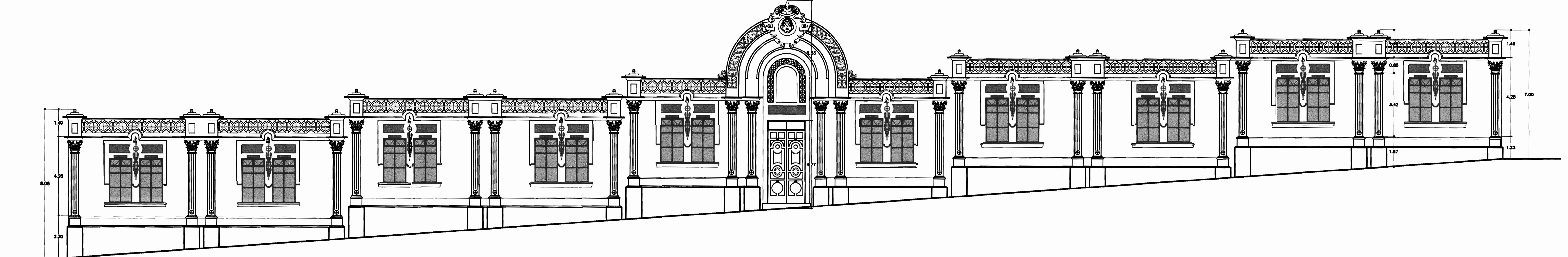
FACHADA NORTE (ESCUELA). ESCALA 1:100.
