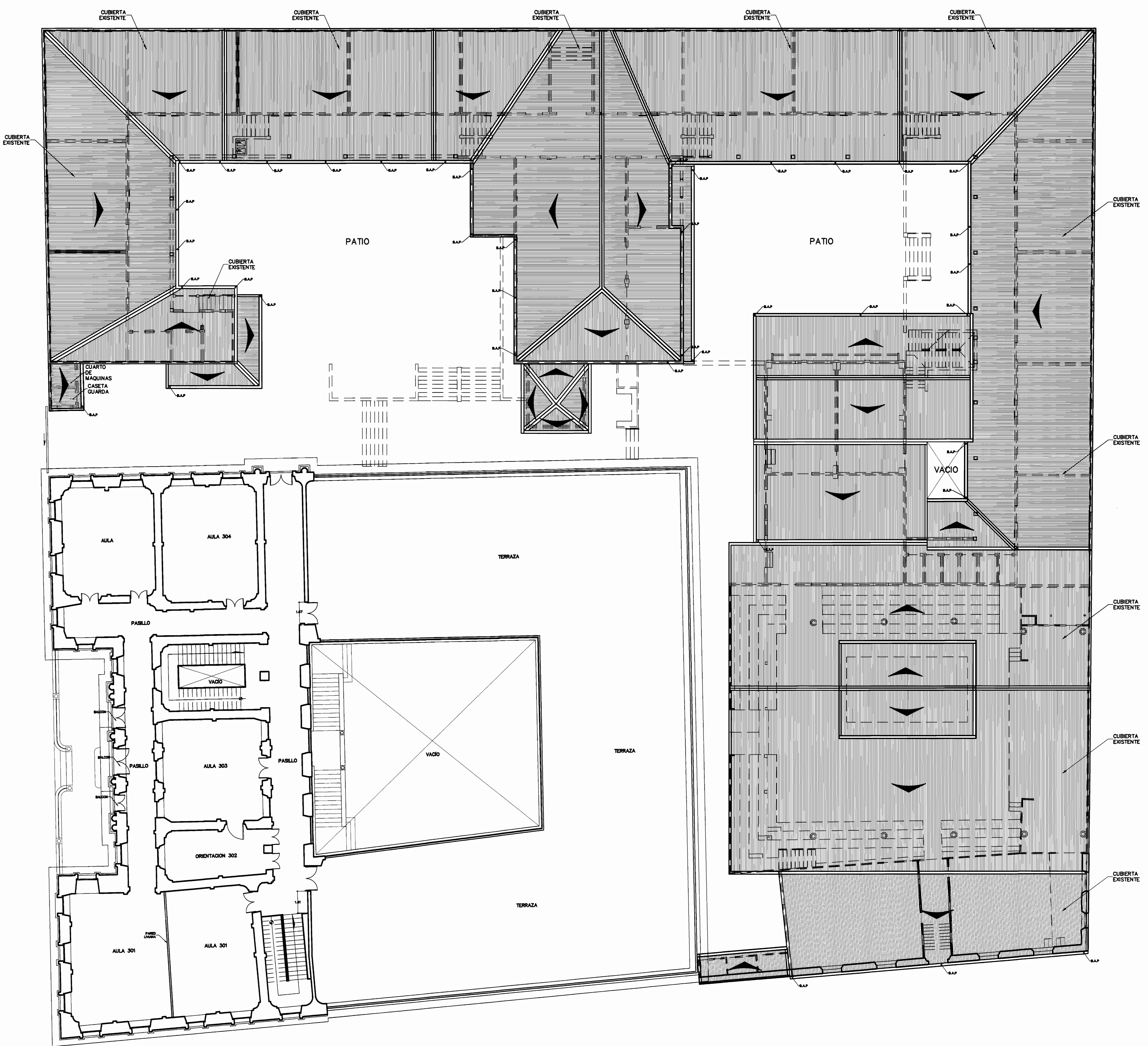
PLANTA CONJUNTO SEGUNDO NIVEL. ESCALA 1:125.
