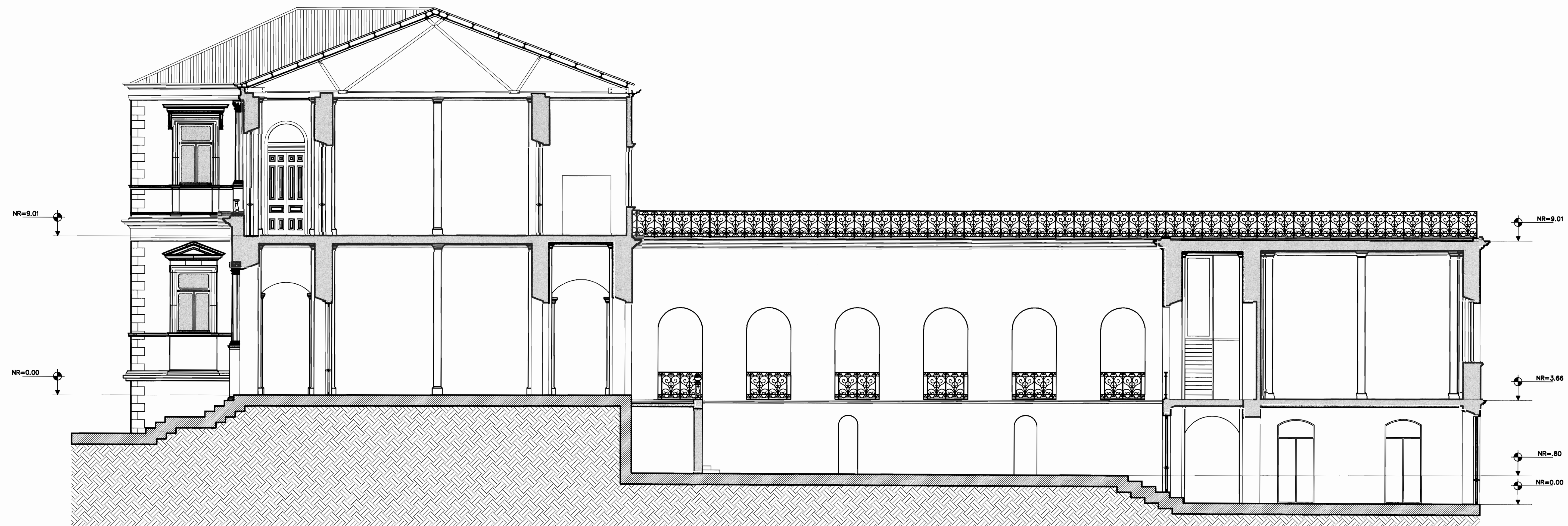
CORTE POR D-D. ESCALA 1:75.
