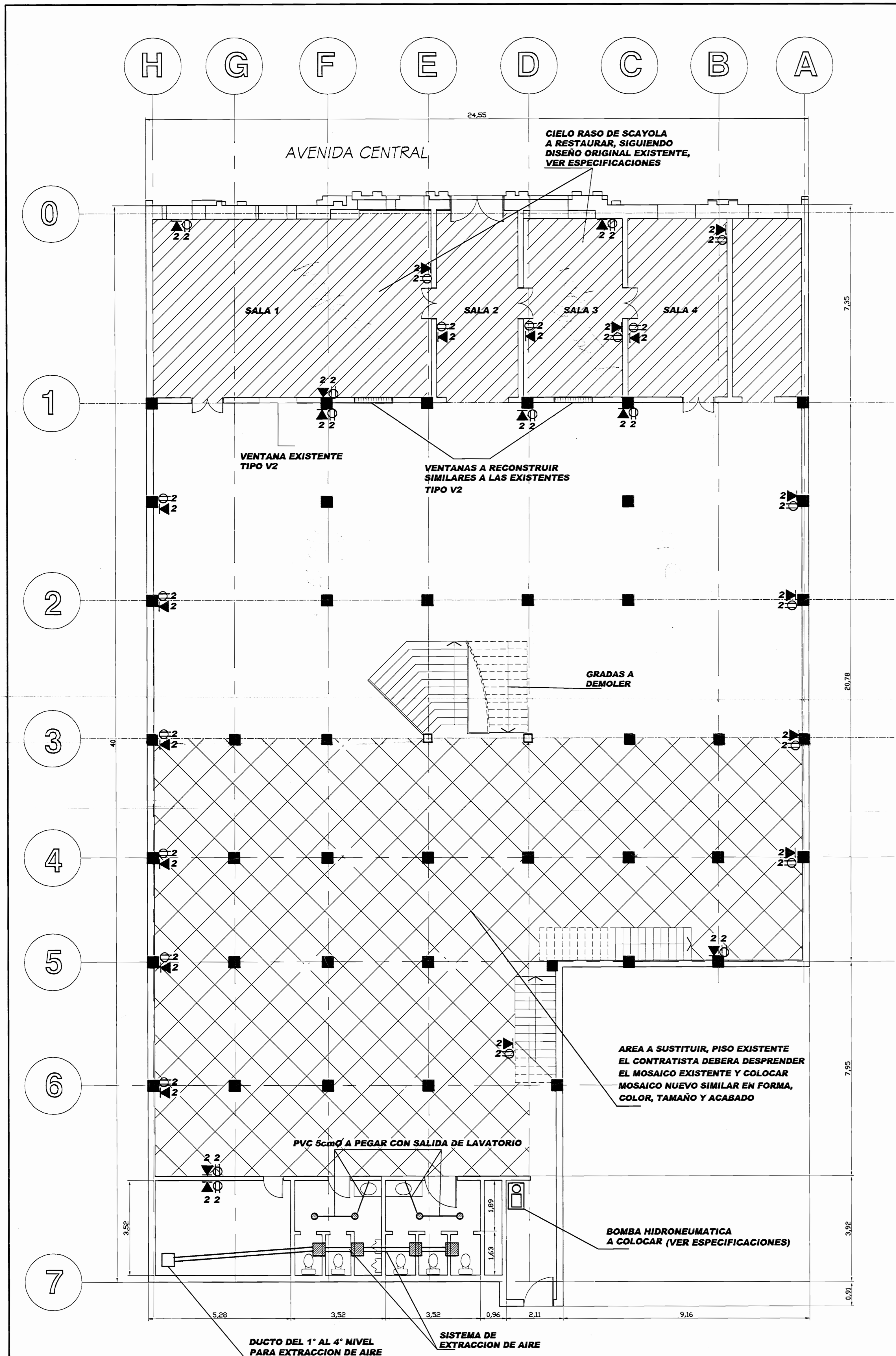
PLANTA PRIMER NIVEL NIVEL 0+0.00
