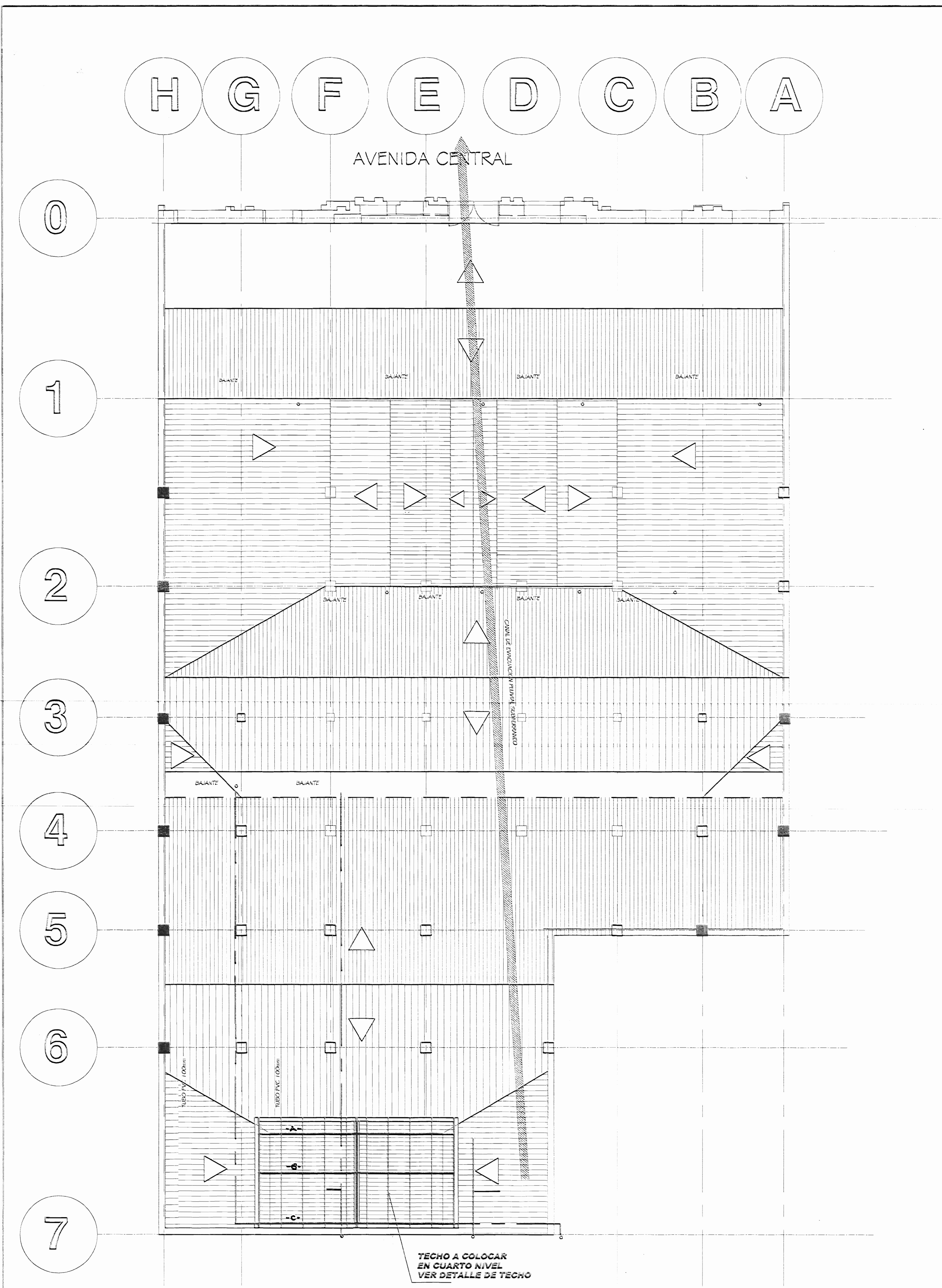
PLANTA DE TECHOS ESC. 1 : 75
