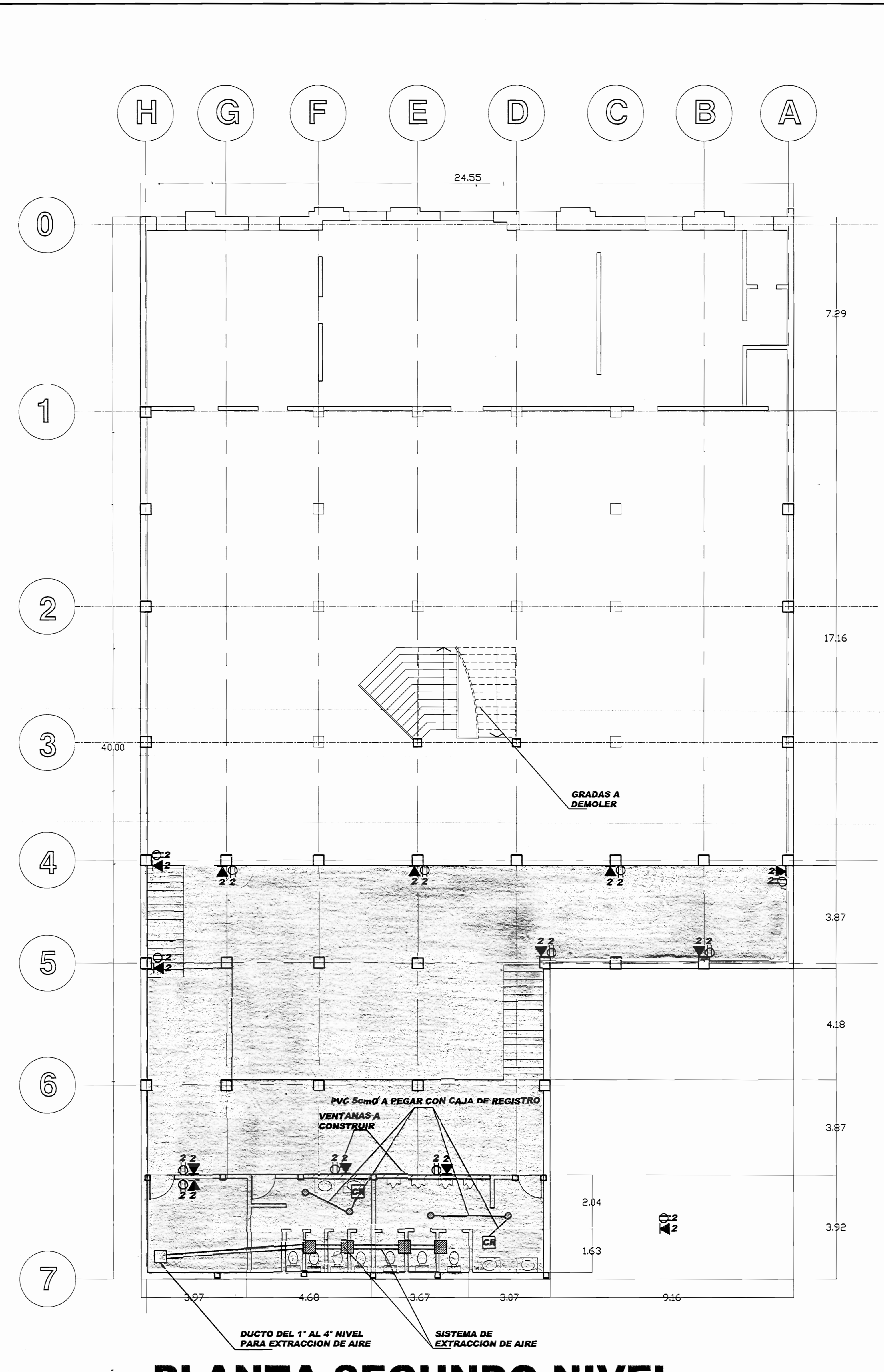
PLANTA SEGUNDO NIVEL NIVEL 0+3.00
