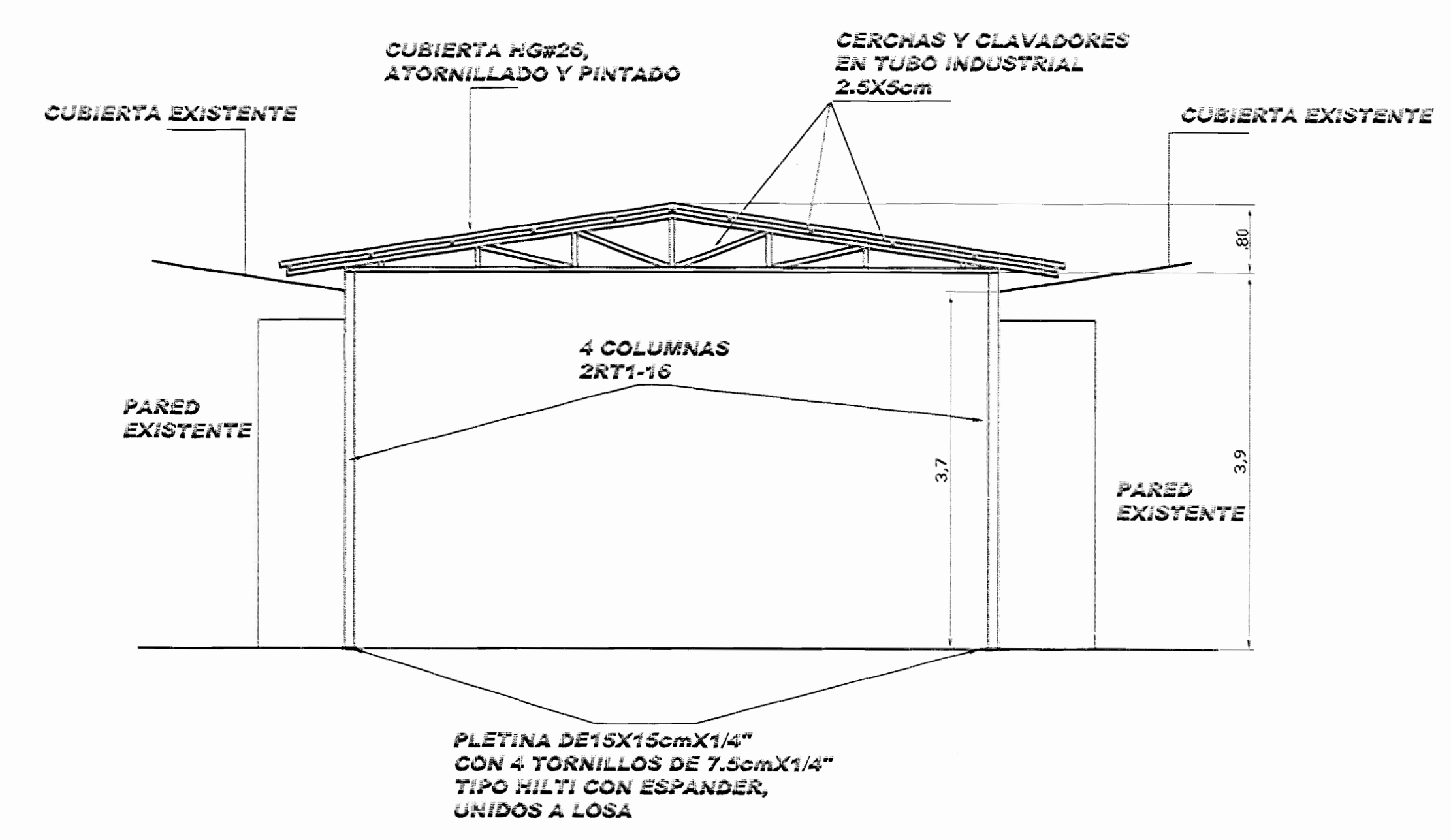
DET. DE TECHO ESC. 1 : 50
