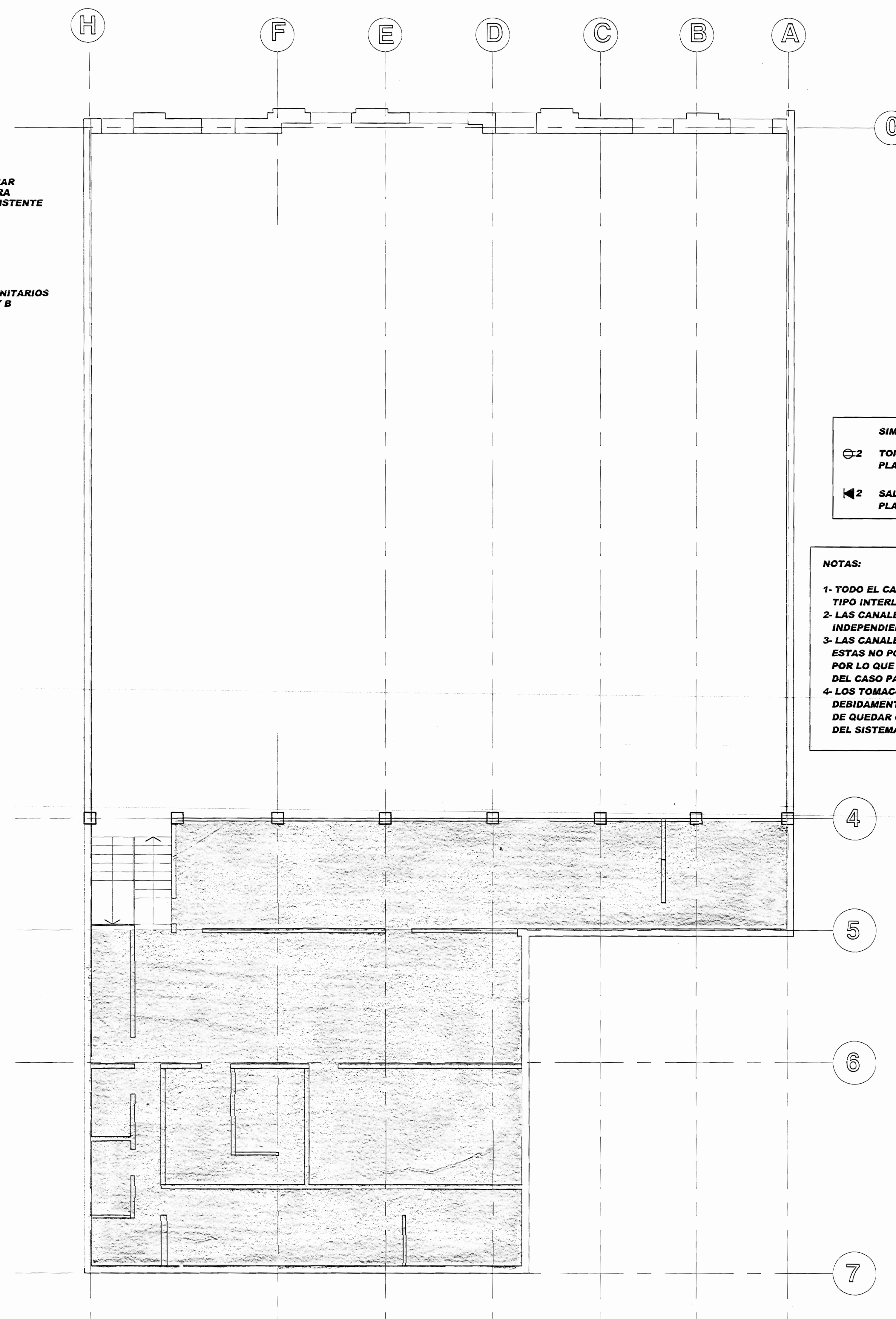
PLANTA CUARTO NIVEL NIVEL 0+5.80
