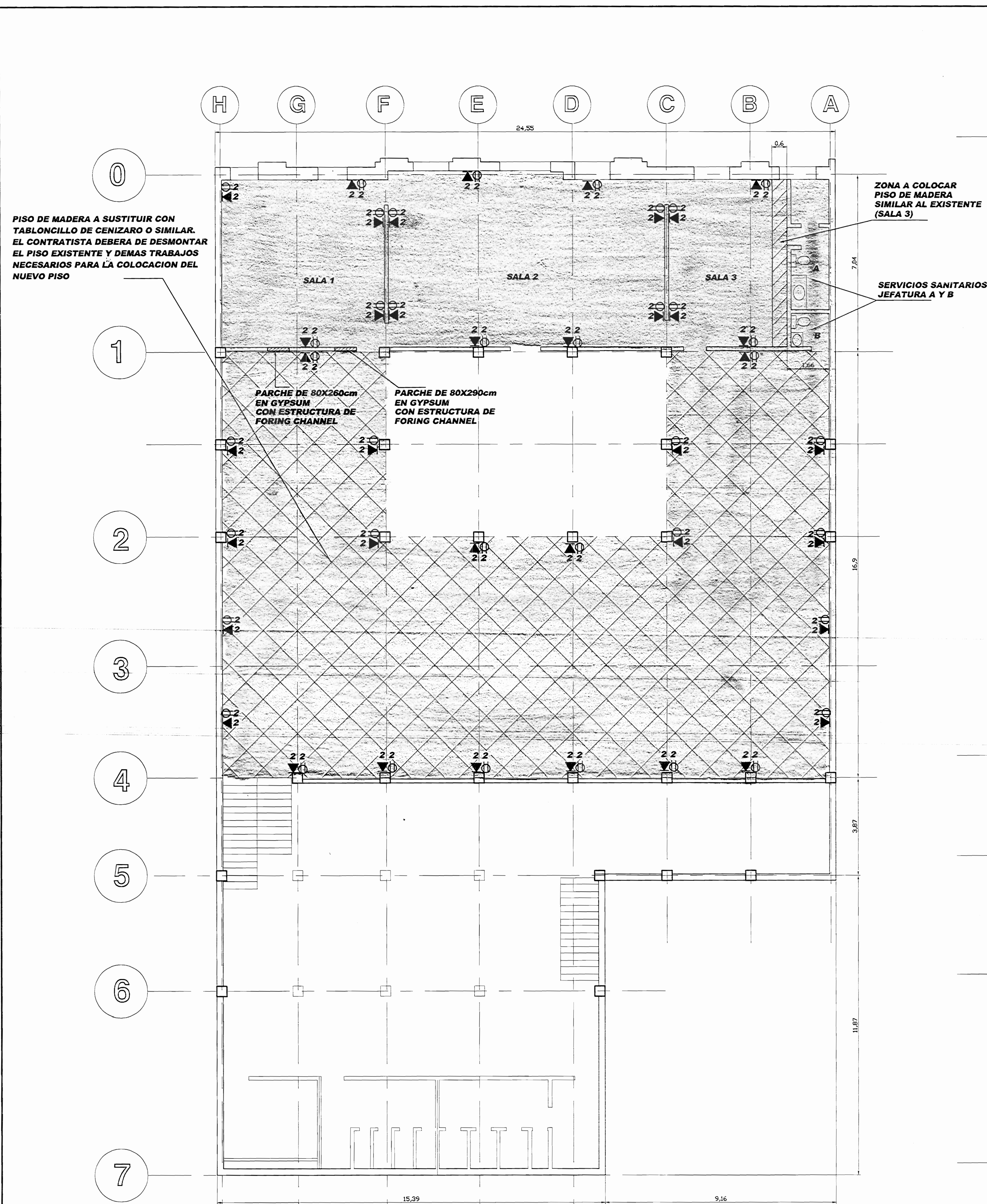
PLANTA TERCER NIVEL NIVEL 0+4.80
