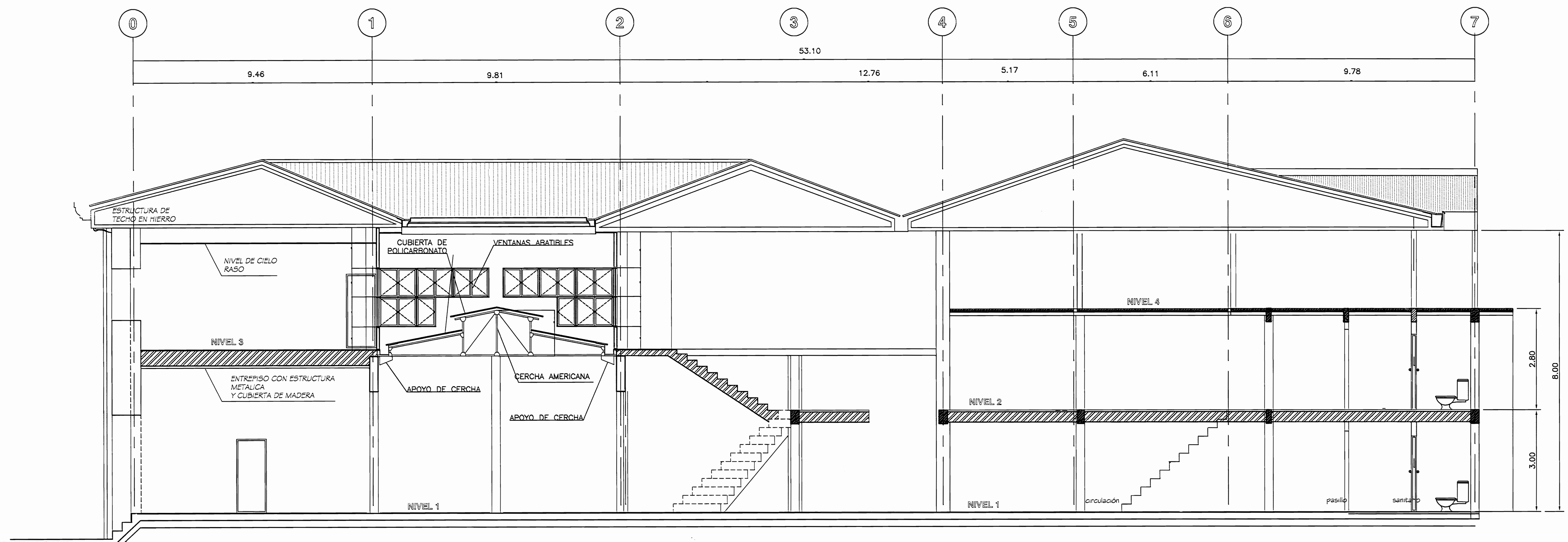
CORTE LONGITUDINAL
