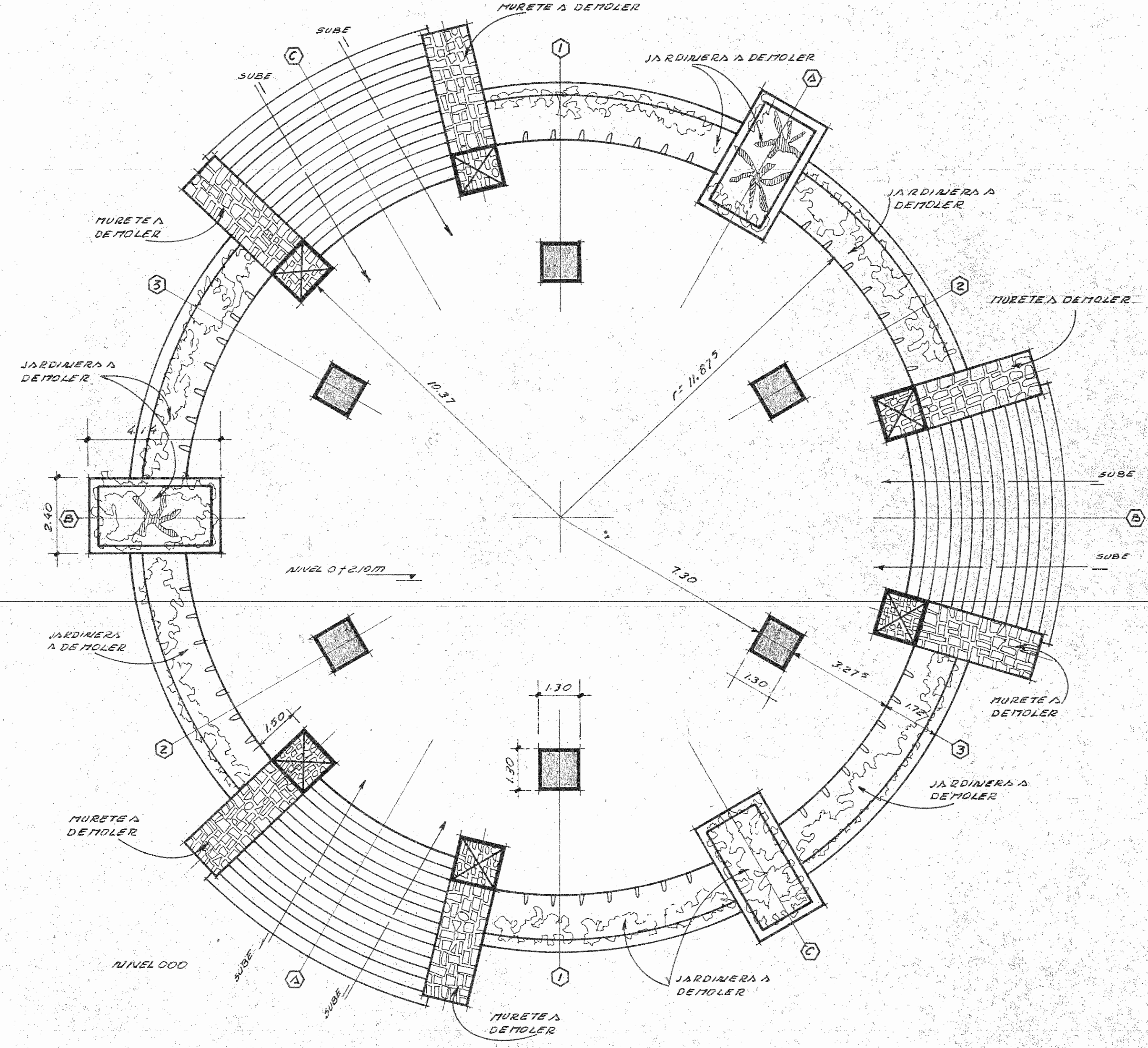
PLANTA ARQUITECTONICA N=0+2.10m Escala 1:100 EXISTENTE.
