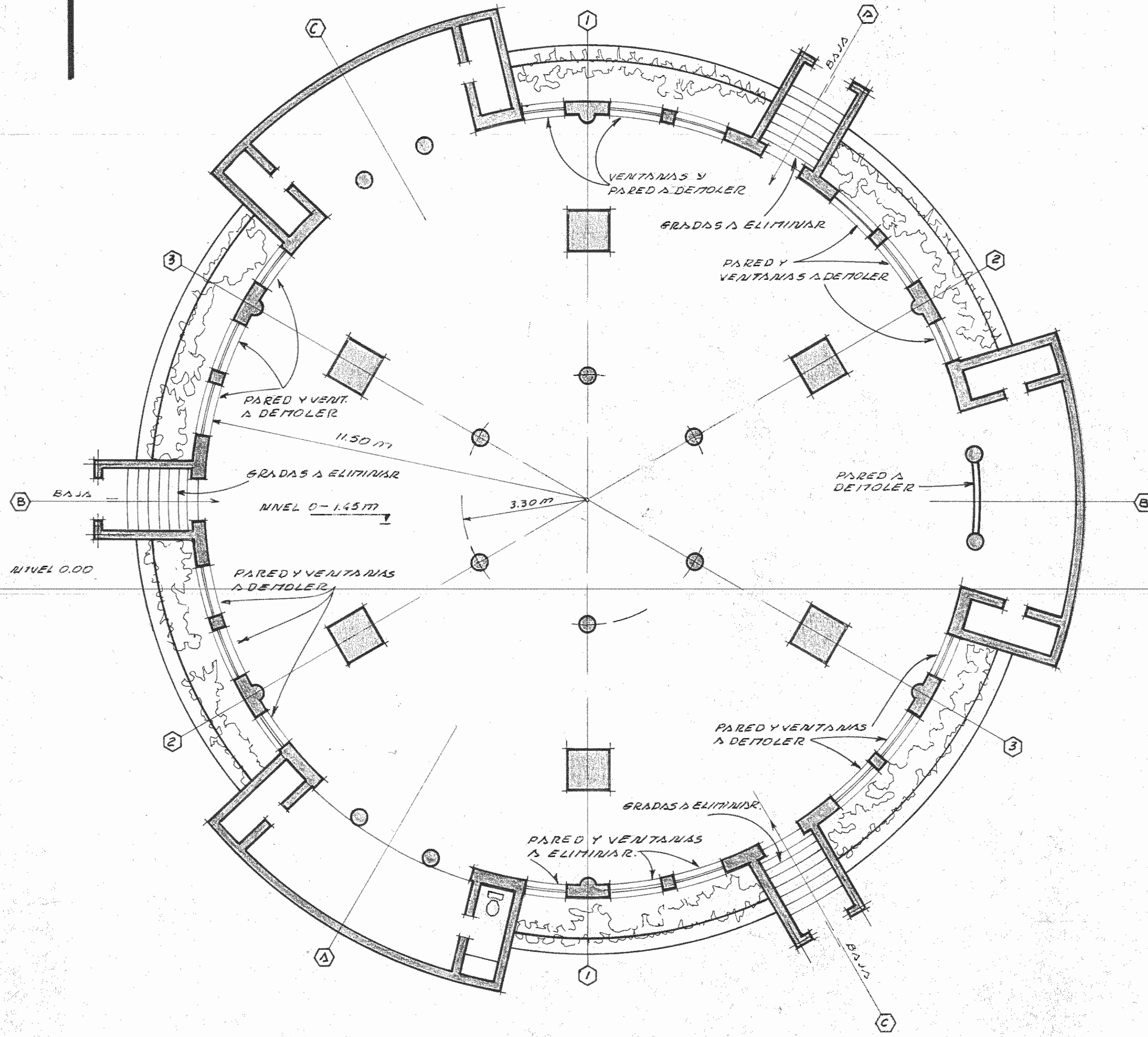
PLANTA ARQUITECTONICA N=0-1.45m Escala 1:100 EXISTENTE. (sotano)
