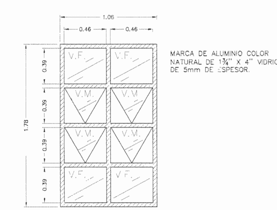
VENTANA TIPO A
