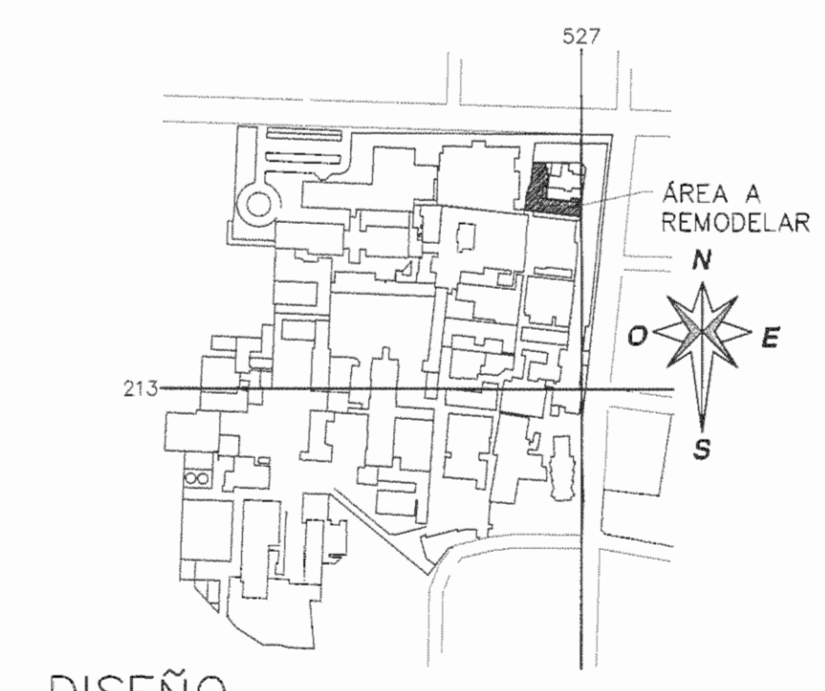
DISEÑO ESCALA 1:4000
