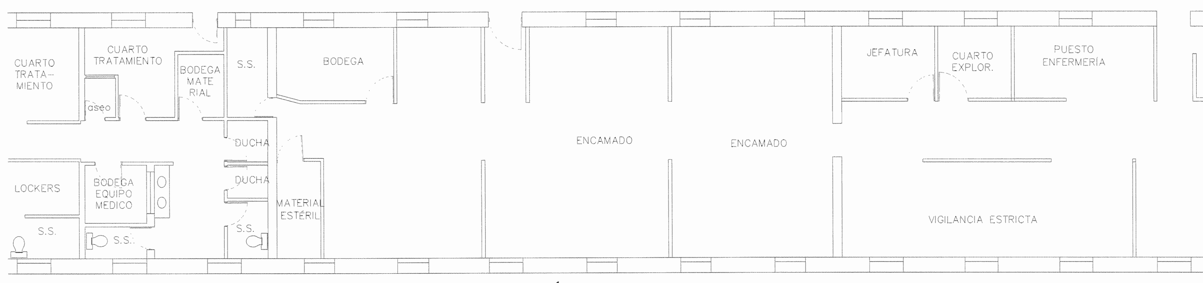
PLANTA DE TUBERIA DE GASES MEDICOS SALÓN DE UROLOGIA - REMODELACION ESCALA 1:75
