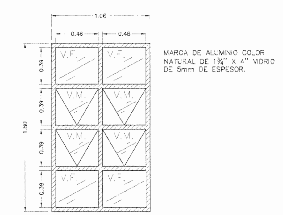
VENTANA TIPO B
