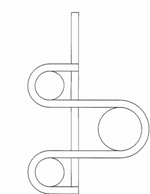
Detalle del soporte vertical para tuberías.
