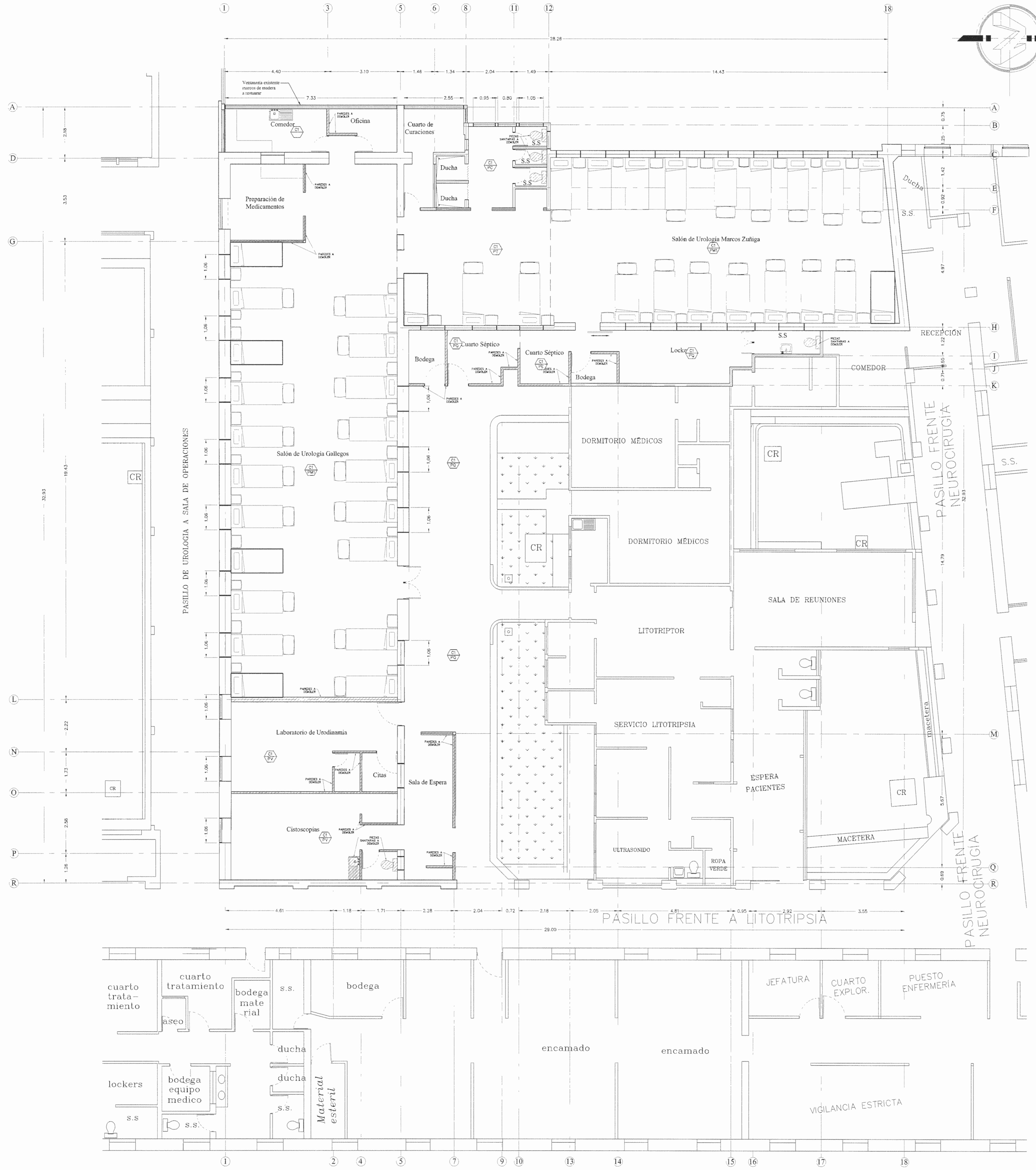
PLANTA ARQUITECTÓNICA SALÓN DE UROLOGÍA - ESTADO ACTUAL ESCALA 1:75
