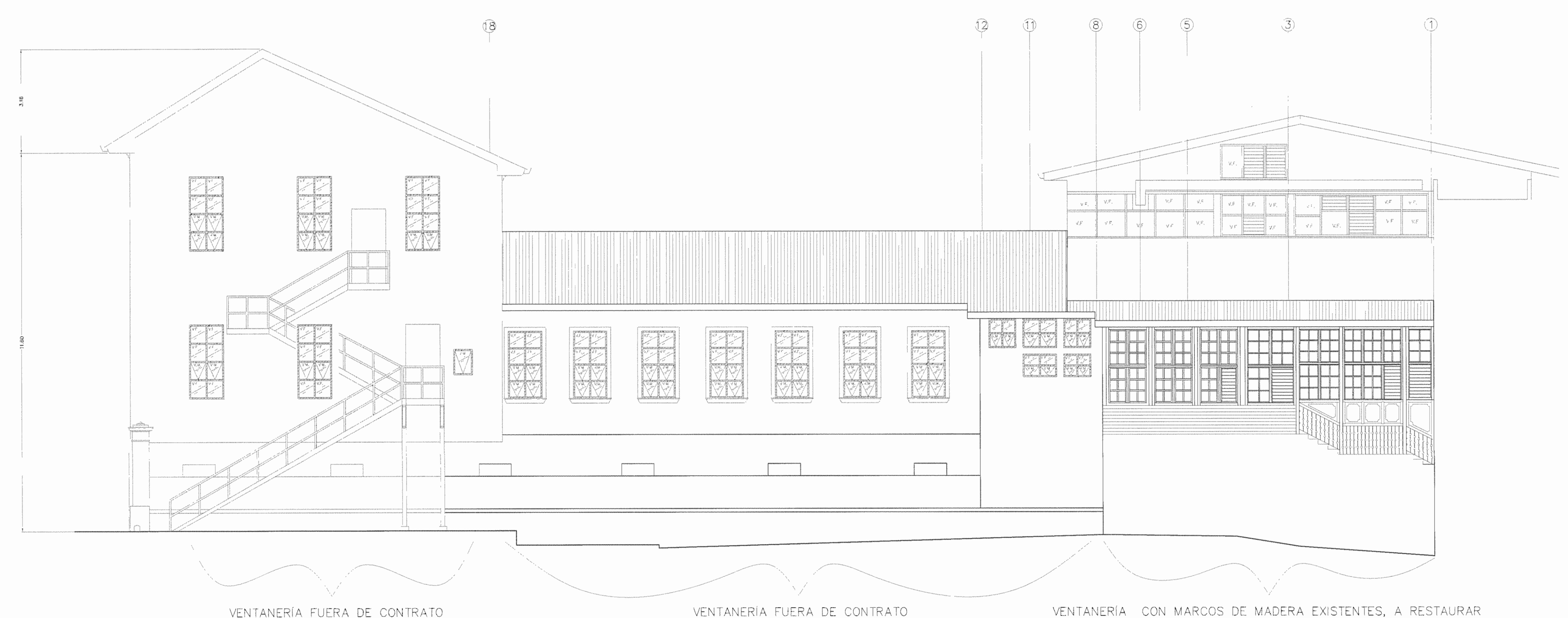
ELEVACIÓN OESTE
