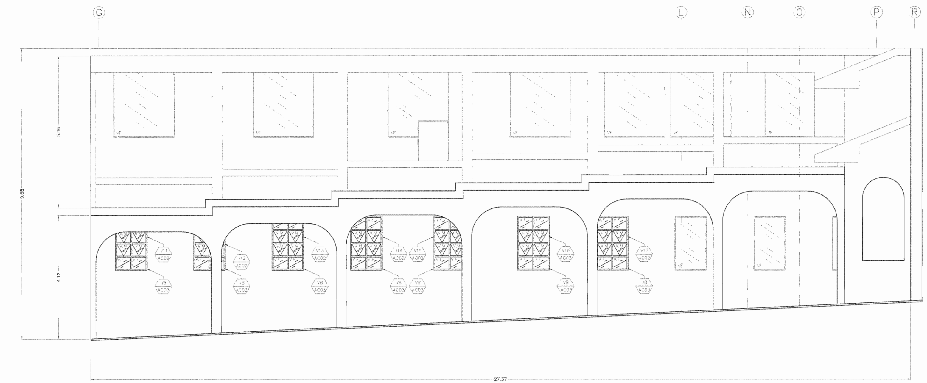
ELEVACIÓN SUR
