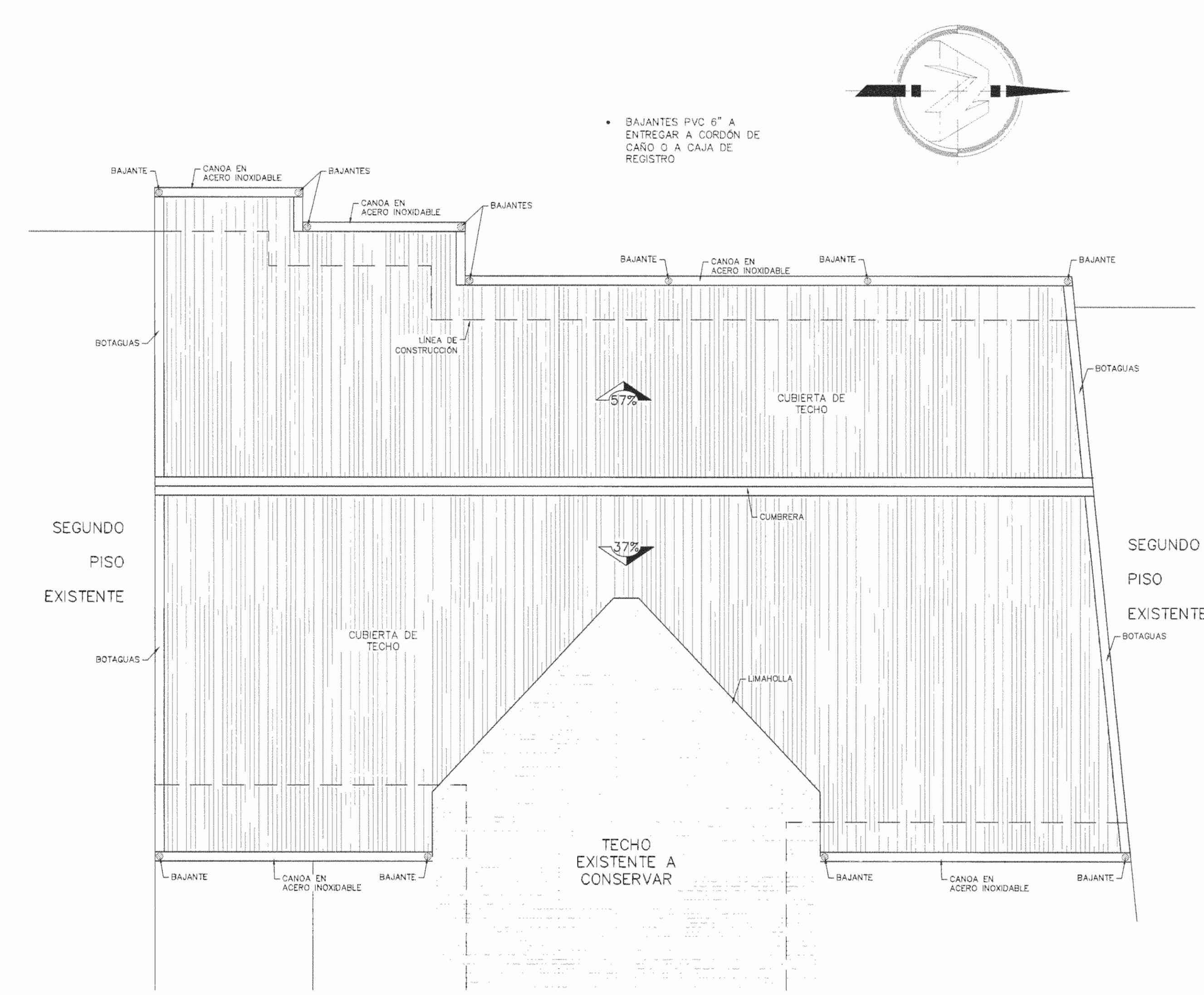
PLANTA DE TECHOS SALÓN DE UROLOGIA - REMODELACION ESCALA 1:75
