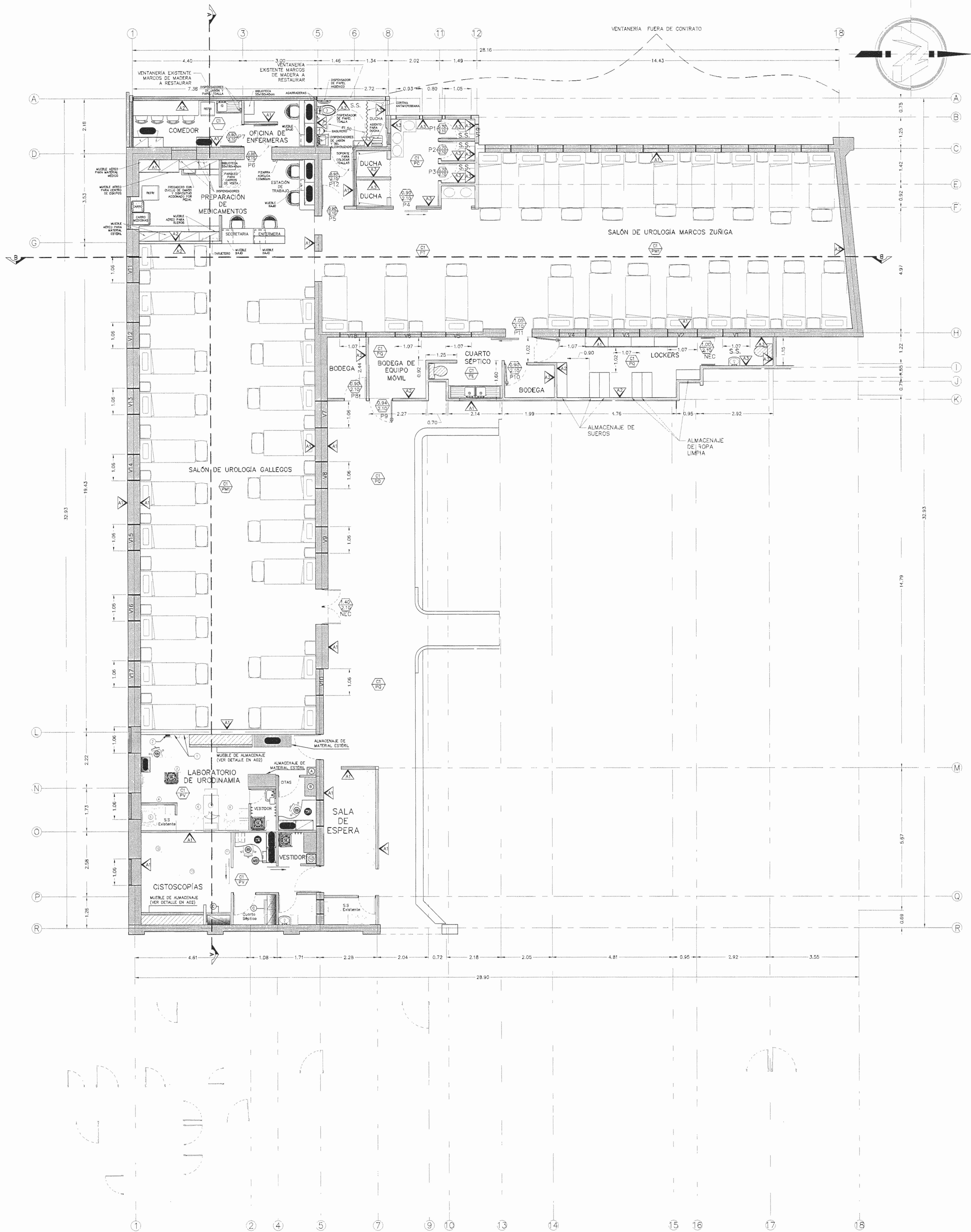
PLANTA ARQUITECTÓNICA SALÓN DE UROLOGIA - REMODELACIÓN ESCALA 1:75
