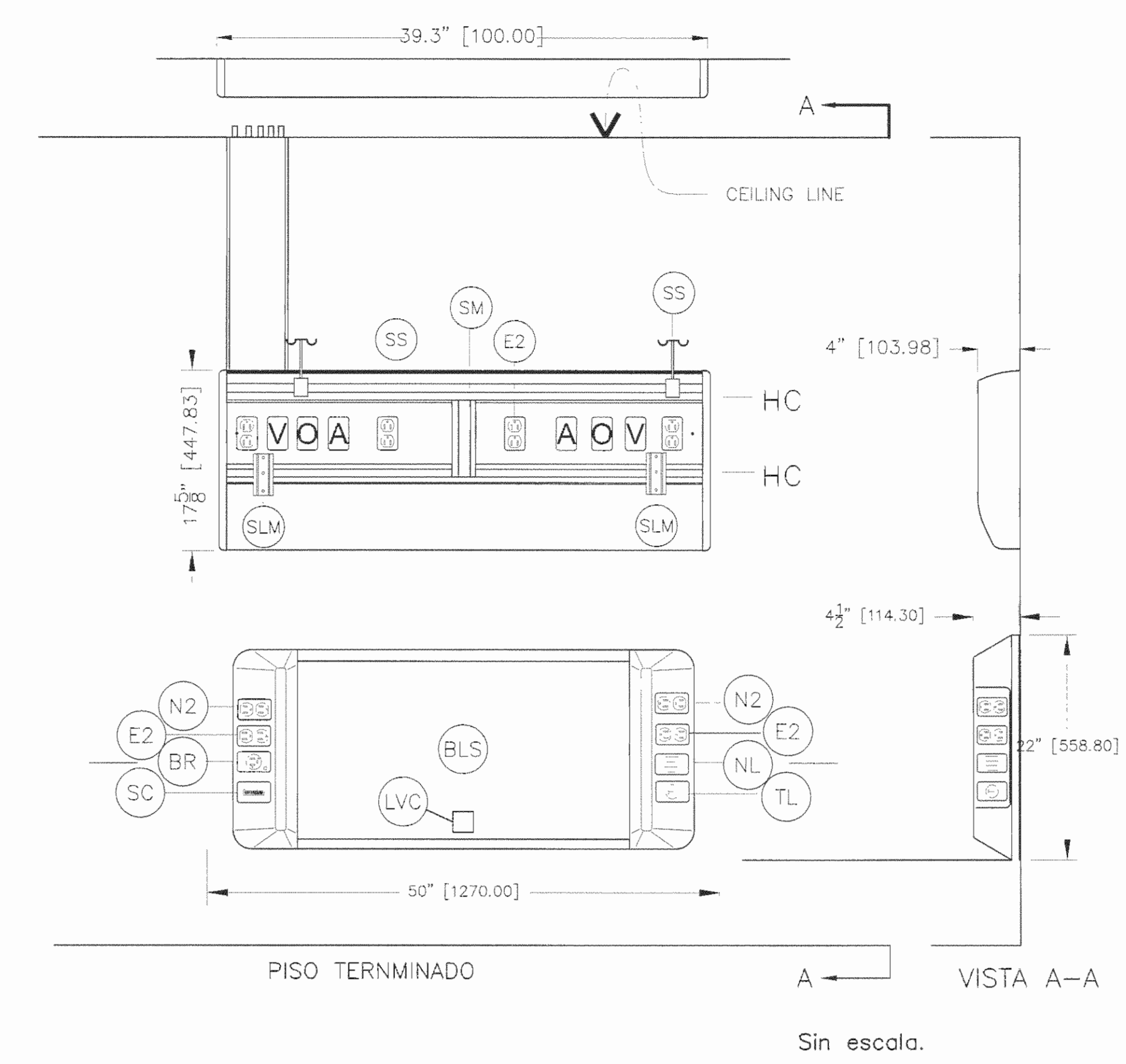
Detalle del panel para gases médicos y el localizador de cama.
