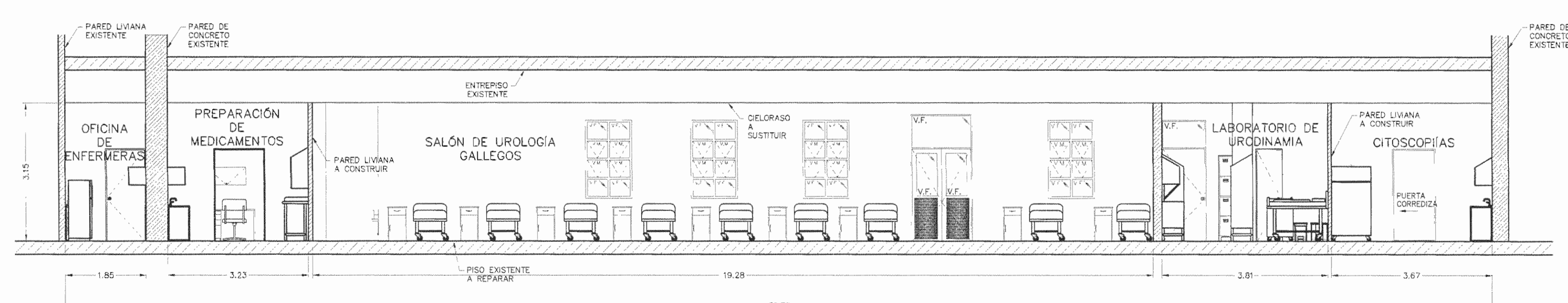
CORTE A-A SALÓN DE UROLOGIA - REMODELACIÓN ESCALA 1:75
