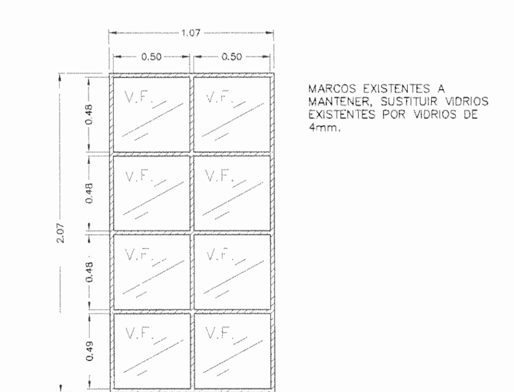
VENTANA TIPO C
