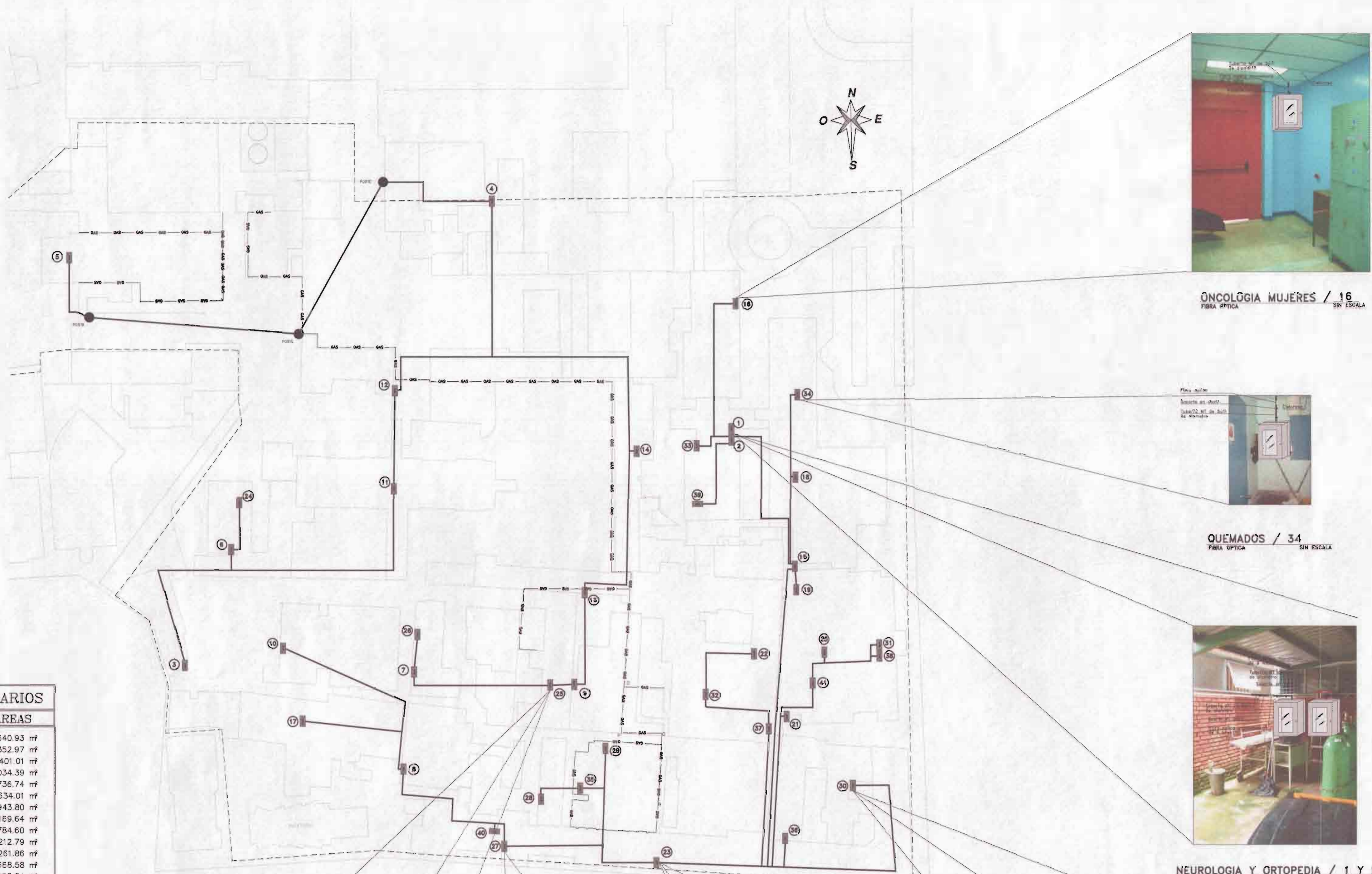
PLANTA DE DISTRIBUCION DE RACKS FIBRA OPTICA / HOSPITAL SAN JUAN DE DIOS ESCALA 1:750
