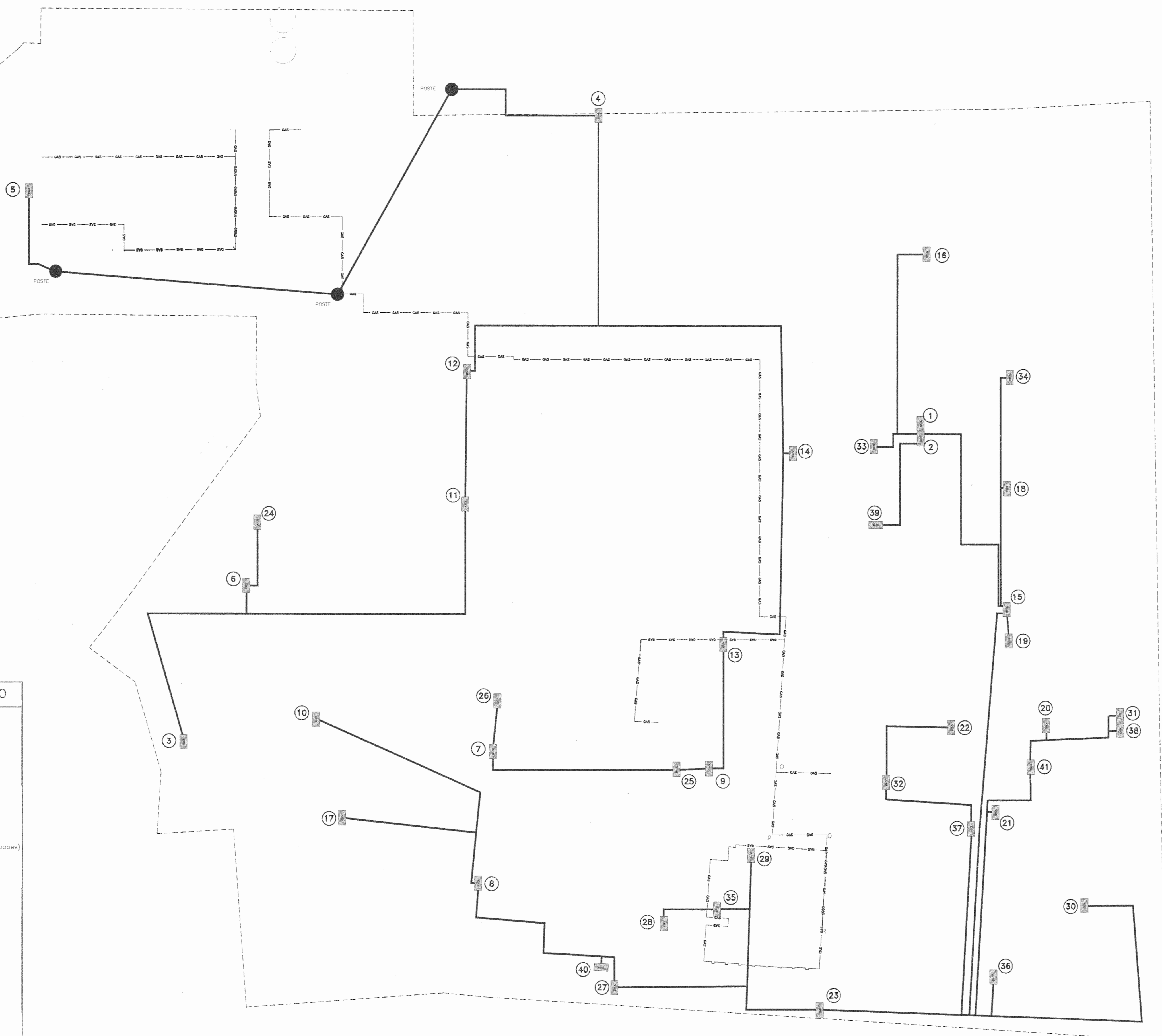
PLANTA DE DISTRIBUCION DE RACKS FIBRA OPTICA / HOSPITAL SAN JUAN DE DIOS
