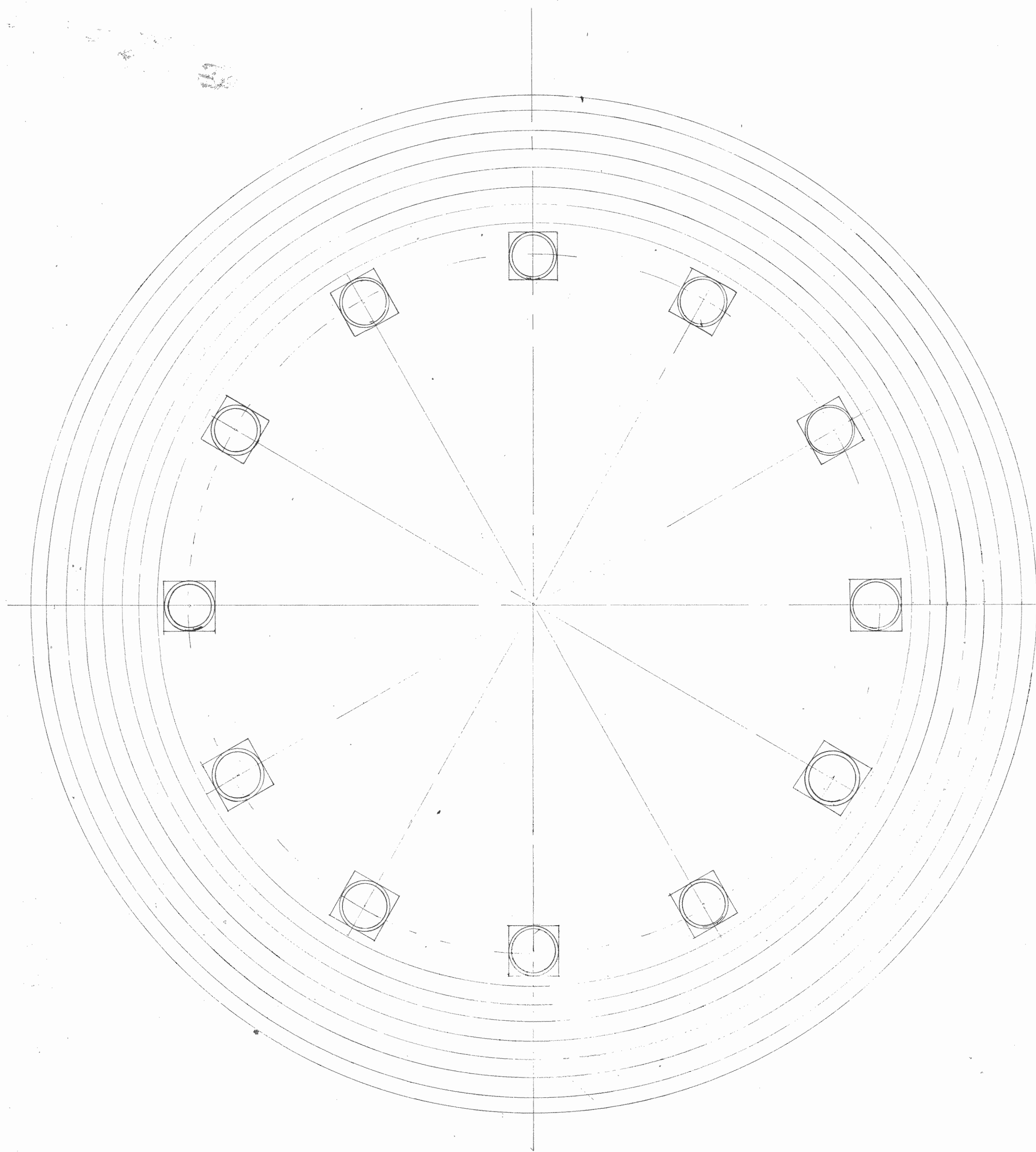
PLANTA ESCALA 1:50
