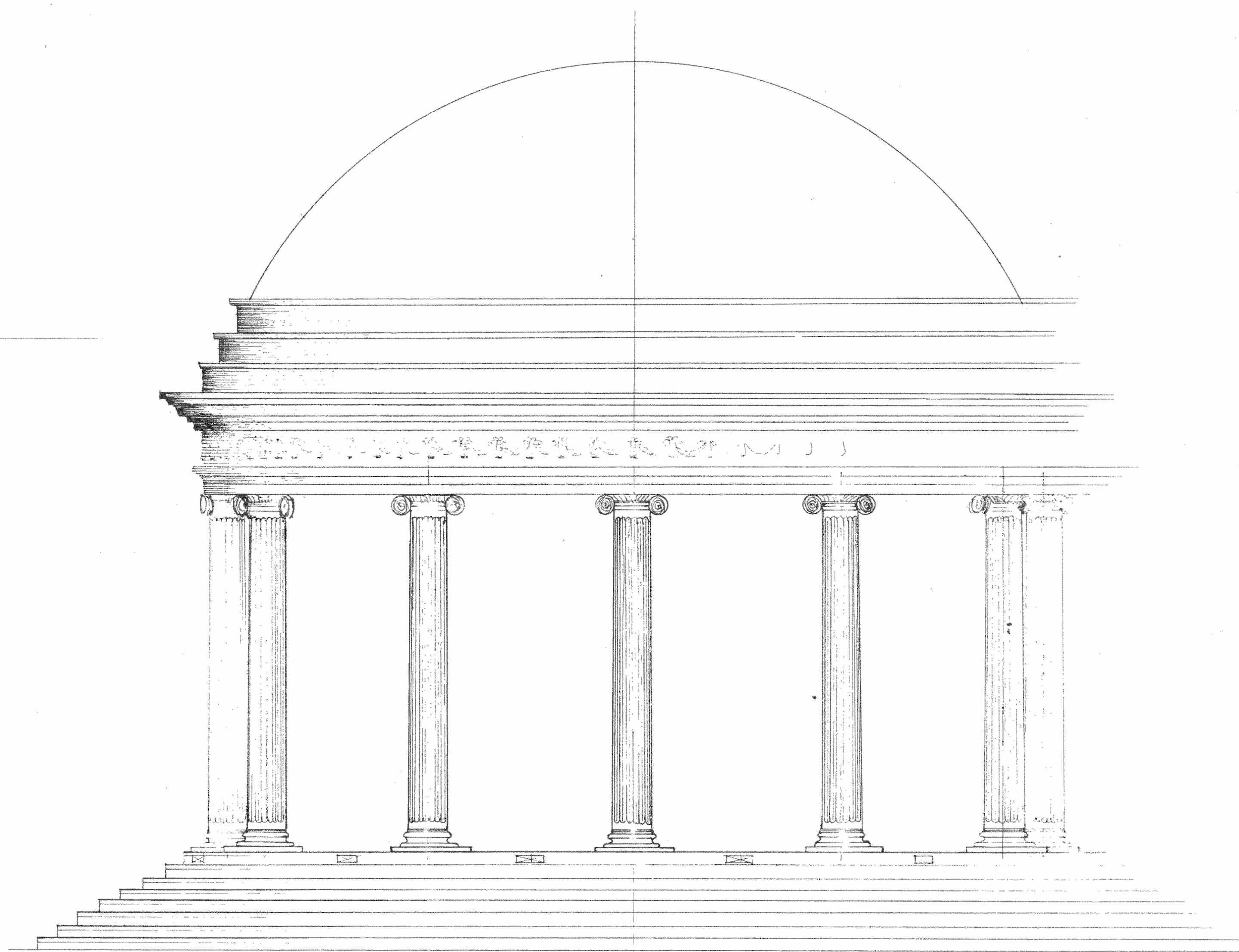
ELEVACION ESCALA 1:50
