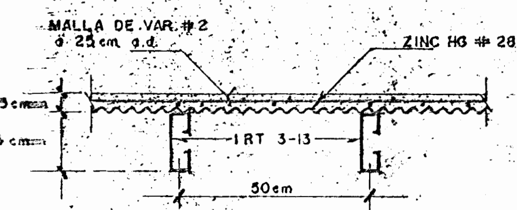
DET. DE ENTREPISO
