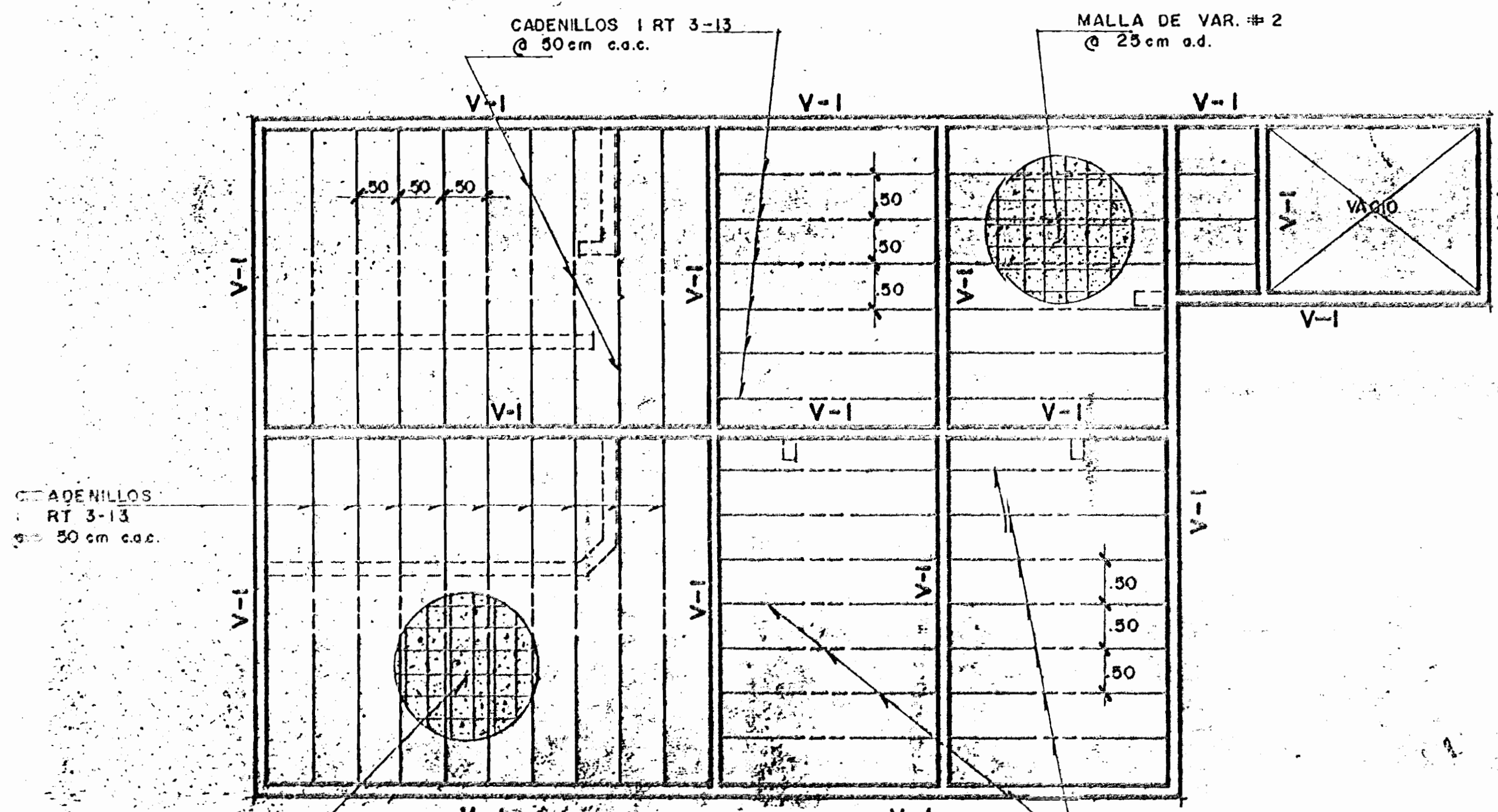
PLANTA DE ENTREPISO
