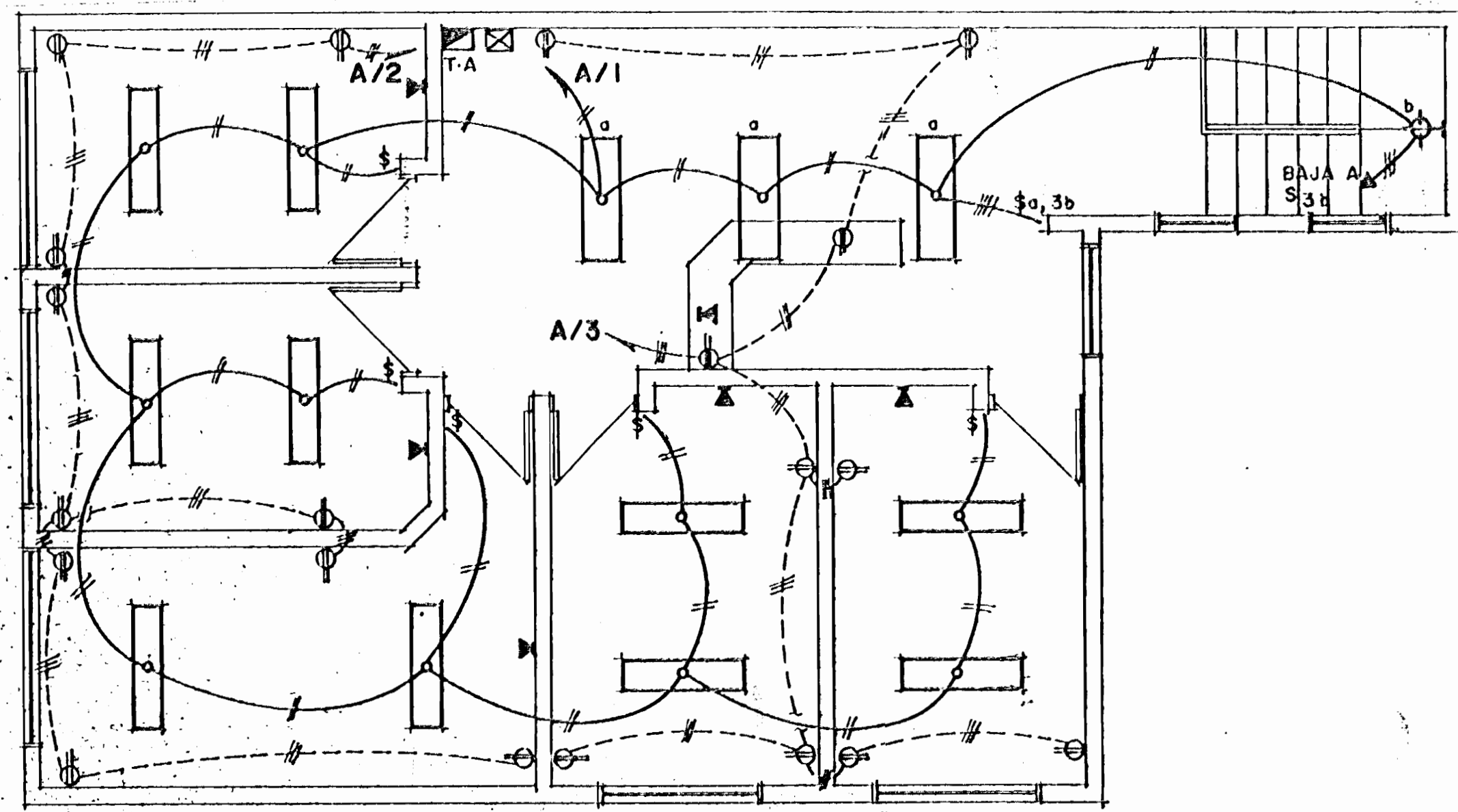
SISTEMA ELECTRICO PLANTA ALTA
