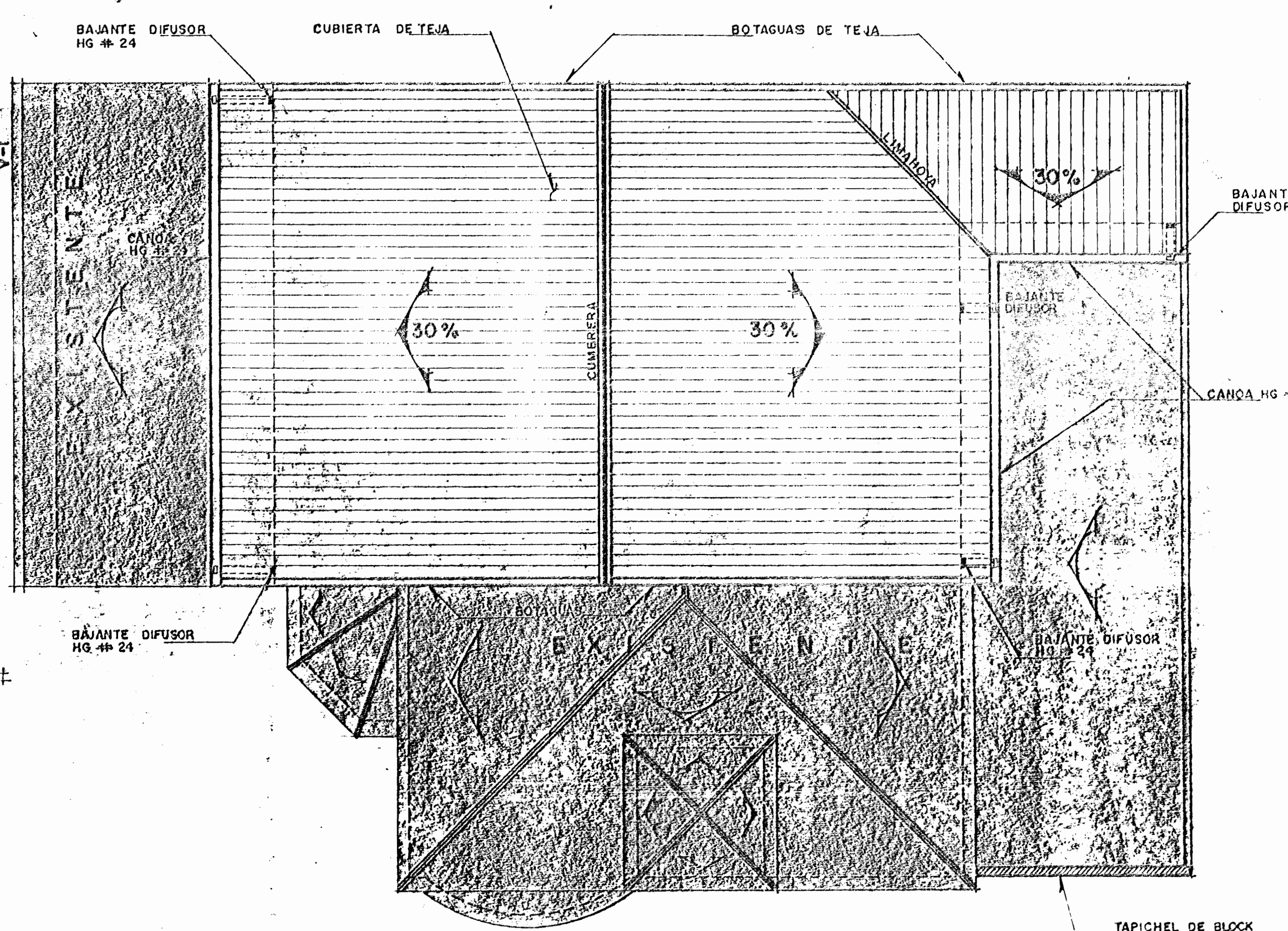
PLANTA DE TECHOS
