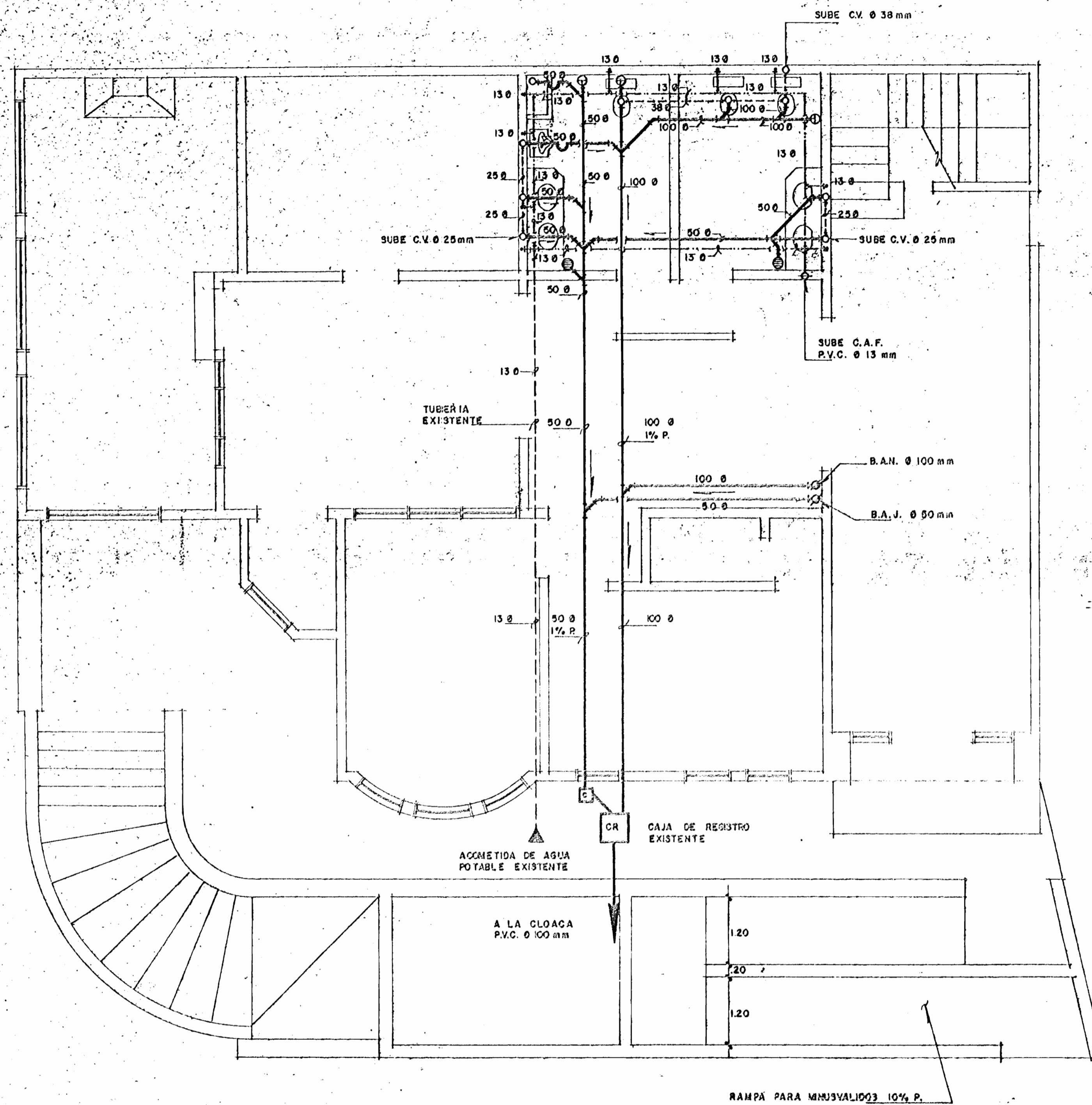
PLANTA SISTEMA MECANICO
