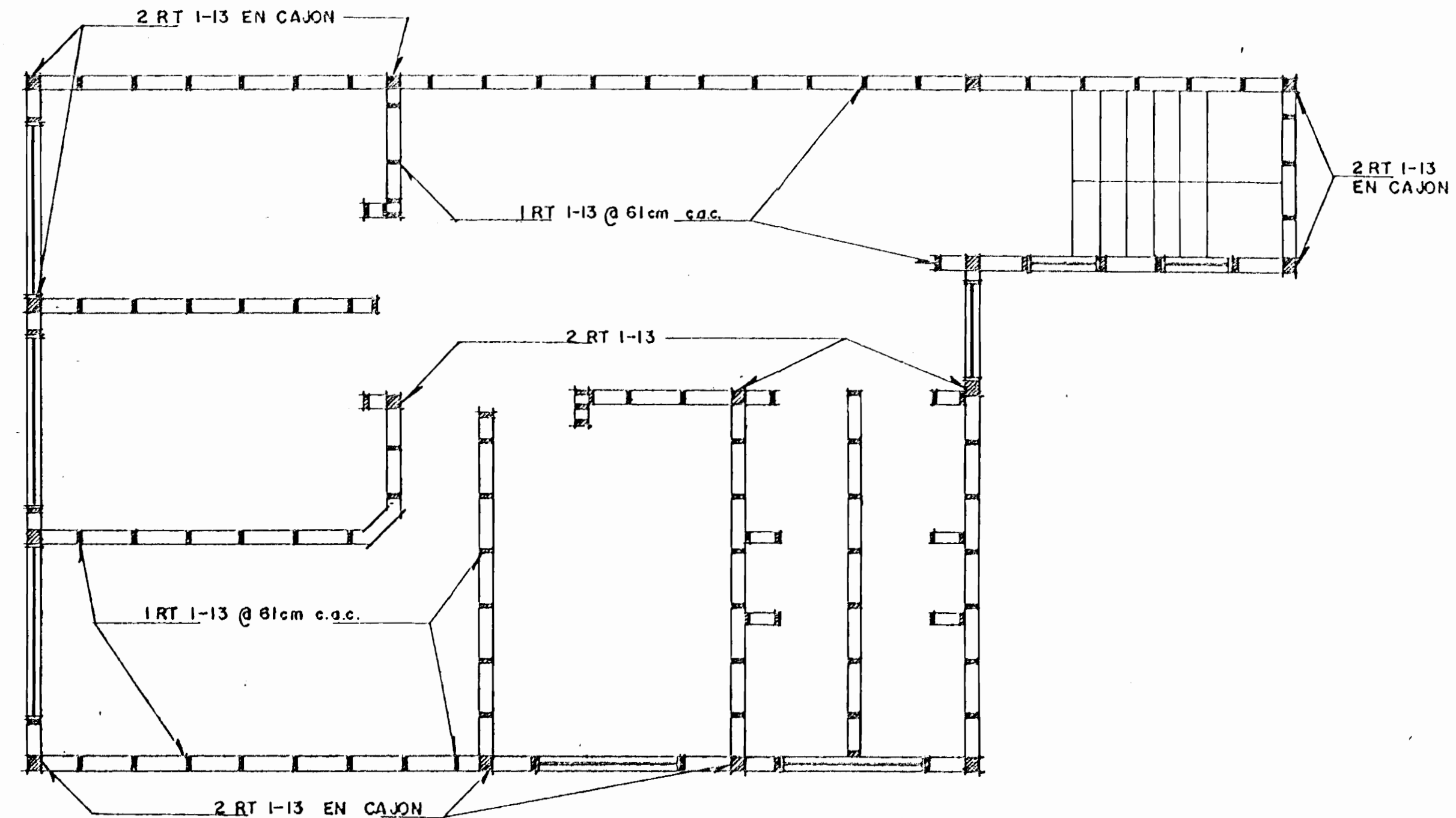
PLANTA ALTA ESTRUCTURAL
