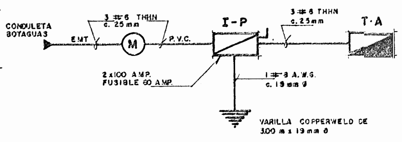
DIAGRAMA UNIFILAR ELECTRICO
