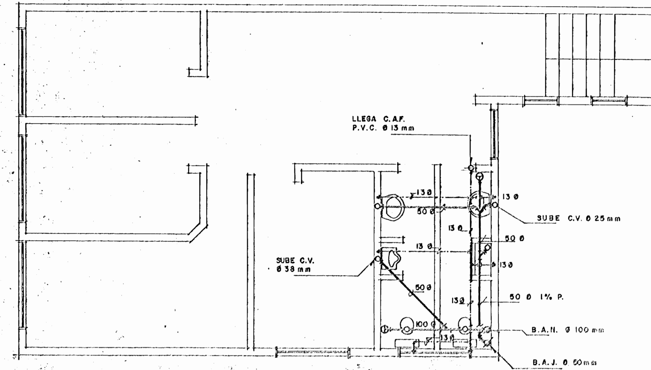
PLANTA ALTA SISTEMA MECANICO
