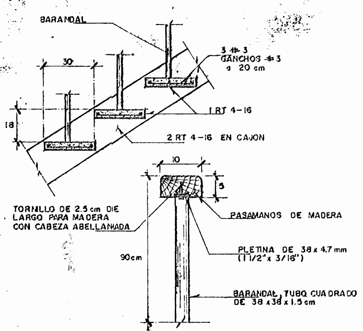
DET. DE ESCALERA
