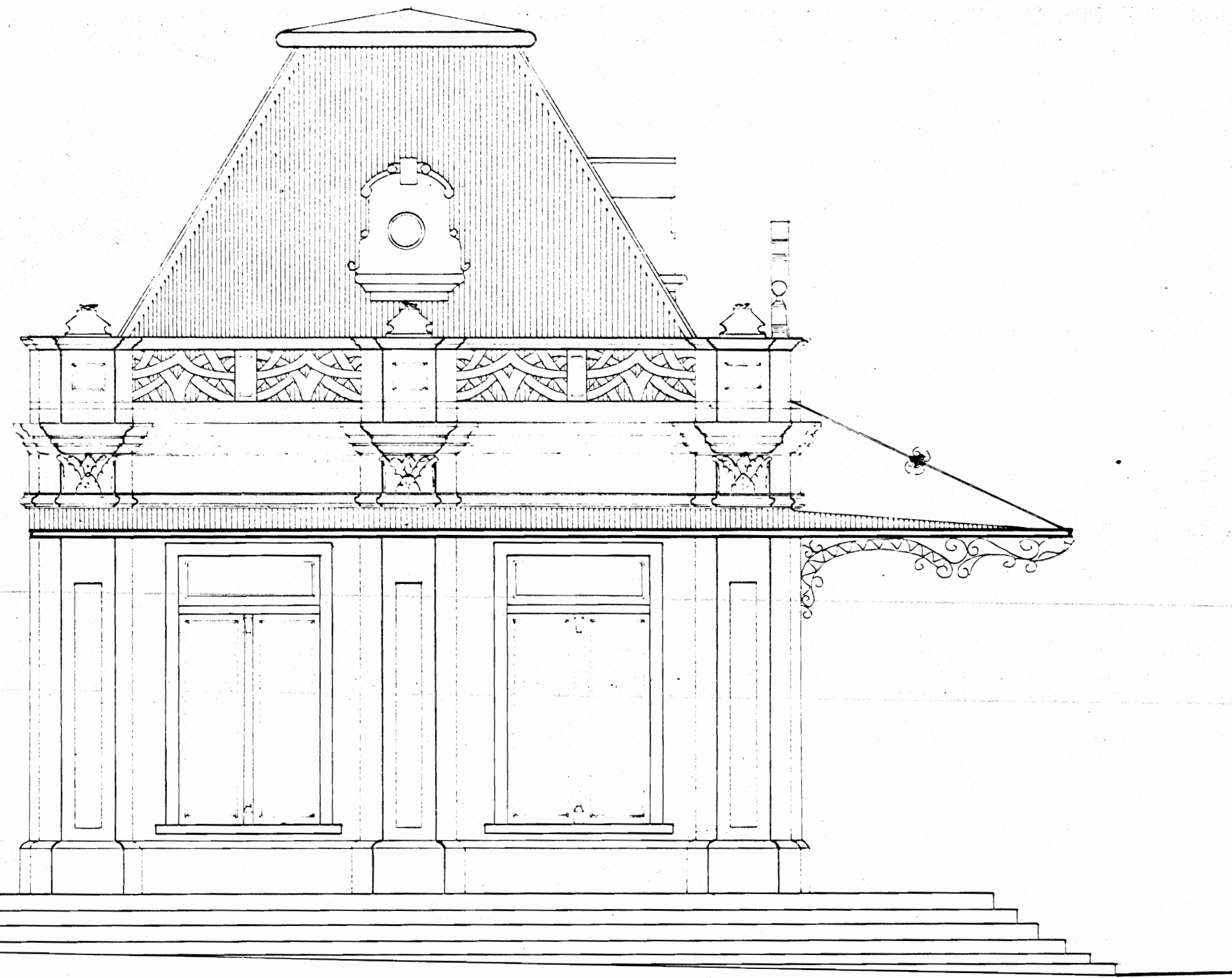
FACHADA OESTE Escala 1:50
