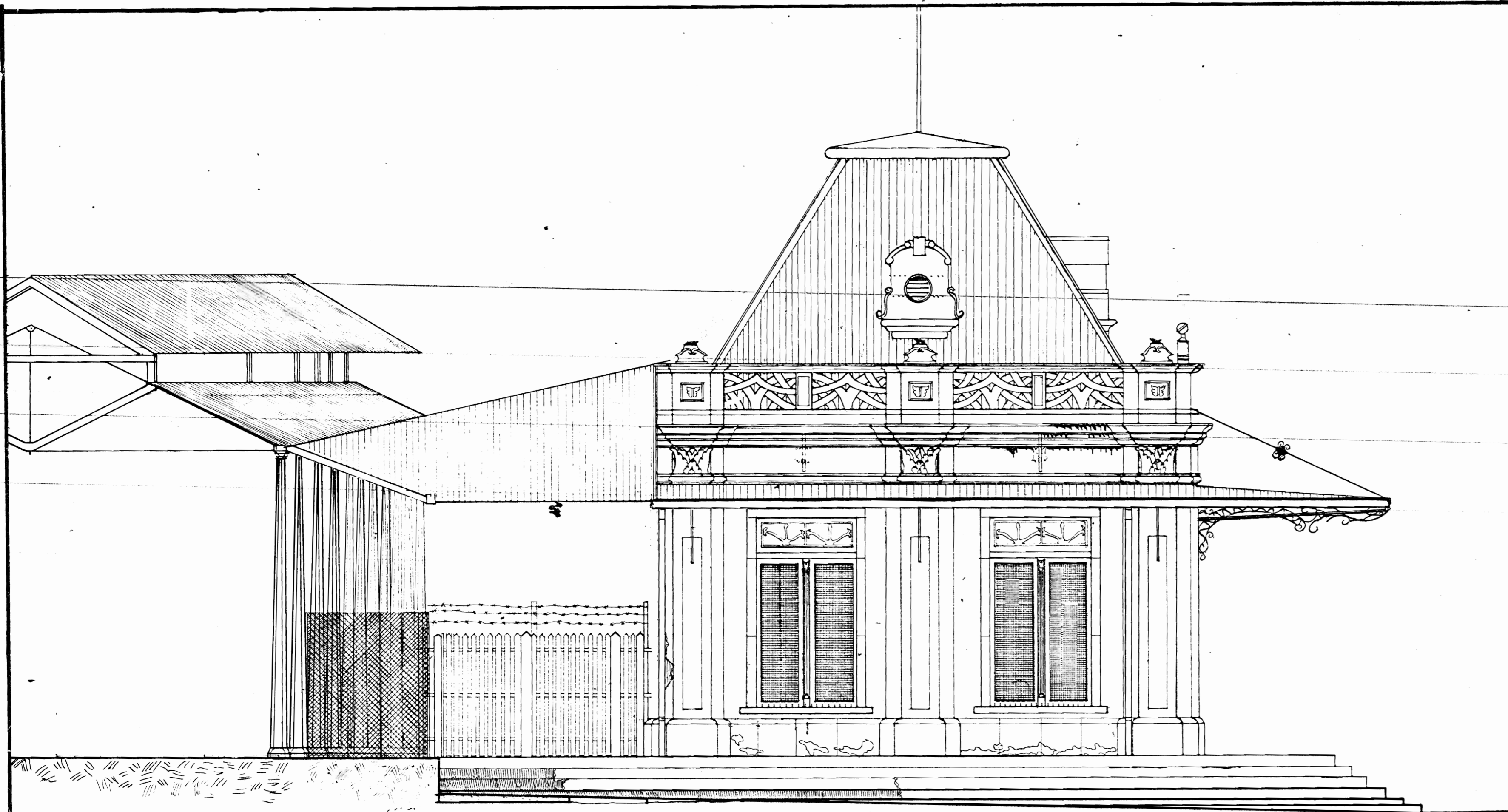
FACHADA OESTE ESTADO ACTUAL Escala 1:50
