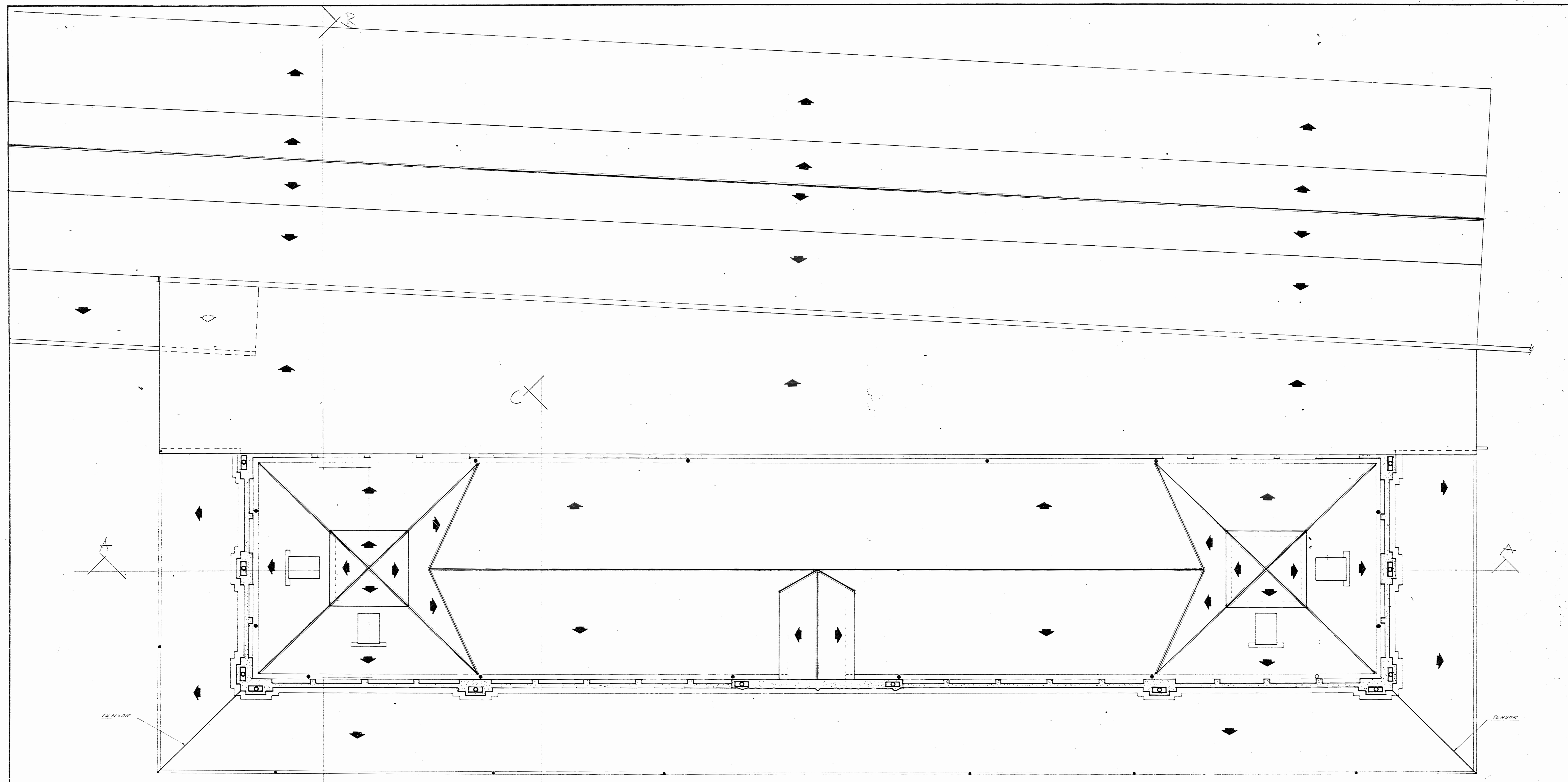
PLANTA DE TECHOS ESTADO ACTUAL Escala 1:50
