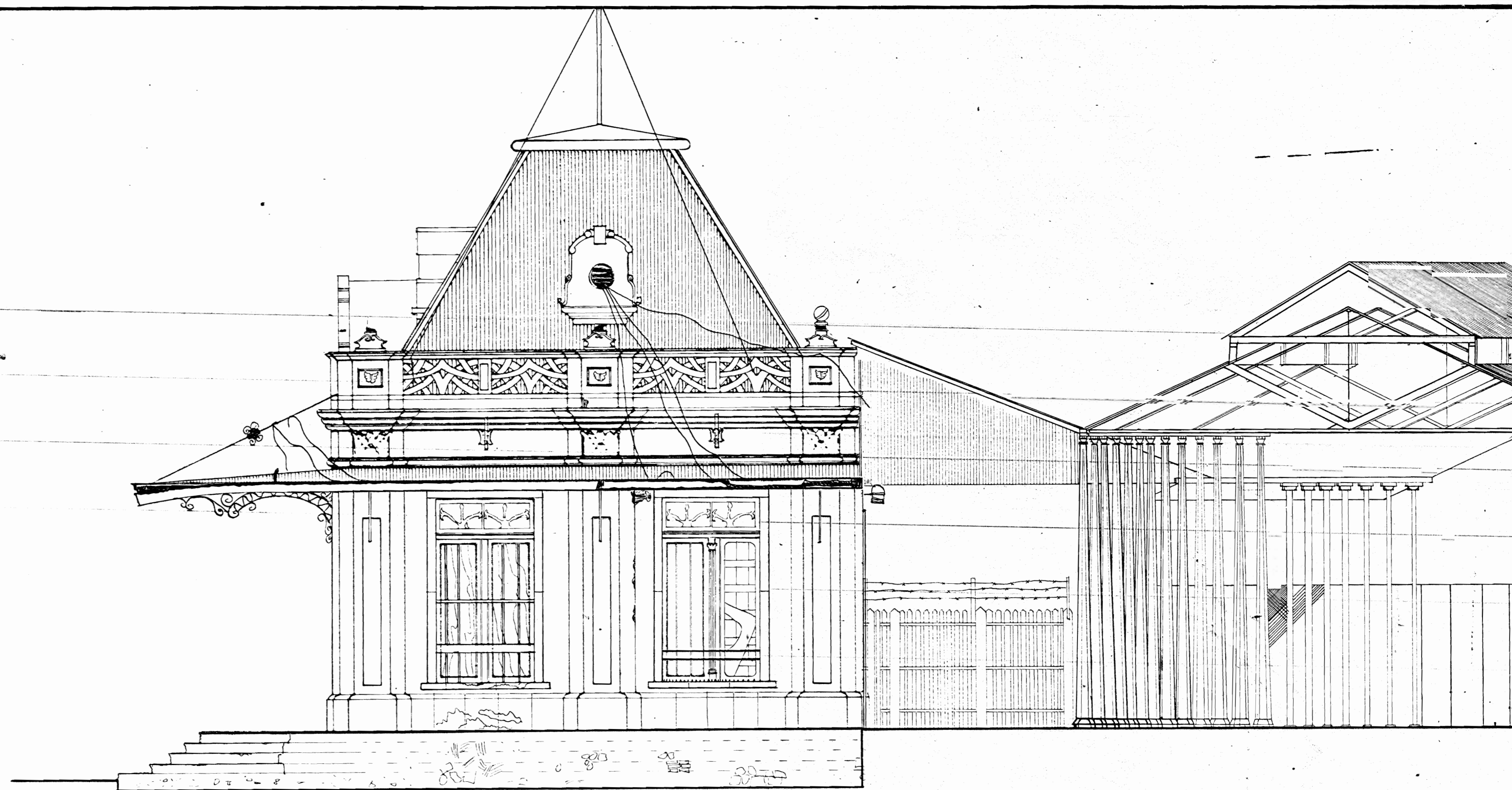
FACHADA ESTE ESTADO ACTUAL Escala 1:50
